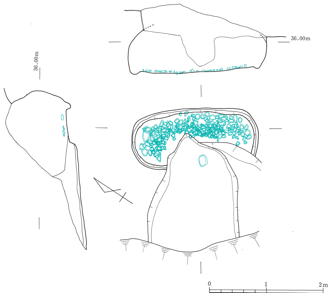
第431図 79号横穴墓平・断面図
