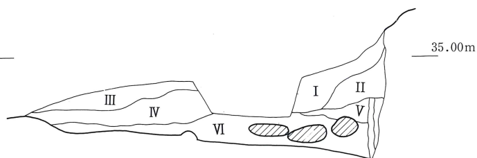
第421図 75号横穴墓平・断面図及び縦断土層図
