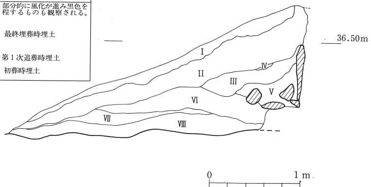
第422図 76号横穴墓縦断土層図
