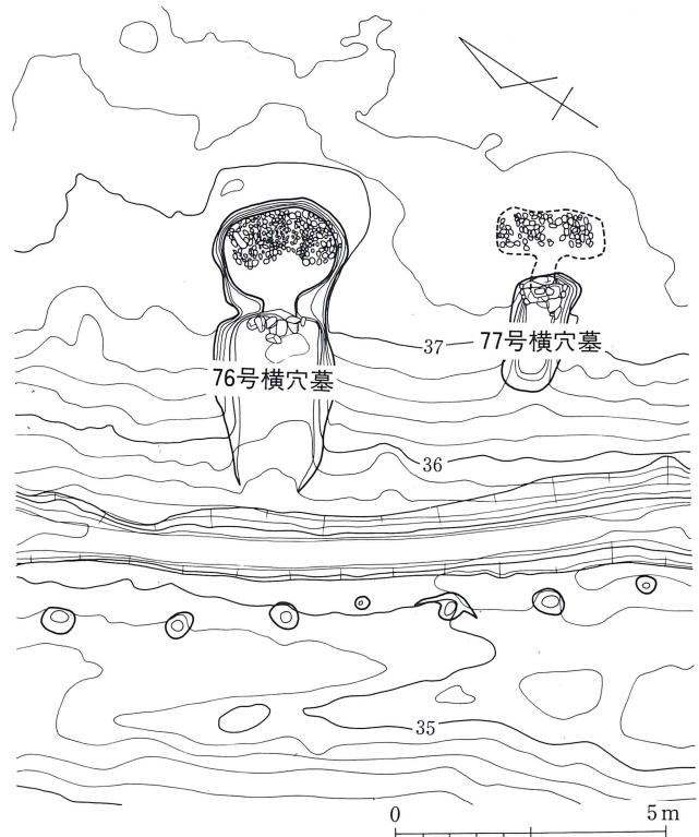
第425図 77号横穴墓周辺平面図
