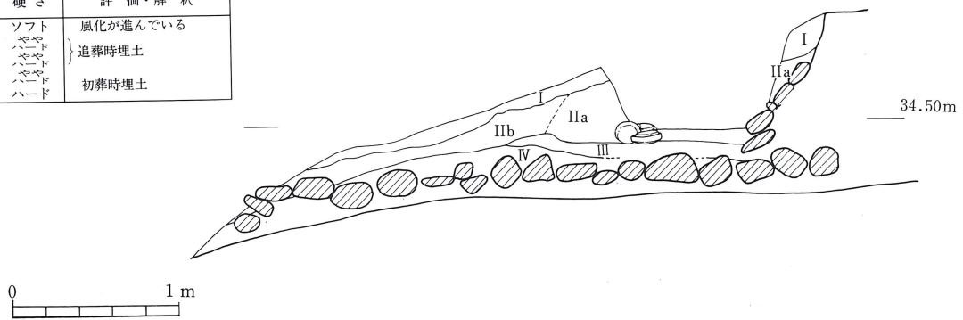
第415図 73号横穴墓縦断土層図
