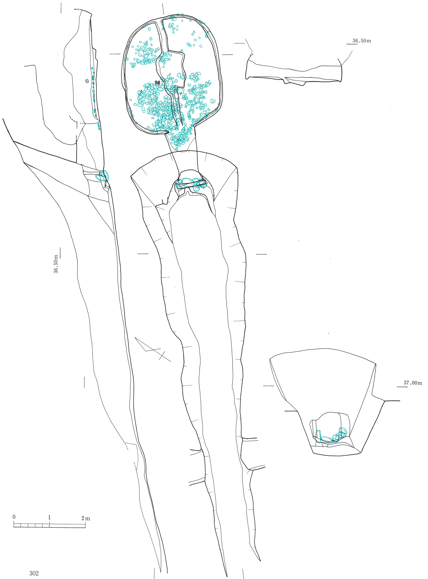
第419图 74号横穴墓平·断面图
