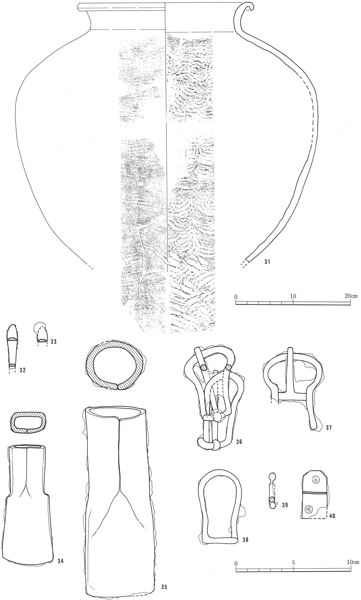
第438图 80号横穴墓出土遗物实测图(4)
