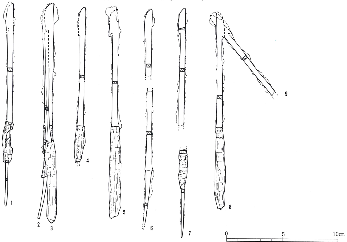
第424図 76号横穴墓出土遺物実測図
