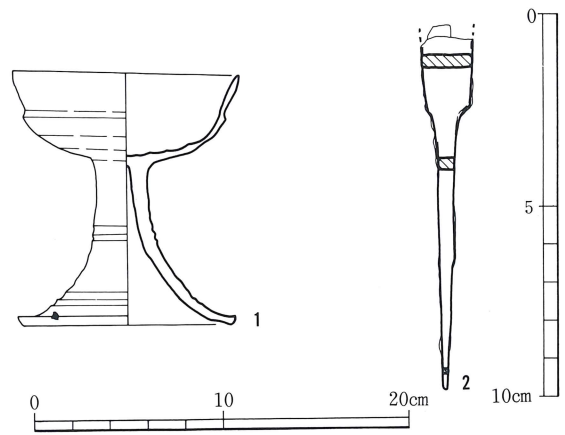
第420図 74号横穴墓出土遺物実測図
