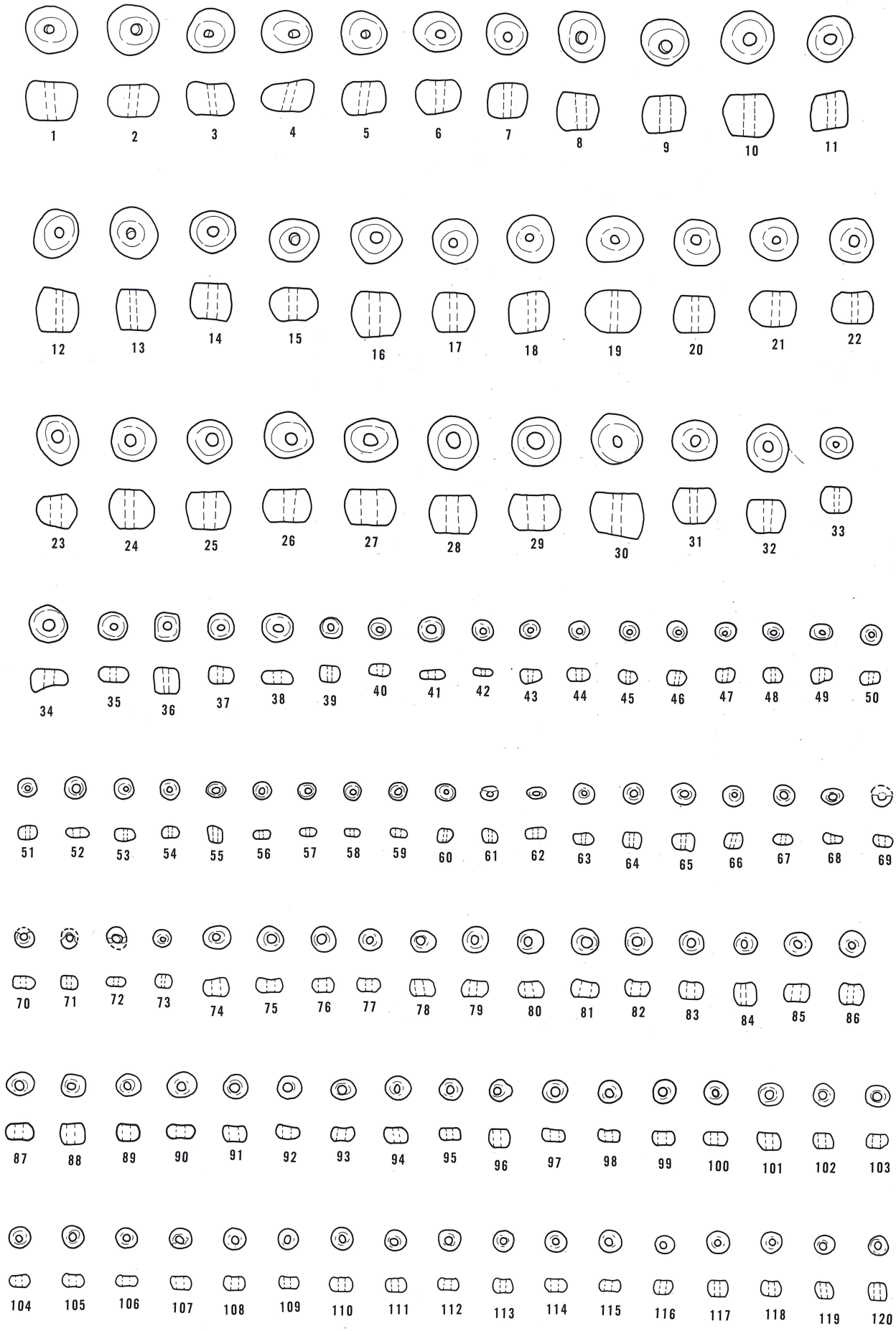
第428图 78号横穴墓出土遗物实测图(1)
