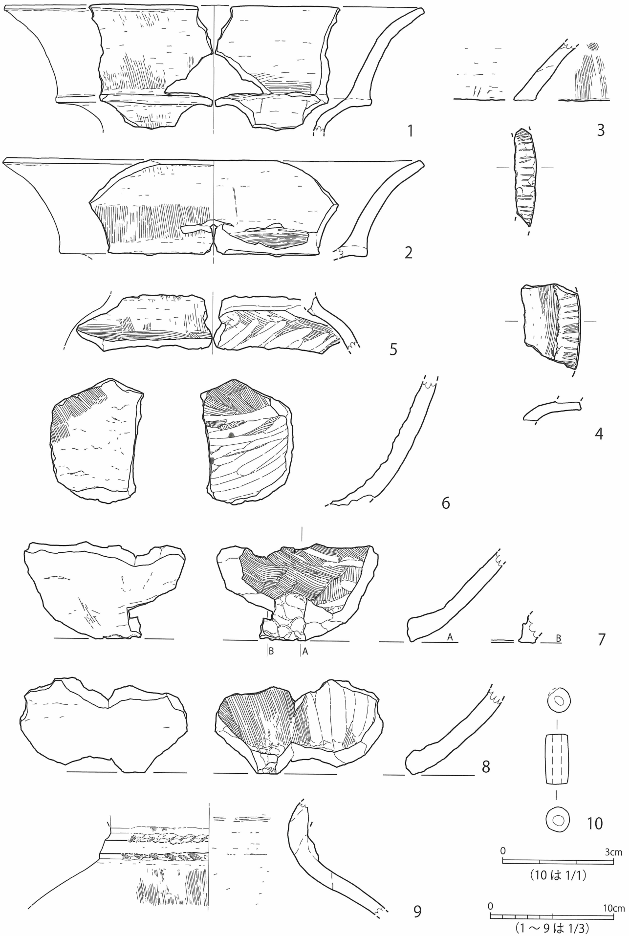
第2図 横尾貝塚出土遺物実測図
