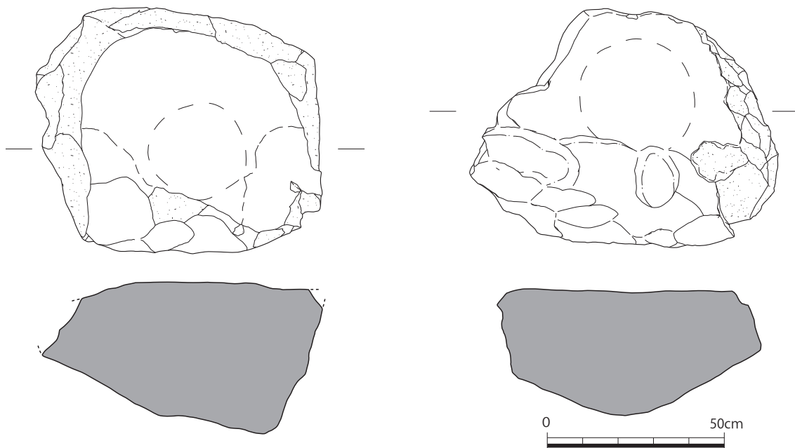
第7-260図 10-SE271出土遺物実測図①(礎石、1/15)
