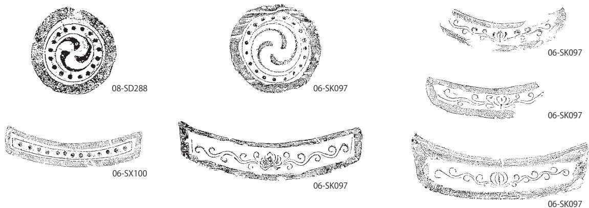
I期 (14世紀前半) の瓦=創建期 (1/6)
