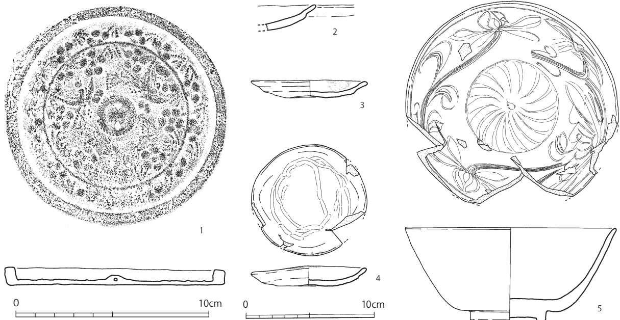
第7-268図 10-ST155出土遺物実測図 (1/2、1/3)
