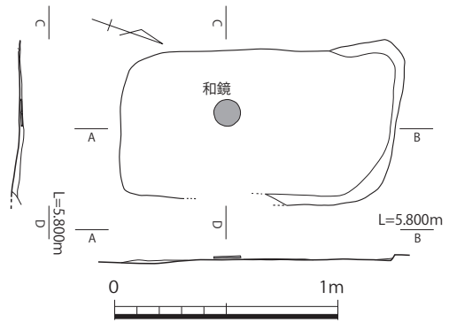
第7-267図 10-ST155実測図 (1/30)
