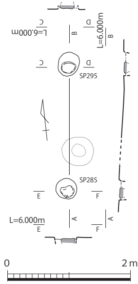
第7-271図 10-SP285・10-SP295実測図 (1/60)
