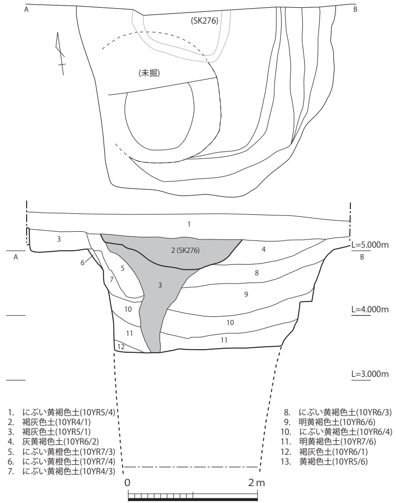
第7-263図 10-SE278実測図 (1/60)
