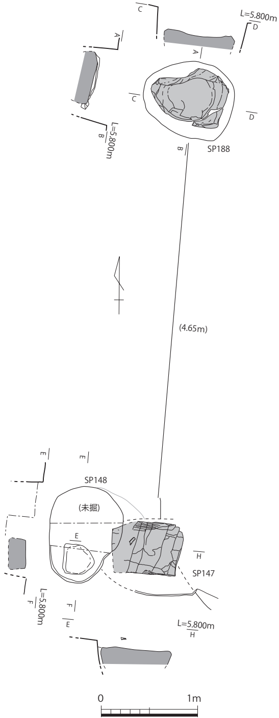
第7-269図 10-SP147・10-SP148・10-SP188実測図(1/40)
