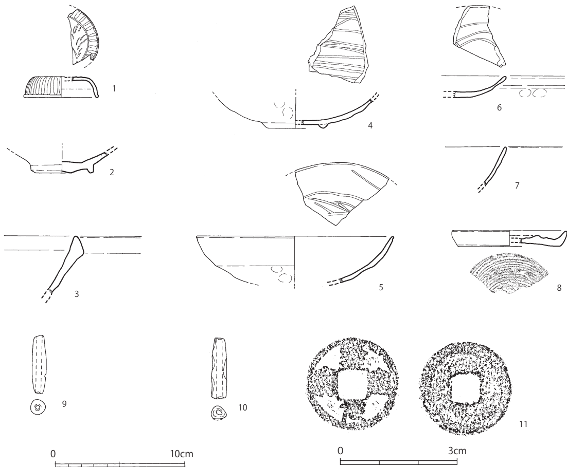
第7-266図 10-SE440出土遺物実測図 (1/3、1/1)
