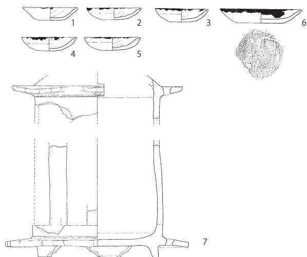
08-SD068出土遺物 (1/6)
