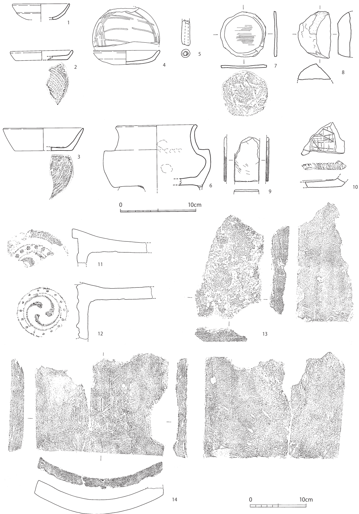
第7-275図 柱穴出土遺物実測図 (1/3、1/4)
