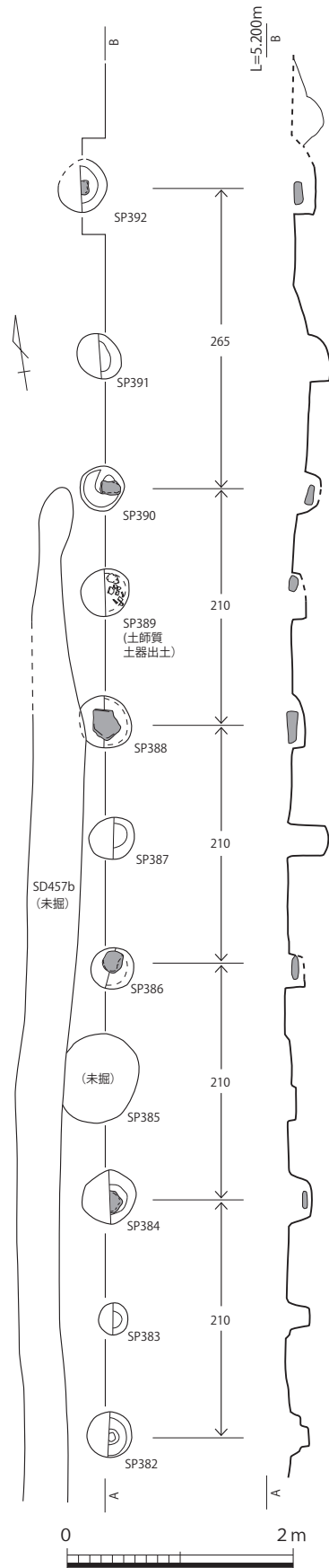
第7-273図 柱穴列実測図 (1/60)
