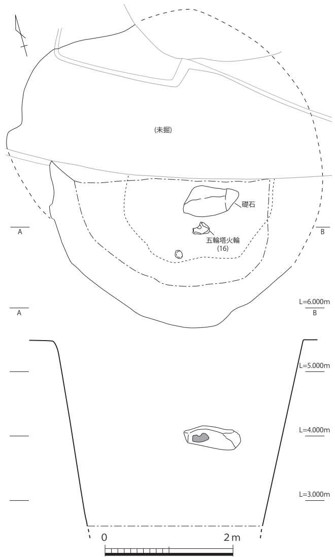
第7-259図 10-SE271実測図(1/50)
