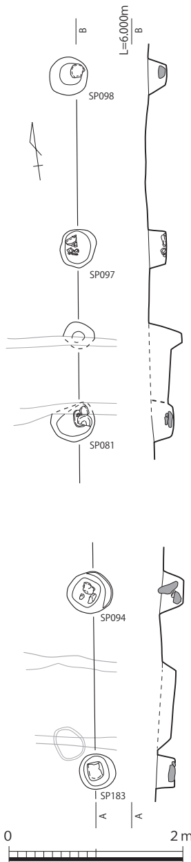
第7-272図 10-SP098ほか実測図 (1/60)
