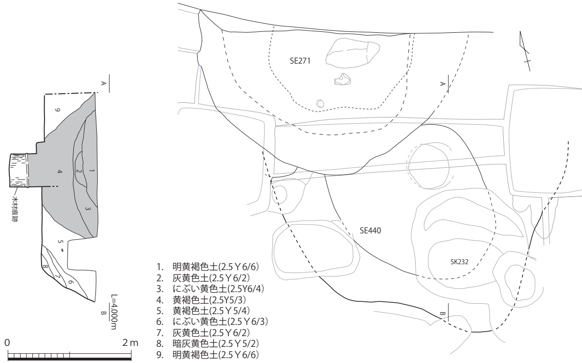
第7-265図 10-SE440実測図 (1/60)
