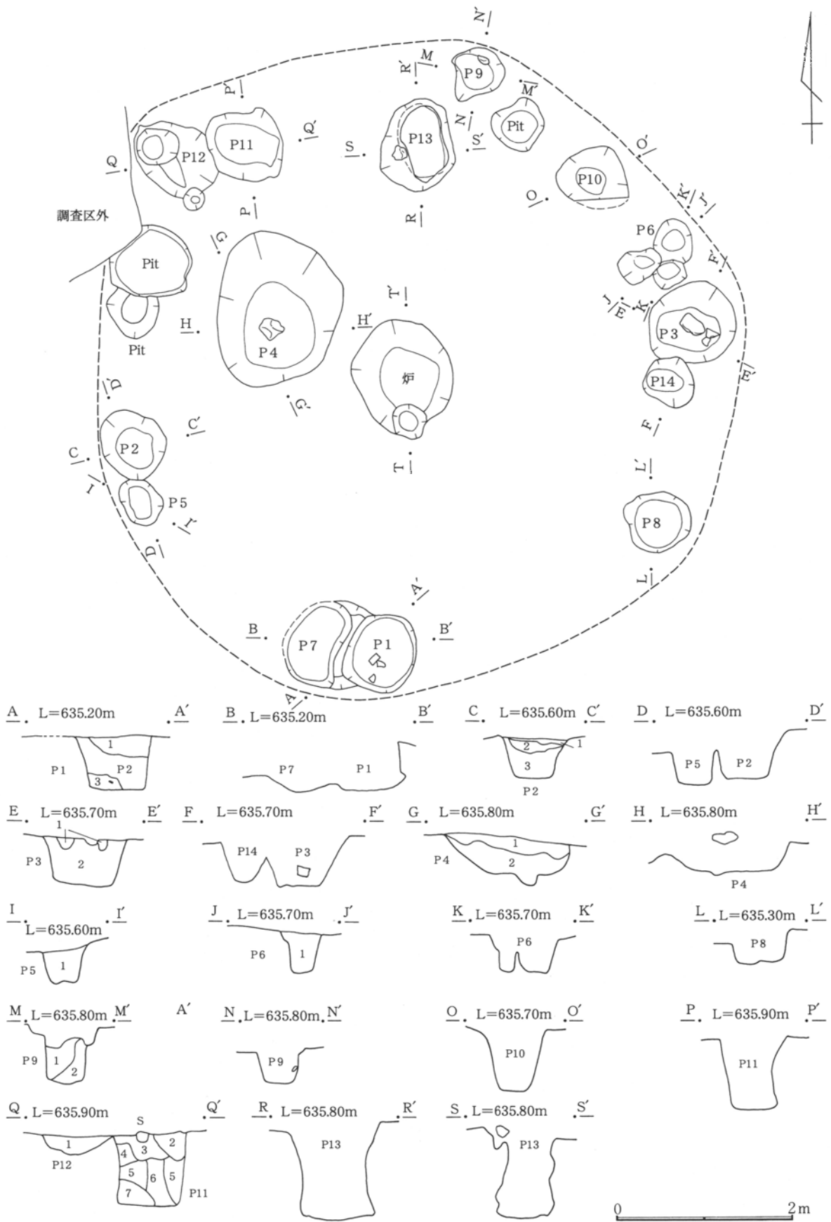
第48图 5—28号住居跡(1)
