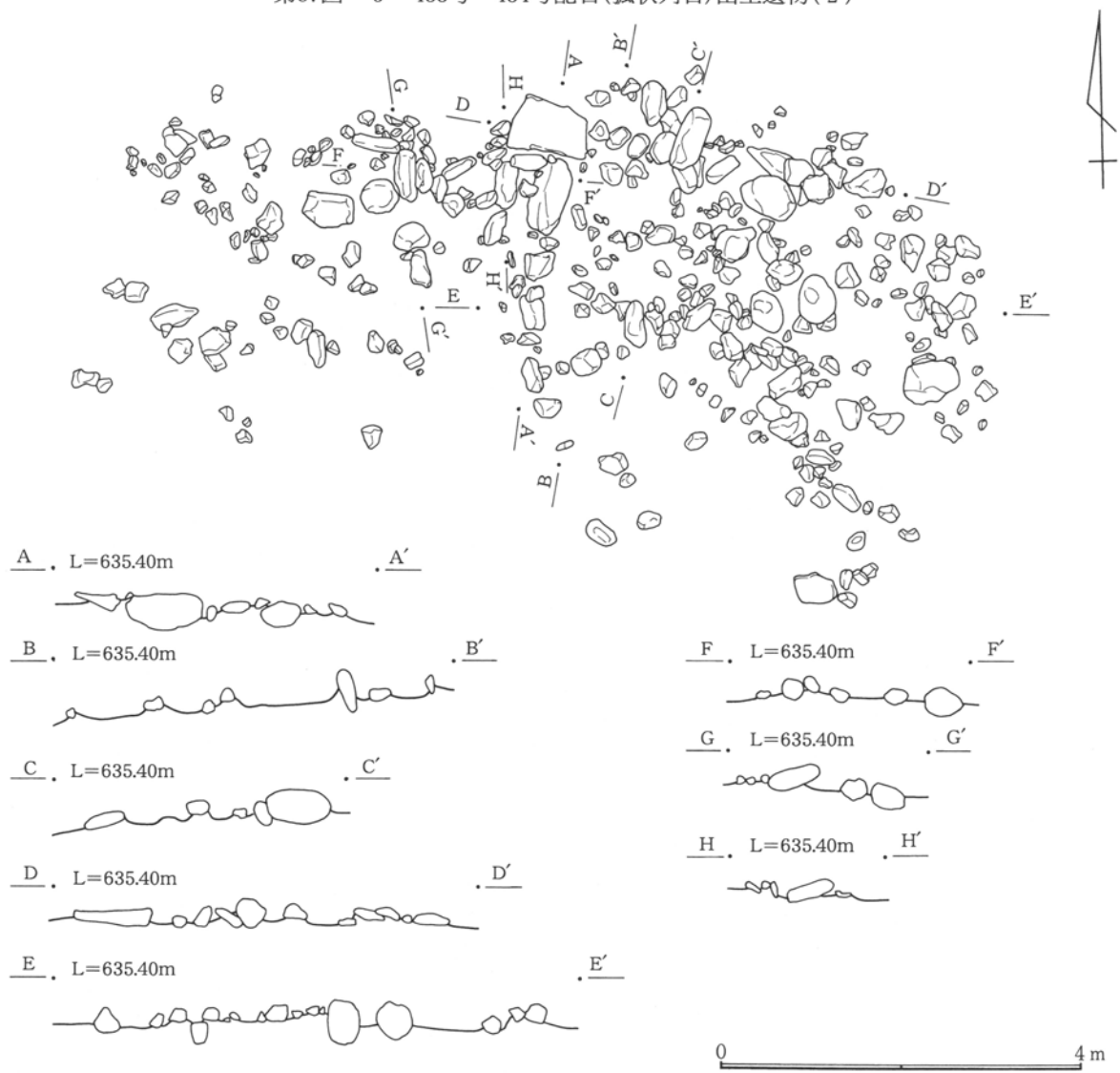
第88图 5—435号配石(弧状列石)
