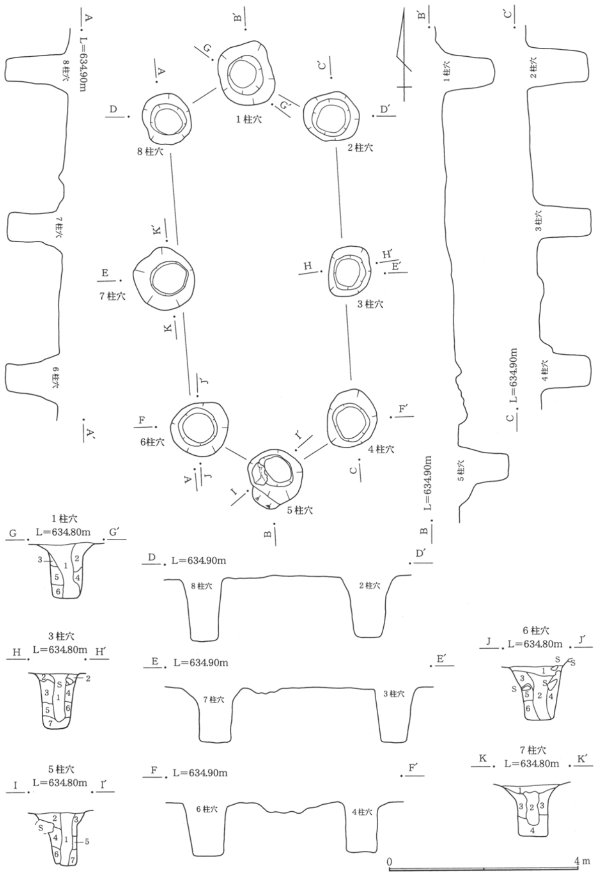
第75图 5-1号柱穴列
