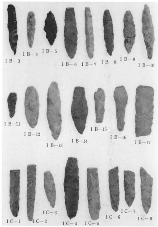
石錐 (I B, I C類)
