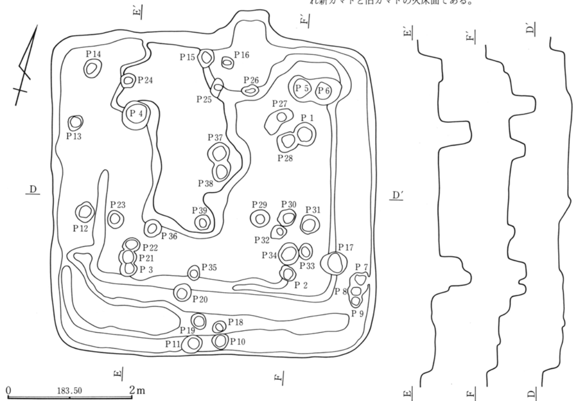
掘り方平面図
