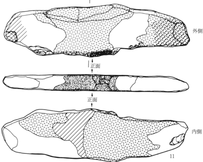
①焚口天井石
