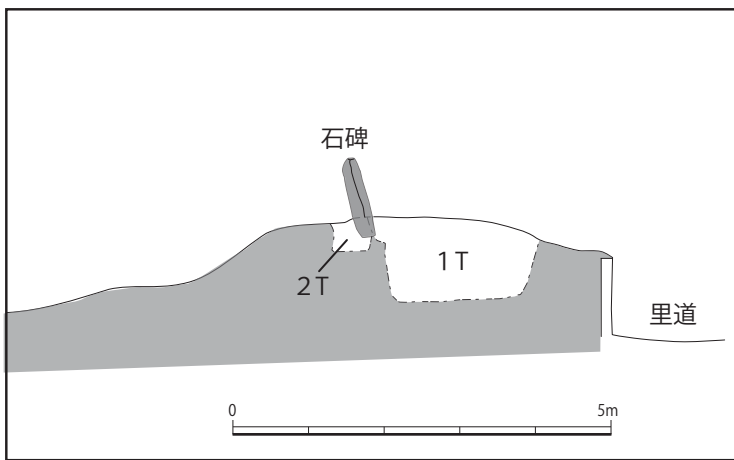
第41図 西林坊トレンチ平面・断面図
