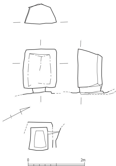
第 65 図 石貫ナギノ横穴群 5号墓実測図 (※西住・宮本 1980 より)
