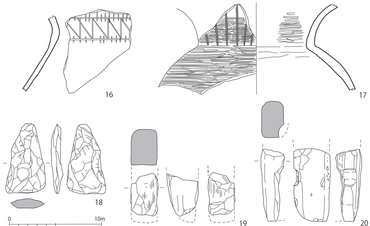
第58図 年の神遺跡（B地点）周辺出土遺物実測図
