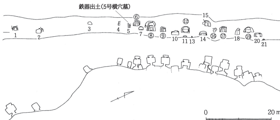
第 64 図 石貫ナギノ横穴群配置図 (部分)
