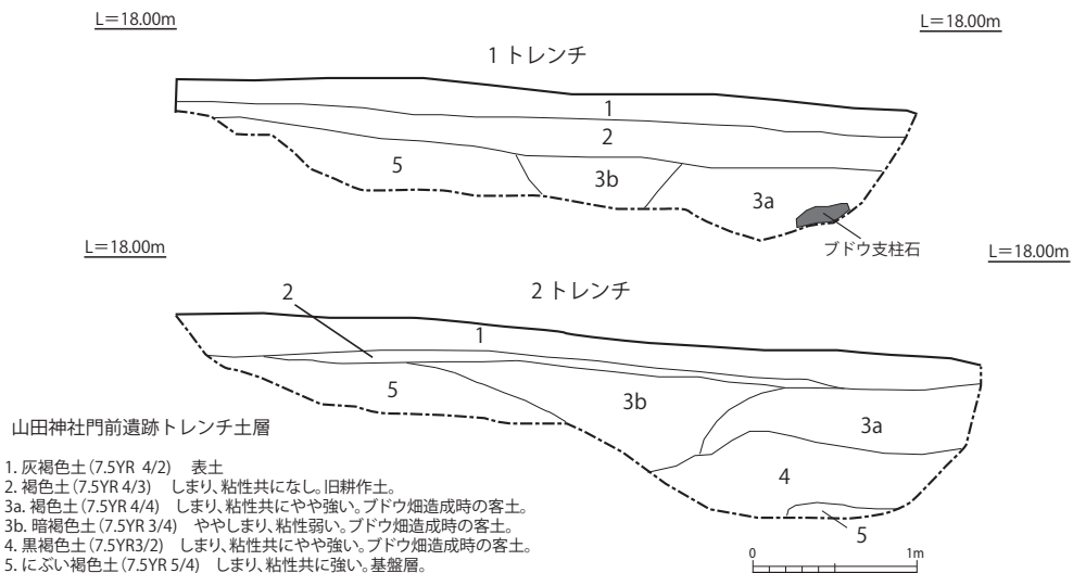
第 35 図 山田神社門前遺跡群 (A 地点) トレンチ土層図
