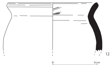
第46図 寺田久保遺跡出土遺物実測図
