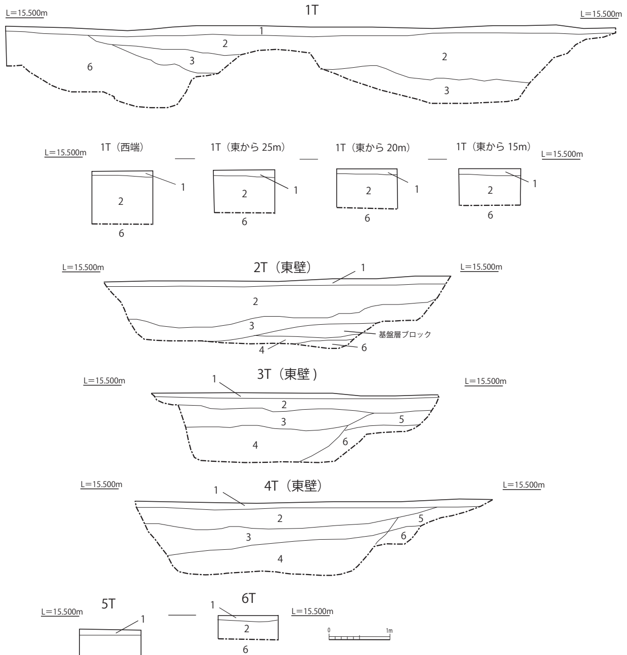
年の神遺跡 A 地点トレンチ土層
