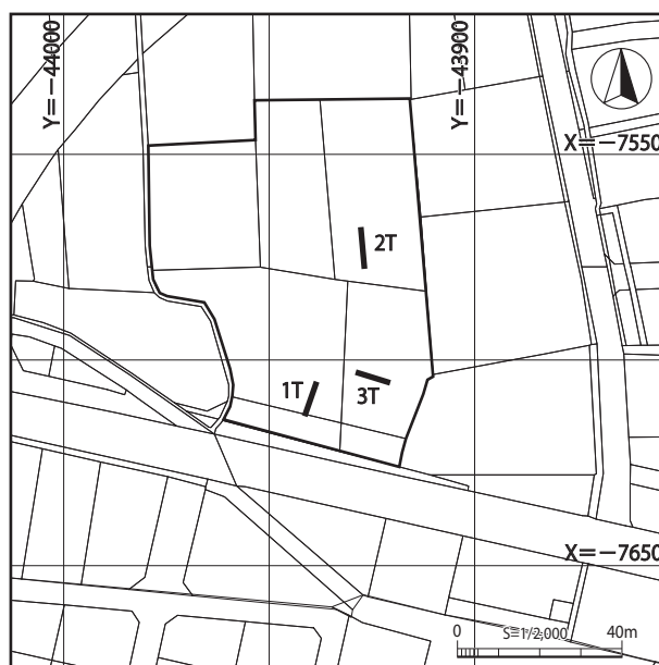
第 60 図 今見堂遺跡トレンチ配置図
