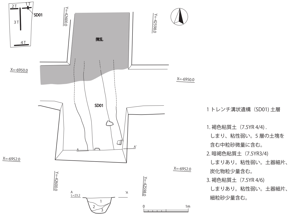
第51図 1 トレンチ溝状遺構平面・断面図
