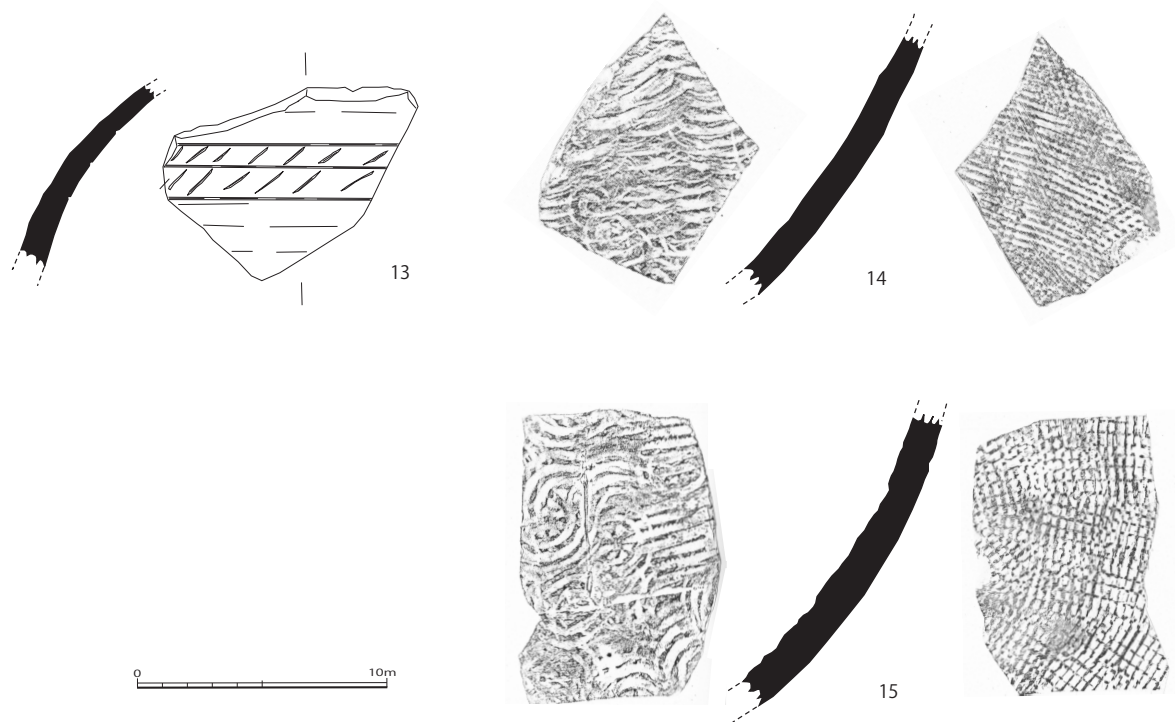
第 53 図 高岡原遺跡出土遺物実測図
