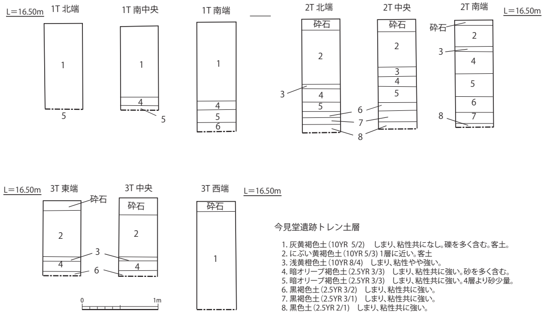
第 61 図 今見堂遺跡トレンチ土層図
