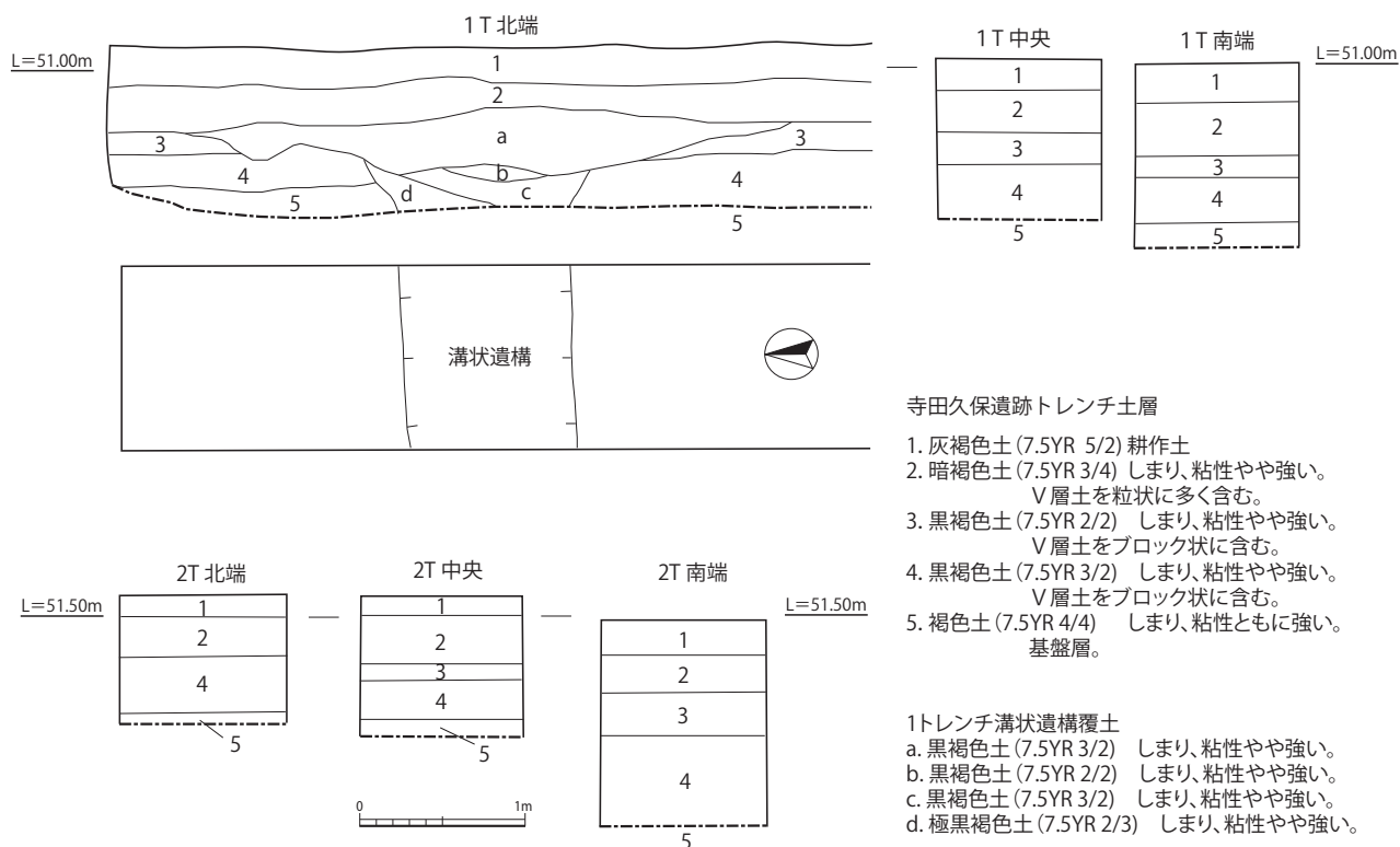
第 47 図 寺田久保遺跡トレンチ土層図
