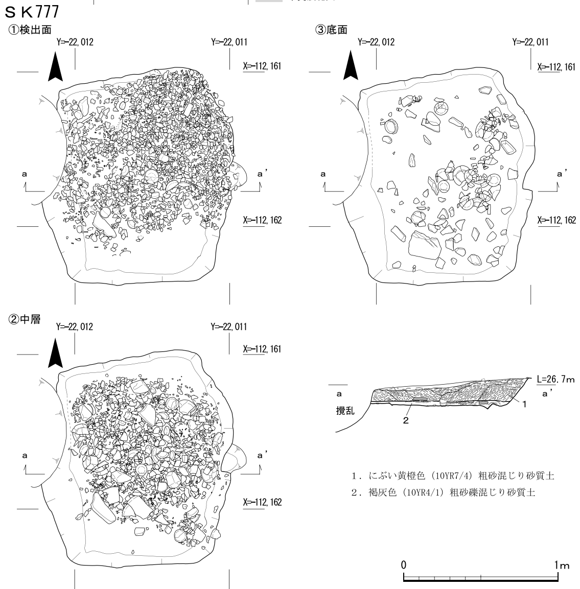
第42図 S K 775・777実測図
