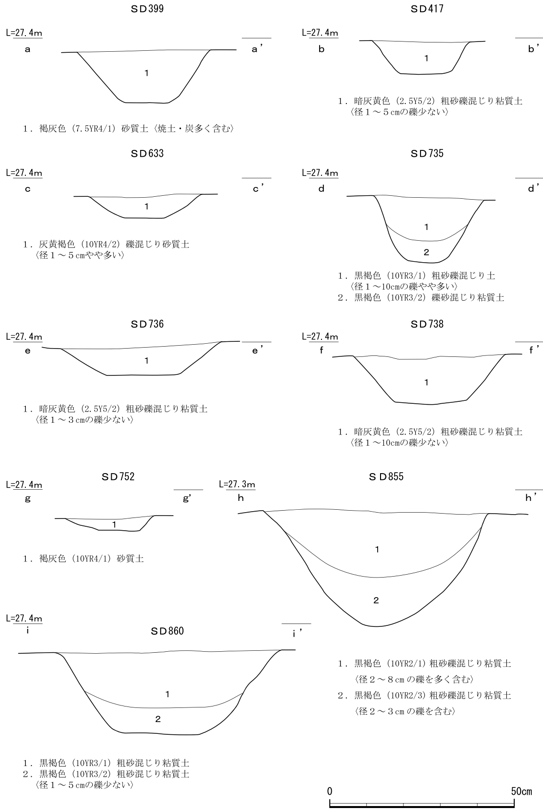
第50図 溝断面一覧
