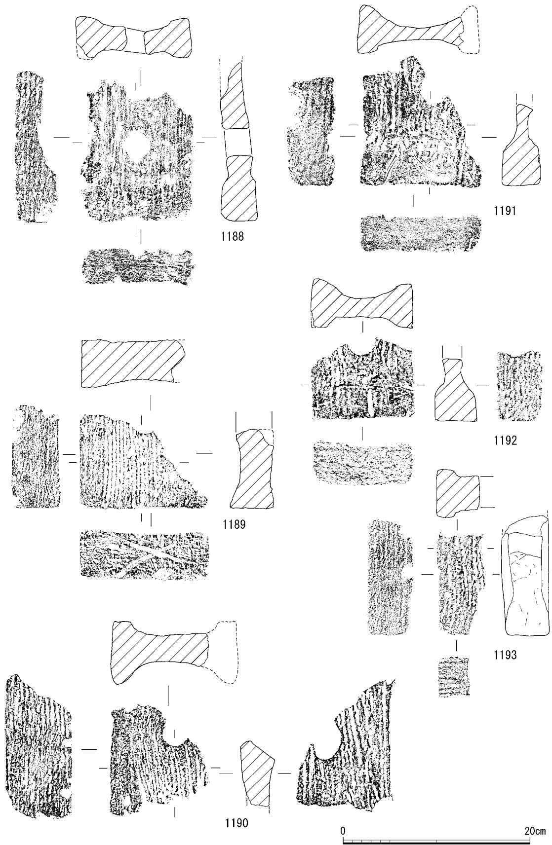
第80図 出土遺物実測図 埴(3)
