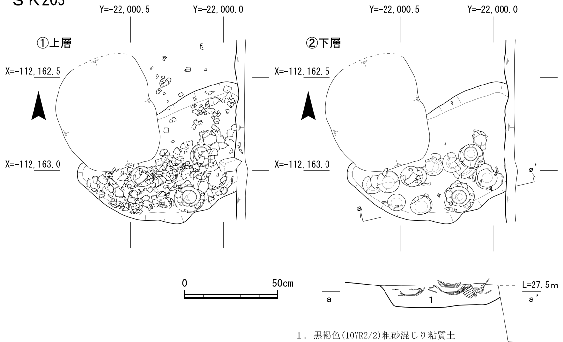
第33図 S K 127・203実測図
