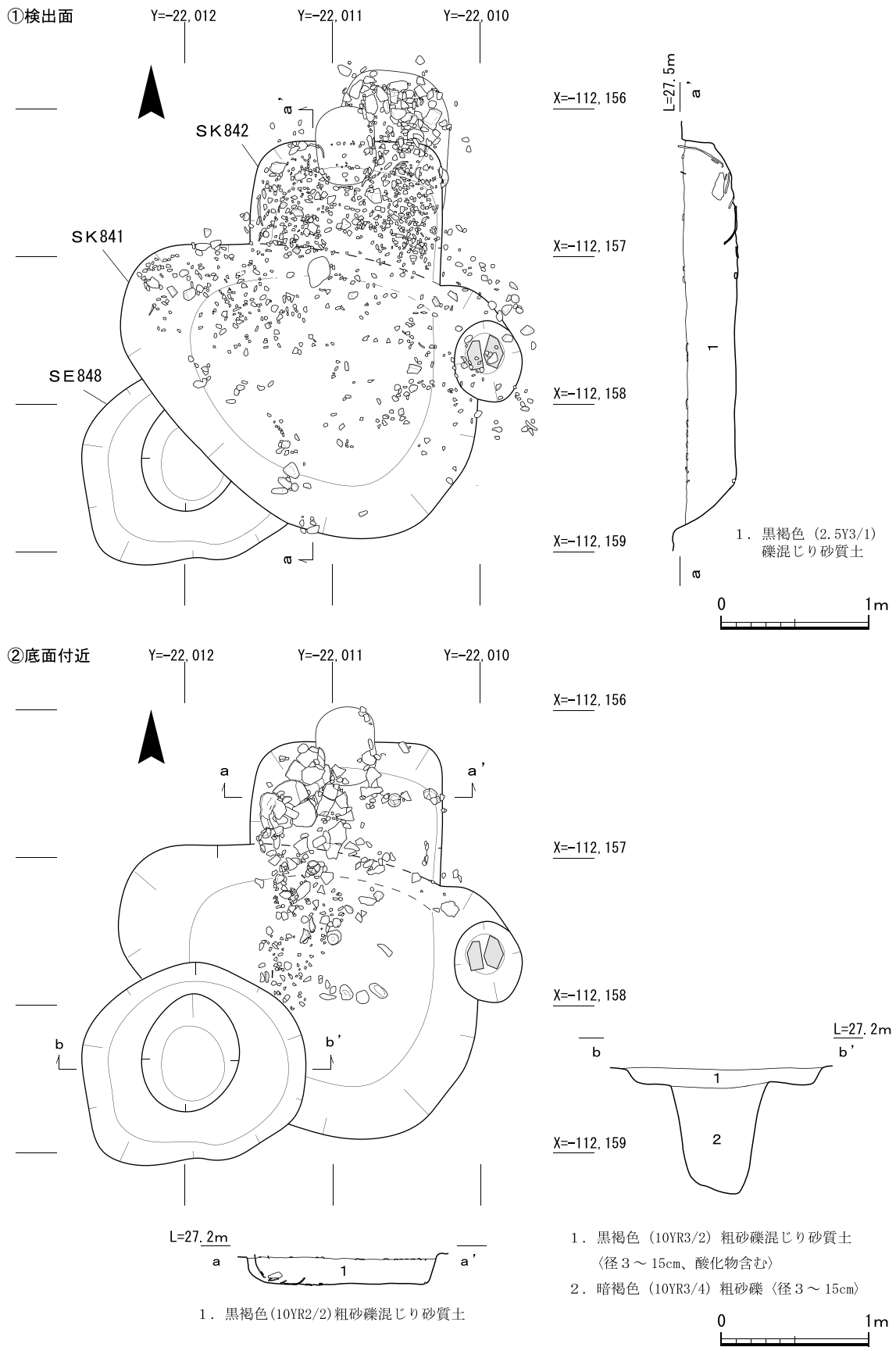
第44図 SK841・842・SE848実測図
