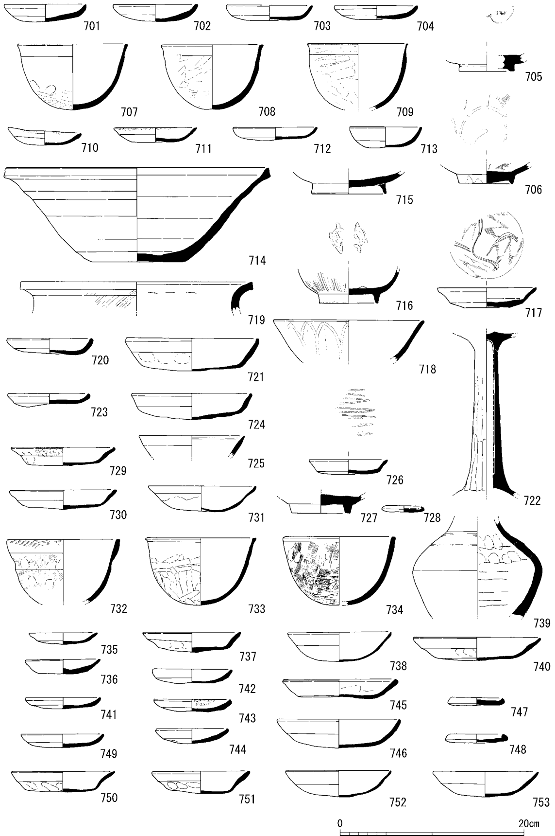
第62図 出土遺物実測図
