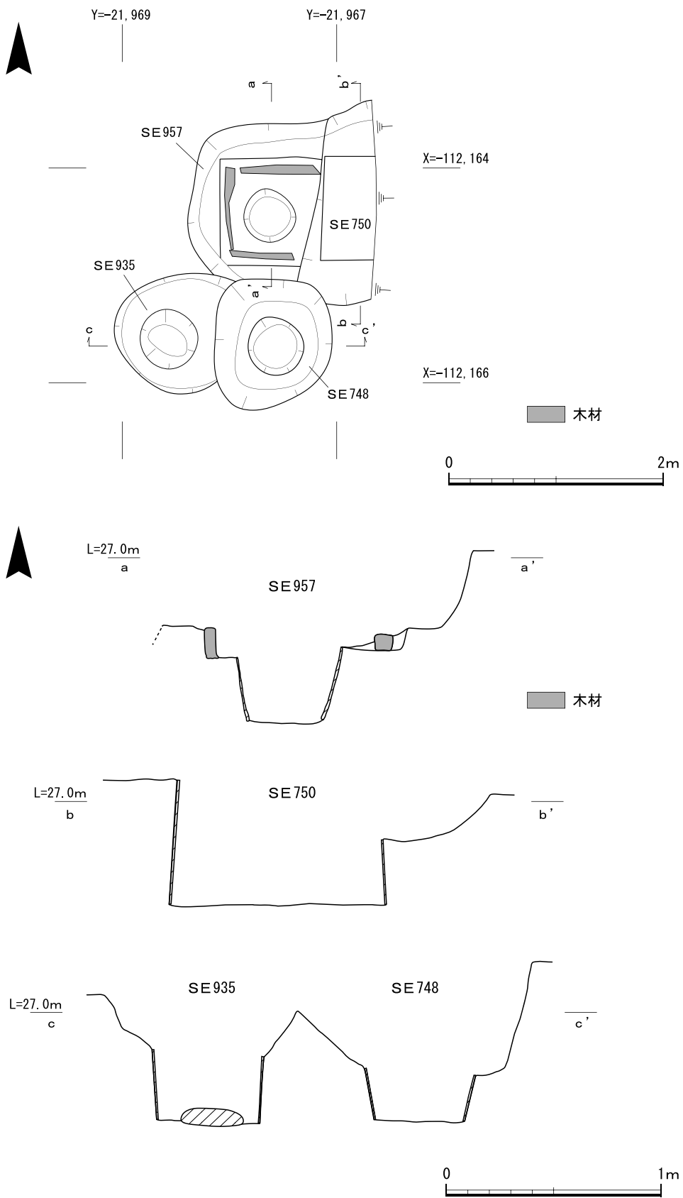
第48図 SE748・750・935・957実測図
