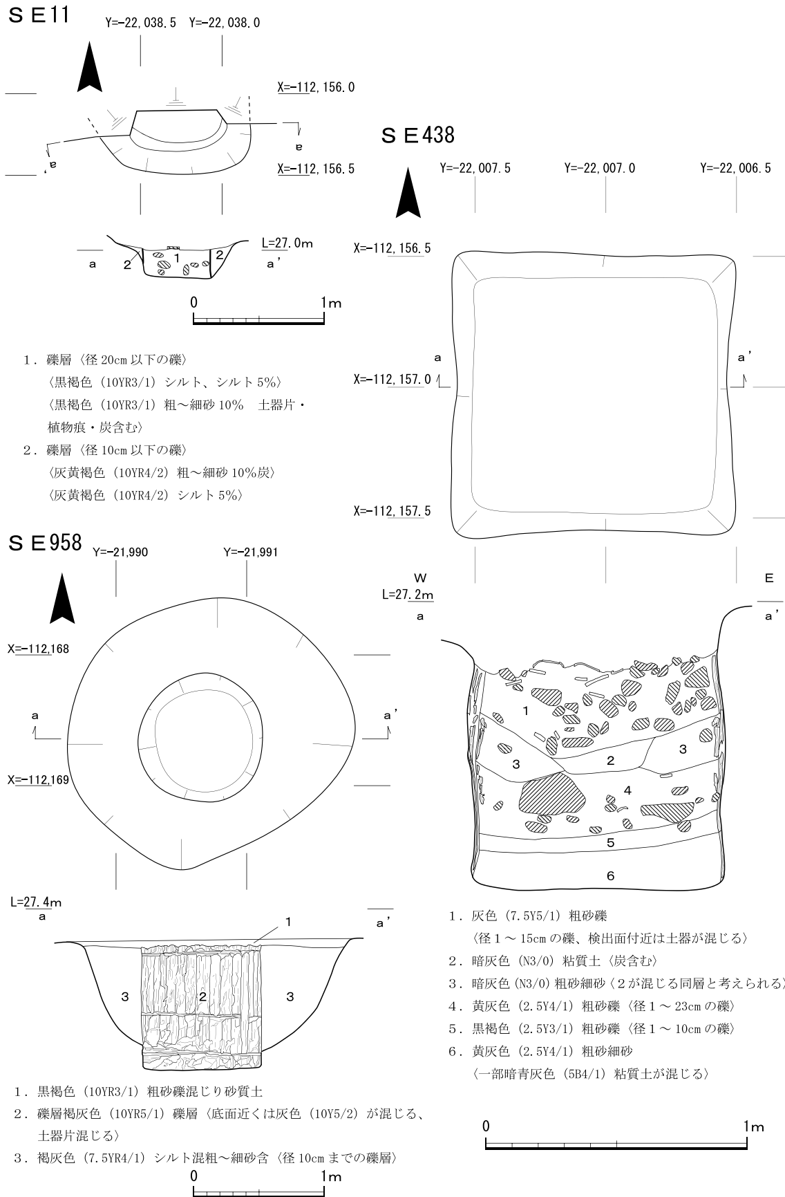
第47図 SE11・438・958実測図
