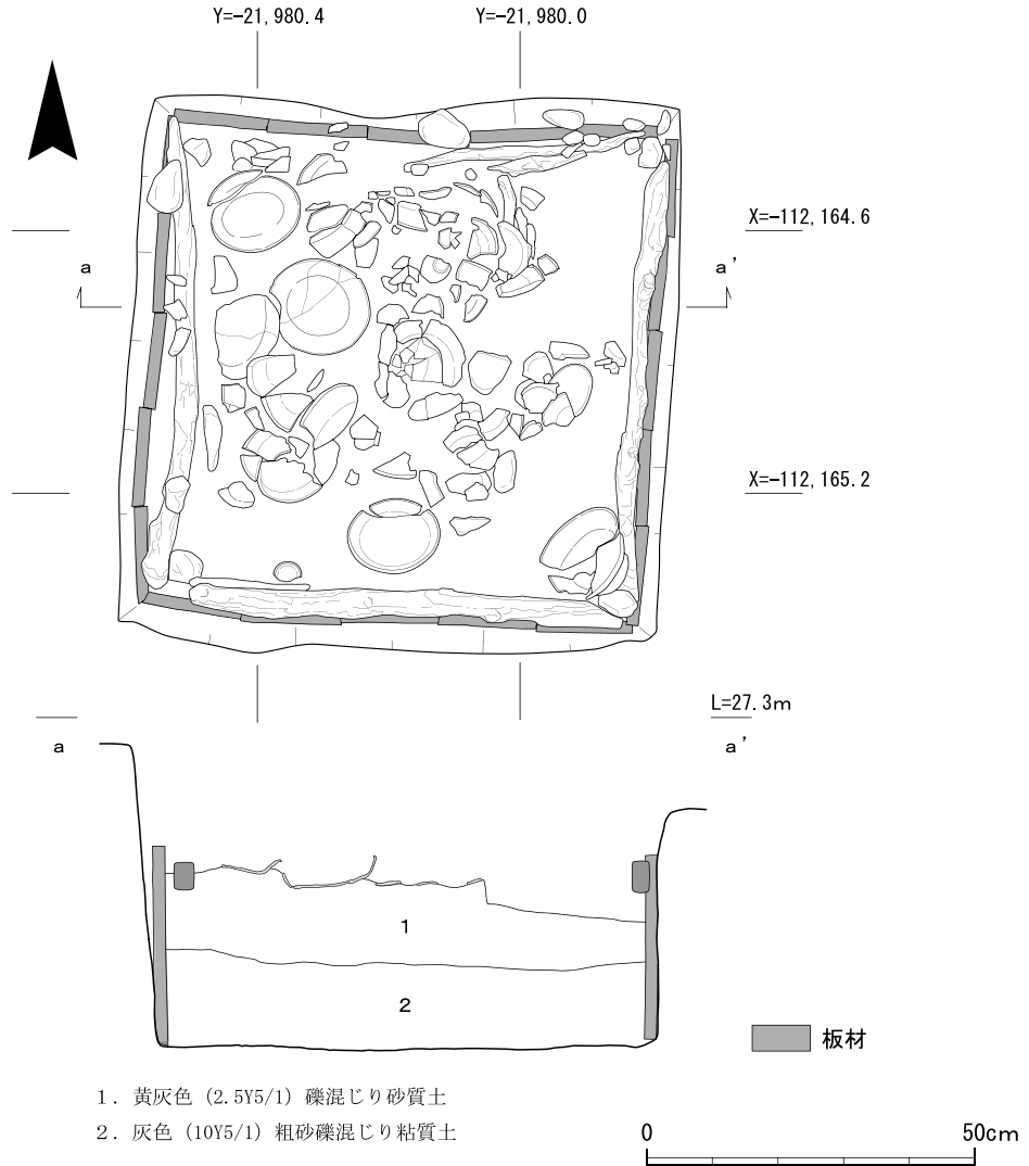
第34図 S K354・972実測図
