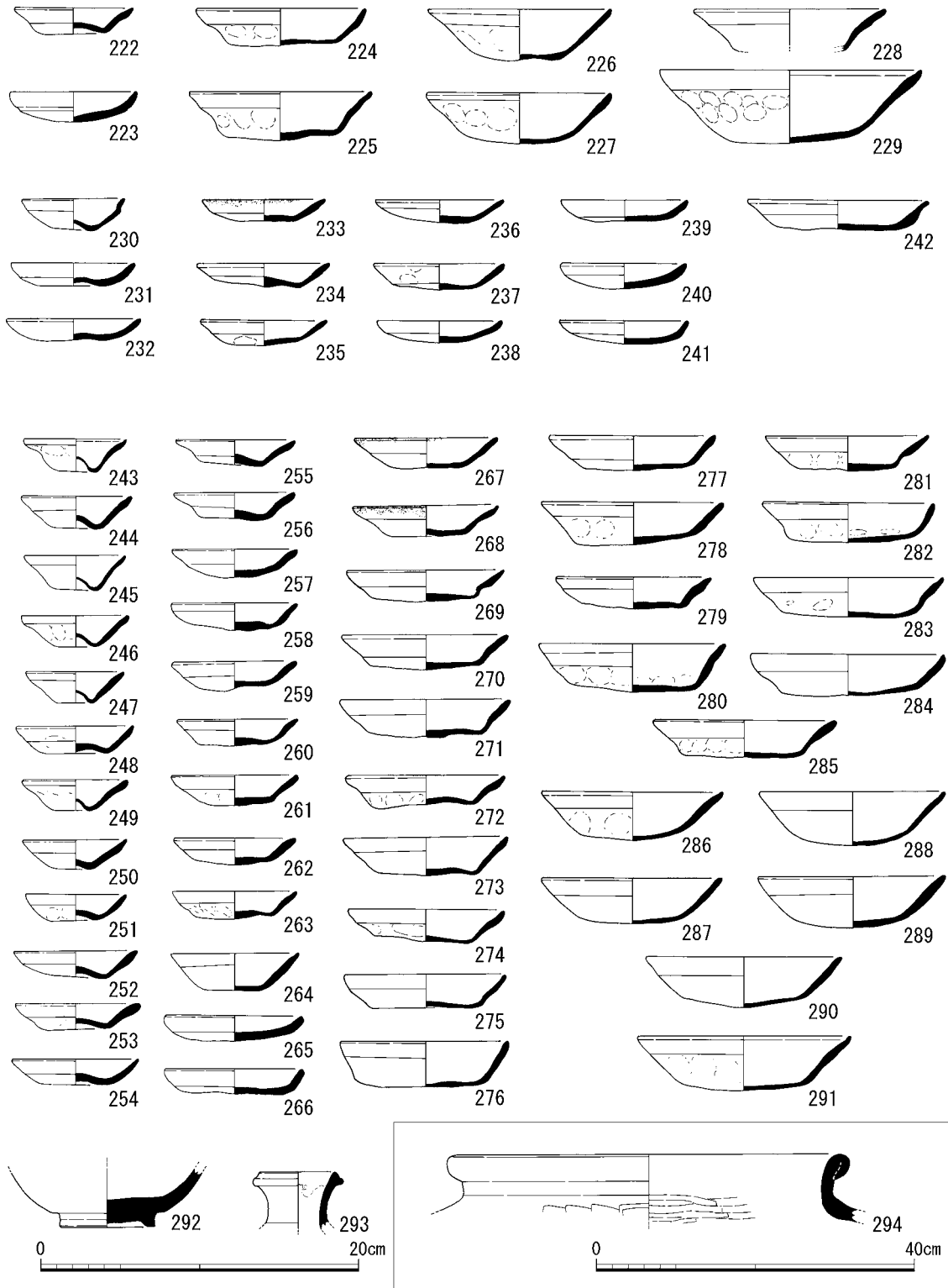
第54図 出土遺物実測図 S K 203・840・126
