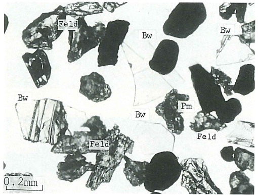
5 試料番号12の軽鉱物
