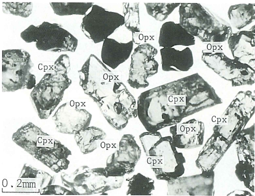
2 試料番号10の重鉱物
