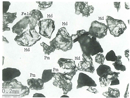
4 試料番号5の軽鉱物
