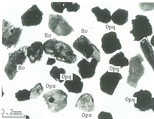
3 試料番号26の重鉱物
