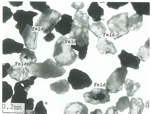
6 試料番号16の軽鉱物
