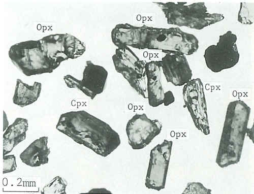
1 試料番号1の重鉱物
