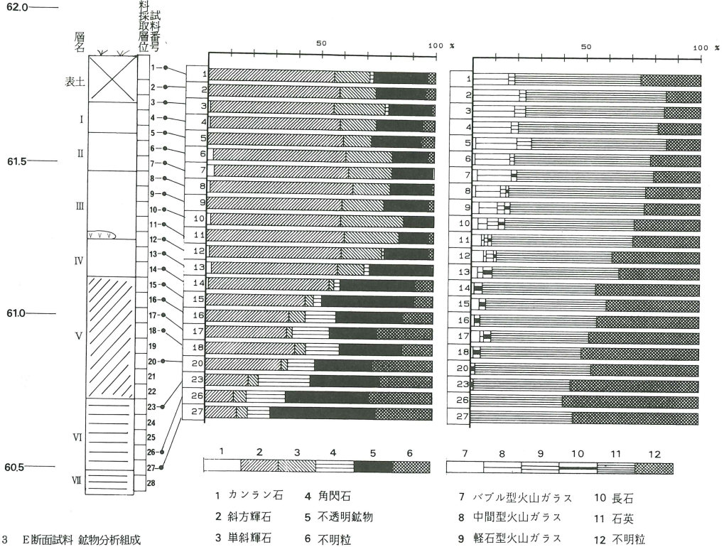
図3 E断面試料 鉱物分析組成
