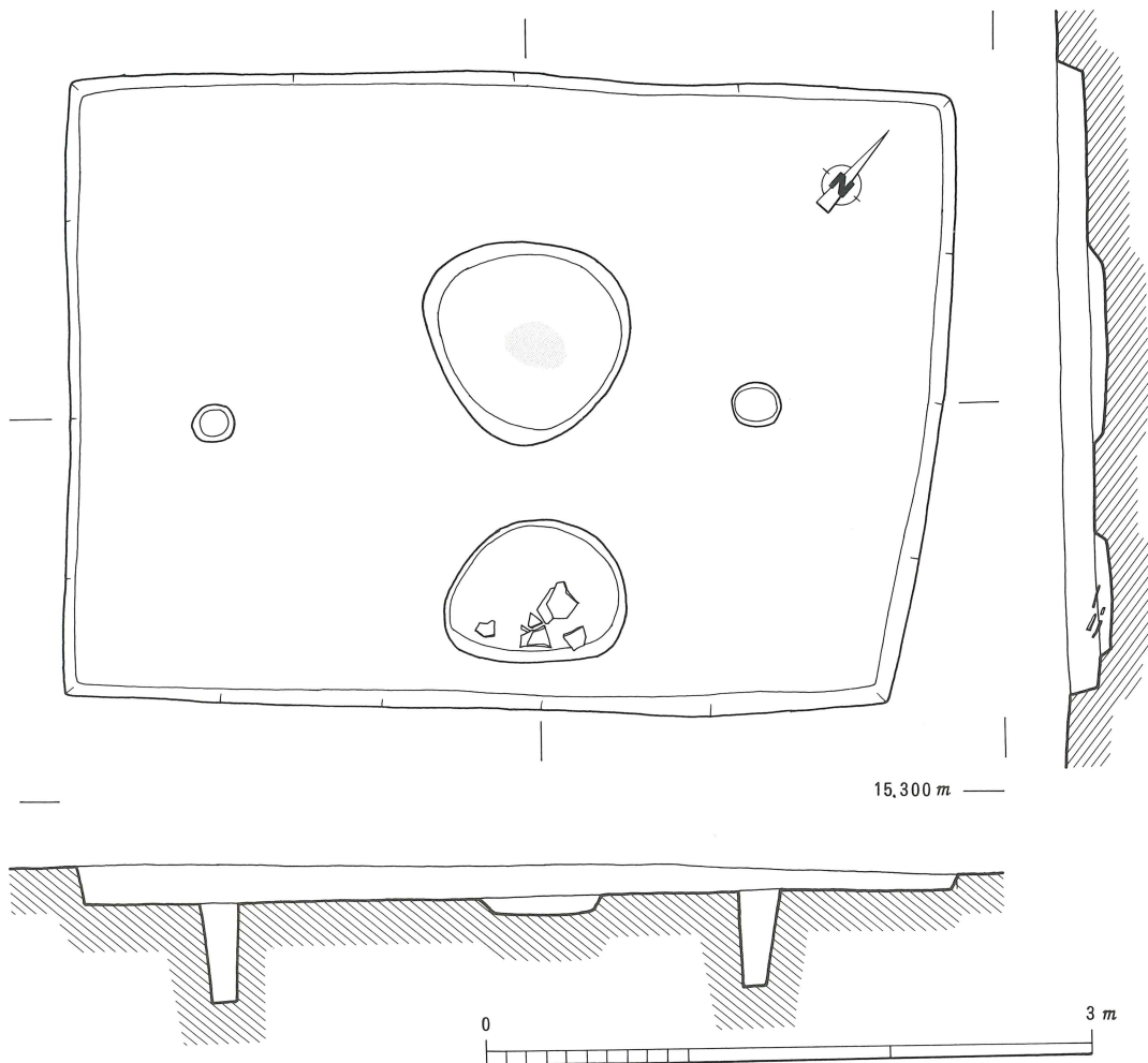
Fig. 6 SH 2 実測図 (トーンは焼土塊)
