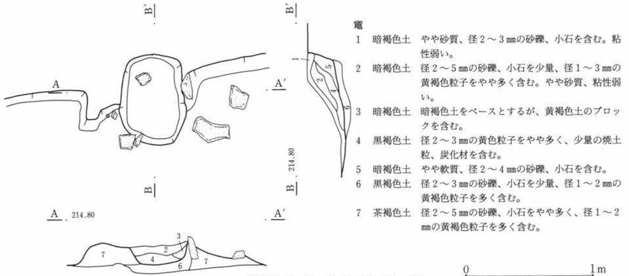
第334図 C-242号住居跡・竈
