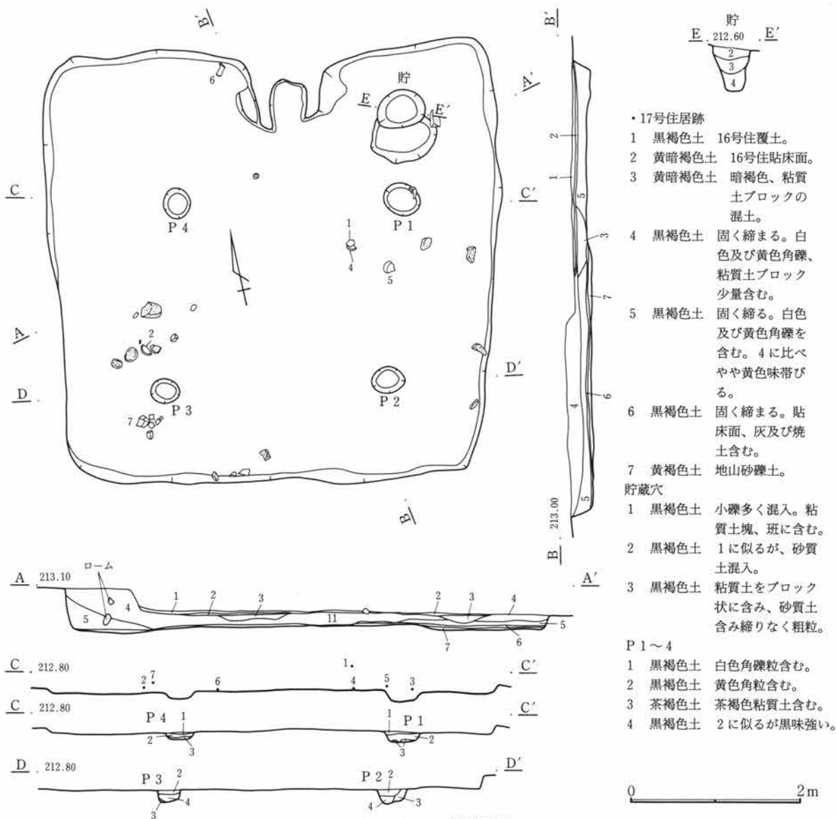
第25図 C—17号住居跡
