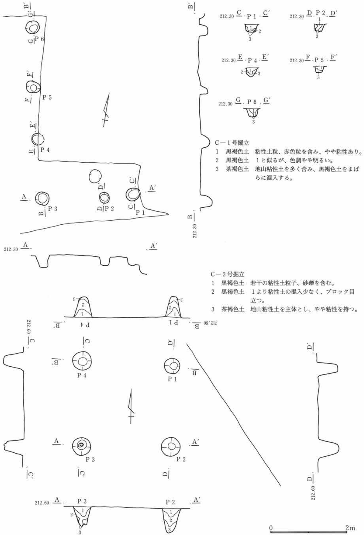
第624図 C-1、2号掘立
