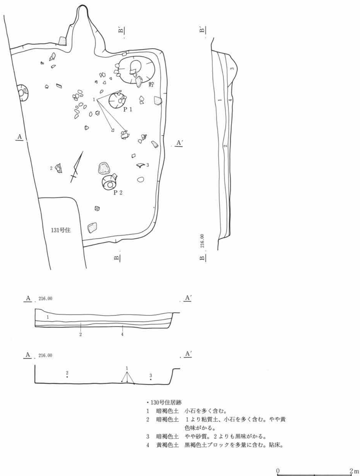
第169図 C-130号住居跡
