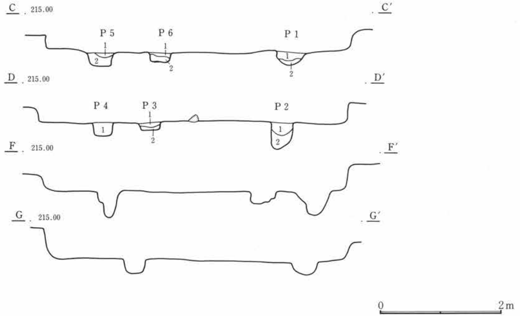
第367図 C-256号住居跡(2)
