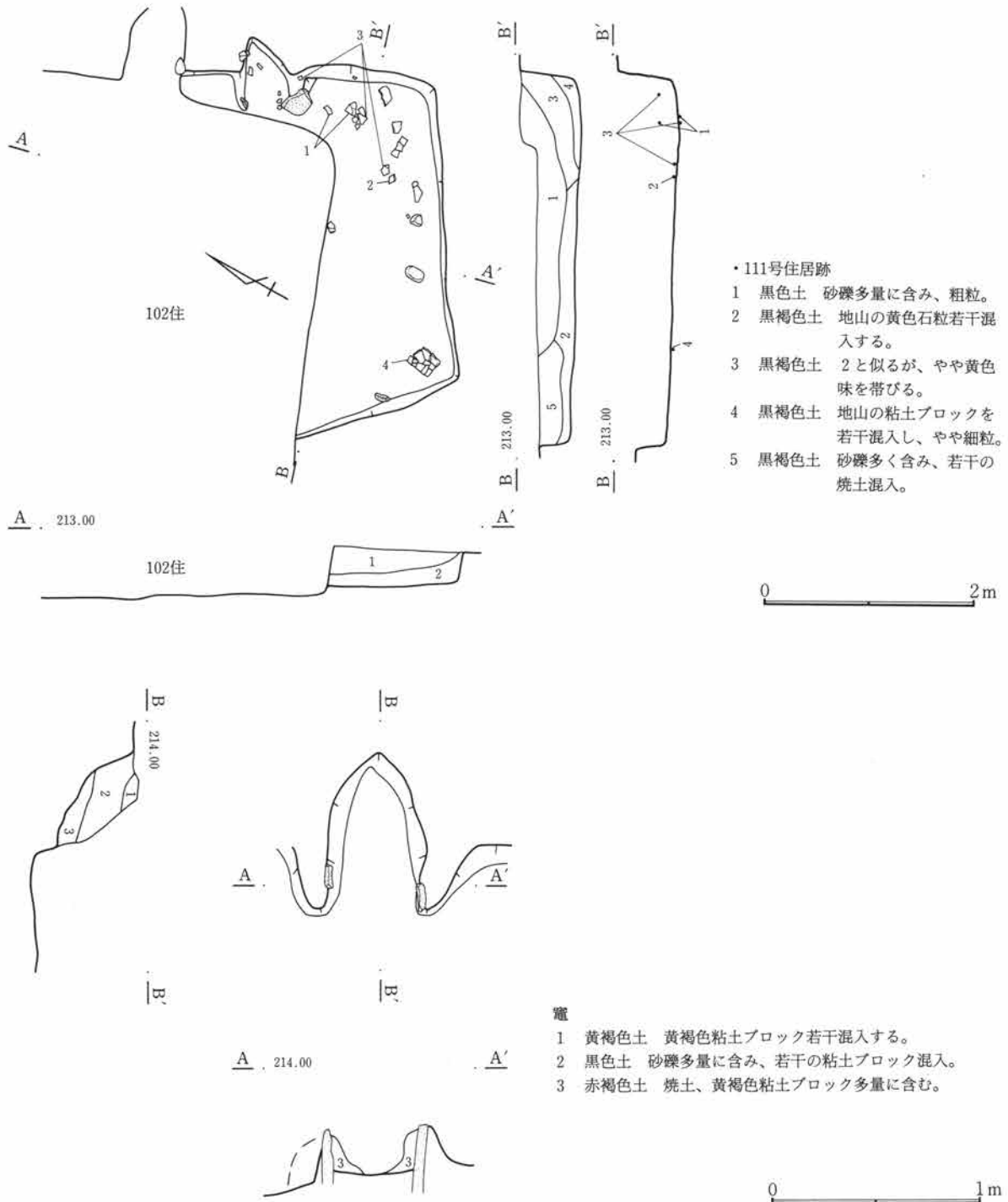
第134図 C-111号住居跡・竈
