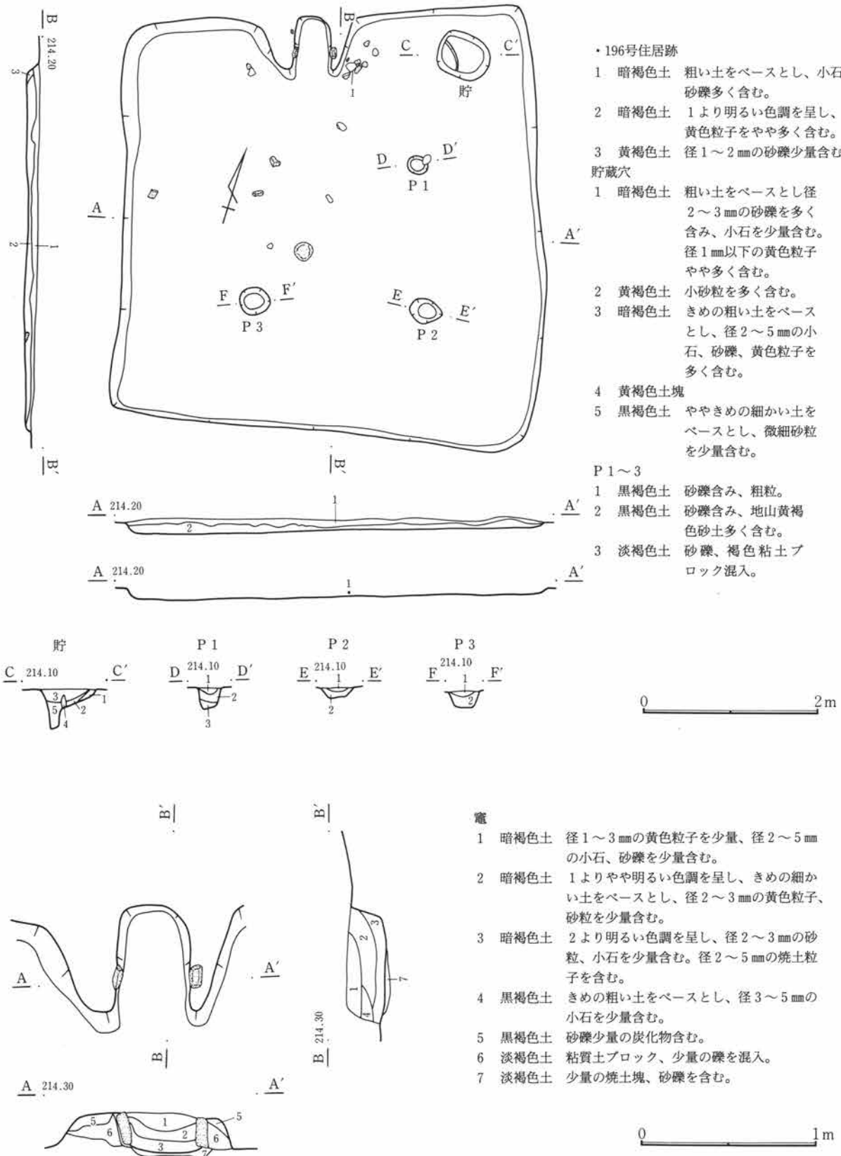
第277図 C-196号住居跡・竈
