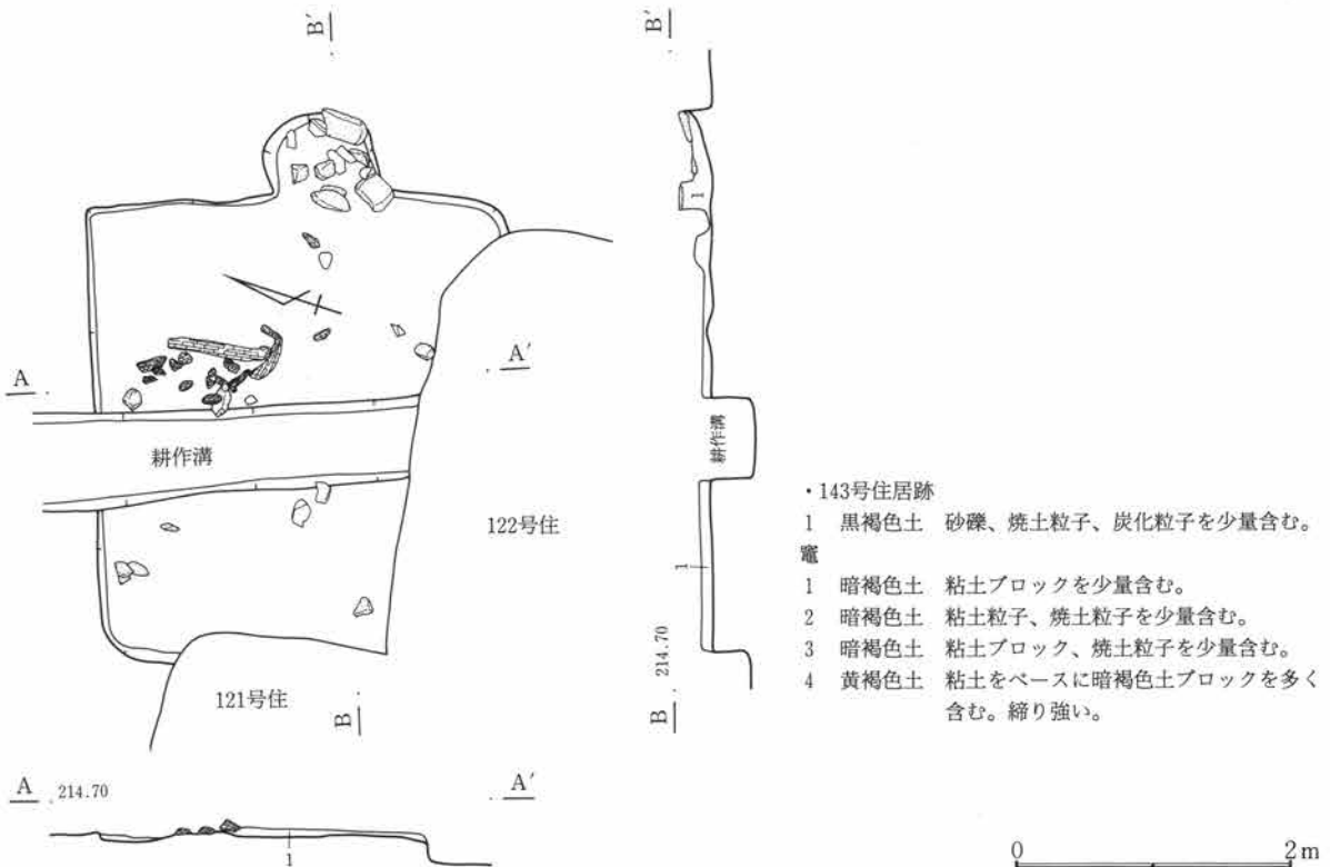
第195図 C-143号住居跡
