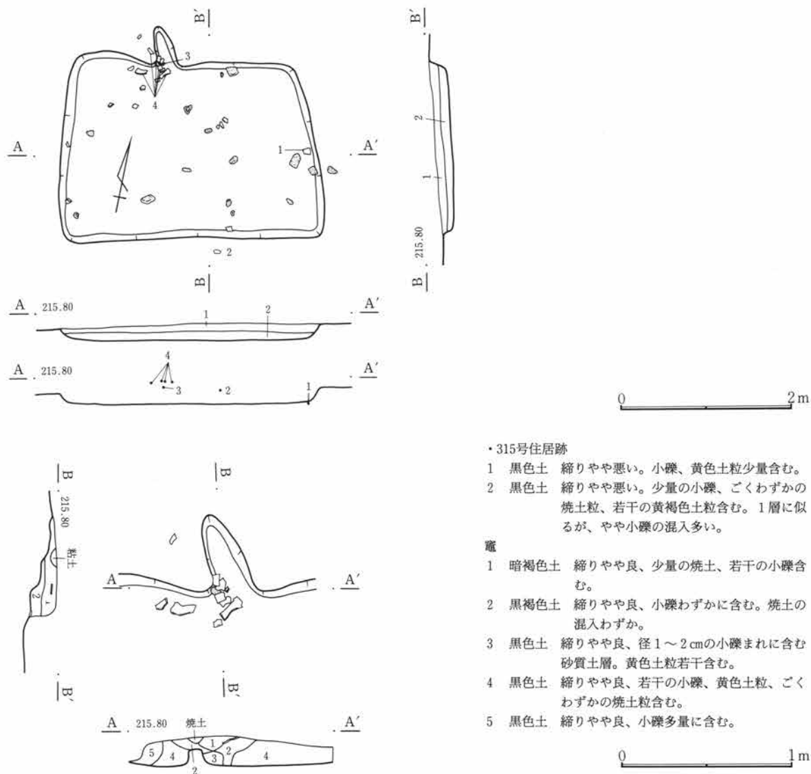
第488図 C-315号住居跡・竈
