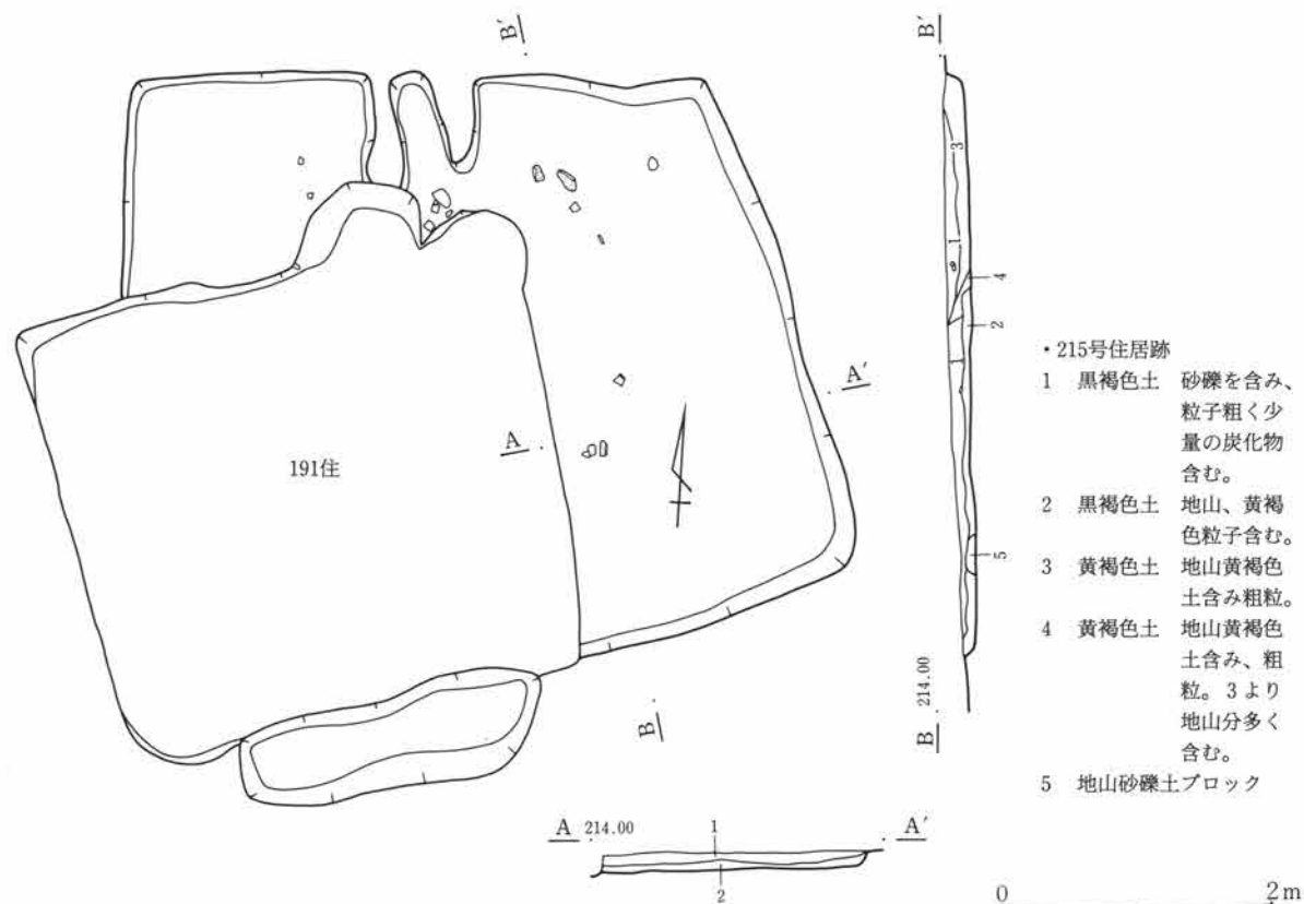
第288図 C-215号住居跡
