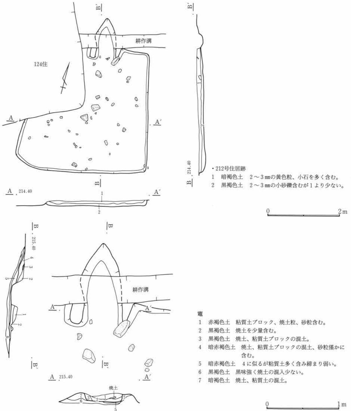
第284図 C-212号住居跡・竈
