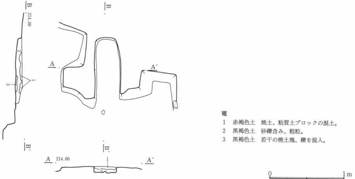
第289図 C-215号住居跡・竈
