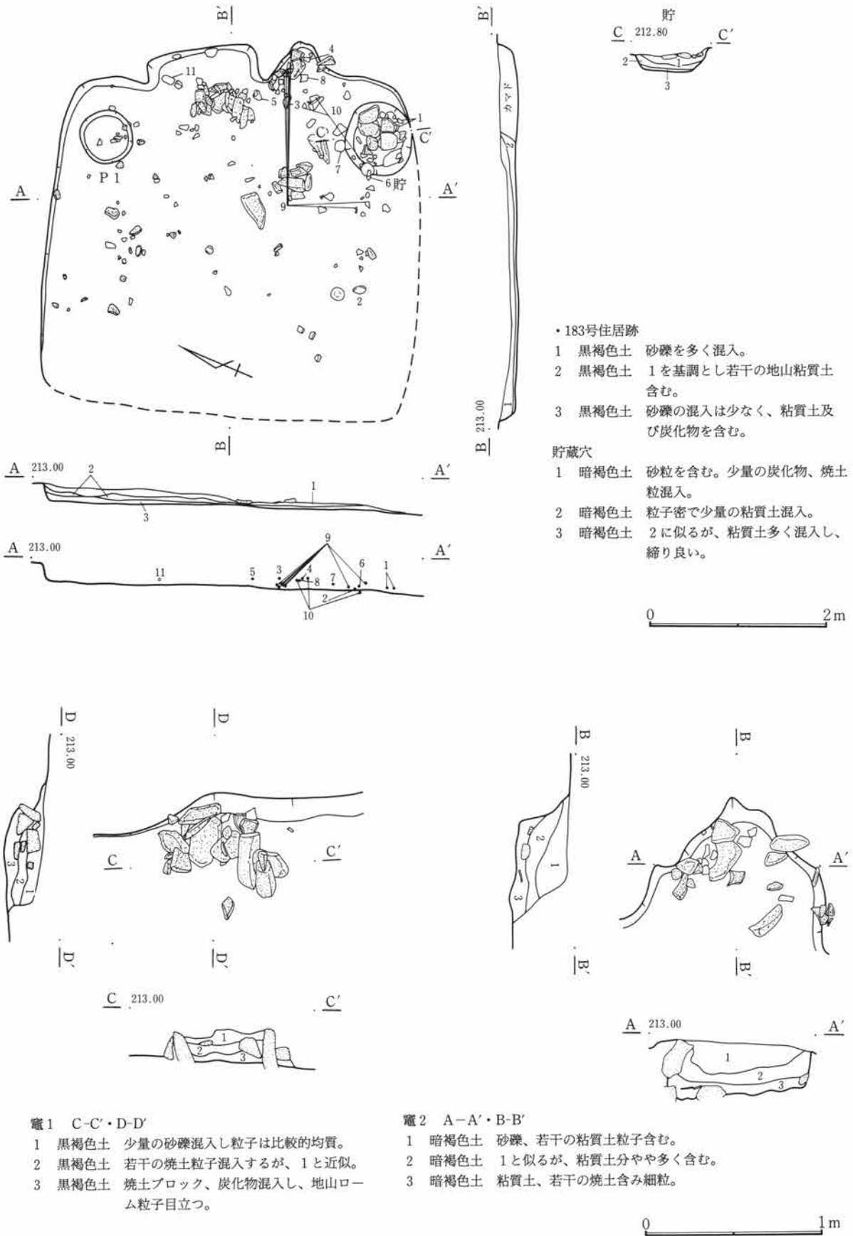
第255図 C—183号住居跡・竈
