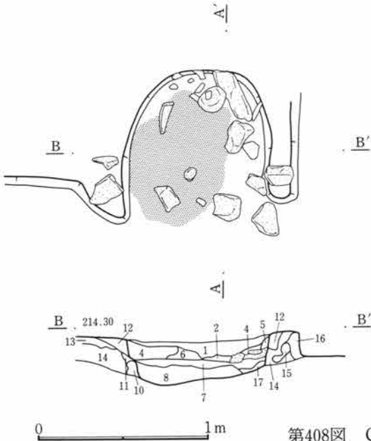
第408図 C-276号住居跡・竈
