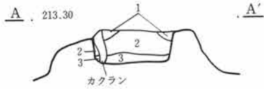
第45図 C-36号住居跡・竈
