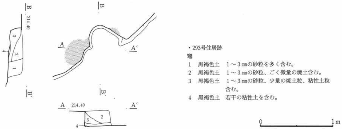
第444図 C-293号住居跡・竈
