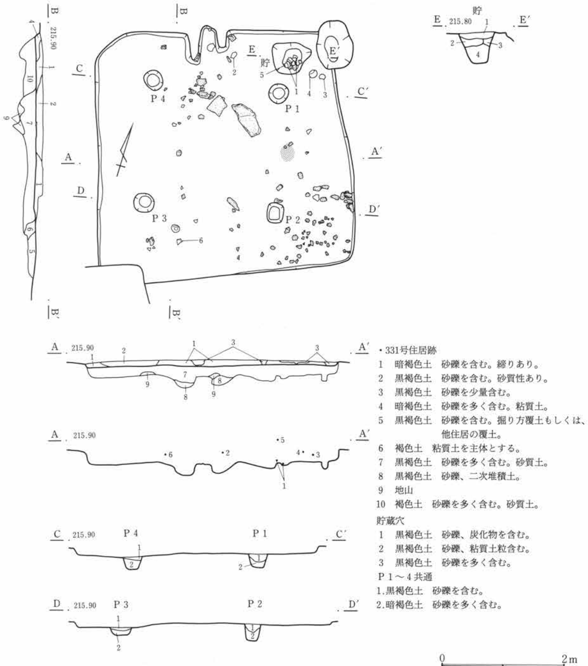
第528図 C-331号住居跡
