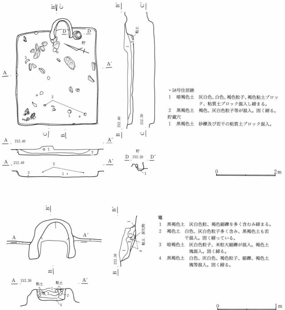
第75図 C-58号住居跡・竈
