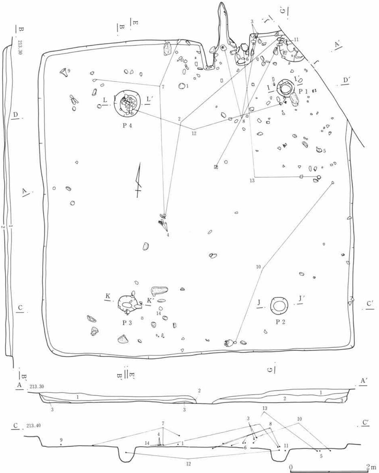
第79図 C-62号住居跡(1)
