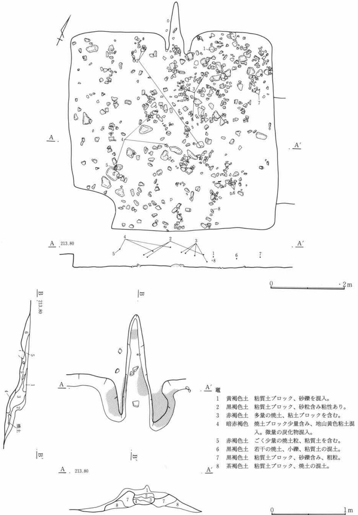
第275図 C-195号住居跡・竈
