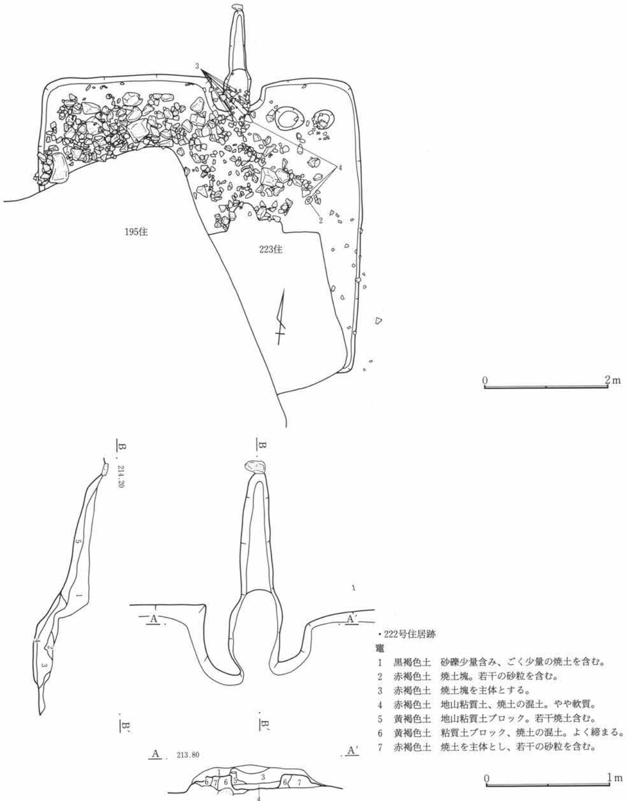
第302図 C—222号住居跡・竈
