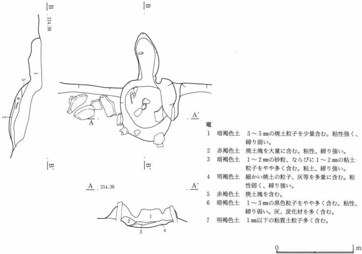
第179図 C—136号住居跡・竈
