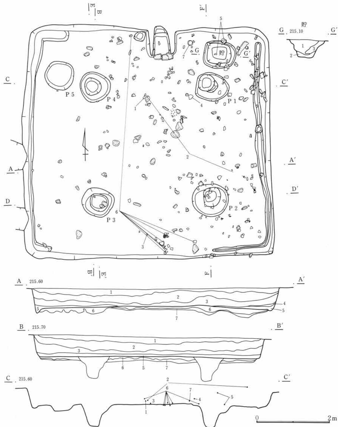
第563図 C-352号住居跡(1)
