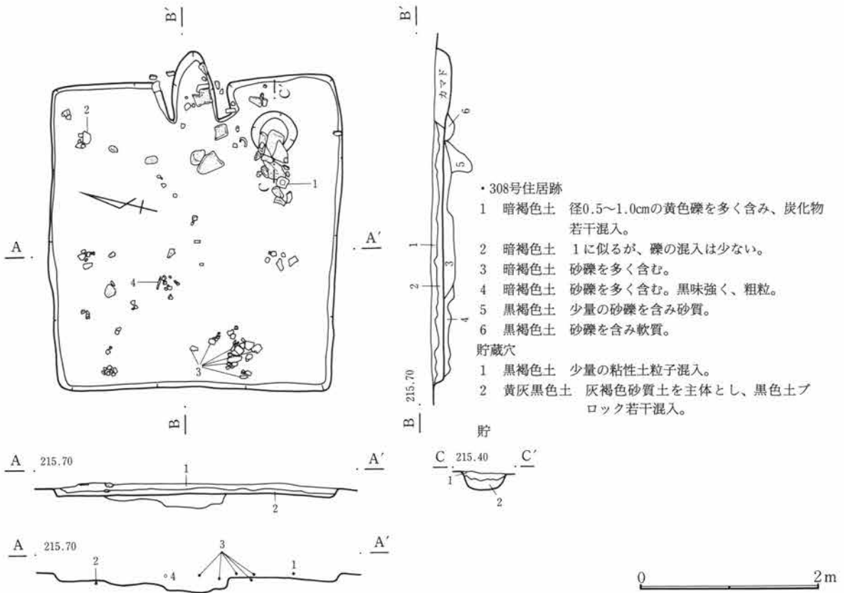
第471図 C-308号住居跡
