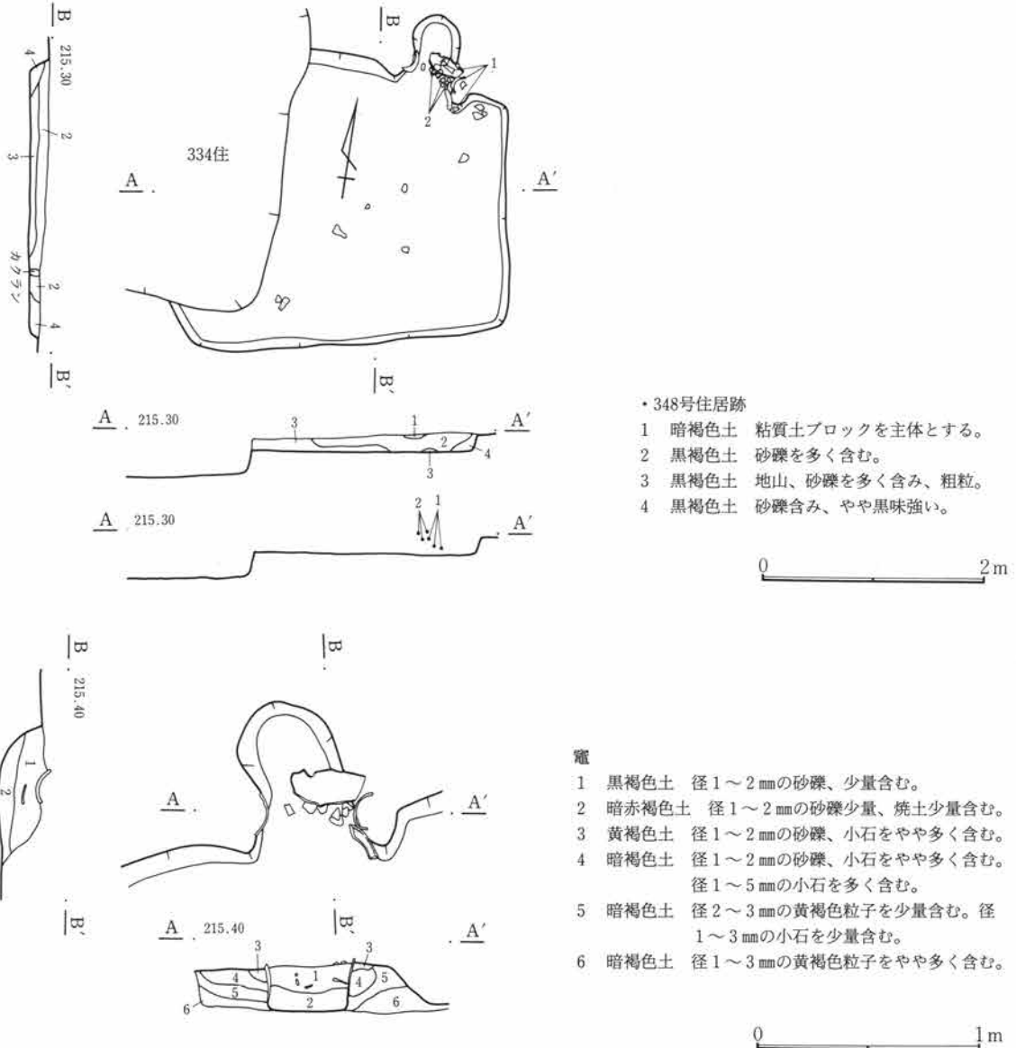
第554図 C-348号住居跡・竈
