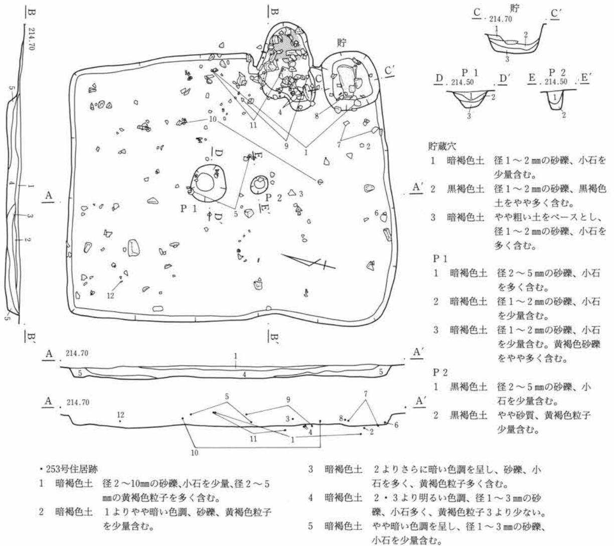
第358図 C-253号住居跡
