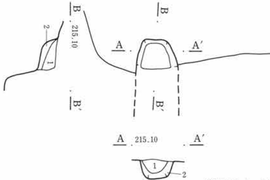
第429図 C-287号住居跡・竈
