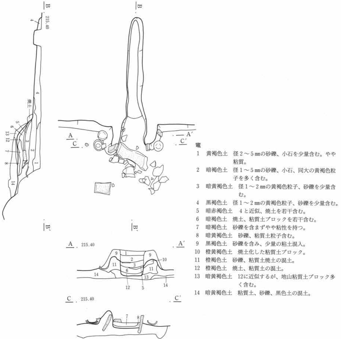
第515図 C-326号住居跡・竈
