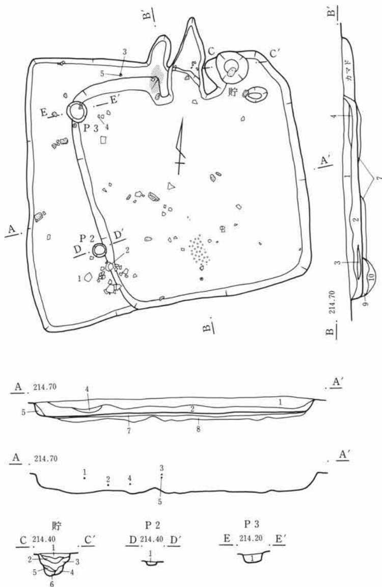
第330図 C-241号住居跡
