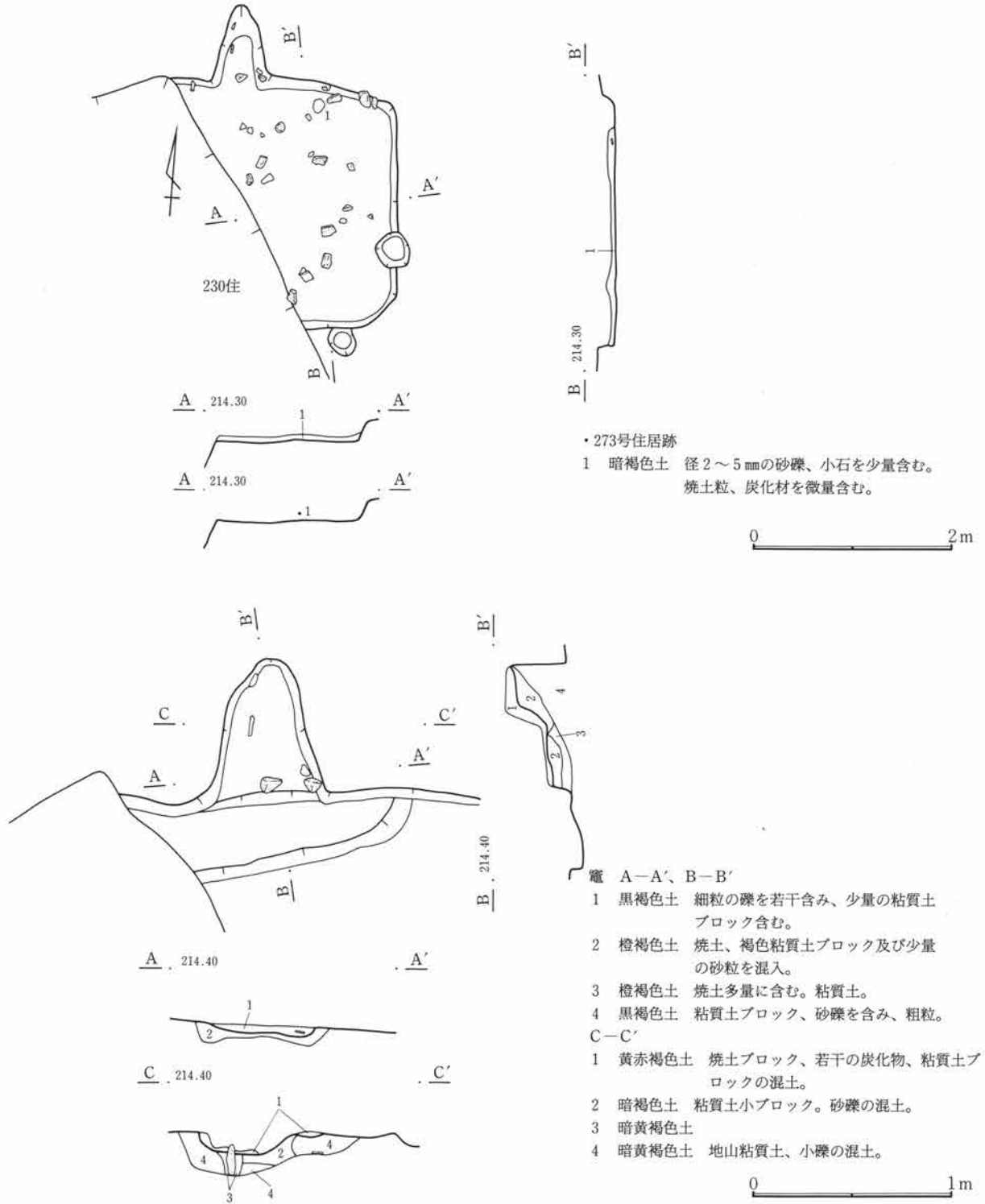
第401図 C-273号住居跡・竈
