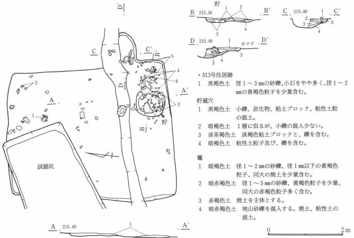
第485図 C-313号住居跡
