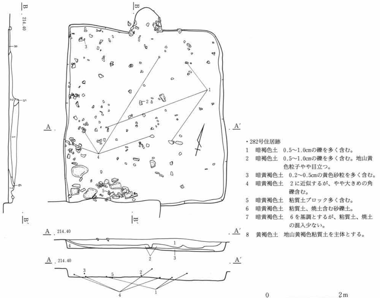
第417図 C-282号住居跡
