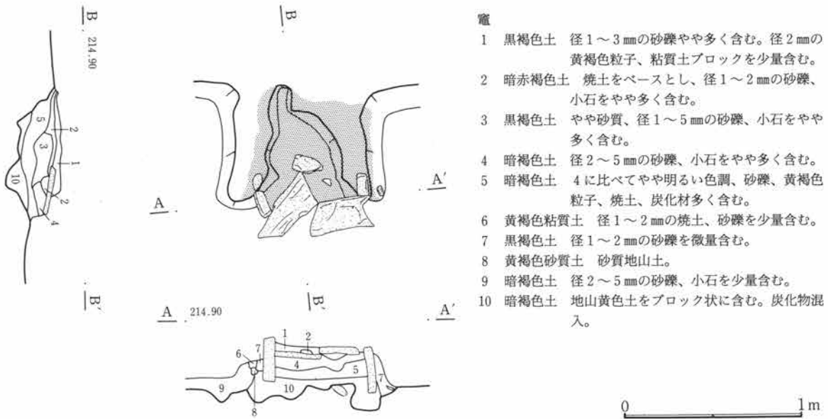
第456図 C-299号住居跡・竈
