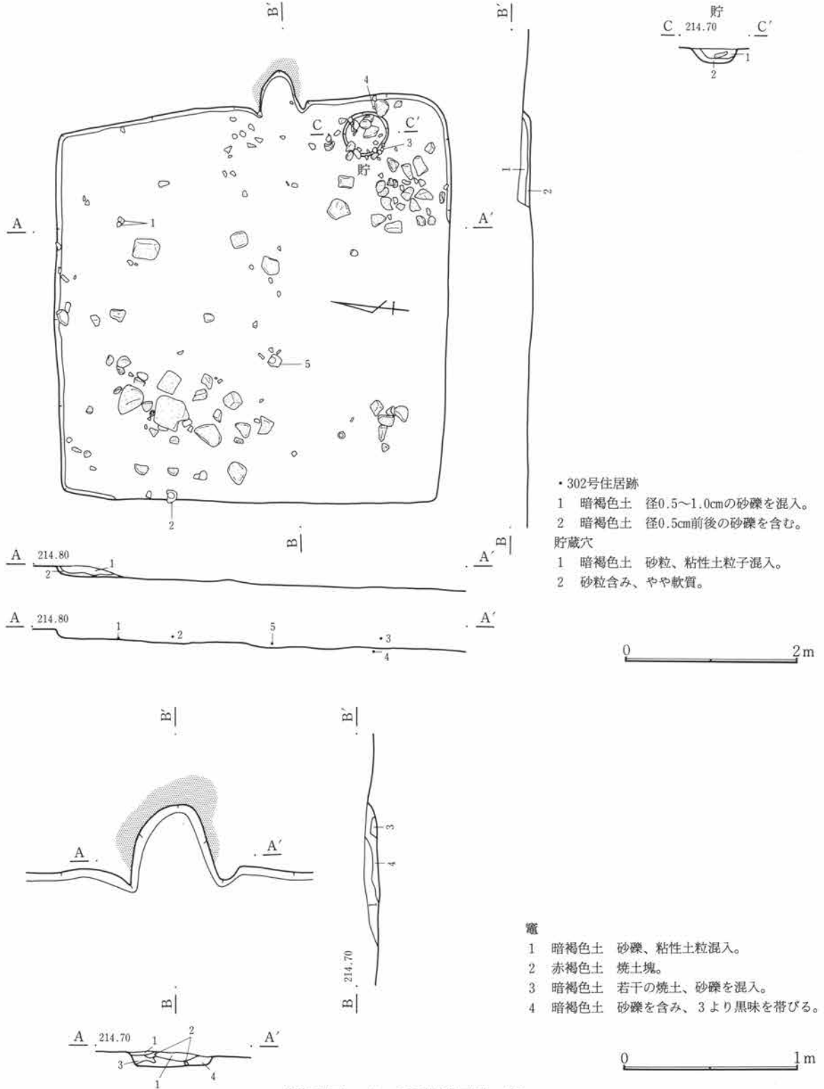
第460図 C-302号住居跡・竈
