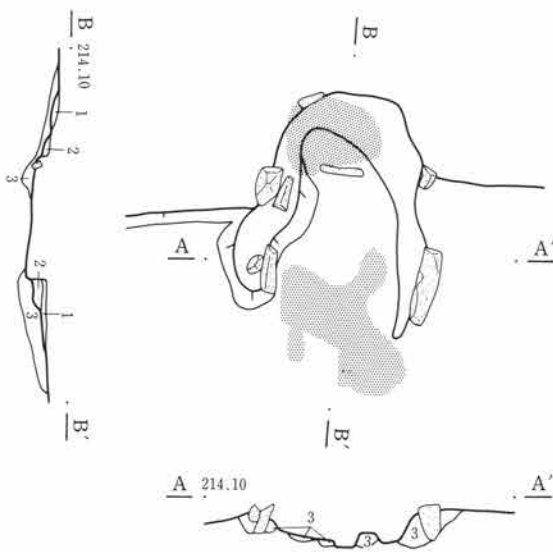
第280図 C-210号住居跡・竈
