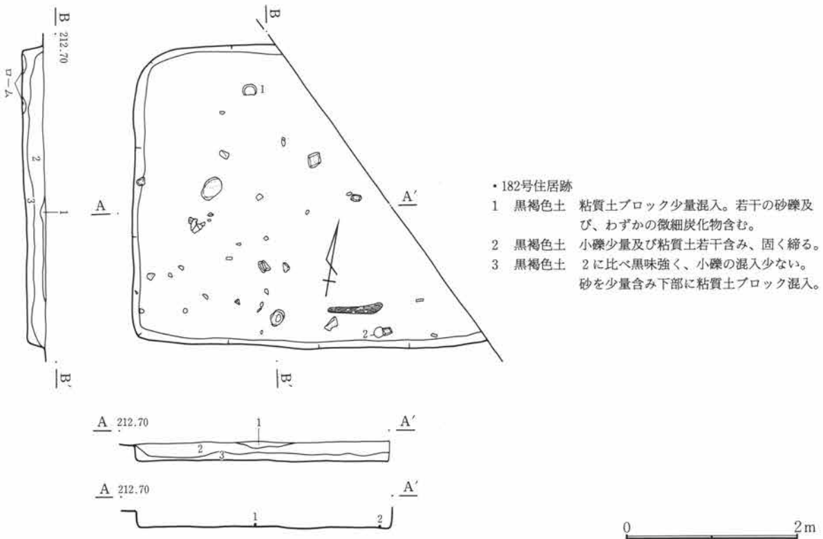
第253図 C-182号住居跡
