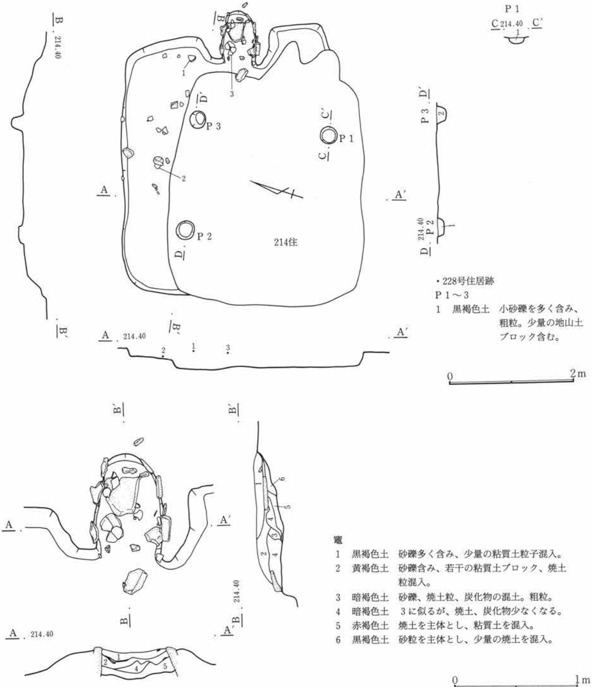
第307図 C-228号住居跡・竈
