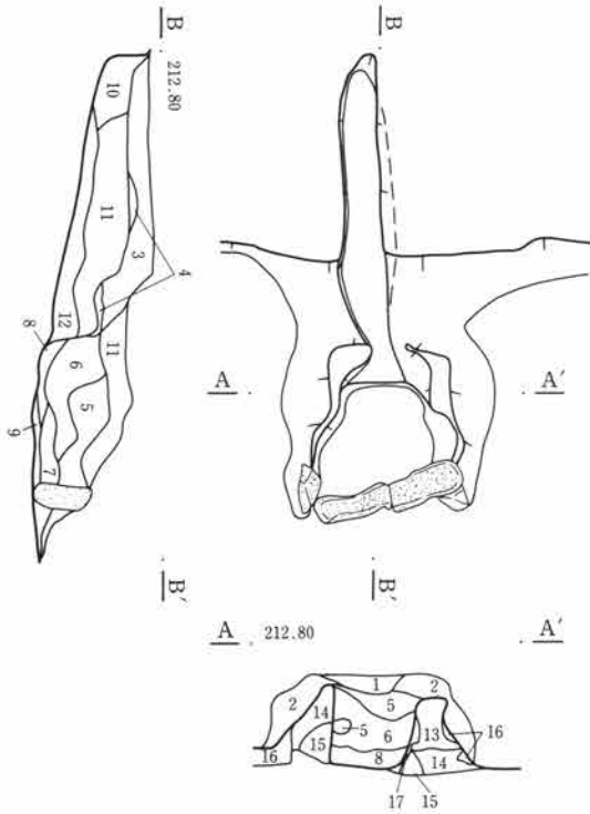
第124図 C-105号住居跡・竈
