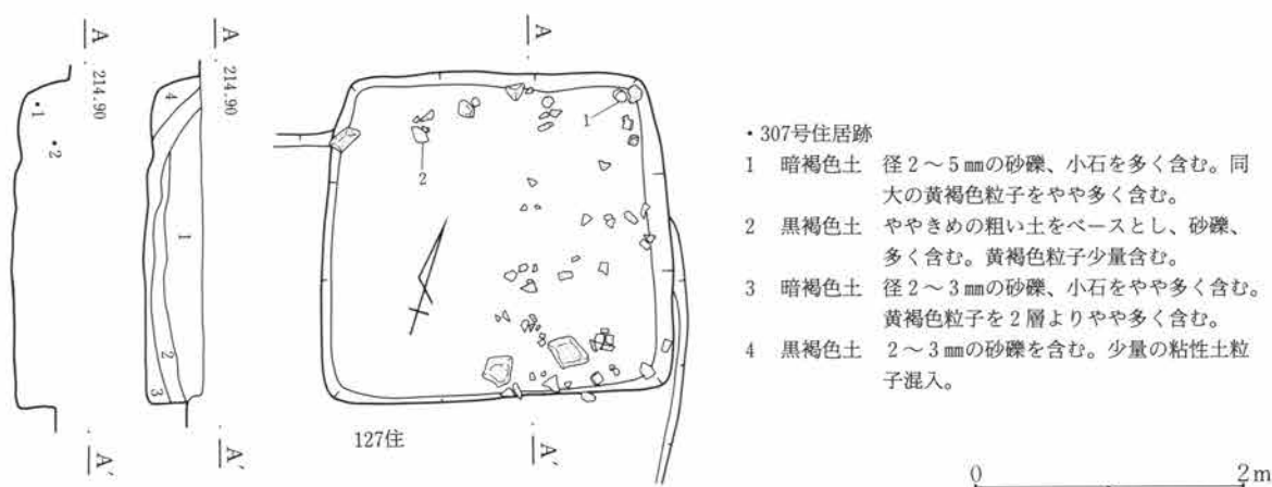
第469図 C-307号住居跡
