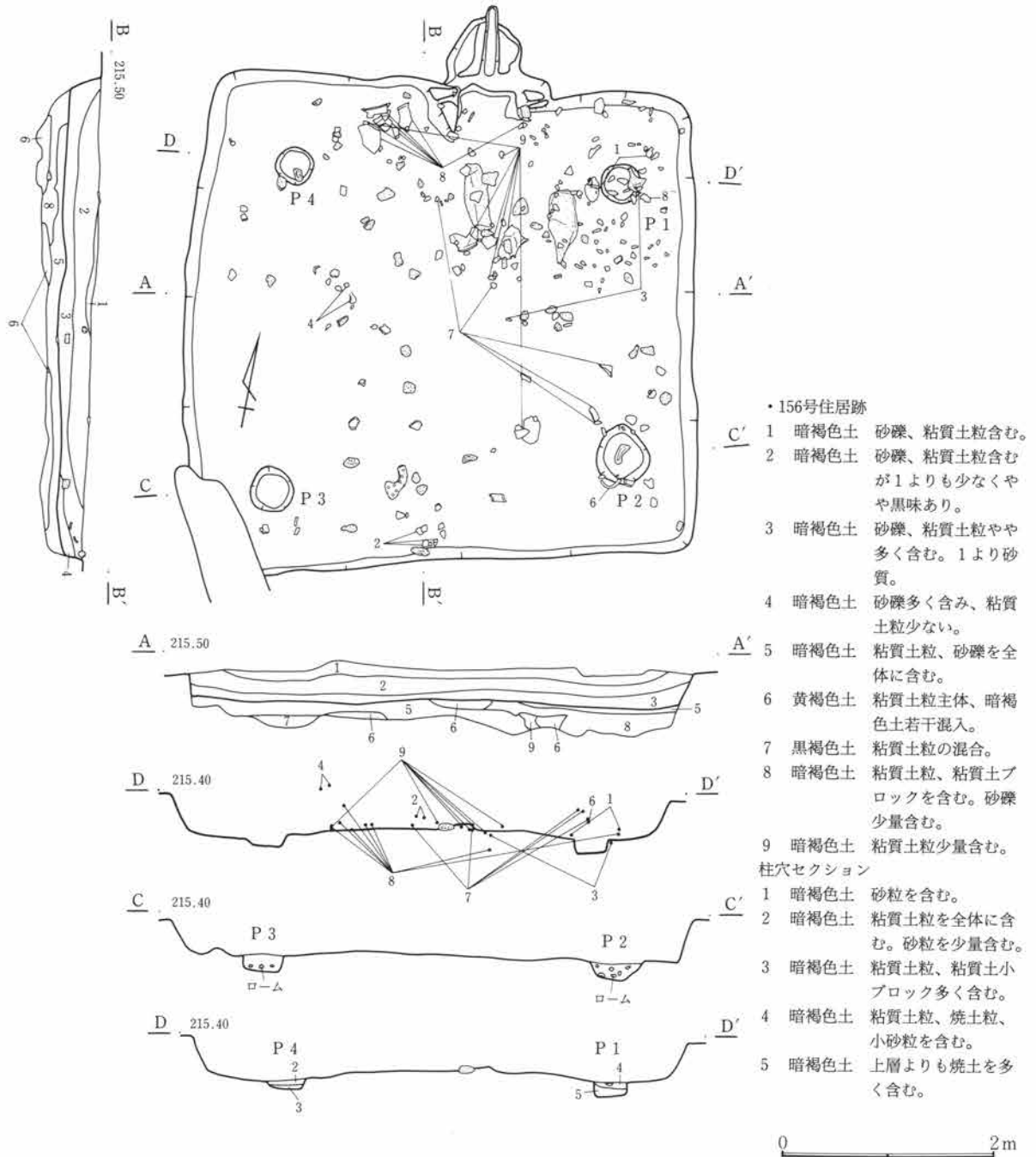
第215図 C—156号住居跡
