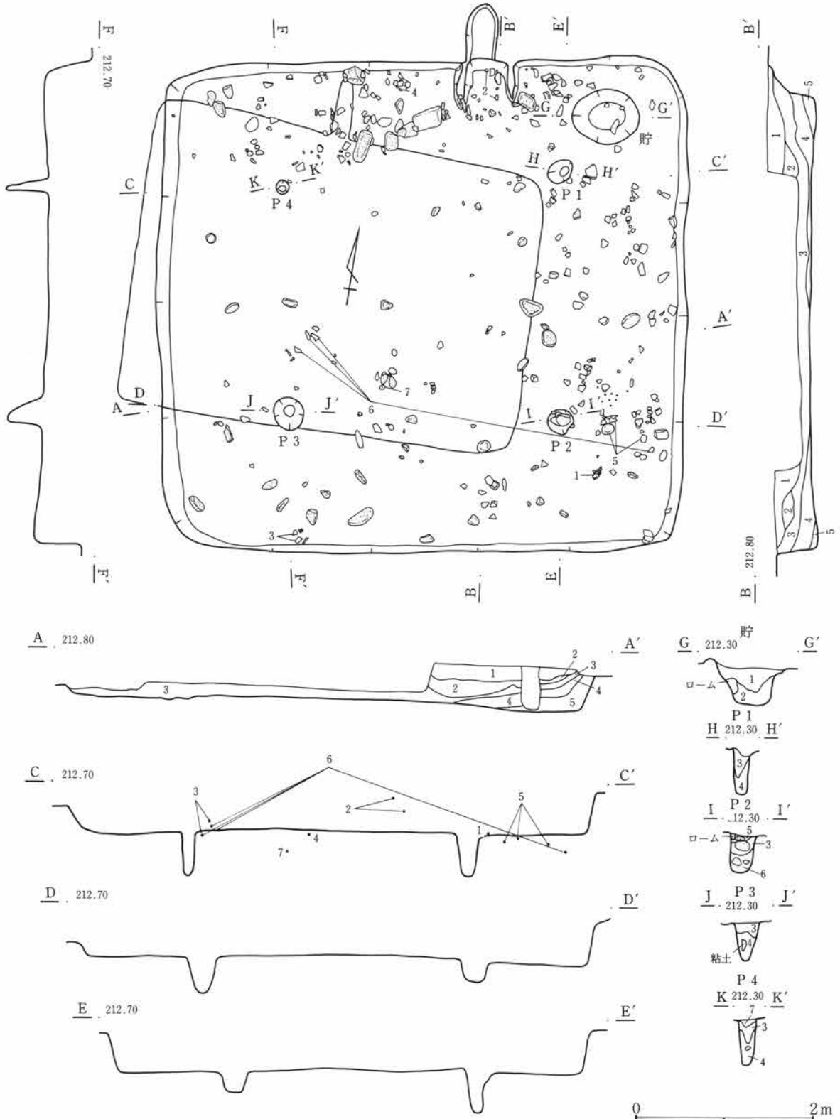
第126図 C-106号住居跡
