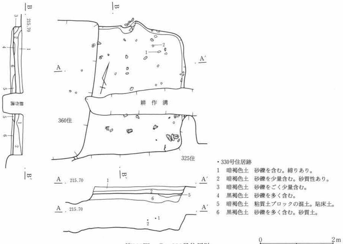
第525図 C-330号住居跡
