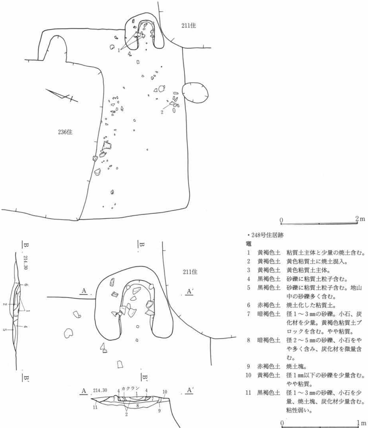
第345図 C-248号住居跡・竈
