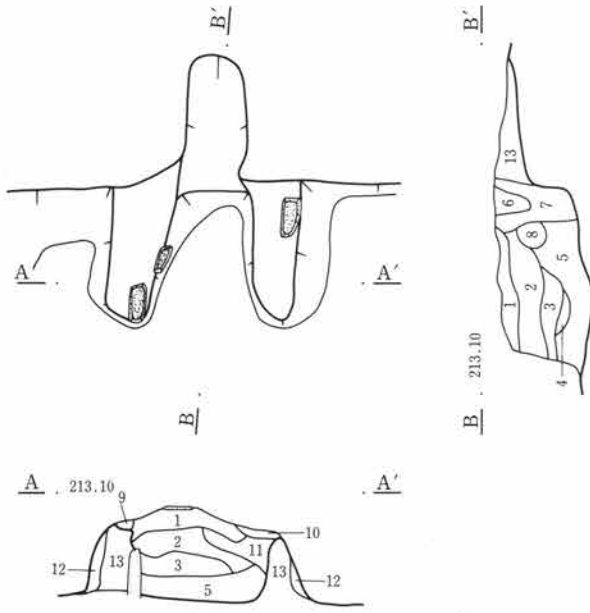
第48図 C-40号住居跡・竈
