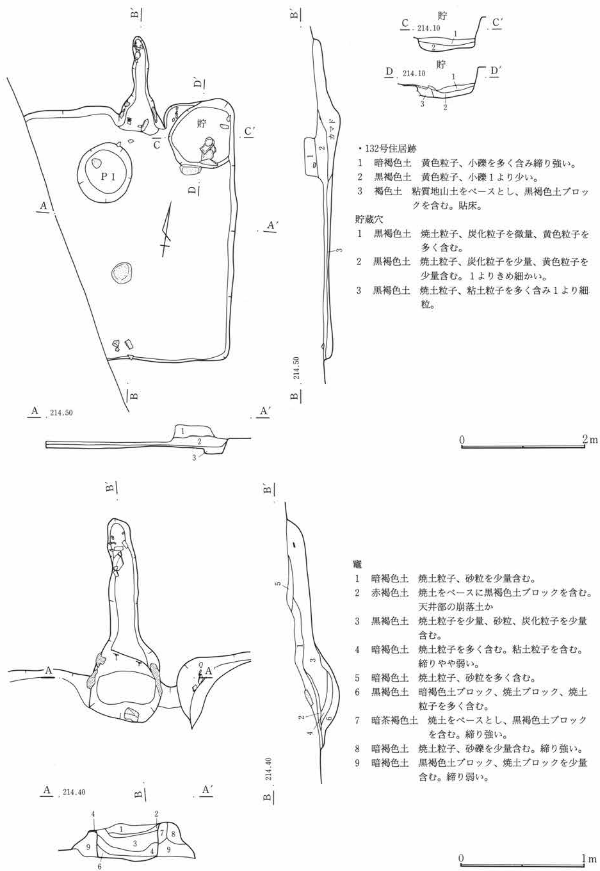
第174図 C-132号住居跡・電
