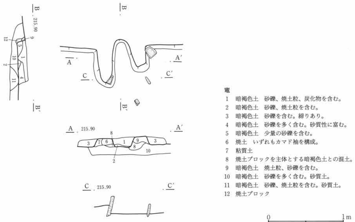
第529図 C-331号住居跡・竈
