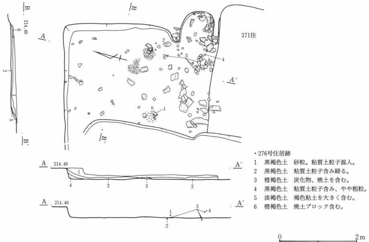
第407図 C-276号住居跡
