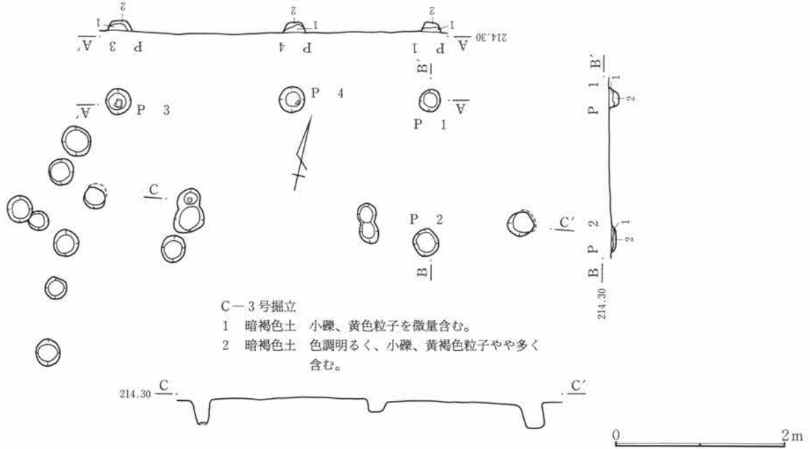
第625図 C-3号掘立
