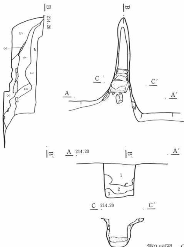
第248図 C-177号住居跡・竈
