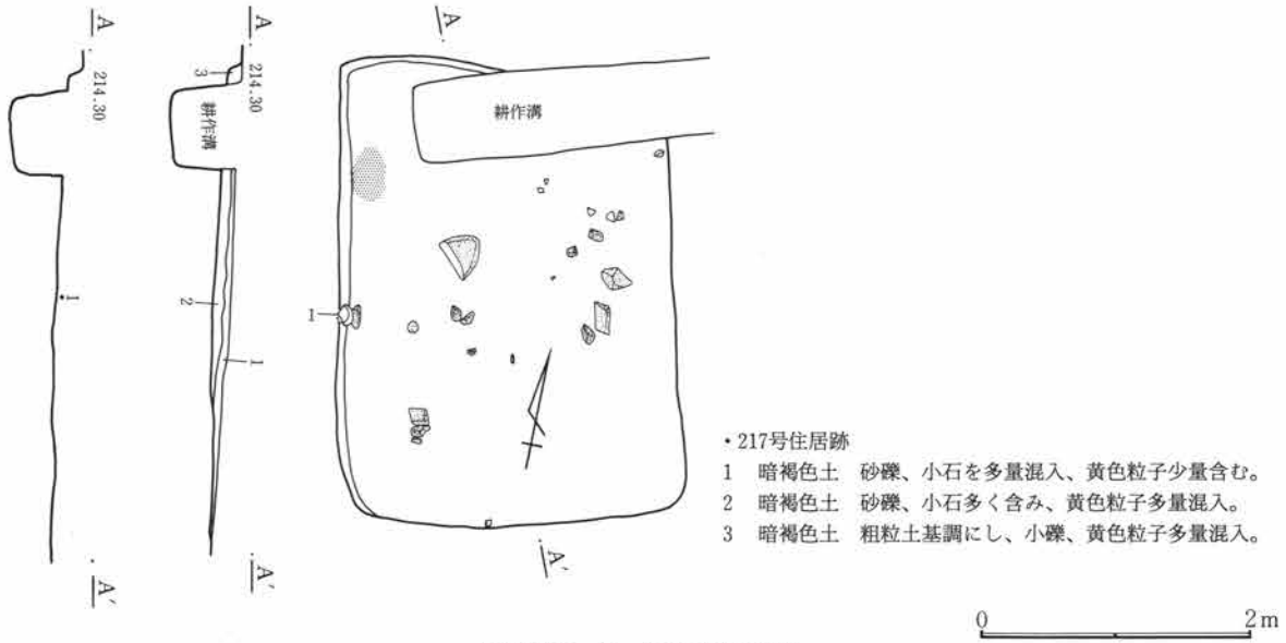
第293図 C-217号住居跡
