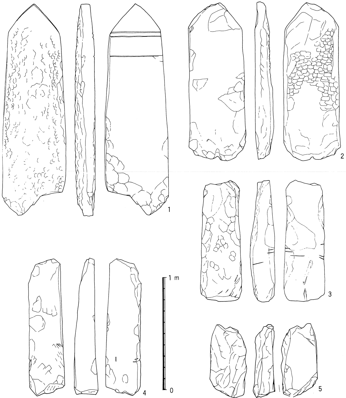
第8図 千塚西遺跡板碑実測図
