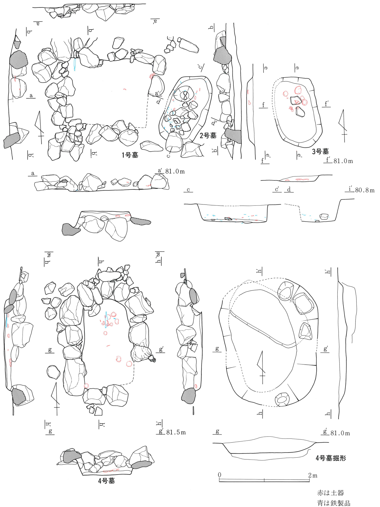
第4図 集石墓下部施設実測図 (1/50)
