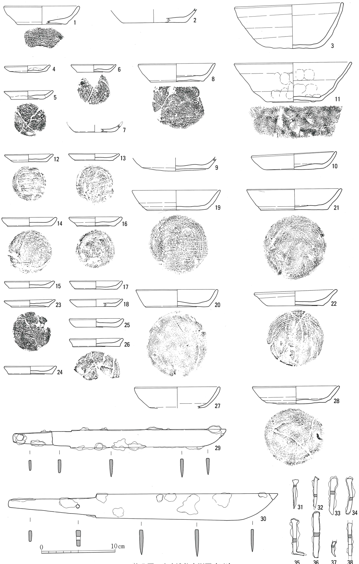
第5図 出土遺物実測図 (1/3)
