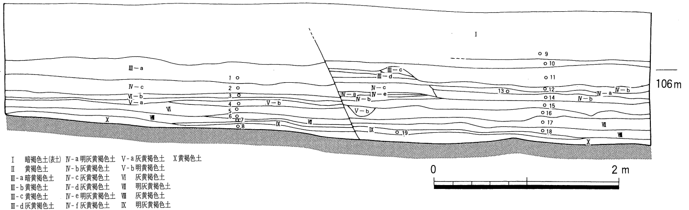
第33図 尾漕遺跡第5次調査区南壁面断面図 (1/40)
