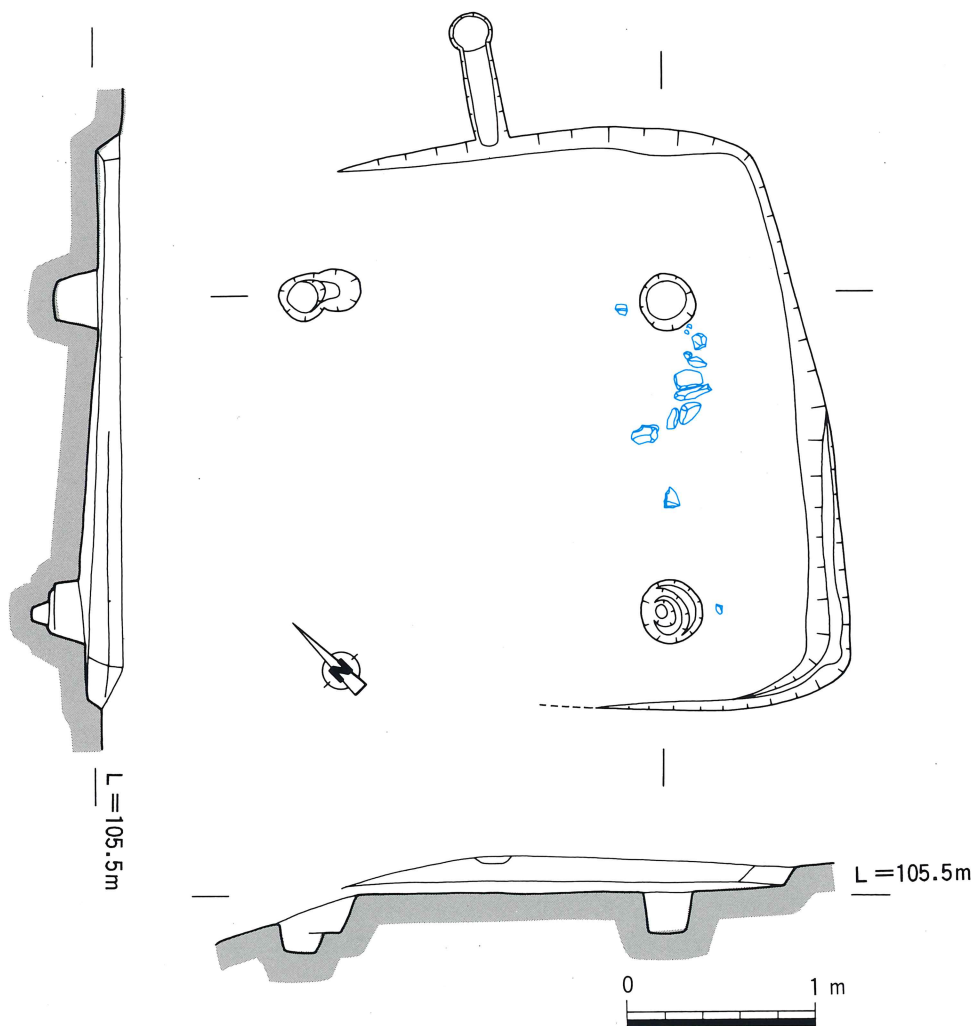
第3図 尾漕遺跡第2次調査区SH1平・断面図（ \frac{1}{40} ）
