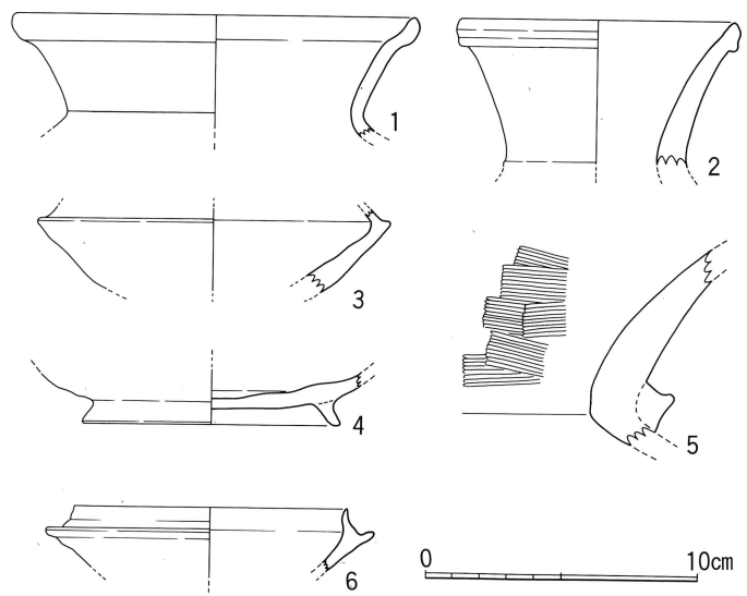
第22図 尾漕遺跡第5次調査区SD 1・2出土遺物実測図 (1/3)
