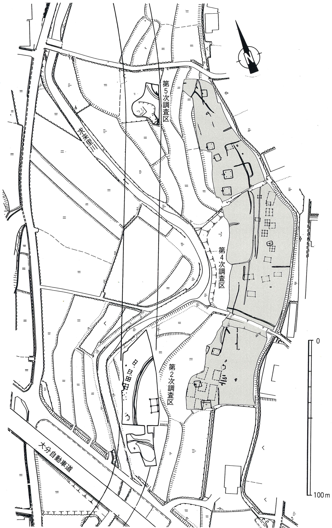
第24図 尾漕遺跡（第2・4・5次調査区）位置図（ \frac{1}{1500} ）
