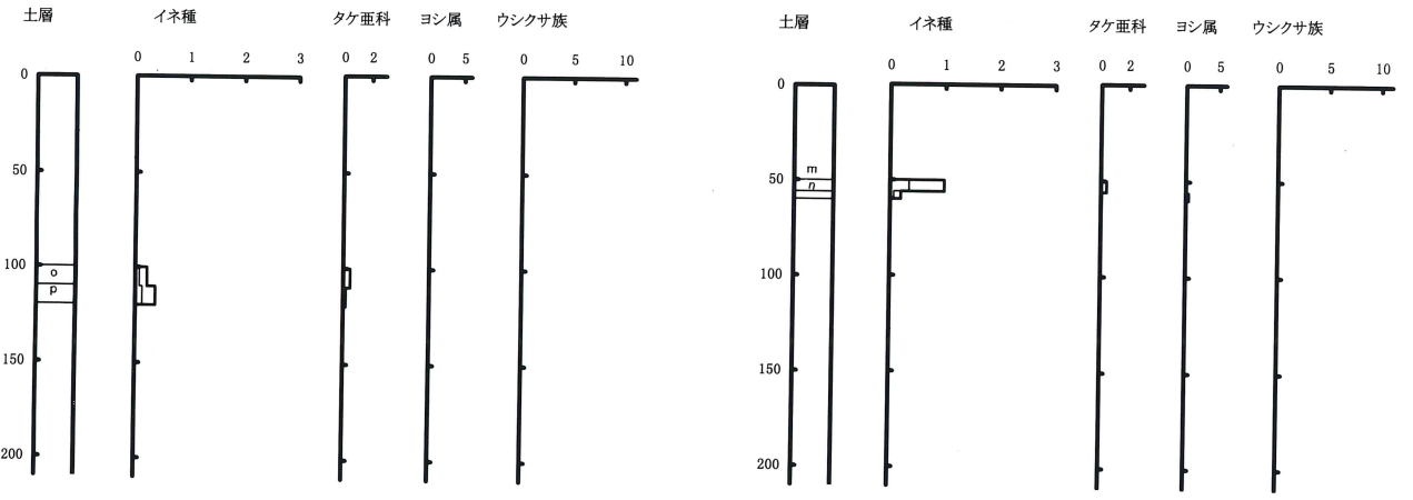
第28図 尾漕遺跡第2次調査区東北部壁面土壌（第27図）のプラント・オパール密度から推定した埋没植物量（t/10a/cm）
