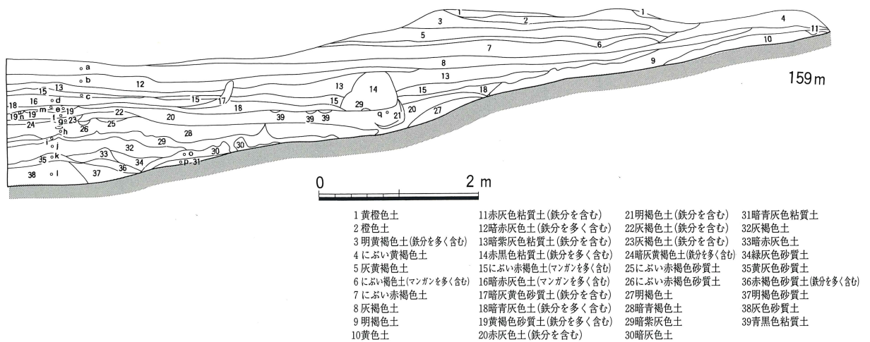
第27図 尾漕遺跡第2次調査区東北部壁面断面図
