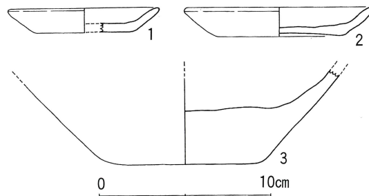
第15図 尾漕遺跡第2次調査区出土遺物実測図 (1/3)
