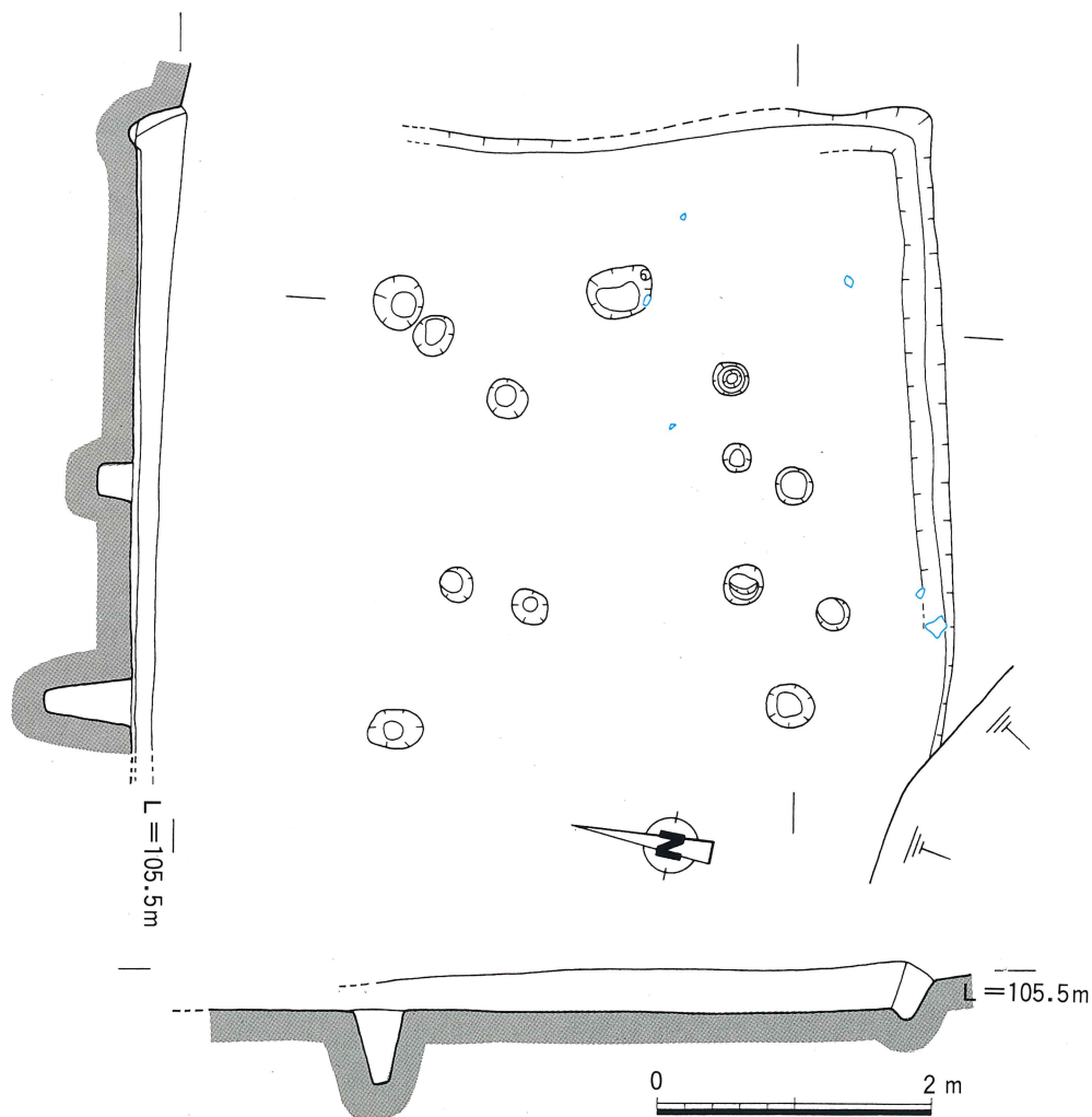
第19図 尾漕遺跡第5次調査区SH 2平・断面図 (1/60)
