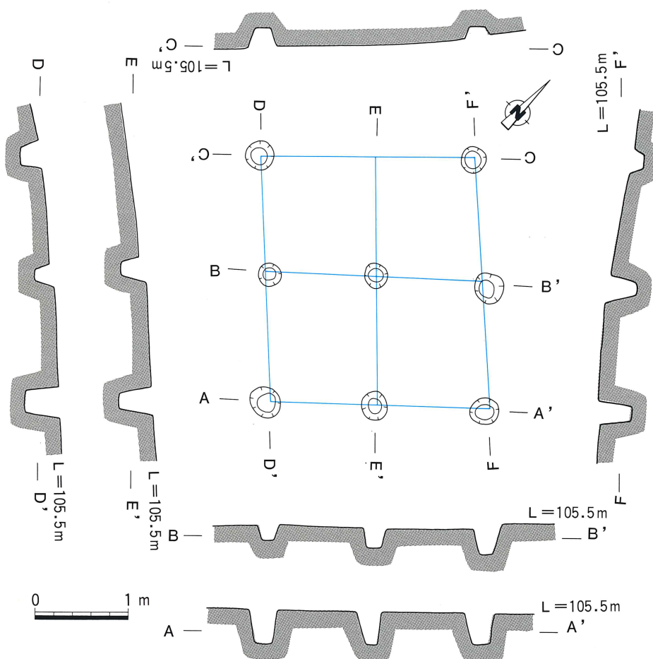
第13図 尾漕遺跡第2次調査区SB 4平・断面図 (1/60)
