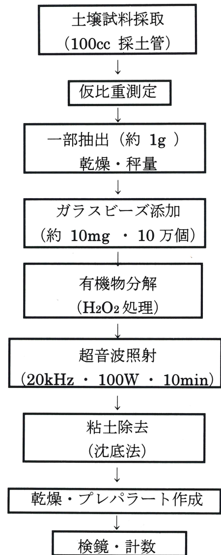
第26図 プラント・オパール 定量分析手順
