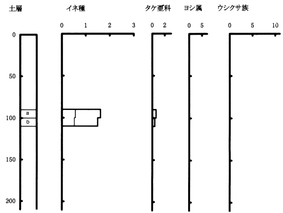
第32図 尾漕遺跡第2次調査区南北連結部東部壁面土壌(第31図)のプラント・オパール密度から推定した埋没植物量 (t/10a/cm)
