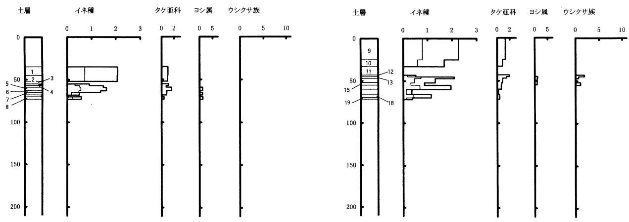
第34図 尾漕遺跡第5次調査区南壁面土壌（第33図）のプラント・オパール密度から推定した埋没植物量（t/10a/cm）
