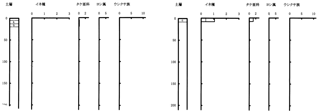
第30図 尾漕遺跡第2次調査区SD2土壌(第8図)のプラント・オパール密度から推定した埋没植物量 (t/10a/cm)
