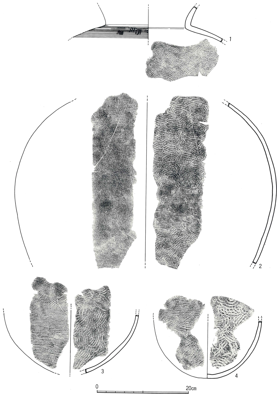
第7図 尾漕遺跡第2次調査区SD1出土遺物実測図(2) (1/4)
