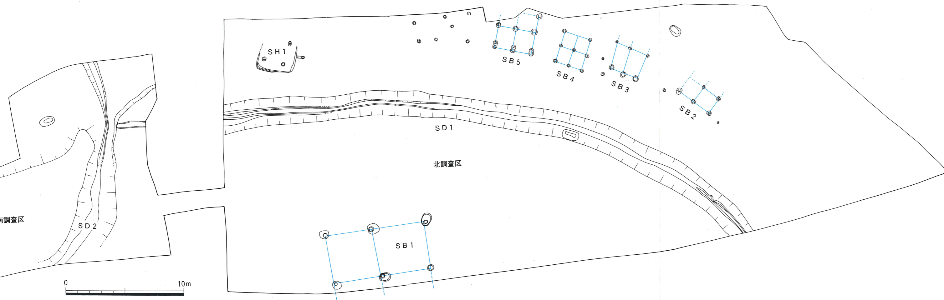
第4図 尾漕遺跡第2調査区遺構配置図 (1/200)
