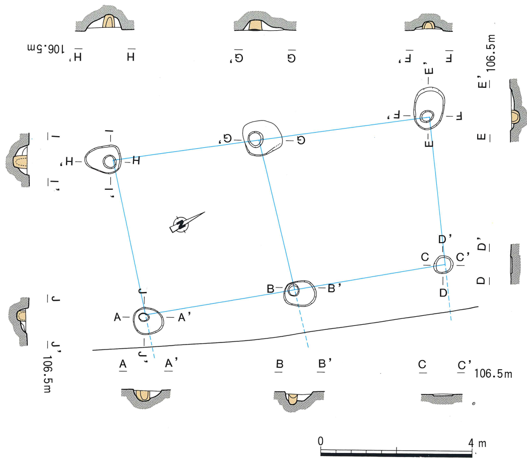
第9図 尾漕遺跡第2次調査区S B 1平・断面図 (1/100)
