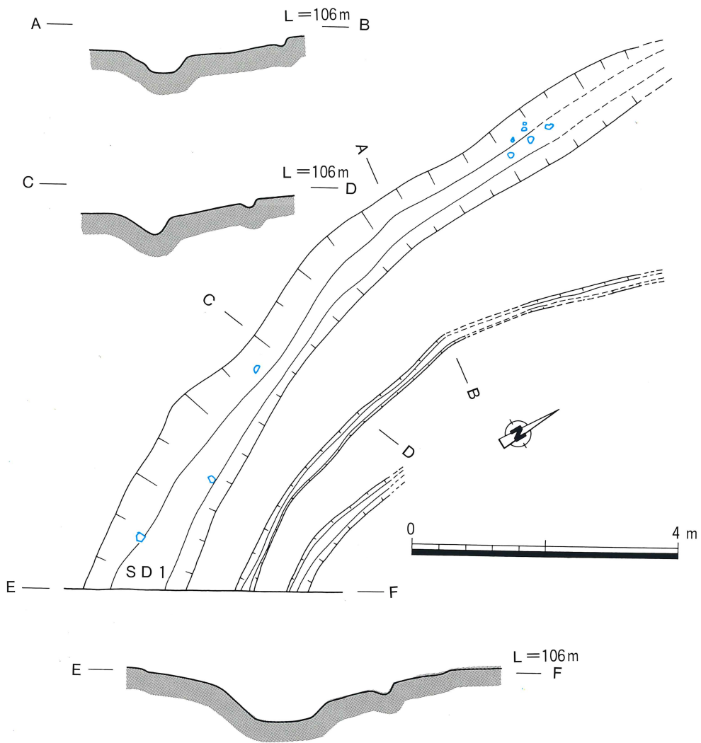
第21図 尾漕遺跡第5次調査区溝状遺構平・断面図 (1/80)
