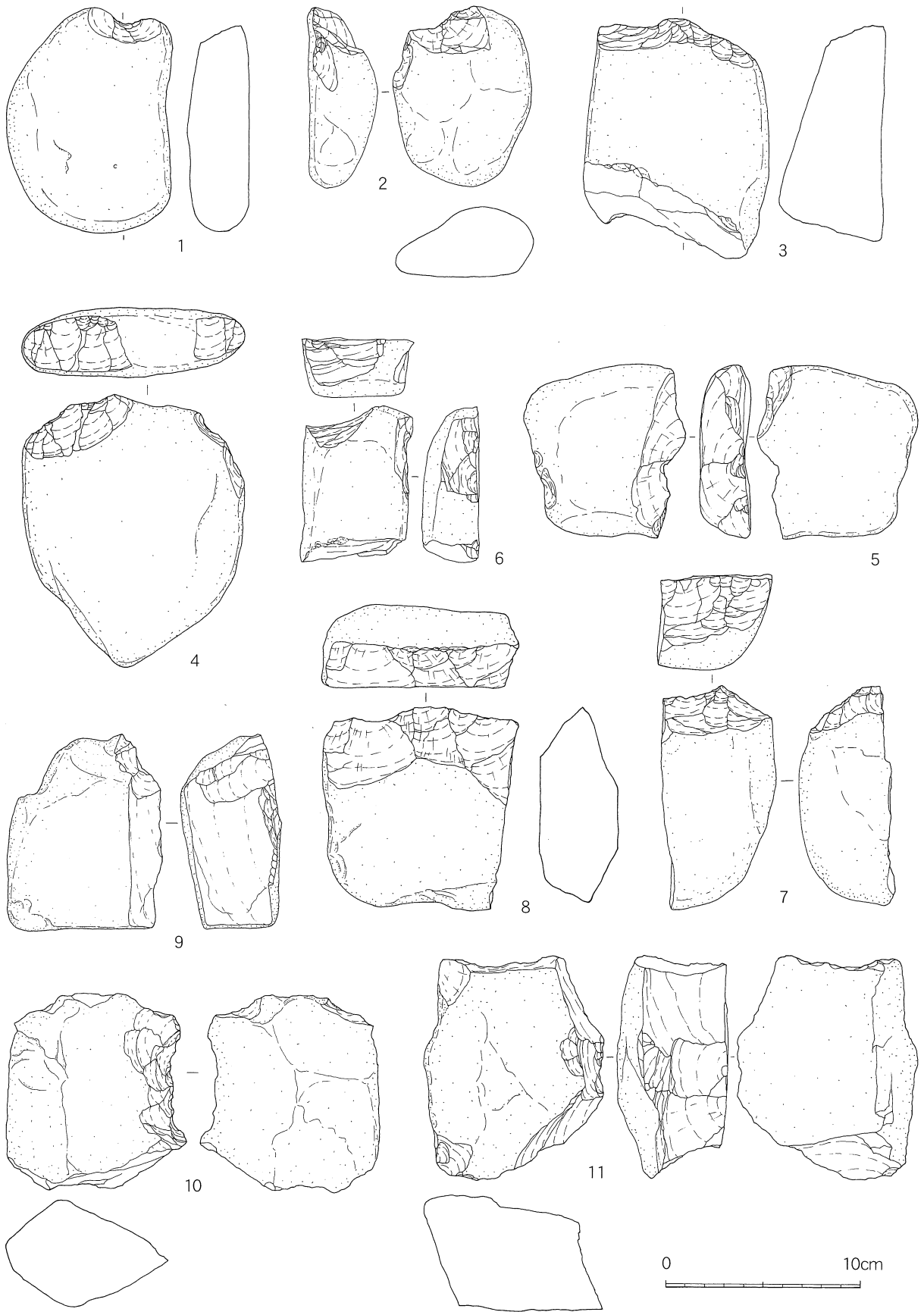
第30図 片刃礫器実測図（その1）
