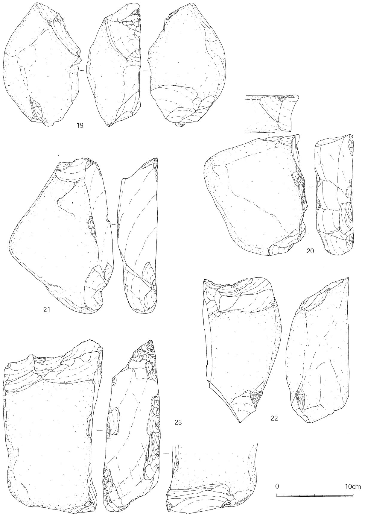
第32図 片刃礫器実測図（その3）
