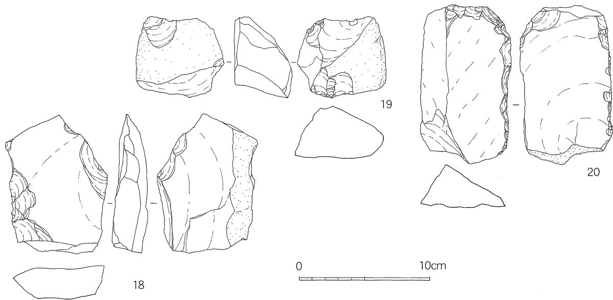
第38図 大型（粗製）剥片石器実測図（その3）
