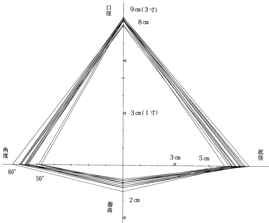
第11図 土師質土器 小皿法量グラフ
