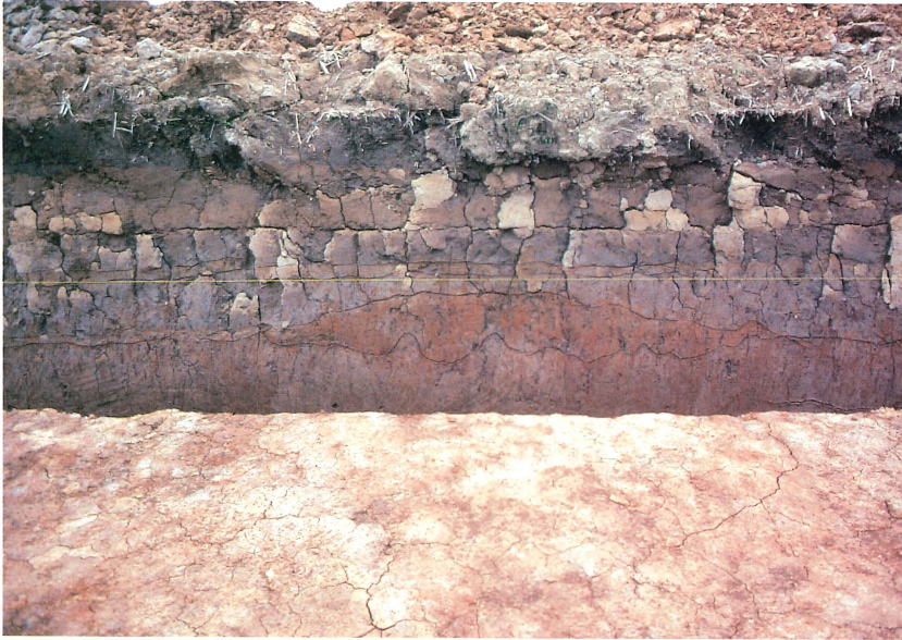
植田条里遺跡F区 南壁土層
