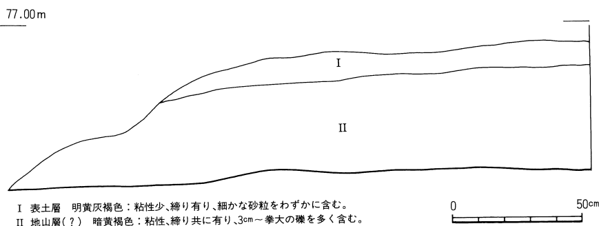
第4図 尾鼻遺跡土層断面図
