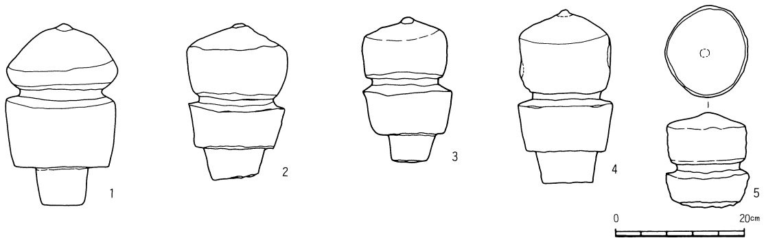
第9図 風・空輪実測図
