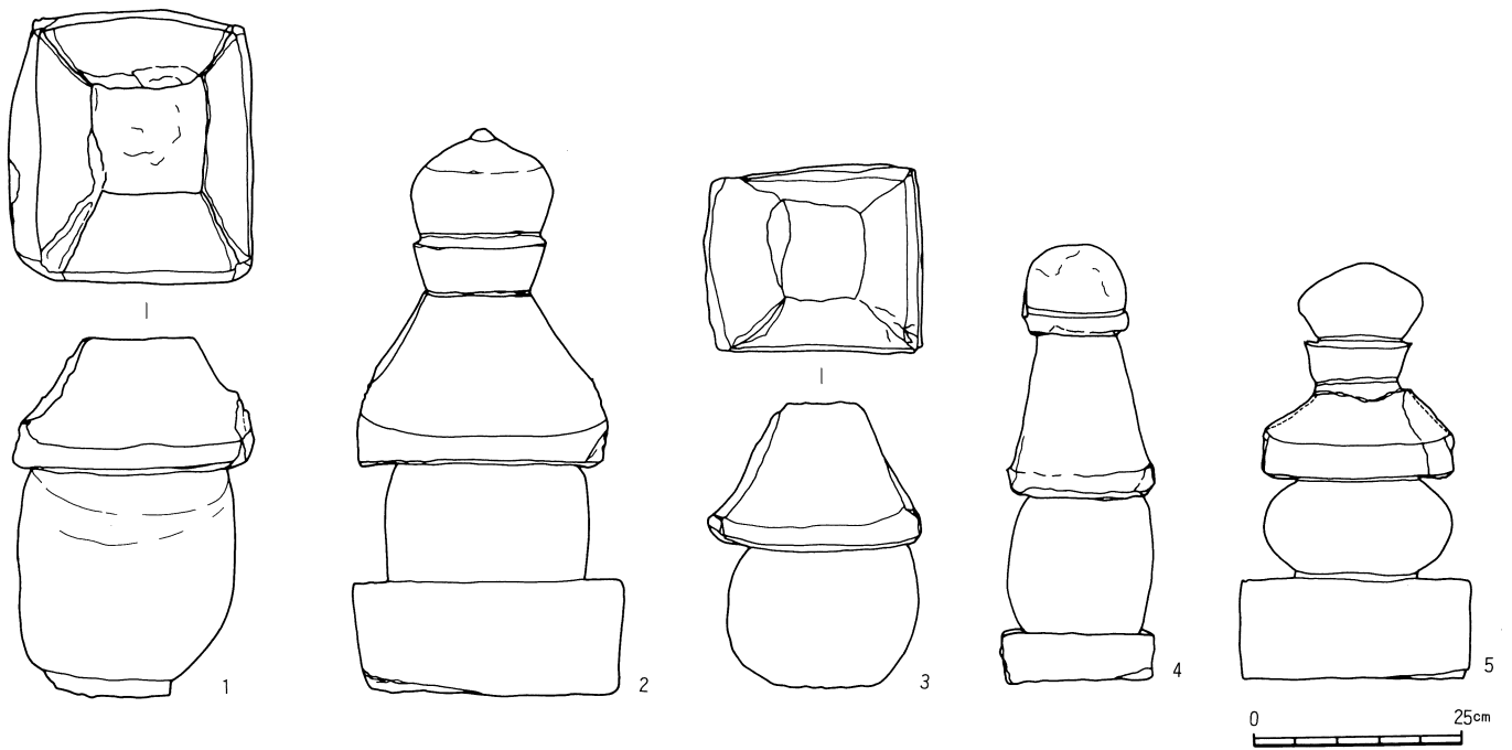
第8図 一石五輪塔実測図
