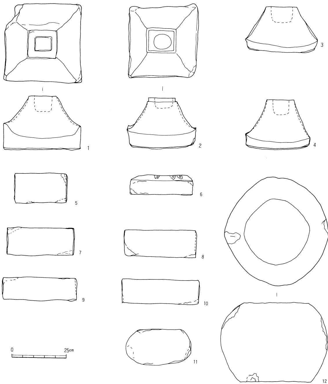
第10図 火輪・水輪・地輪実測図
