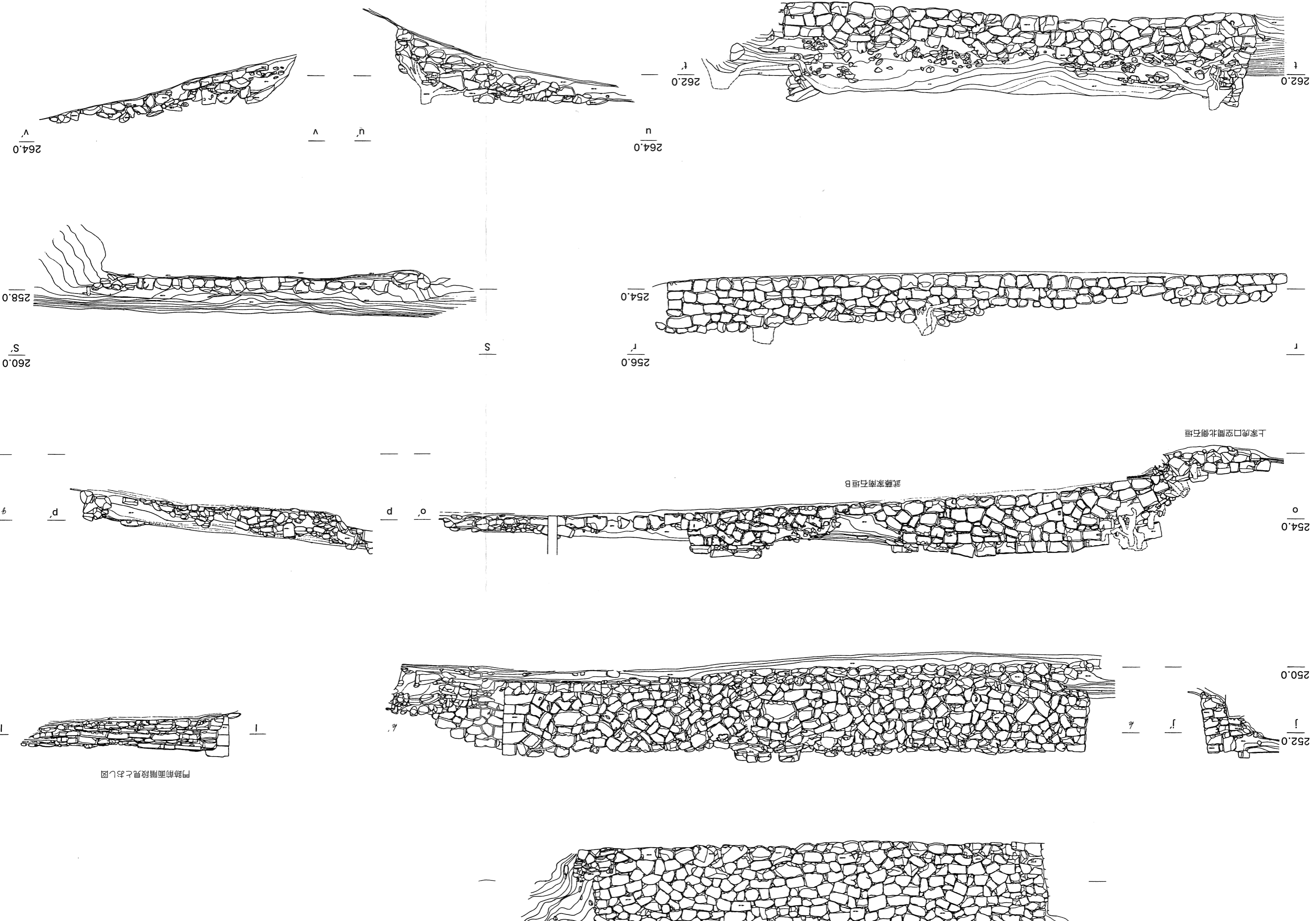
付図7 上家・武藤家屋敷跡石垣立面図
