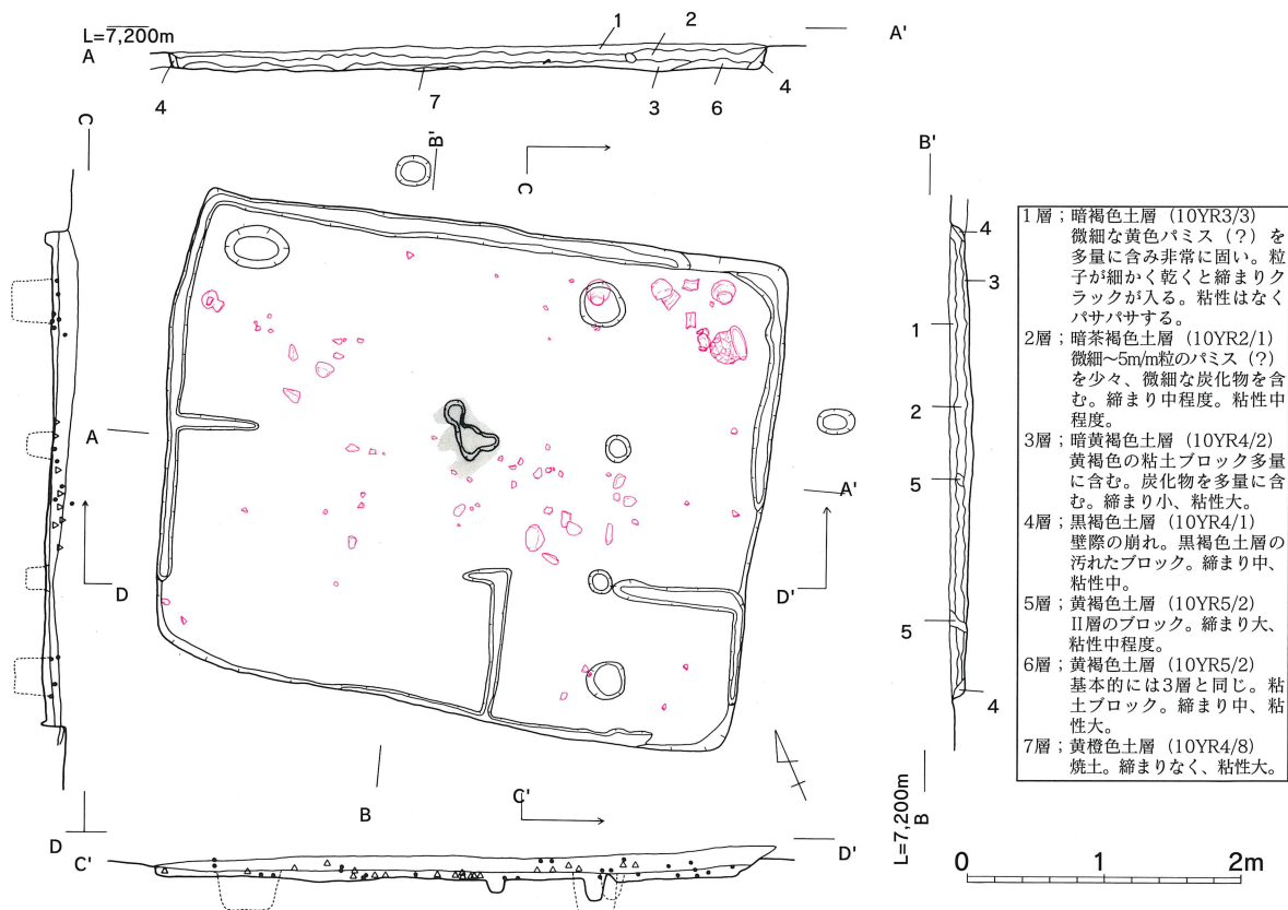
図5 毛井遺跡A地区竪穴 SH-01
