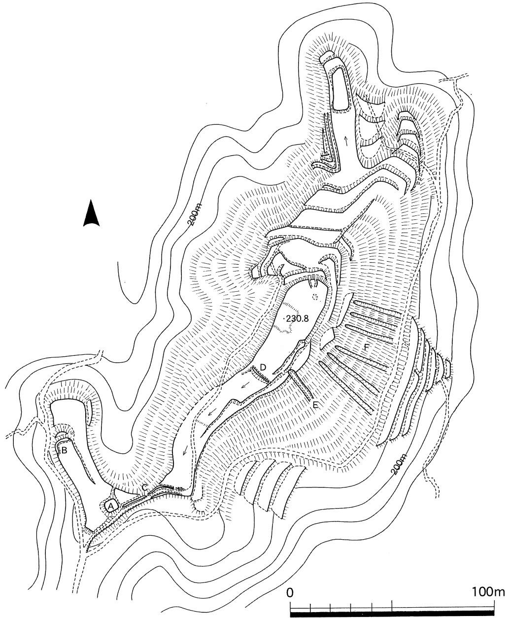
高尾城縄張図(原図:大分市教育委員会 玉永光洋氏)
