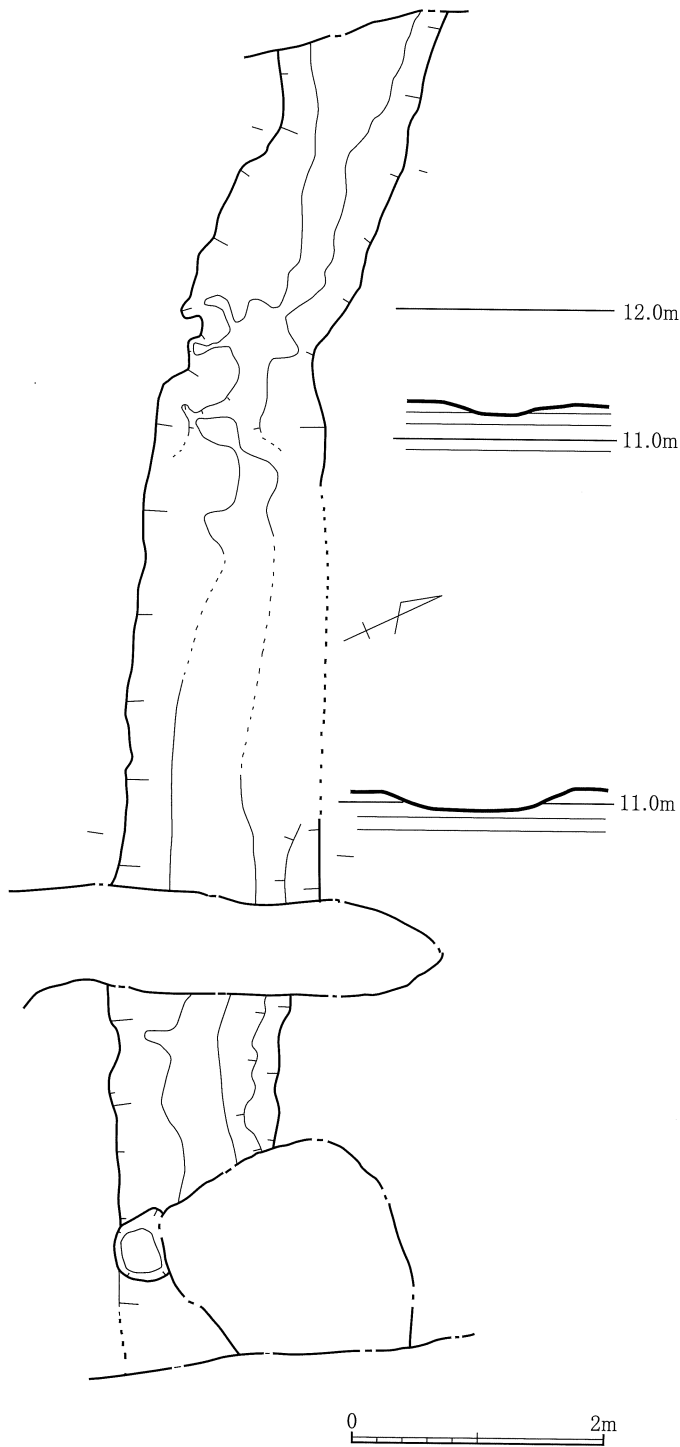
第29図 SD 2 実測図
