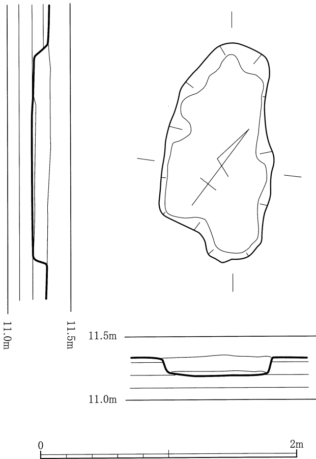
第23図 SK 7 実測図
