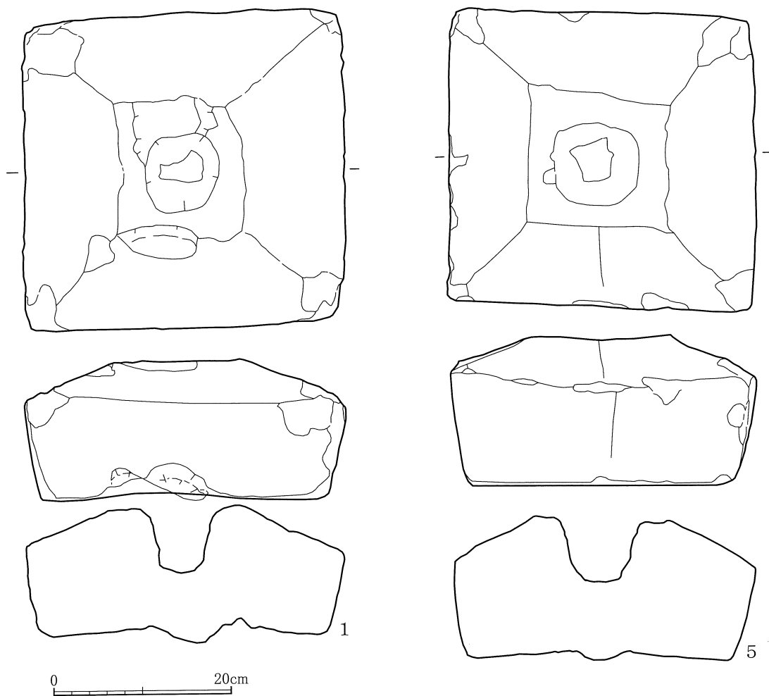
第44図 SE 3 出土遺物実測図
