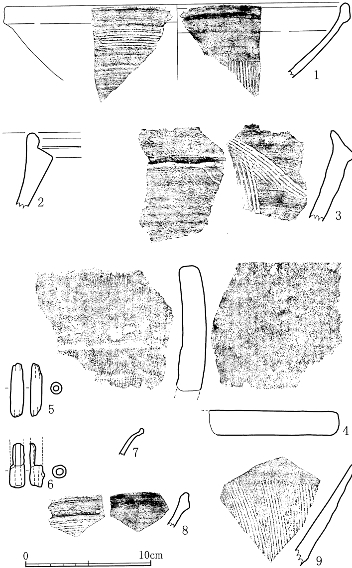
第33図 SD 4 出土遺物実測図
