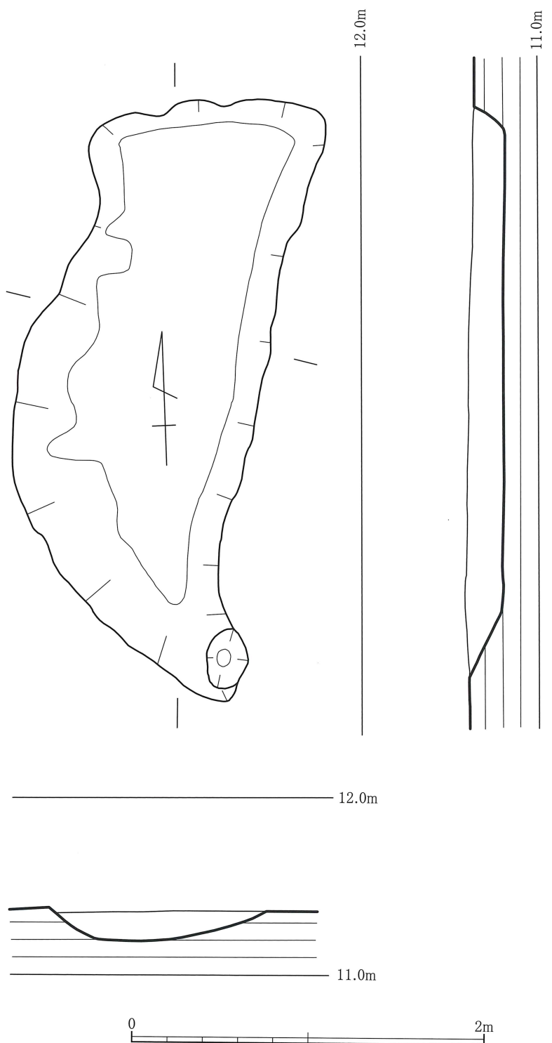
第17図 SK2実測図
