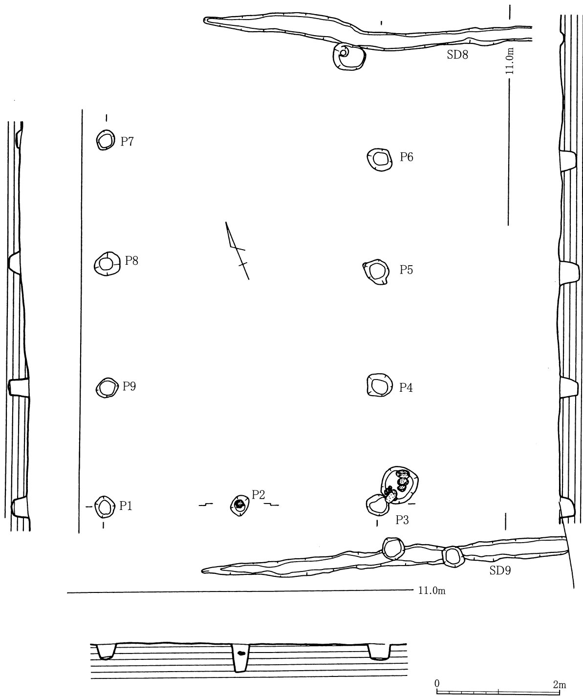
第7図 SB2実測図
