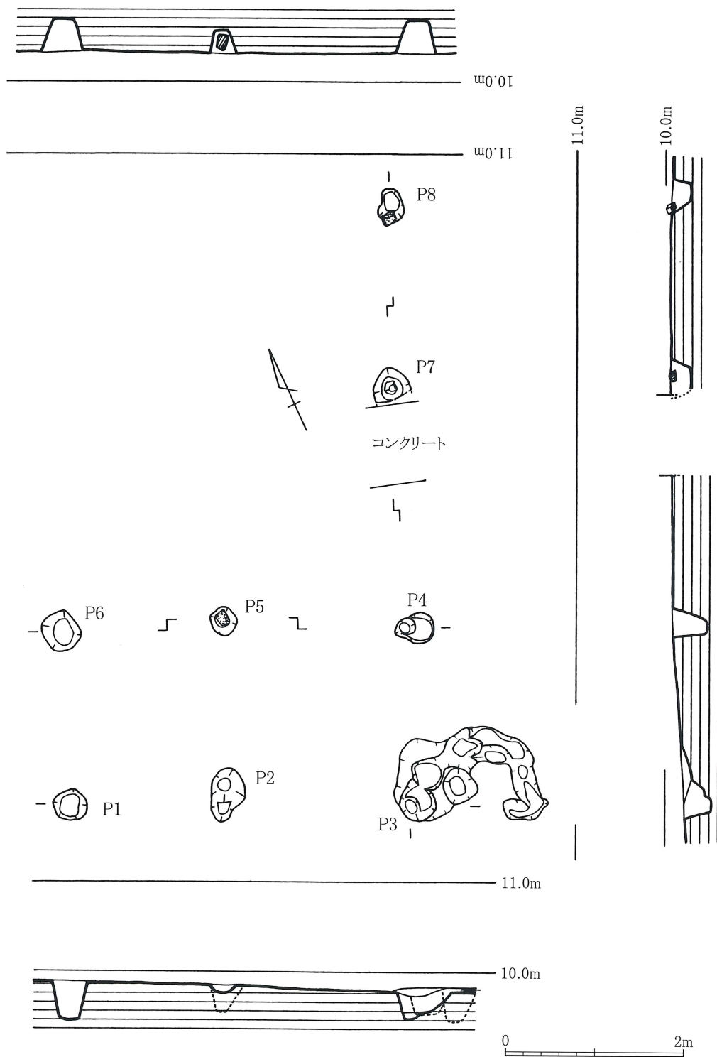
第10図 SB 5 実測図
