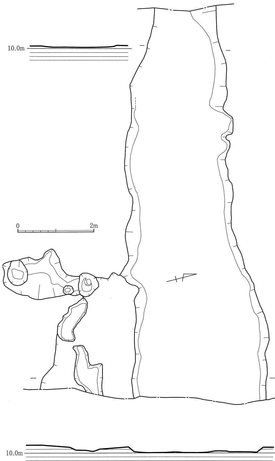
第36図 SD 7 実測図
