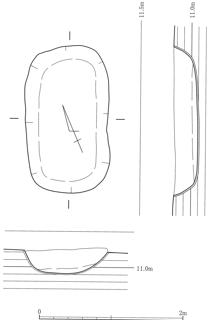
第14図 SK1 実測図
