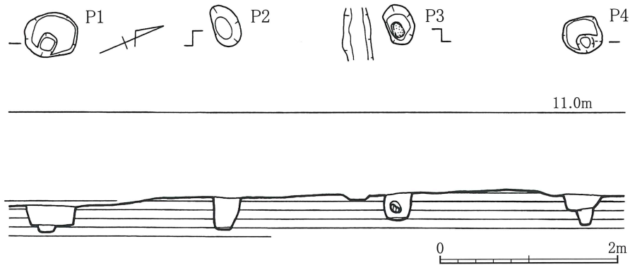
第8図 SB3実測図
