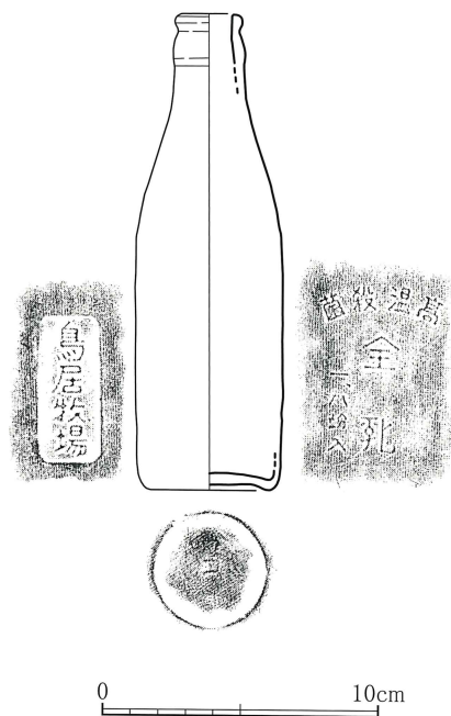
第21図 SK 5 出土遺物実測図
