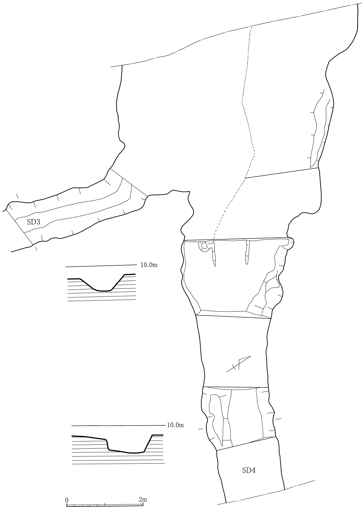
第31図 SD3・SD4実測図
