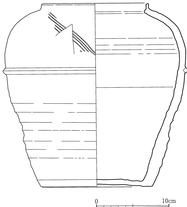
第43図 SE 3 出土遺物実測図
