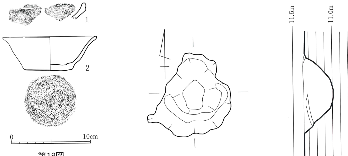
第18図 SK 3 出土遺物実測図
