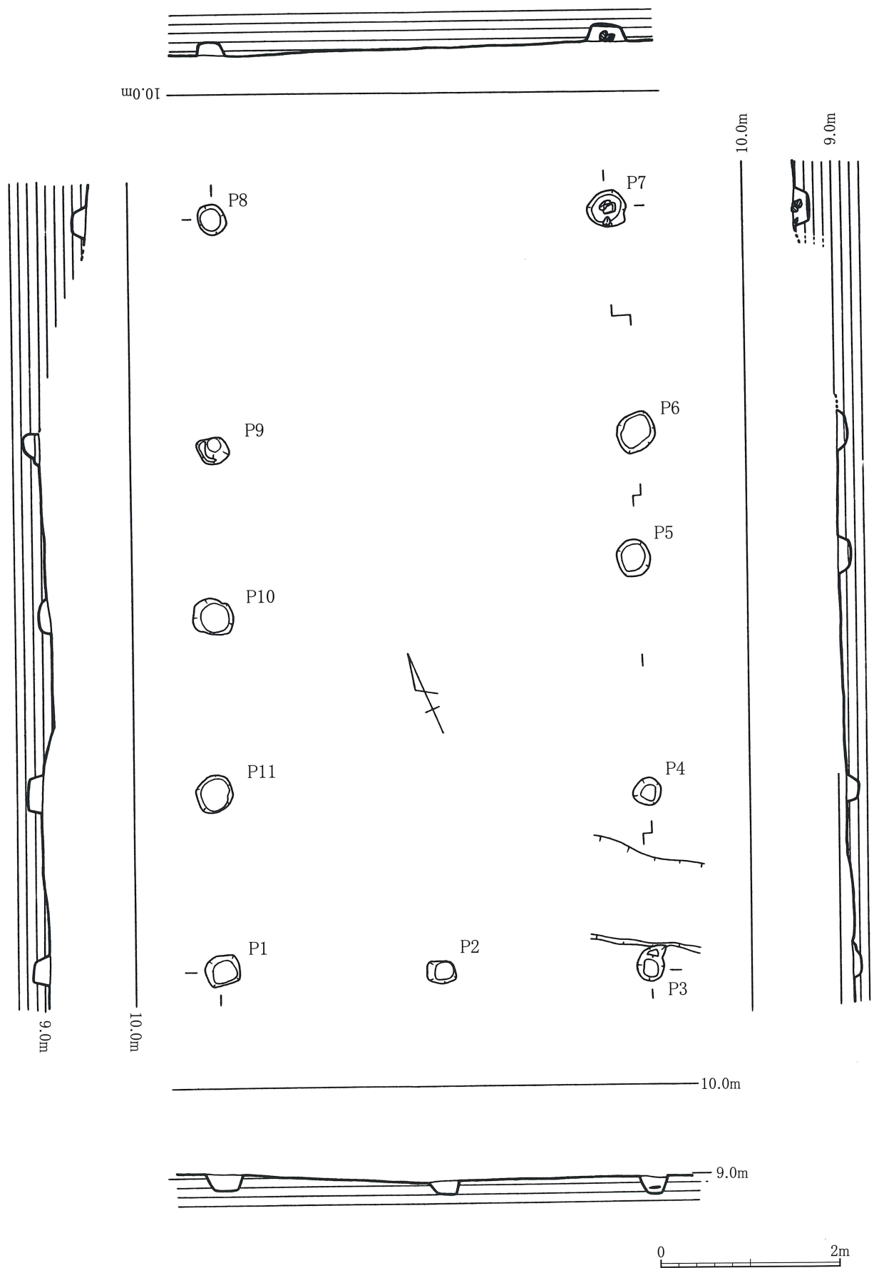
第13图 SB 8 实测图
