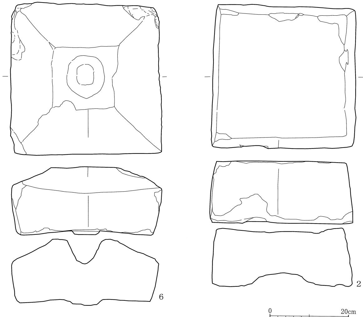
第46図 SE 3 出土遺物実測図
