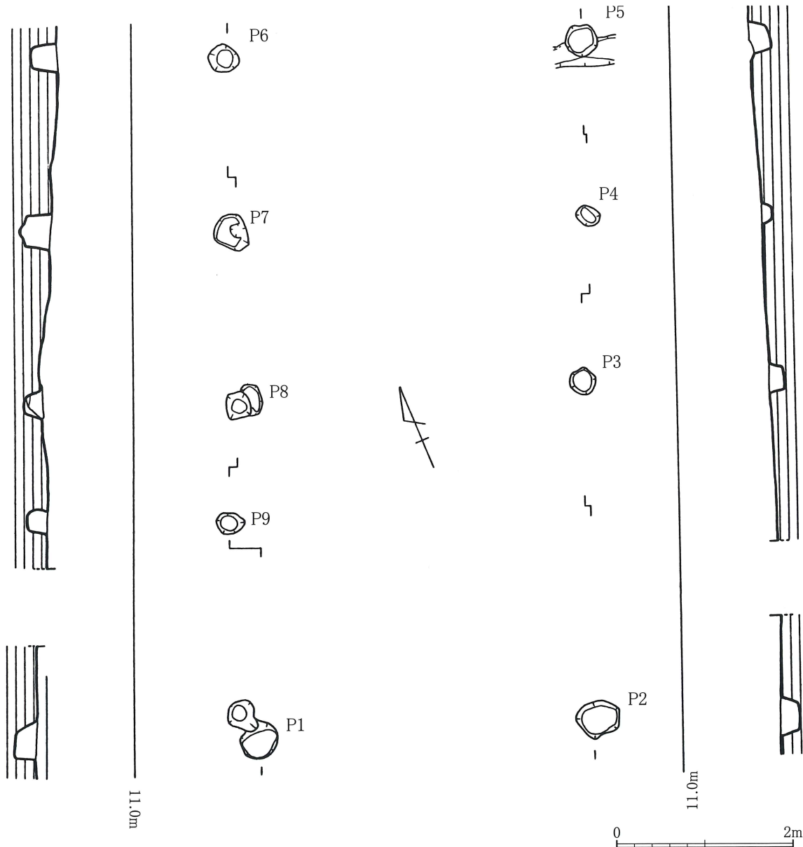
第9図 SB4実測図
