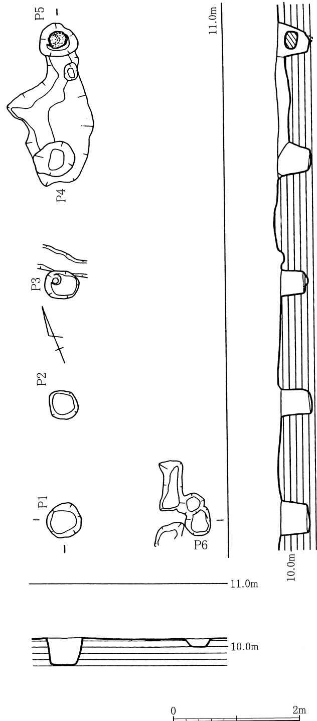
第6図 SB1実測図
