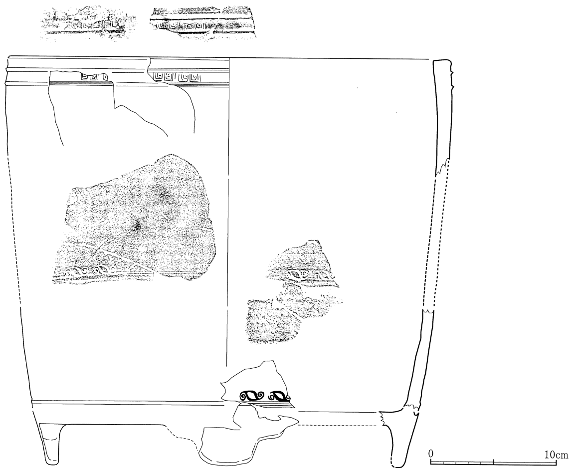
第42図 SE 3 出土遺物実測図
