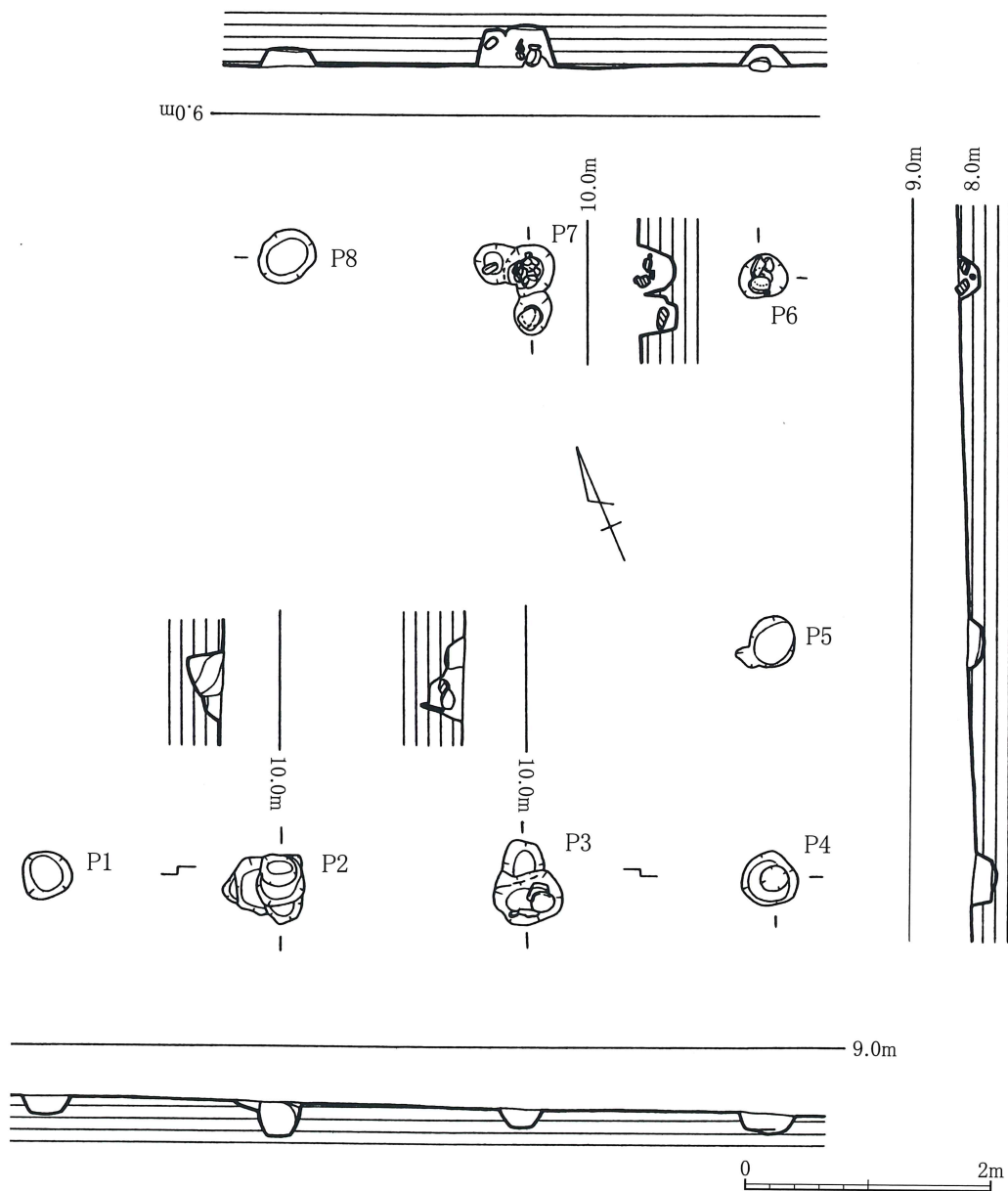
第12図 SB7 実測図
