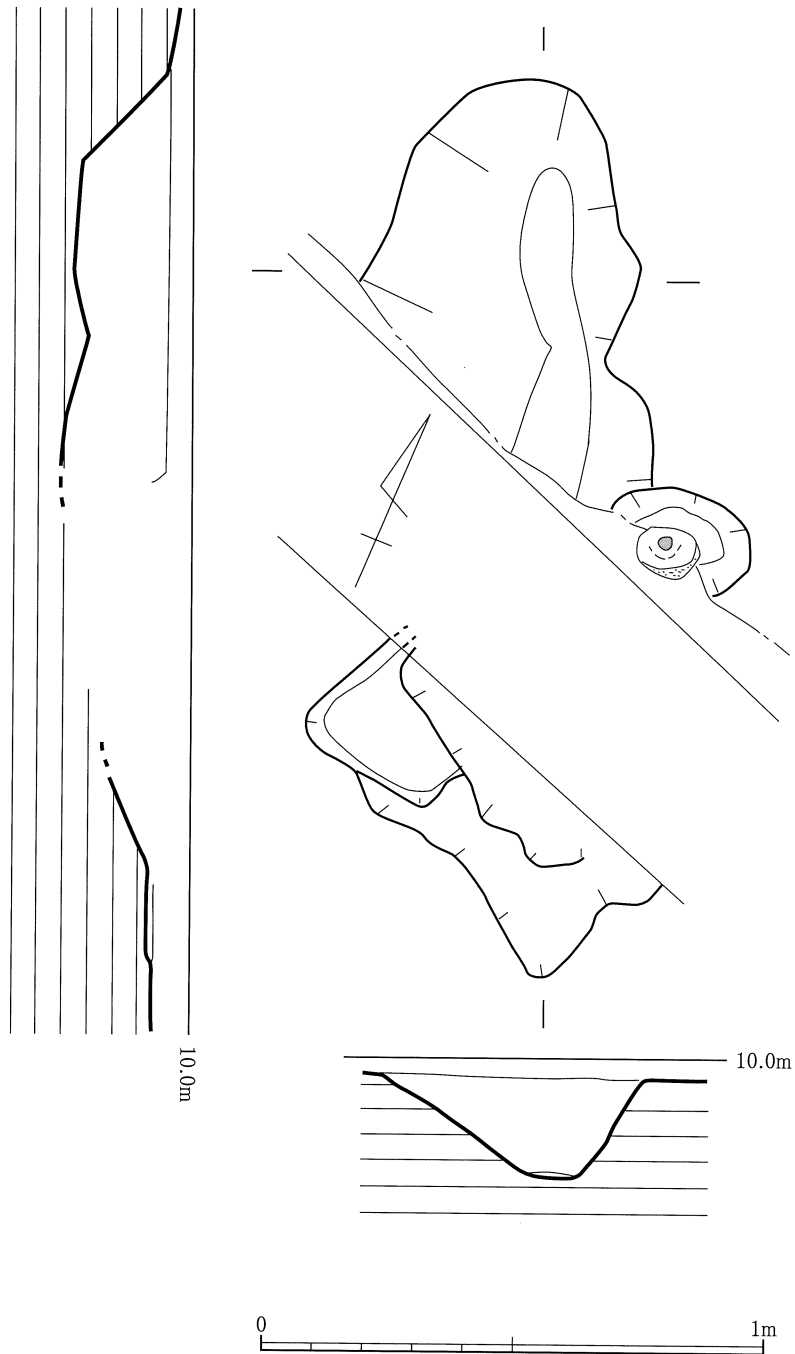
第27図 SK11実測図
