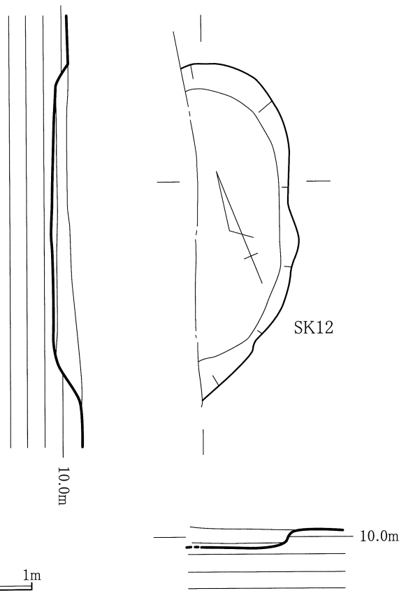
第26図 SK10・12実測図
