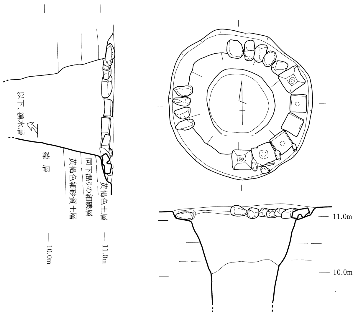
第40図 SE3実測図
