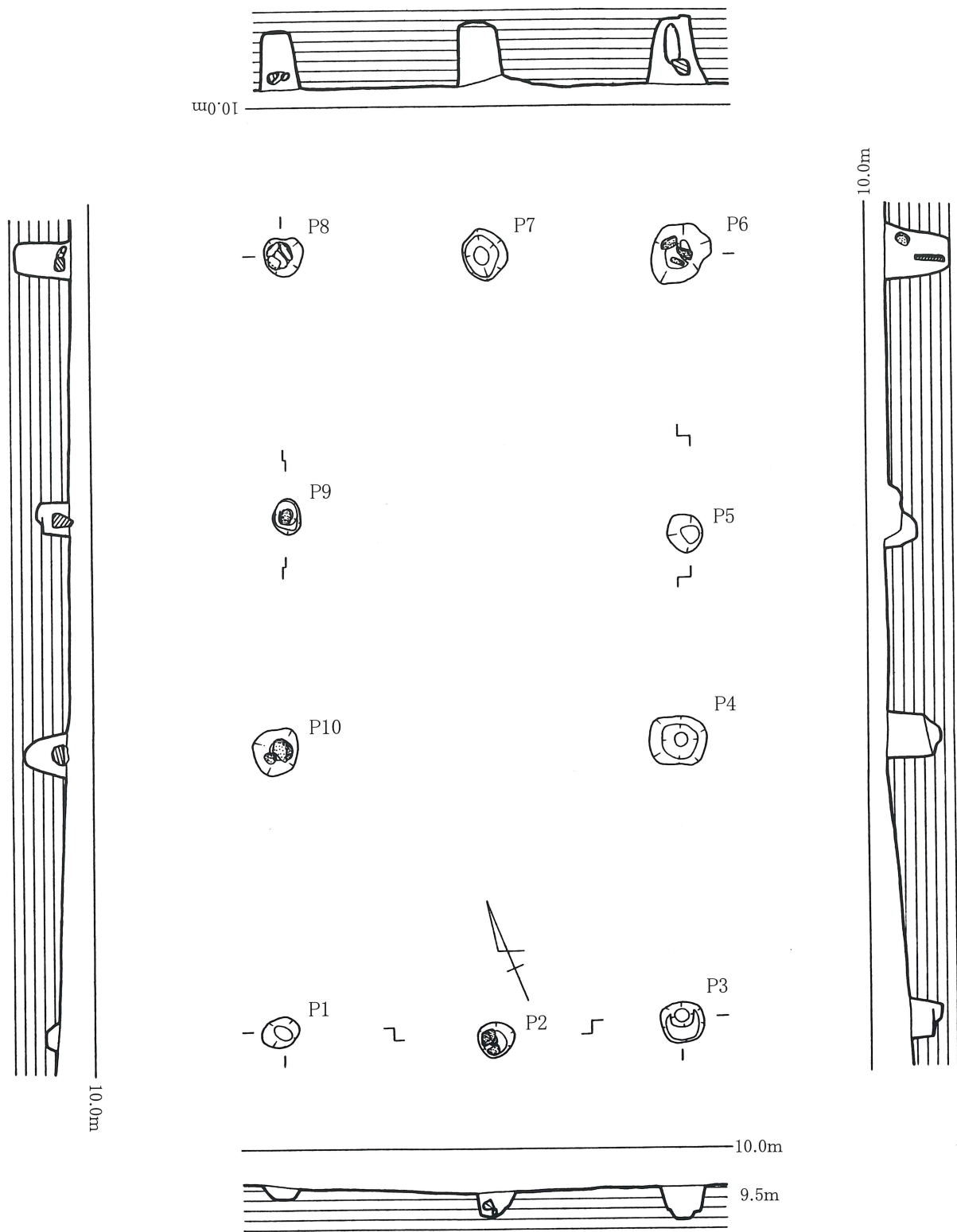
第11図 SB 6 実測図
