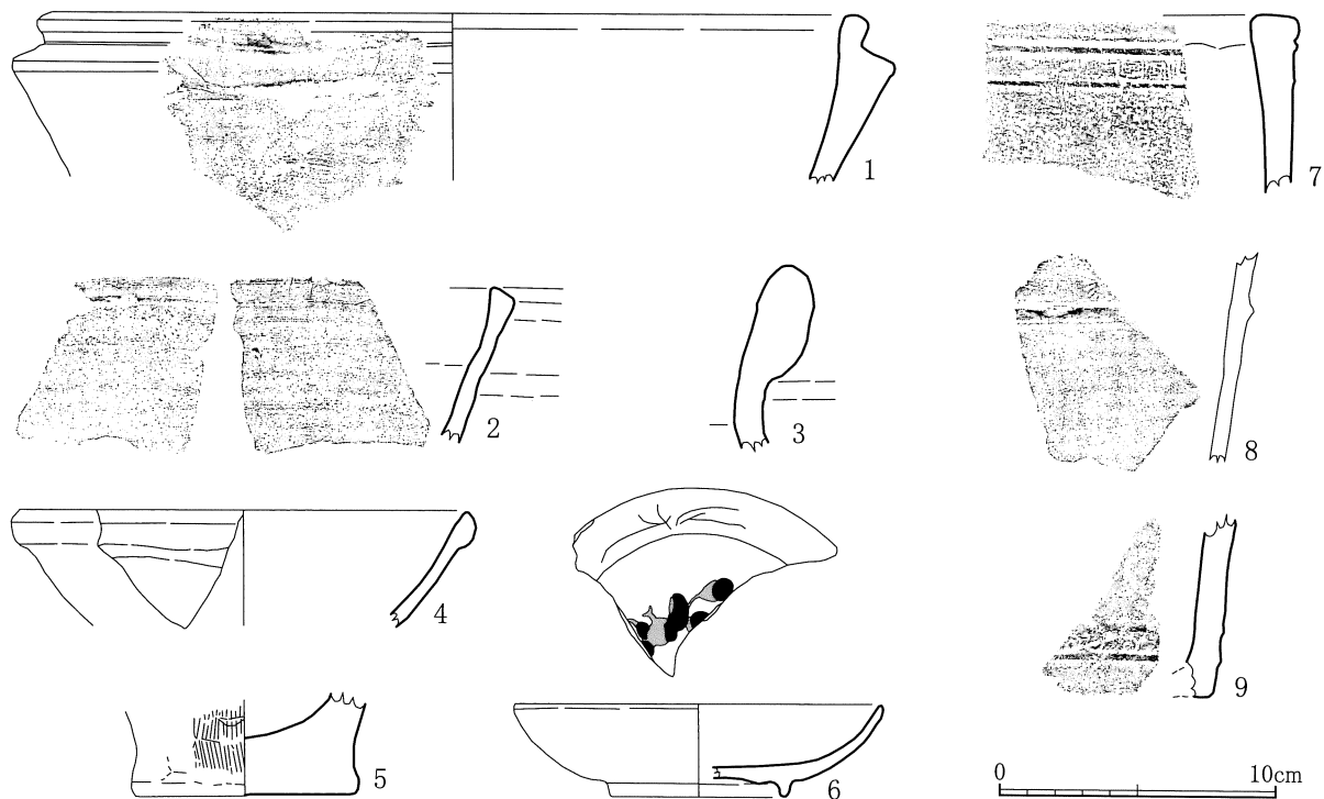
第32図 SD 3 出土遺物実測図
