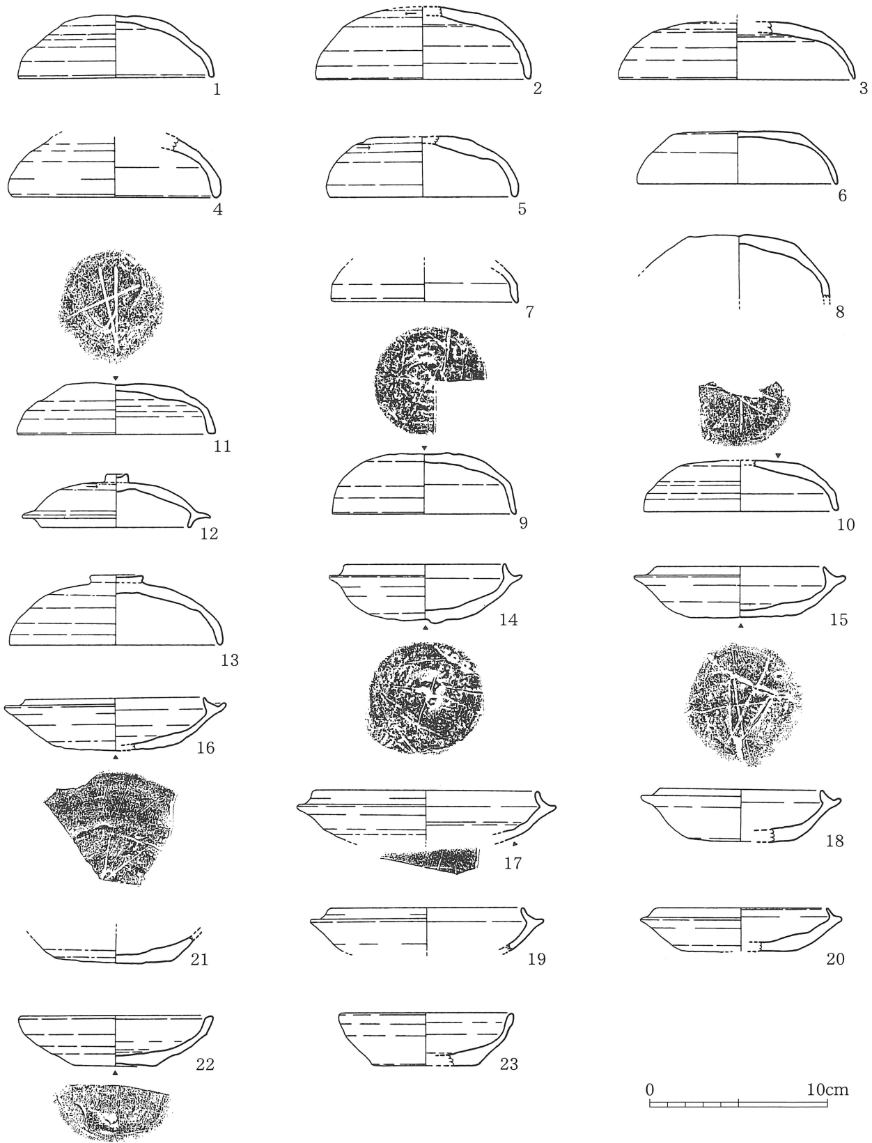
第17図 1-3号墓出土遺物実測図1 (1/3)
