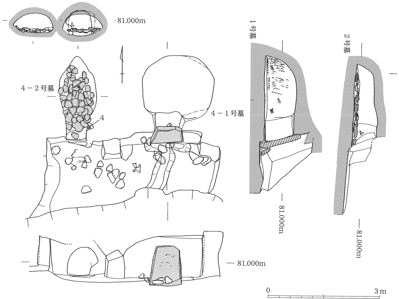
第30図 北友田横穴墓群 4-1・2号墓実測図 (1/60)
