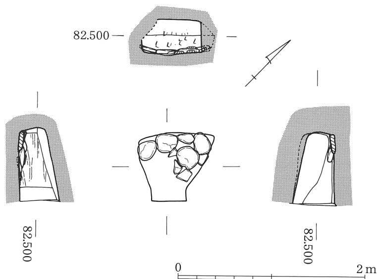
第9図 北友田横穴墓群5号墓実測図（1/40）
