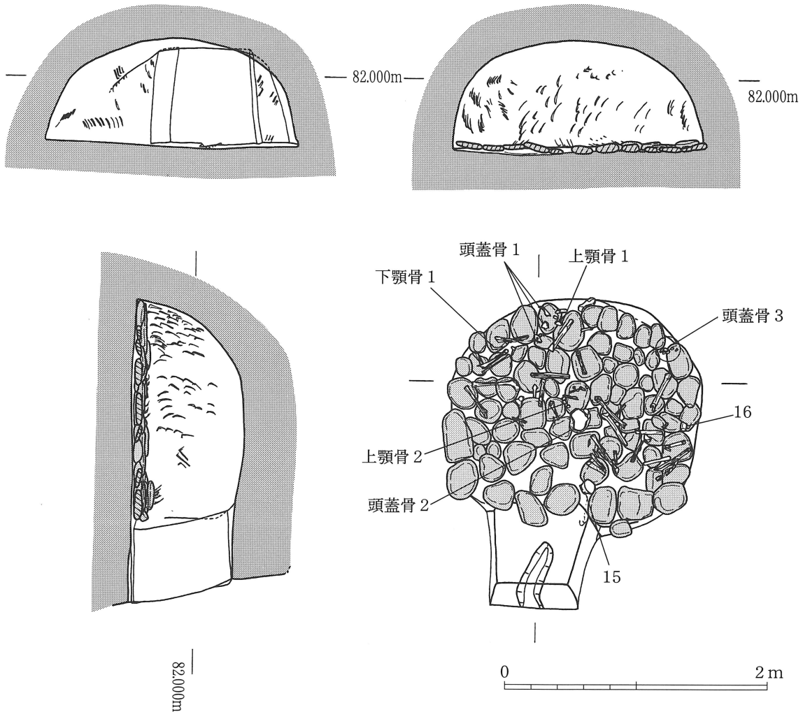
第32図 北友田横穴墓群 4-1号墓実測図（1/40）
