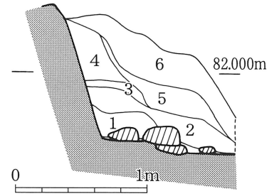
第31図 4-1号墓 前庭部土層図（1/40）
