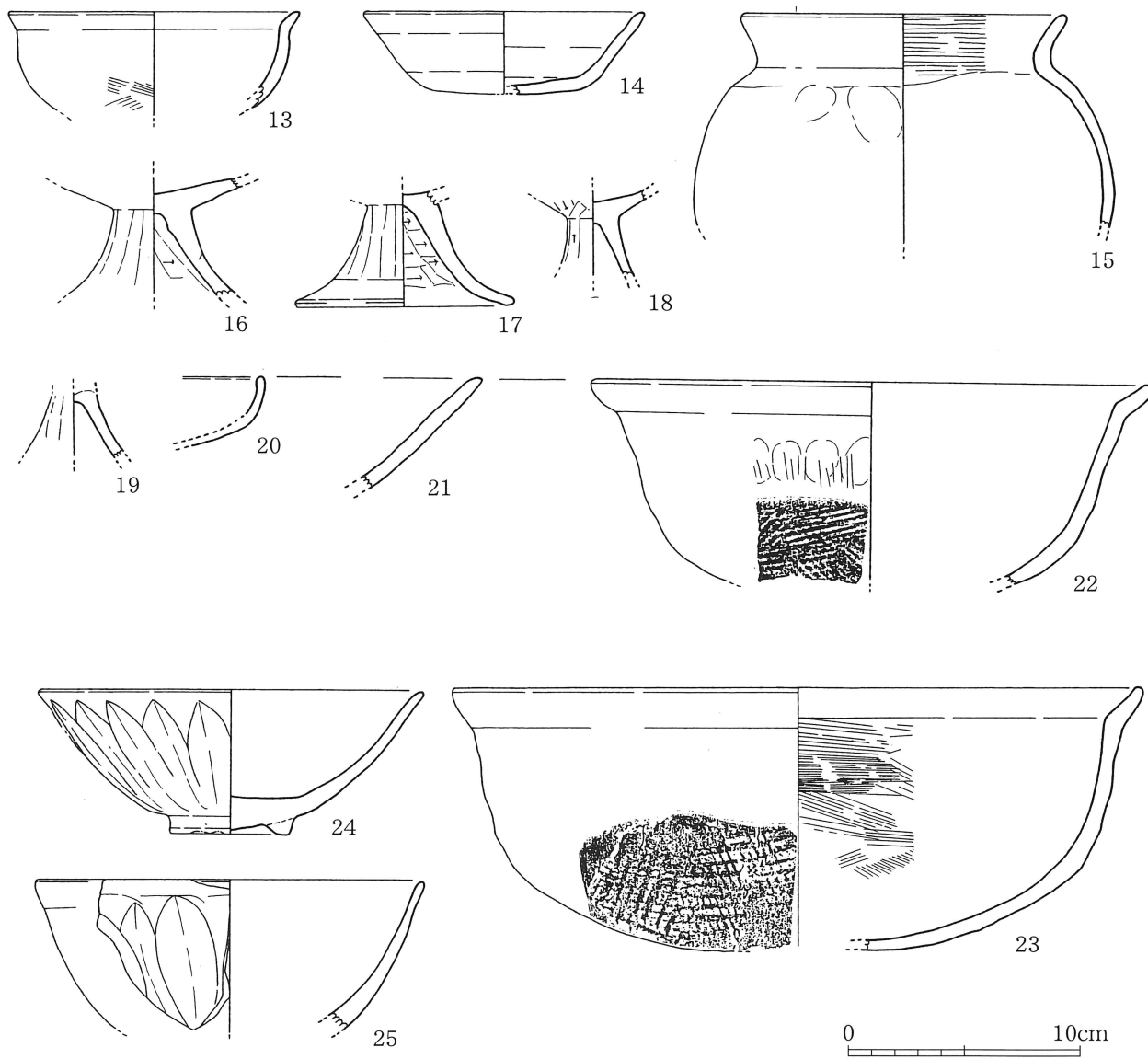
第38図 4-4号墓出土遺物実測図2 (1/3)
