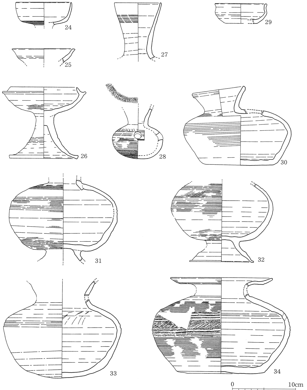
第18図 1 - 3号墓出土遺物実測図2 (1 / 3)
