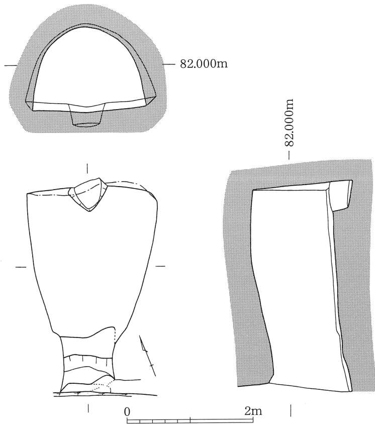
第7図 北友田横穴墓群3号墓実測図(1/60)
