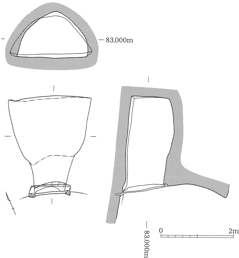
第6図 北友田横穴墓群2号墓実測図(1/60)
