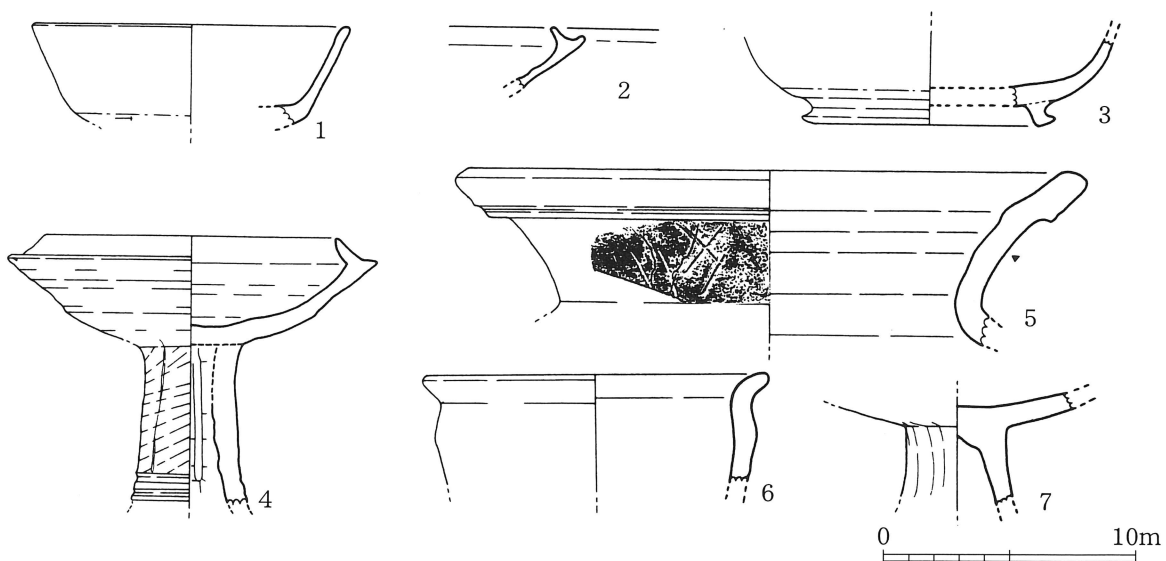
第34図 4-2号墓出土遺物実測図（1/3）
