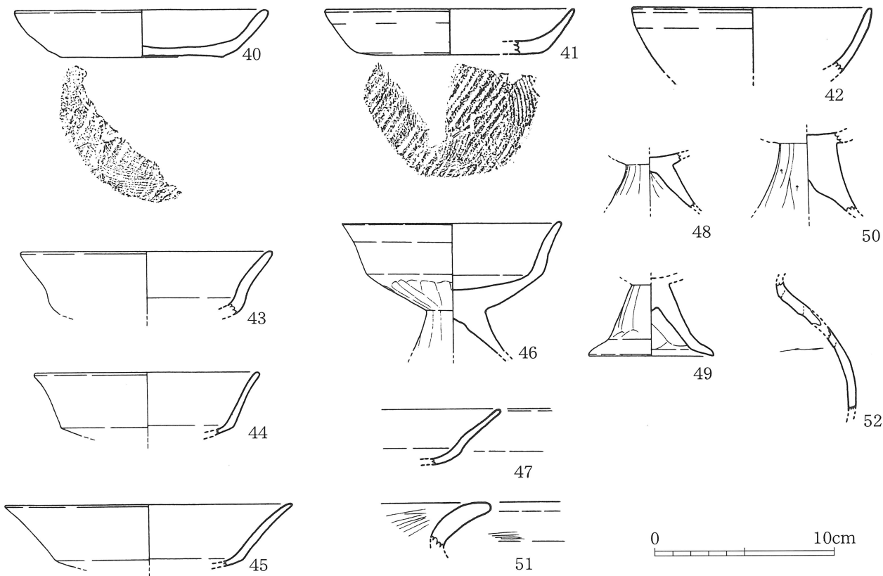
第21図 1-3号墓出土遺物実測図5 (1/3)
