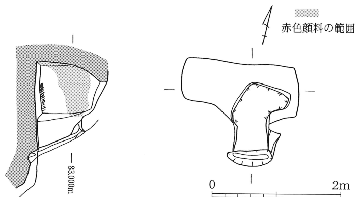
第27図 北友田横穴墓群3-1号墓実測図(1/60)
