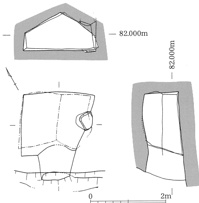
第8図 北友田横穴墓群4号墓実測図(1/60)
