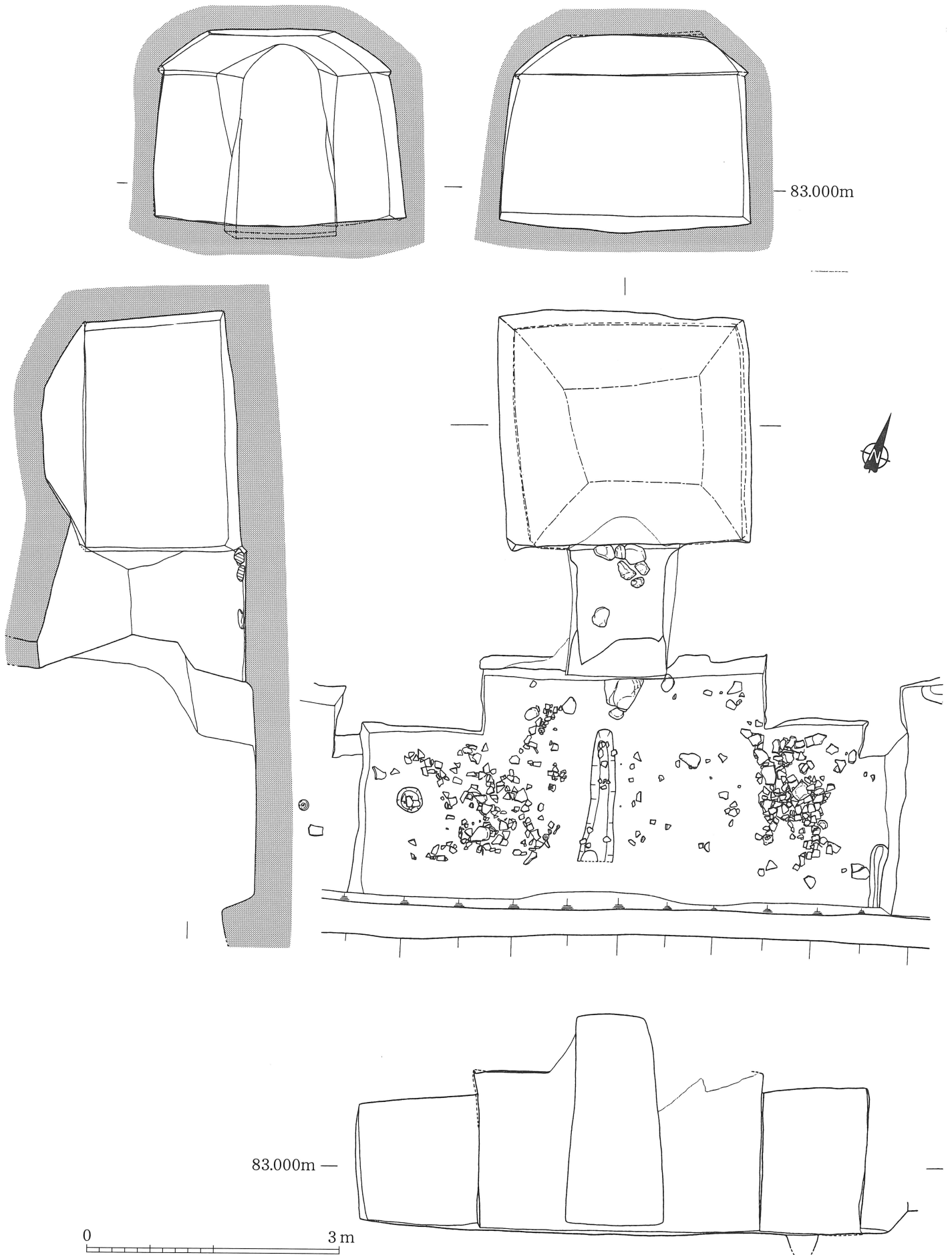
第16图 北友田横穴墓群1-3号墓实测图 (1/60)
