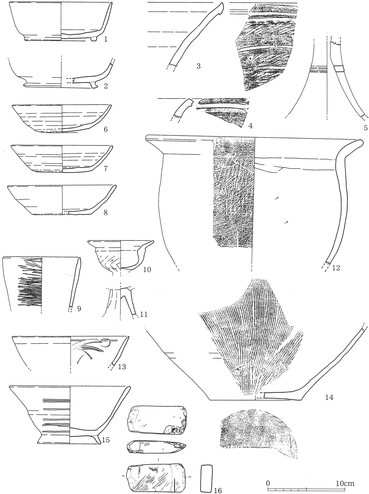
第33図 4-1号墓出土遺物実測図（1/3）
