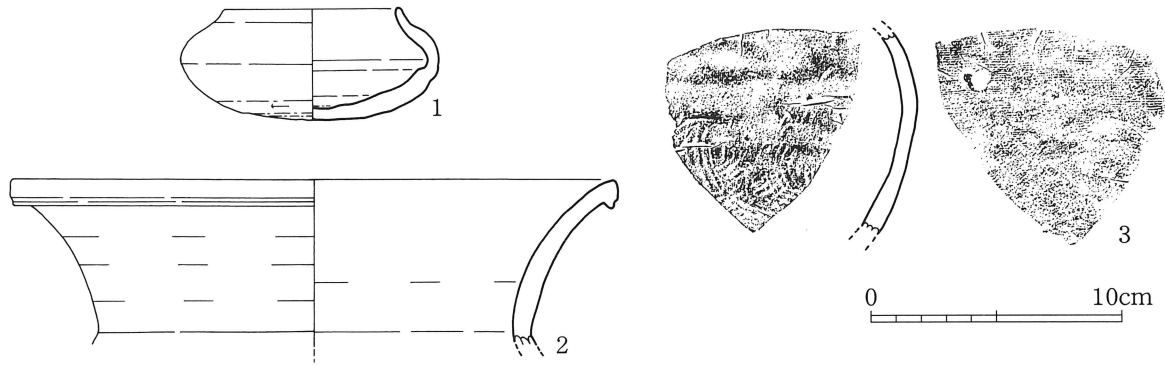
第28図 3-1号墓出土遺物実測図(1/3)
