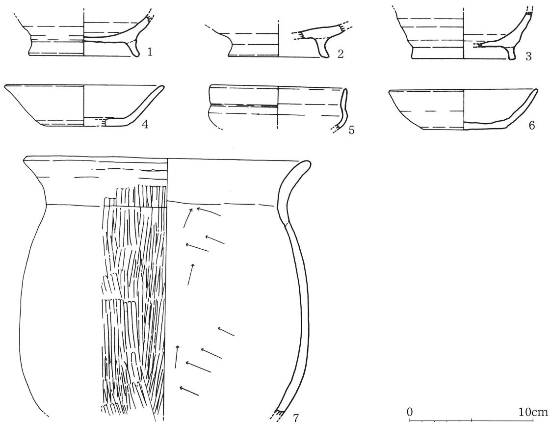
第36図 4-3号墓出土遺物実測図（1/3）
