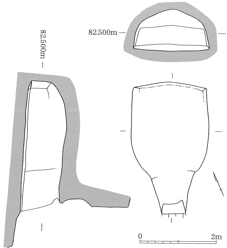
第5図 北友田横穴墓群1号墓実測図(1/60)
