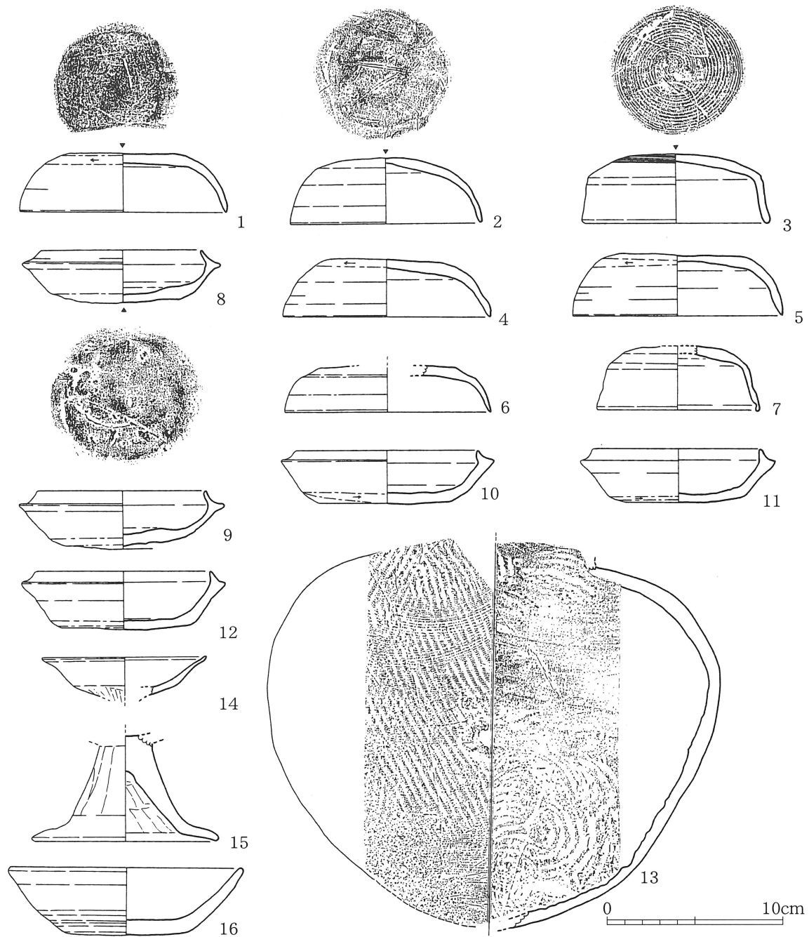
第13図 1-1号墓出土遺物実測図(1/3)
