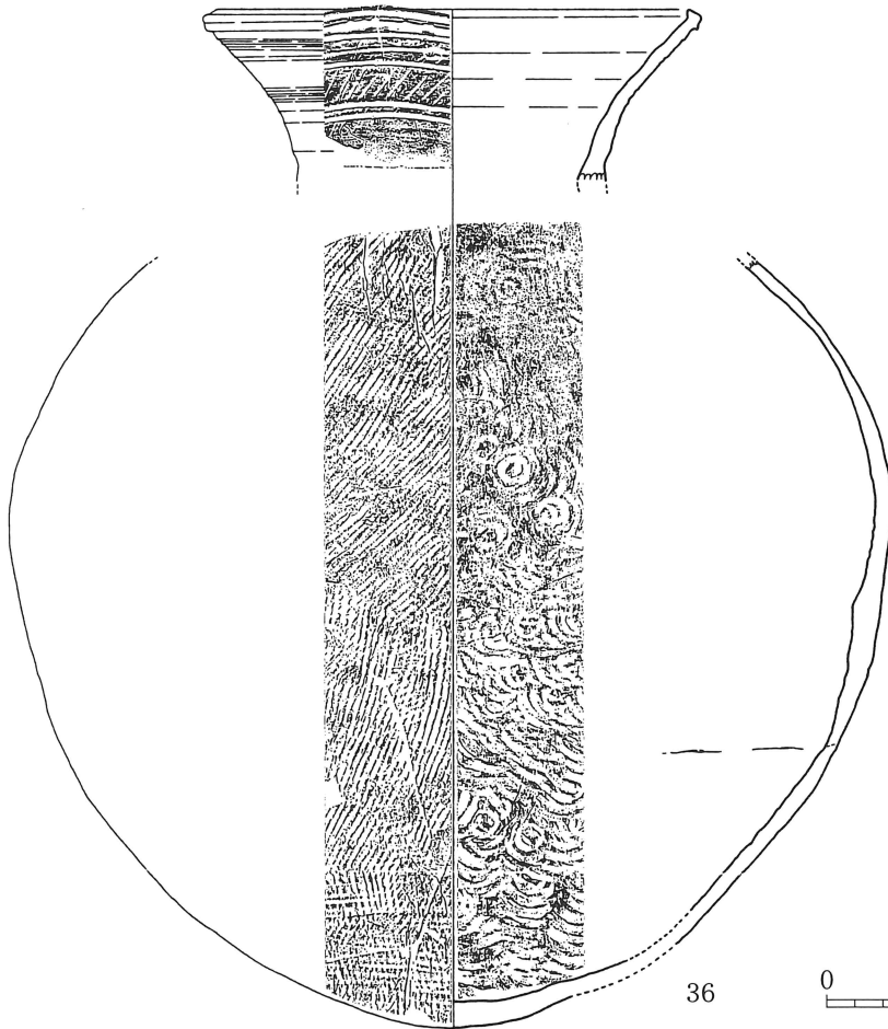
第19图 1-3号墓出土遗物实测图3 (1/6)
