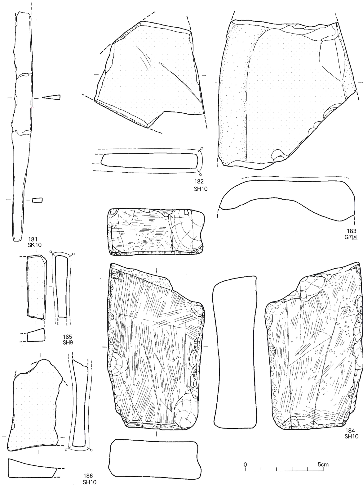
第31図 鉄器・砥石実測図
