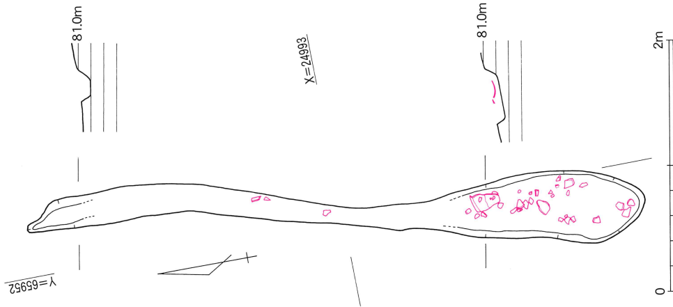
第25図 SD 1実測図
