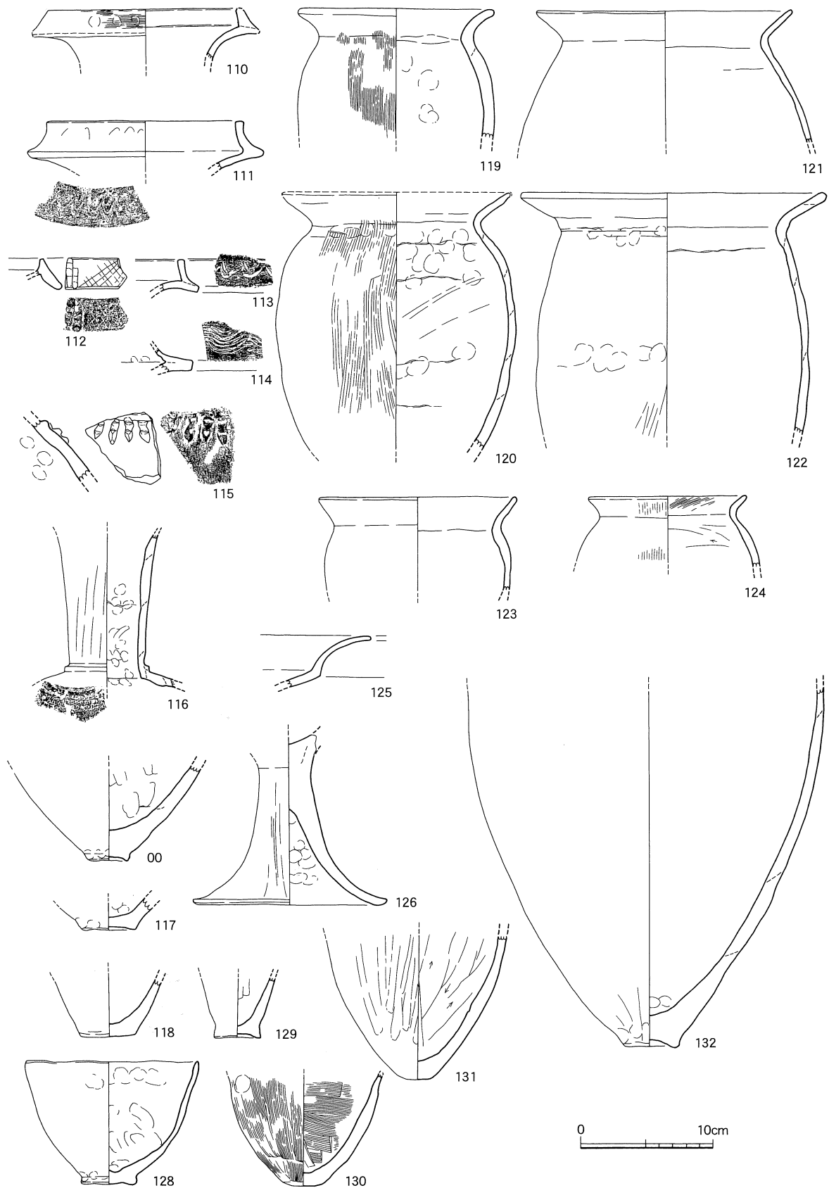
第17图 SH10出土土器实测图
