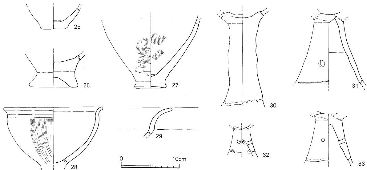
第6図 SH1出土土器実測図(2)
