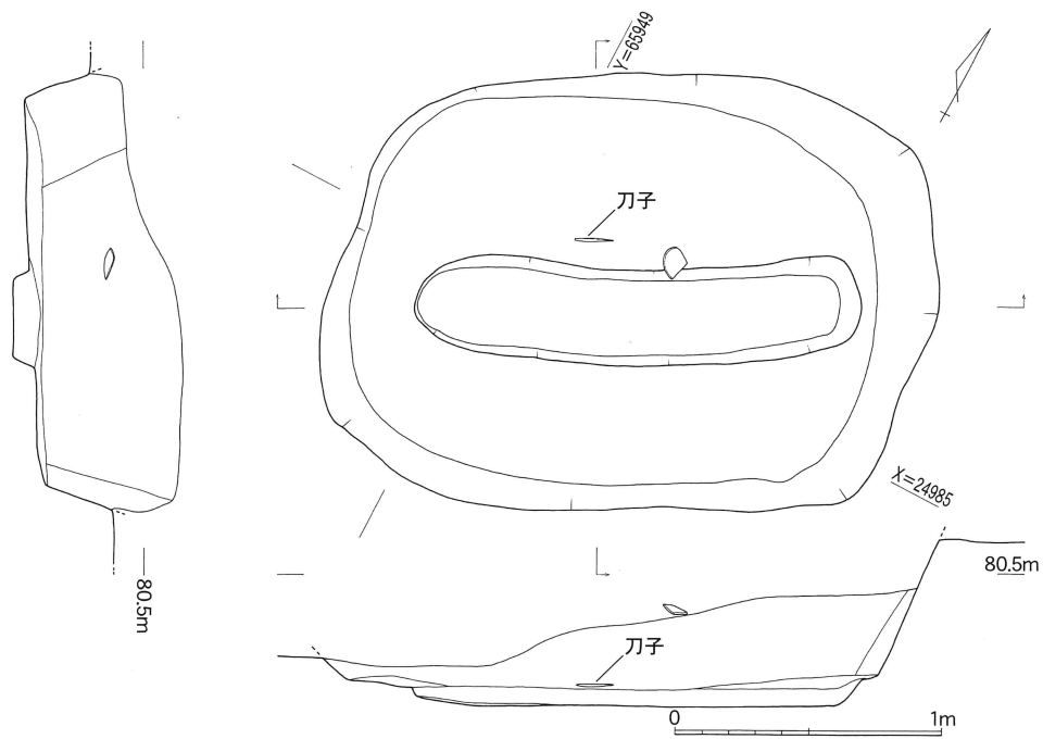
第30图 SK 1 实测图
