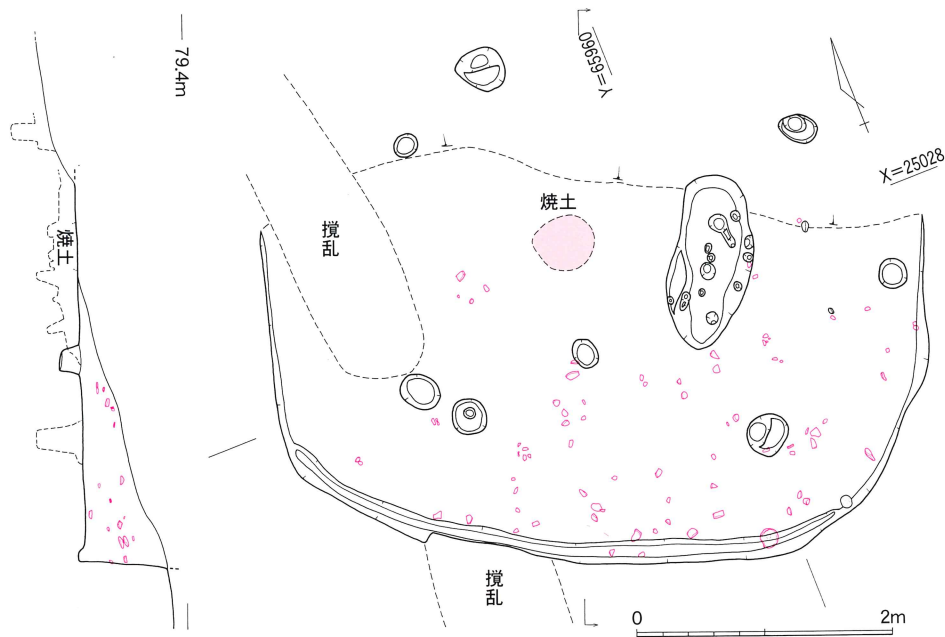
第18図 SH11実測図
