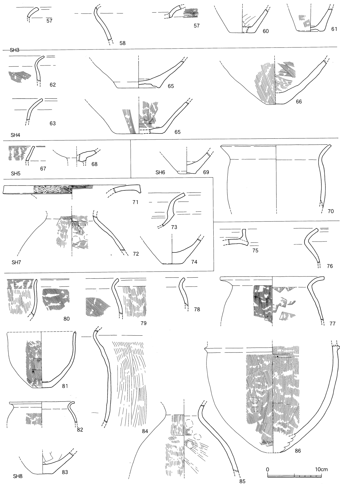
第12图 SH3·SH4·SH5·SH6·SH7·SH8 出土土器实测图
