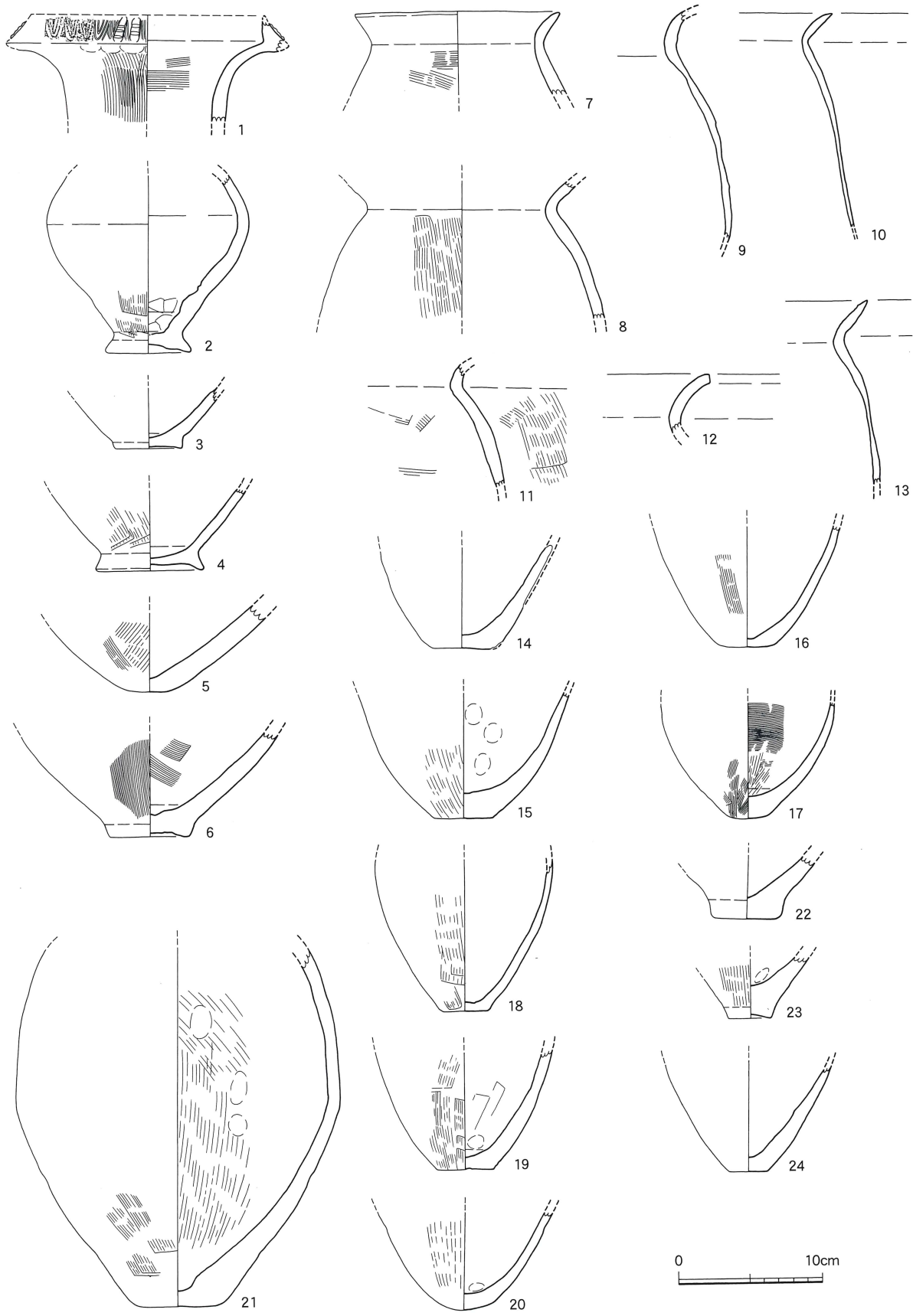
第5图 SH1出土土器实测图(1)
