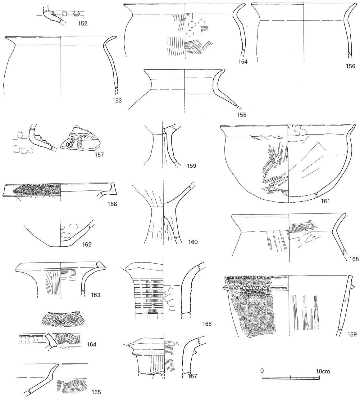
第28図 包含層出土土器実測図
