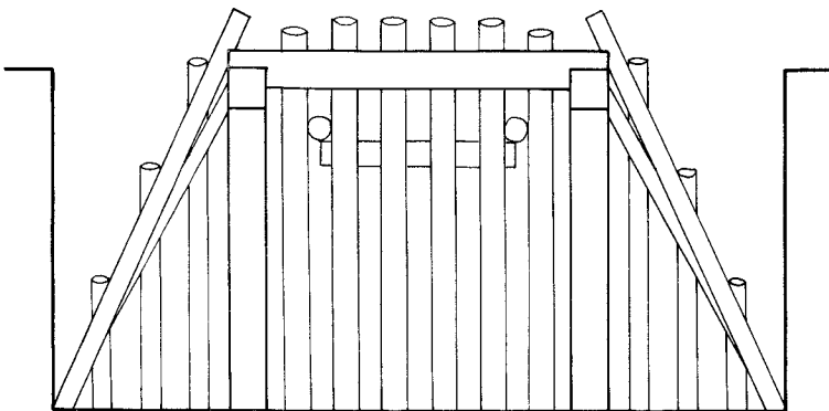
上寺山古墳墓室木組復原図
