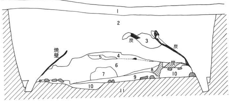
上寺山古墳遺構実測図
