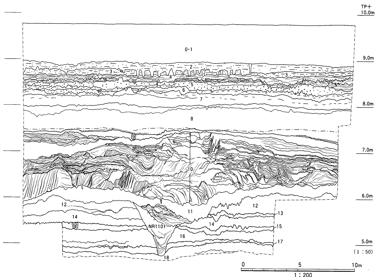
図6 NG05-2次調査南壁地層断面実測図
