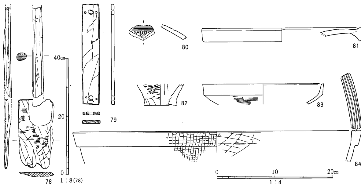
図17 SD2102および第19・21層出土遺物実測図 SD2102(78・79)、第21層(80・81)、第19層(82~84)
