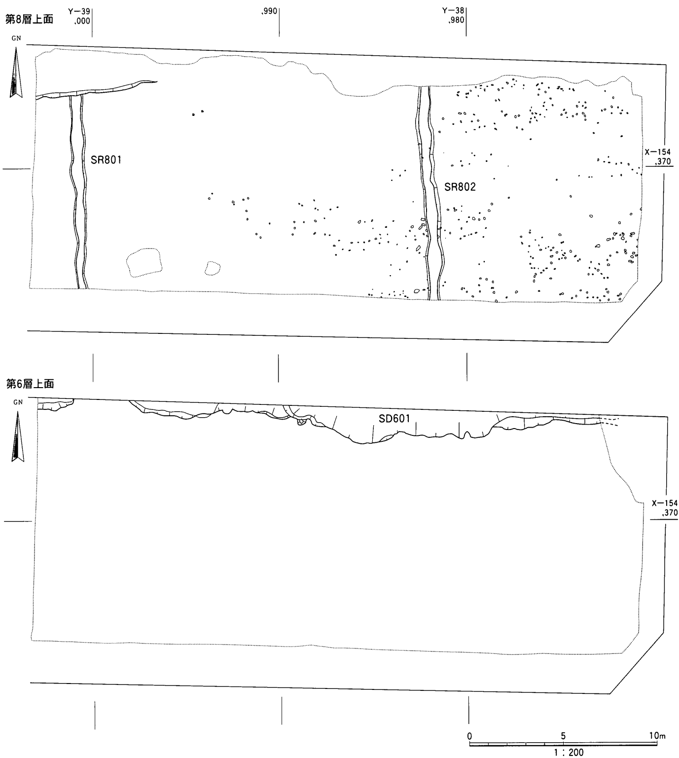
図26 第8層上面および第6層上面遺構平面実測図
