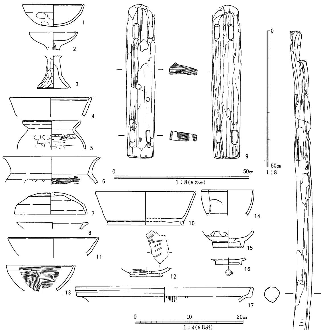
図8 NG05-2次出土遺物実測図
