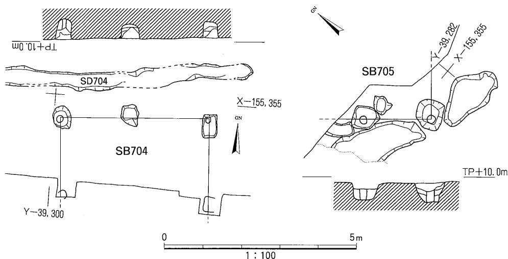
図22 SB704・705実測図
