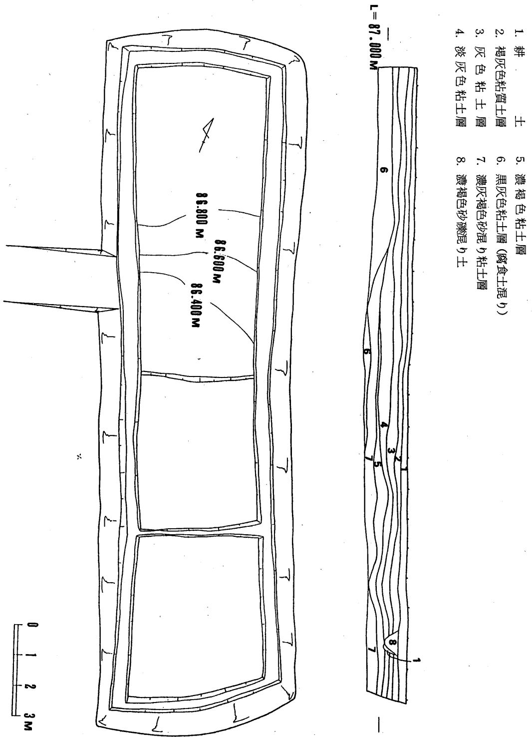
図版 4 2 トレンチ図および東壁断面図
