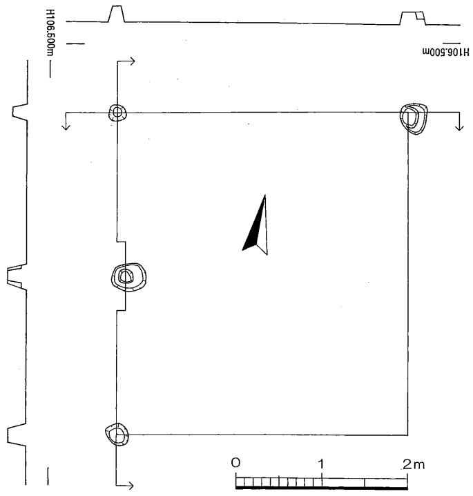
图6 掘立柱建物 (SB01)
