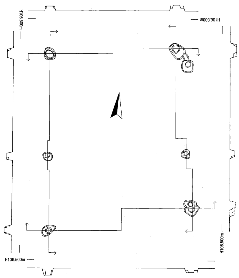
图7 掘立柱建物 (SB02)
