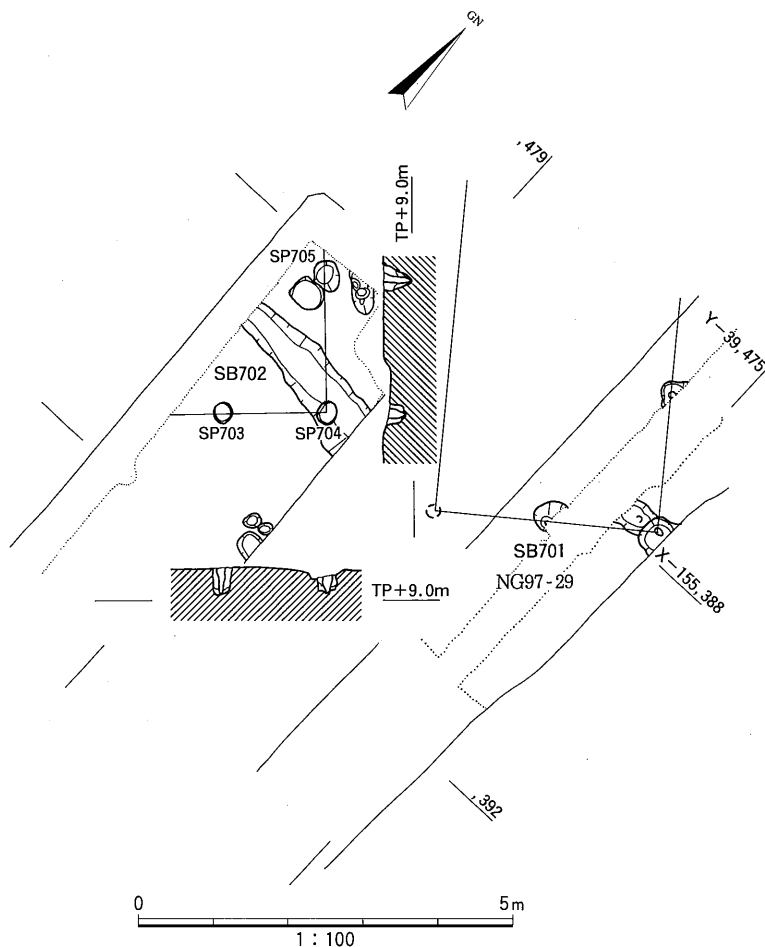
図11 SB702建物配置
