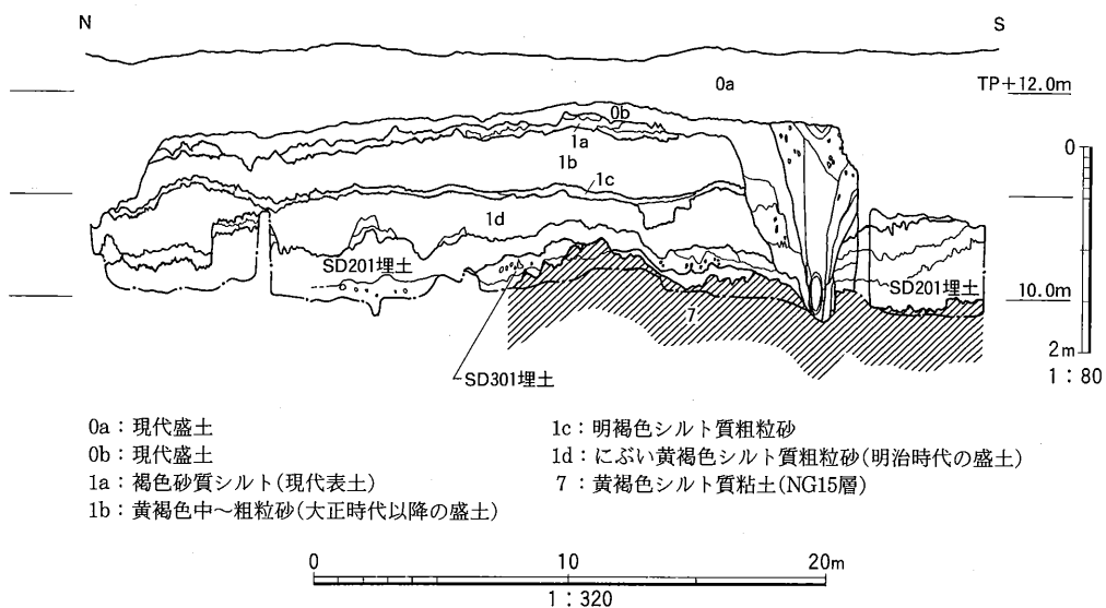
図15 東壁断面図
