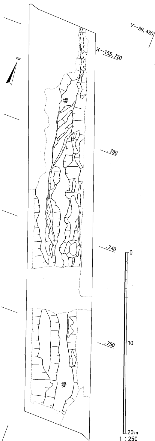
図20 馬池東堤平面図
