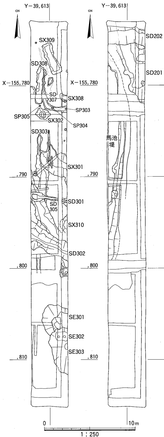
図28 平面図
