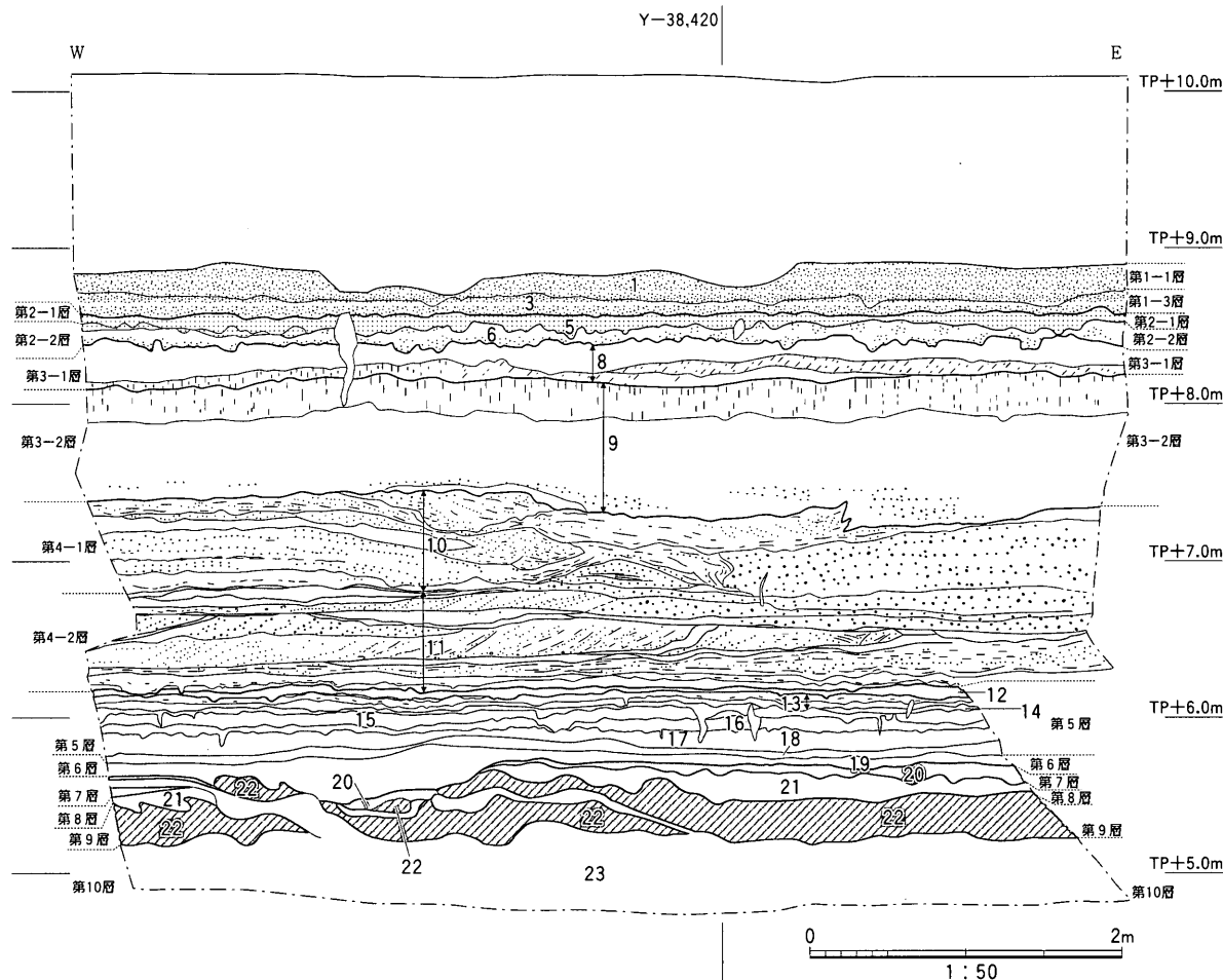
図4 北壁断面図
