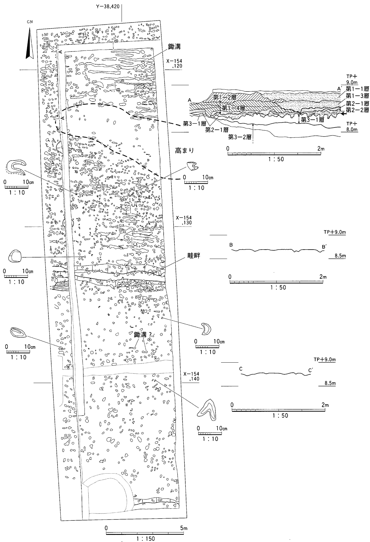
図11 第3-1層上面の遺構平面図・断面図
