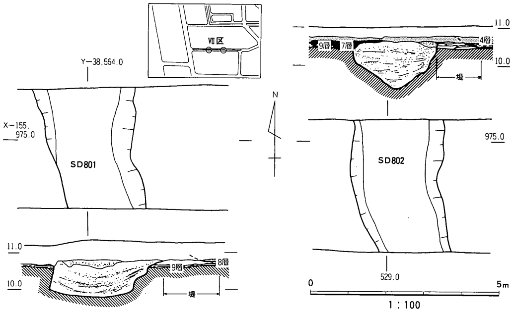
図40 VII区SD801・802実測図
