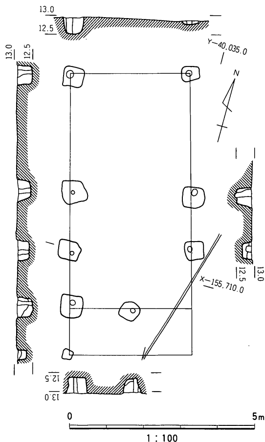
図10 SB01実測図
