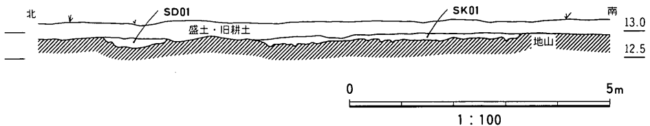
図7 Ⅰ区中央部東壁土層図
