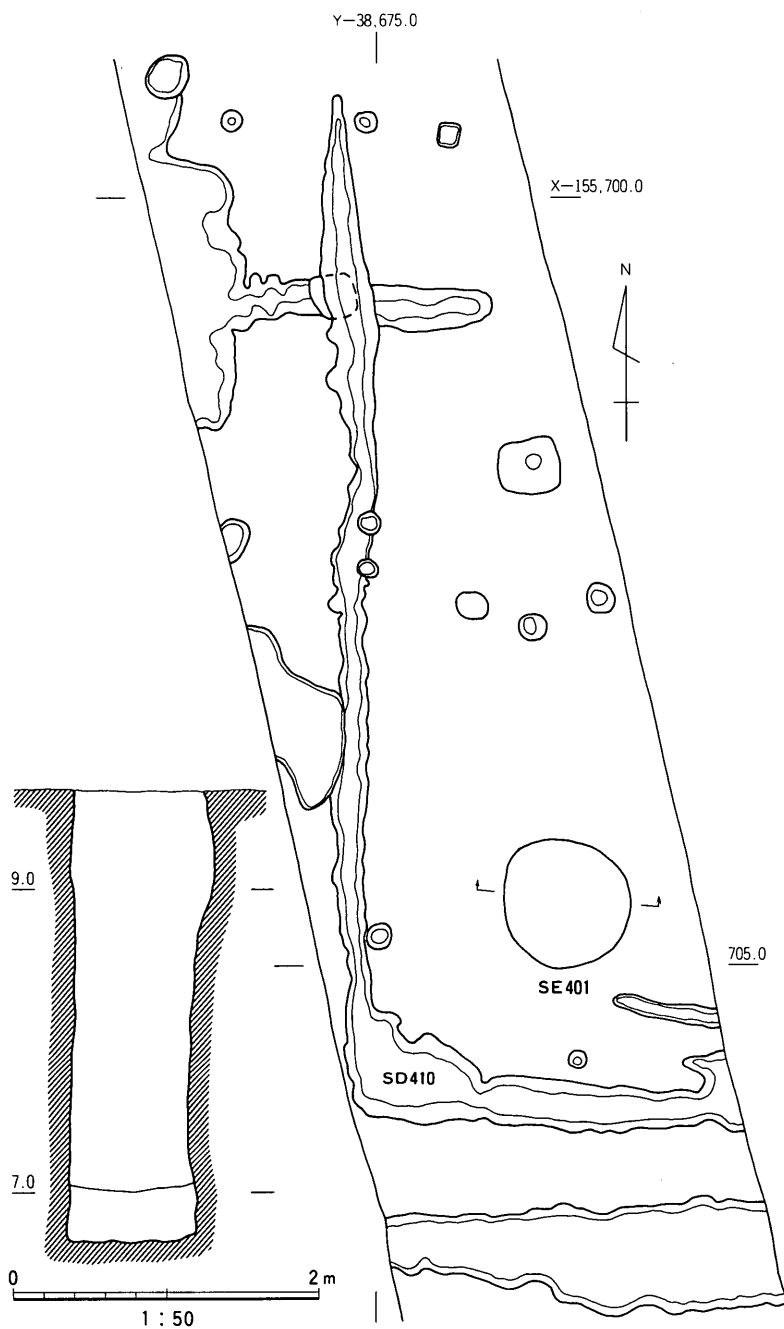
図107 I区SE401・SD410実測図
