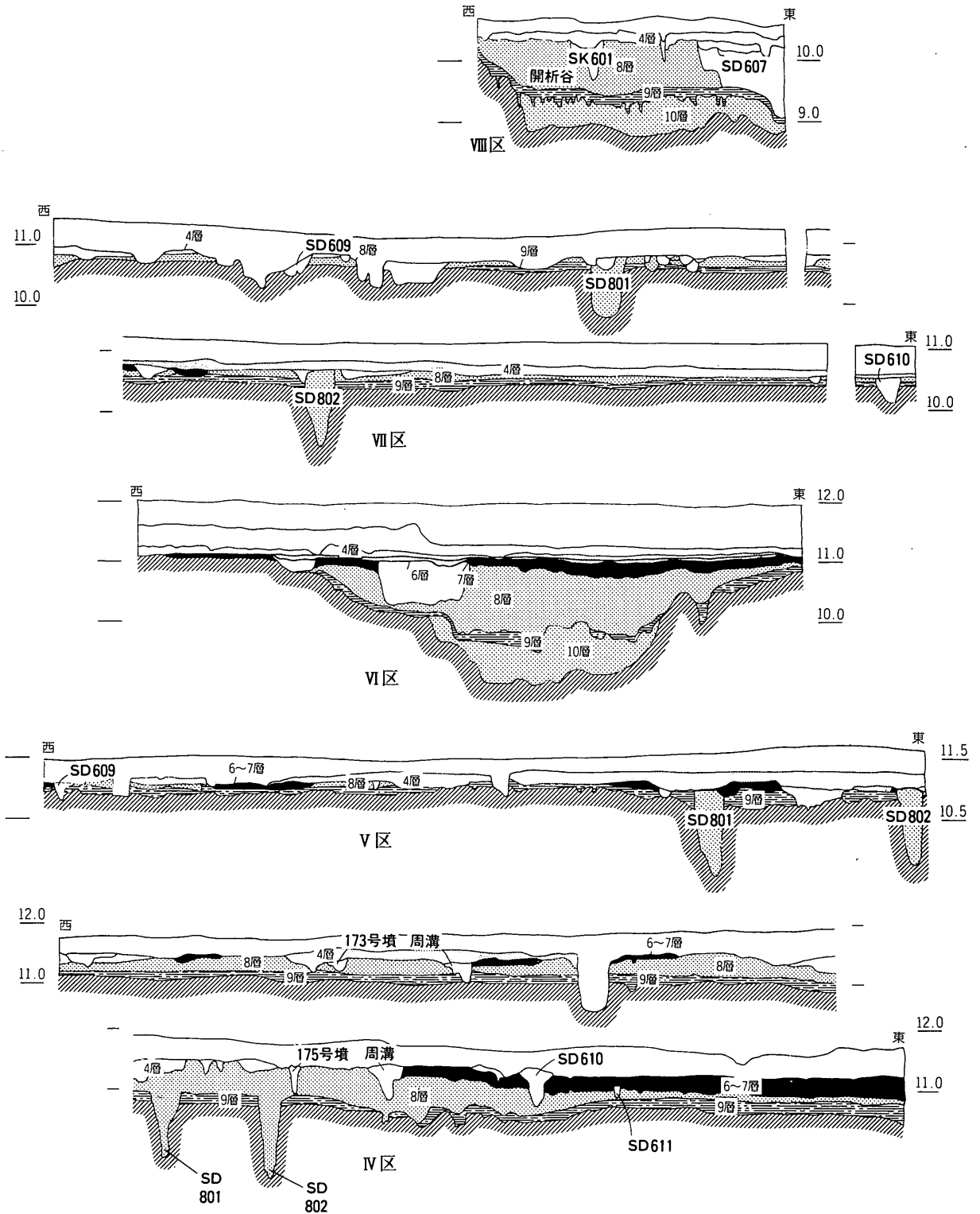
図31 東西方向(Ⅳ・Ⅴ・Ⅵ・Ⅶ・Ⅷ区北壁)土層図
