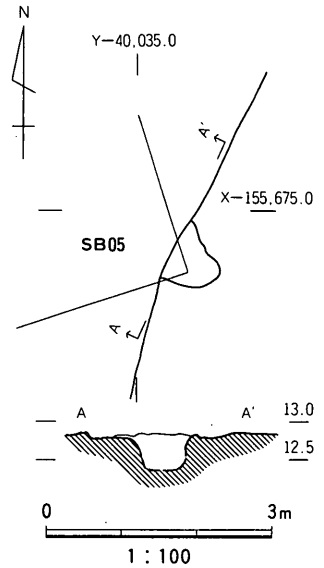
図15 SB05実測図
