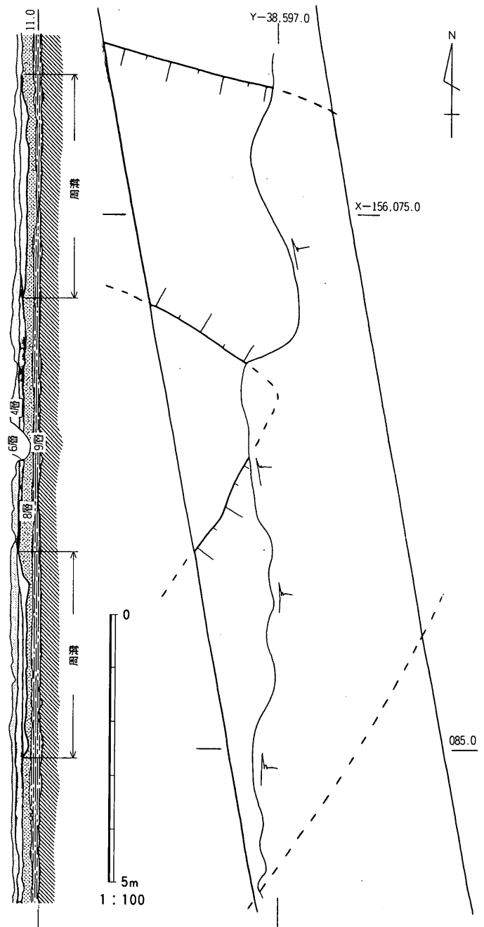
図44 171号墳実測図
