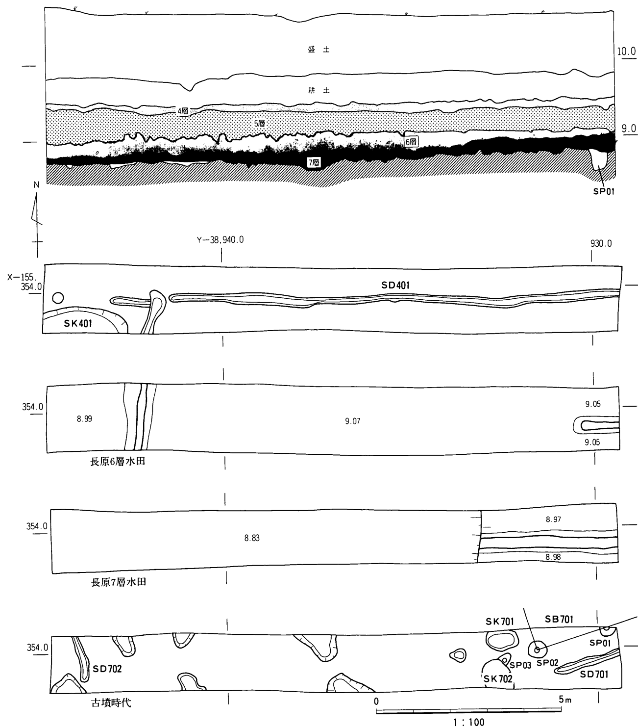
図24 北壁土層図および遺構実測図
