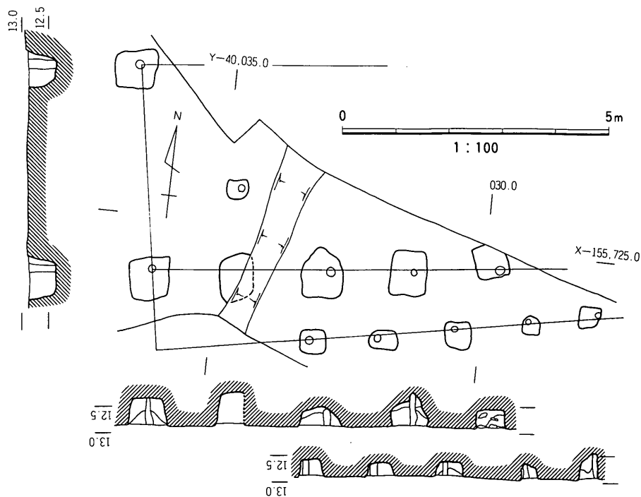
図13 SB03実測図
