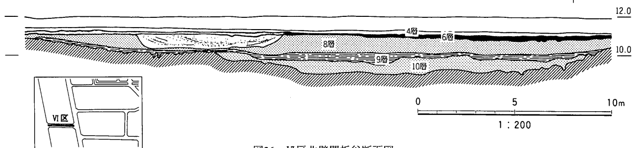
図36 VI区北壁開析谷断面図
