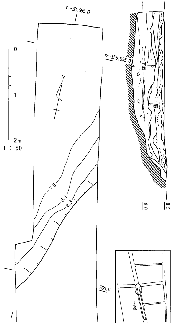
図83 I区 SD701実測図
