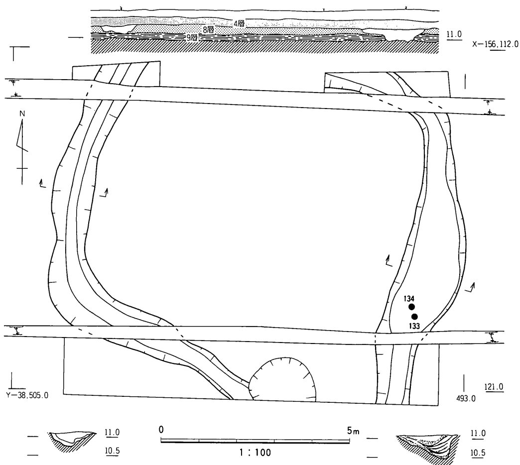
図50 175号墳実測図
