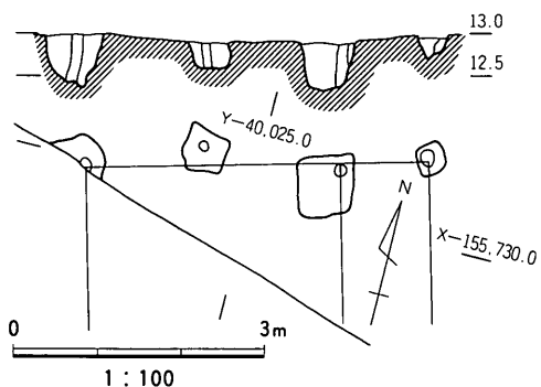
図14 SB04実測図
