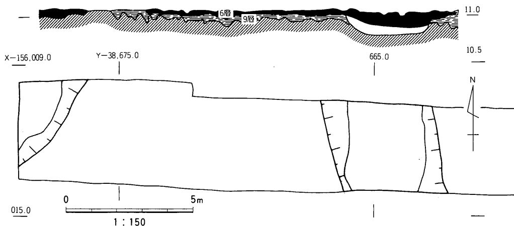
図52 176号墳実測図
