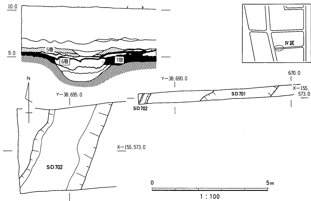
図85 IV区SD702実測図
