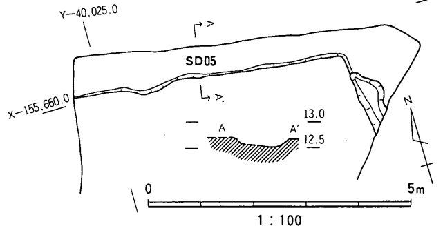
図21 SD05実測図
