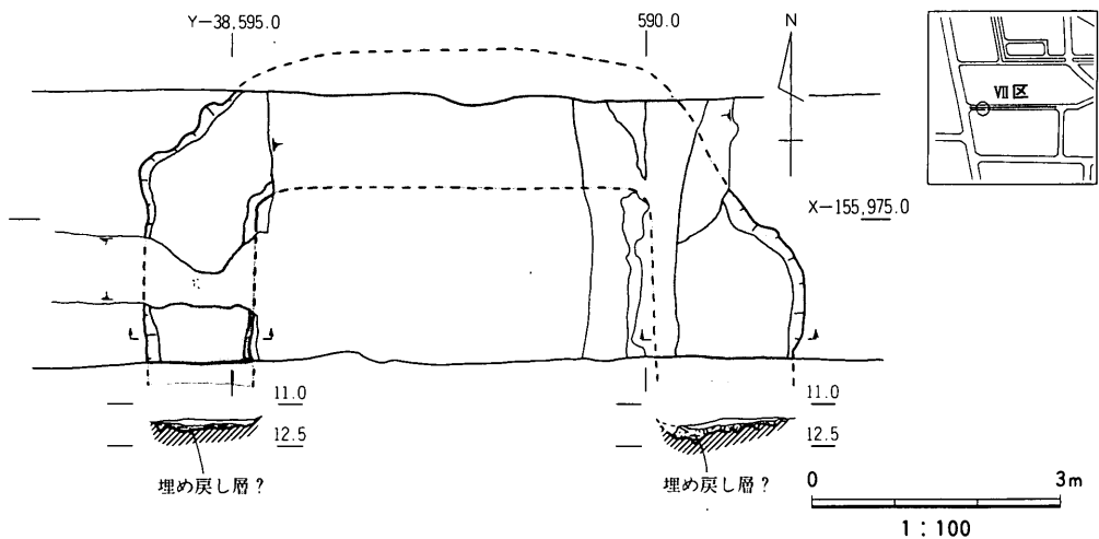
図46 172号墳実測図
