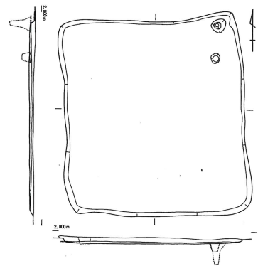
⑦ 竪穴1 (S=1/90)
