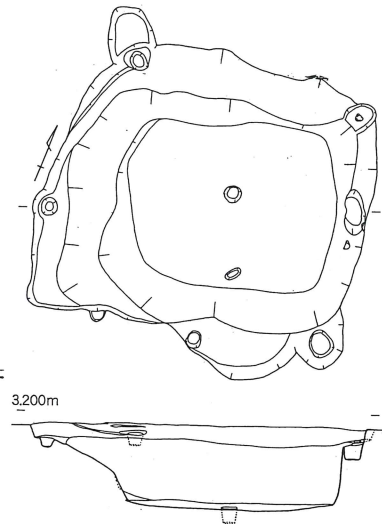
⑥ 竪穴1 (S=1/90)
