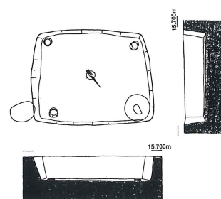
⑰ 1号竪穴 (S=1/90)
