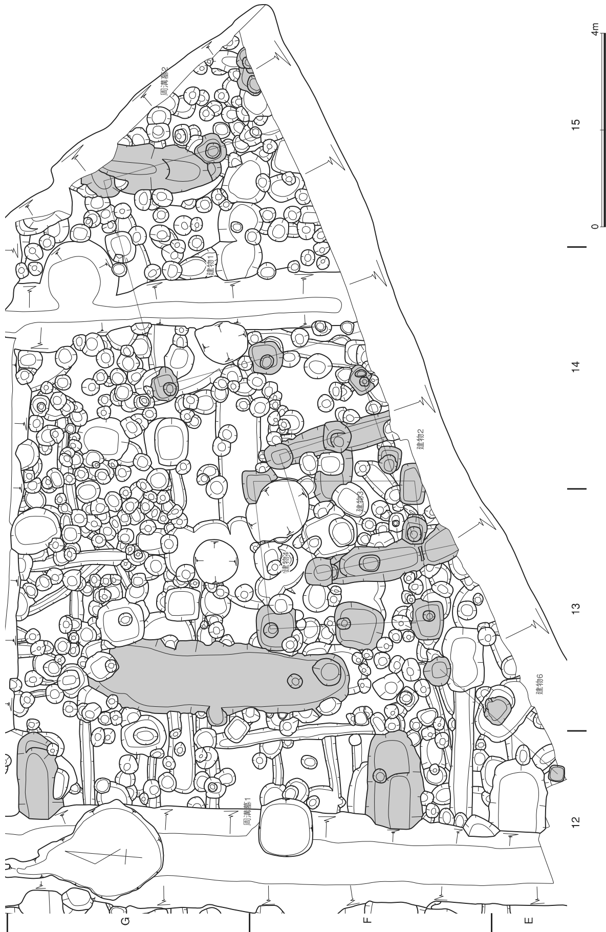
第39图 遺構実測図(8) (縮尺1/80)
