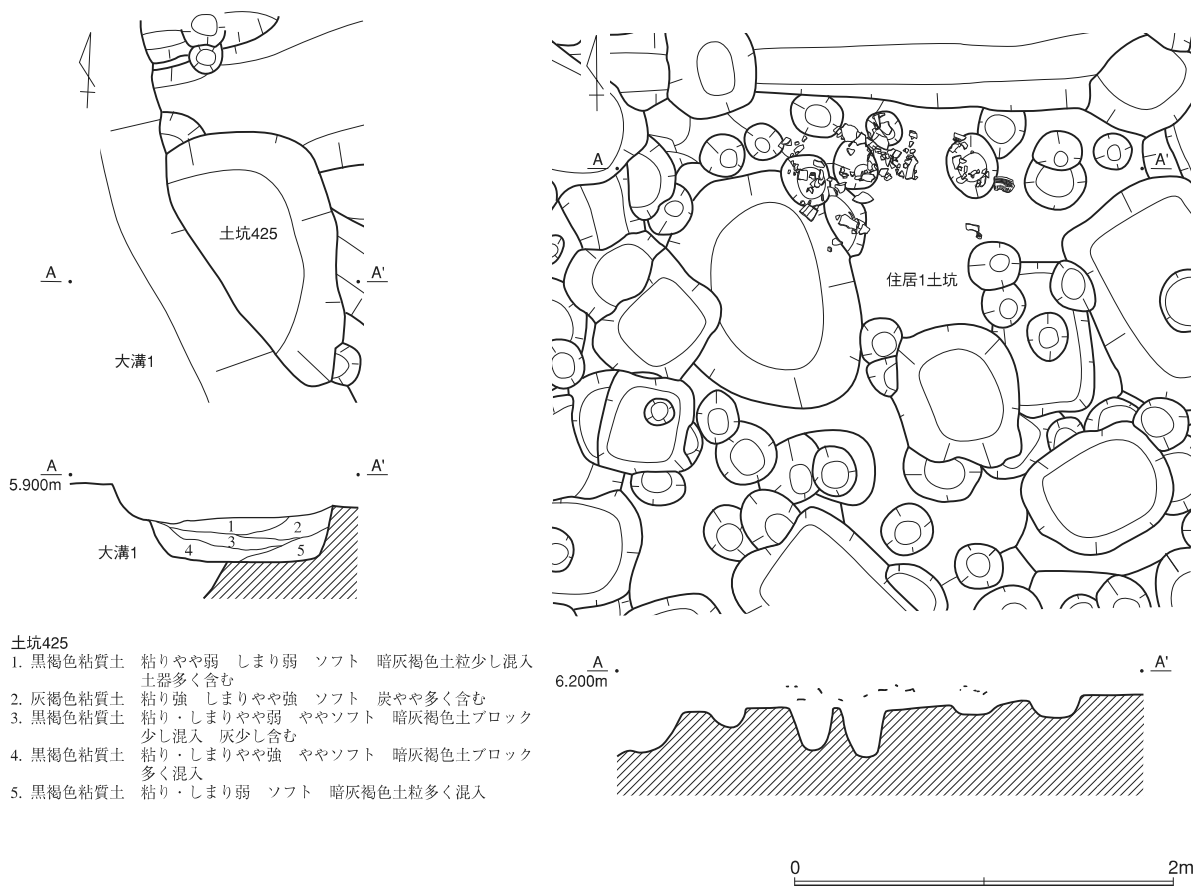
第31図 土坑425・住居1土坑実測図（縮尺1/40）
