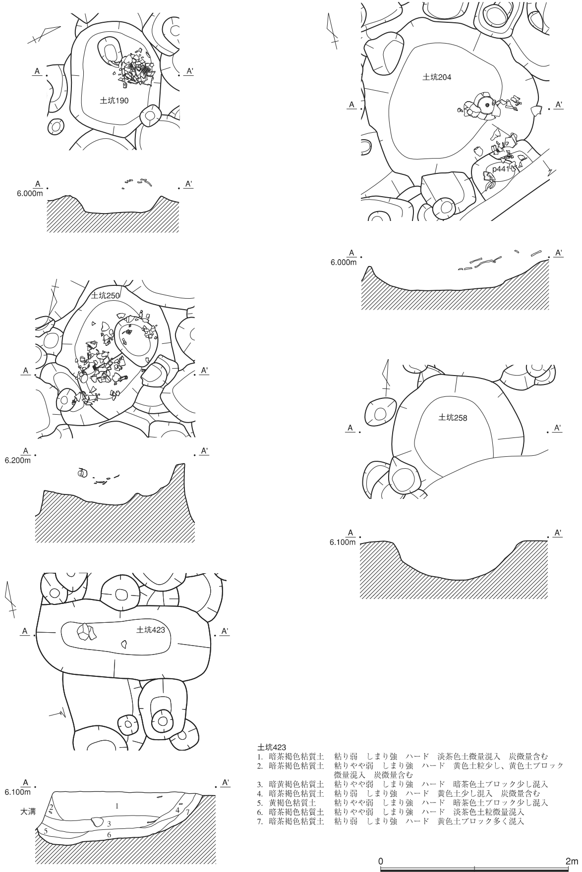
第29図 土坑190・204・250・258・423実測図（縮尺1/40）
