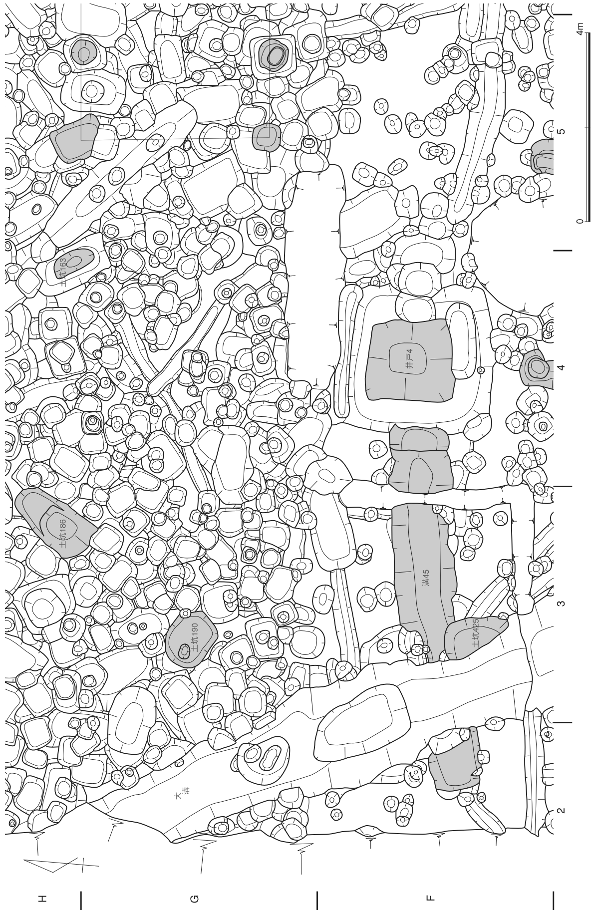
第35図 遺構実測図 (4) (縮尺1/80)
