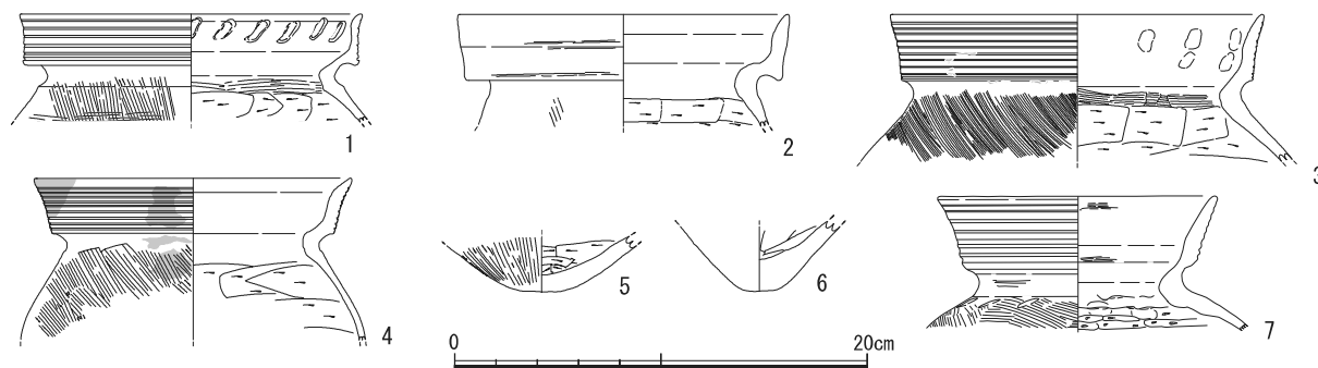
第43図 周溝墓・掘立柱建物出土土器実測図（縮尺1/4）
