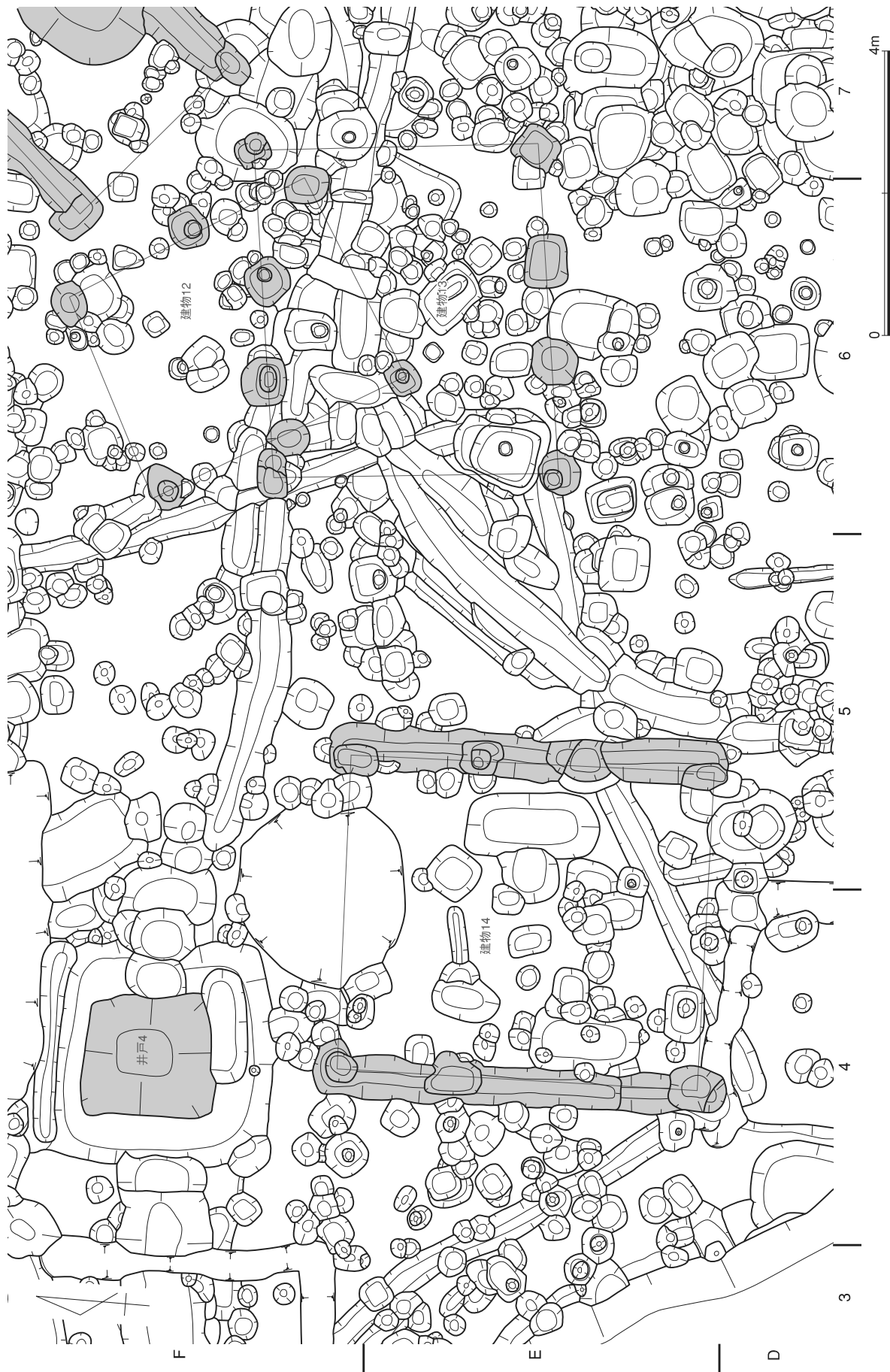
第34図 遺構実測図 (3) (縮尺1/80)
