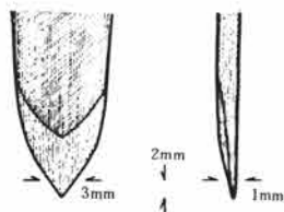
図2 推定刻字工具 (寸法は、土器乾燥～焼成時の収縮を考慮せず推定)
