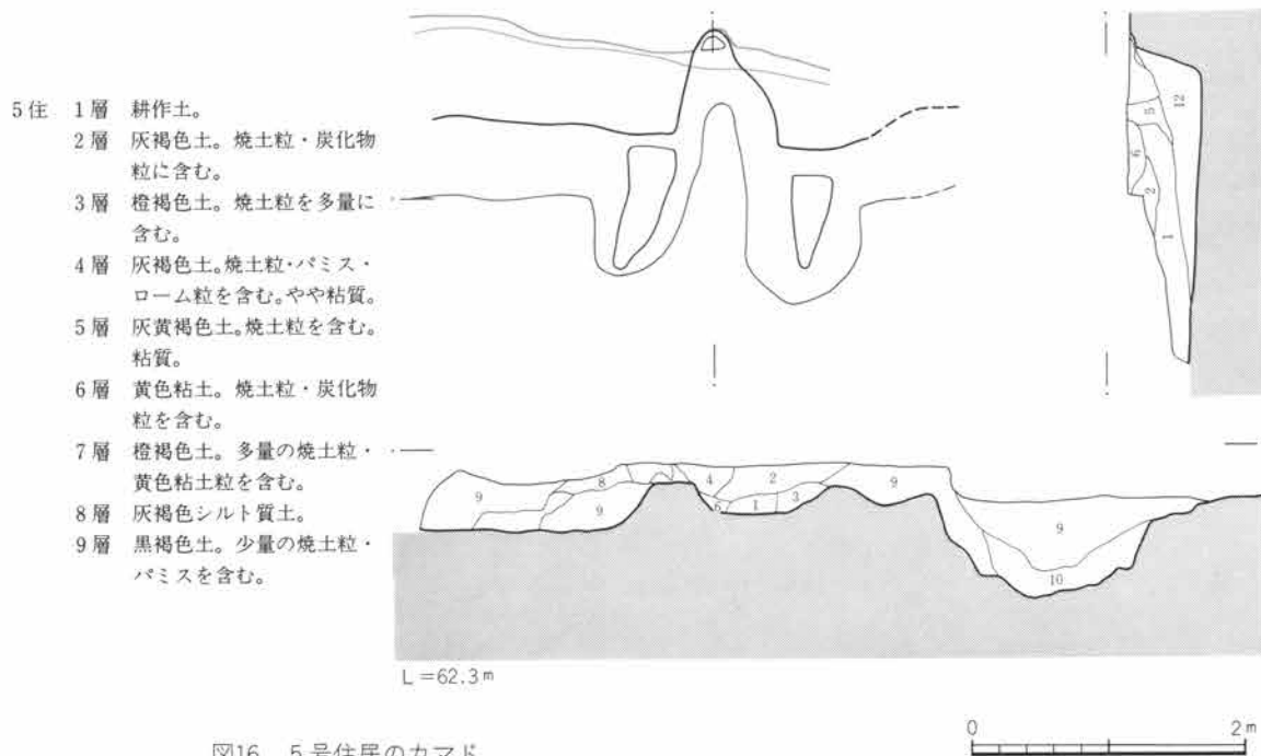
図16 5号住居のカマド
