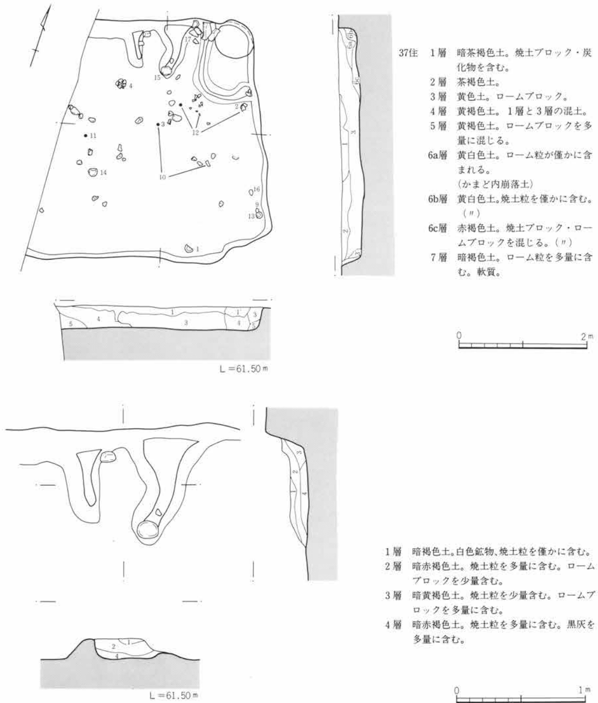
図69 37号住居とカマド
