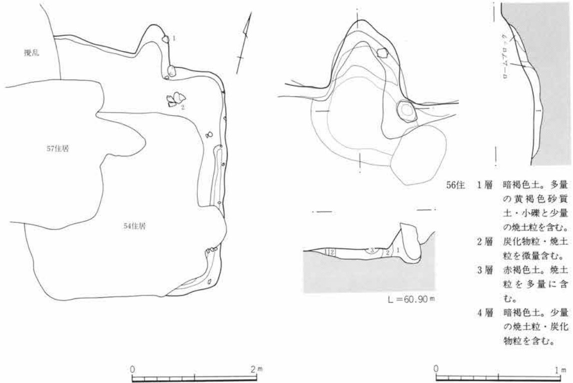
図104 56号住居とカマド
