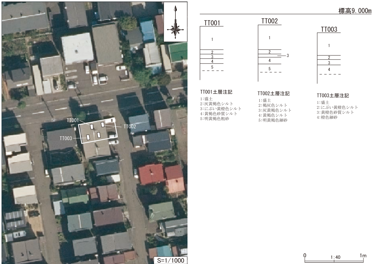
第20図 整理番号 22-2-302 試掘調査実施箇所及び土層断面模式図
