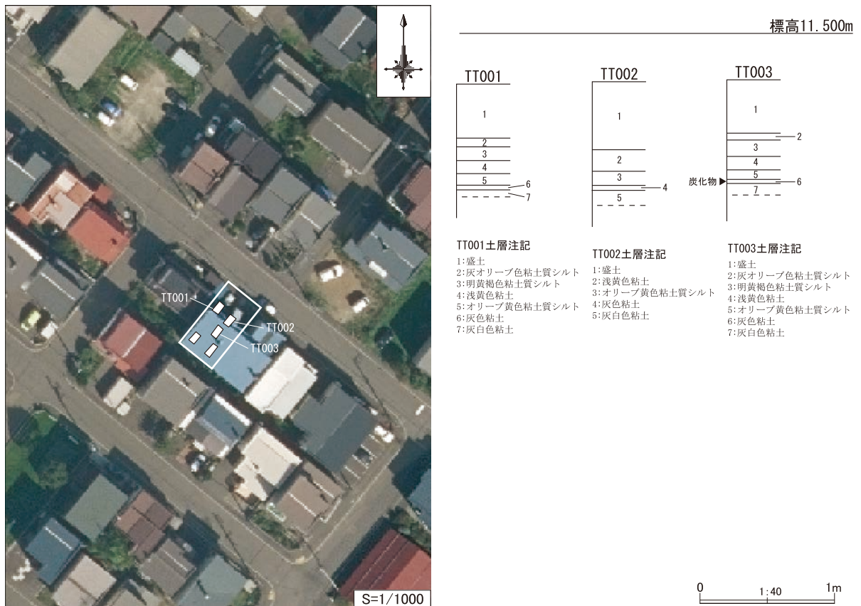
第28図 整理番号 22-2-310 試掘調査実施箇所及び土層断面模式図
