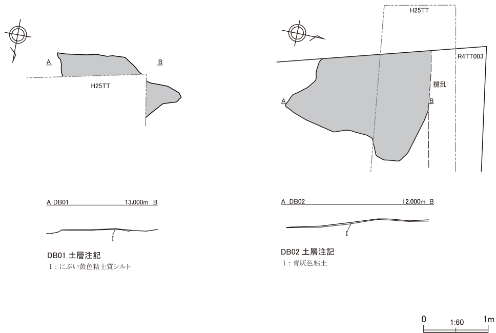
第 31 図 整理番号 22-2-311 焼土粒集中実測図
