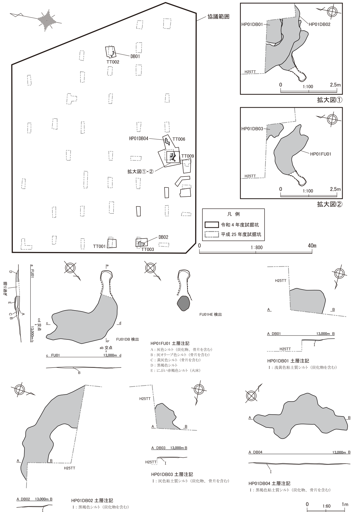
第30図 整理番号 22-2-311 遺構配置図及び竪穴住居跡附属遺構実測図
