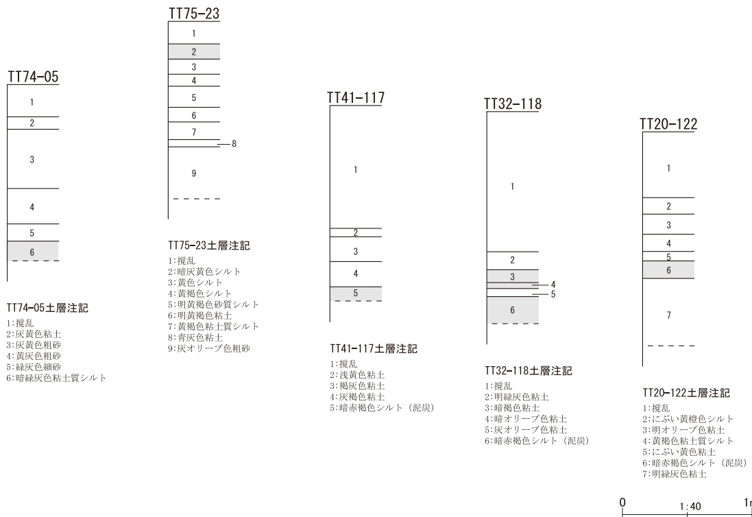
第9図 整理番号 14-3-312 試掘調査実施箇所及び土層断面模式図
