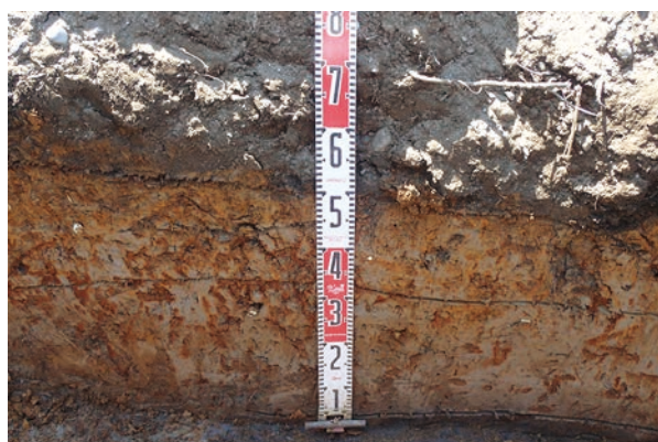
H TT004 土層断面
