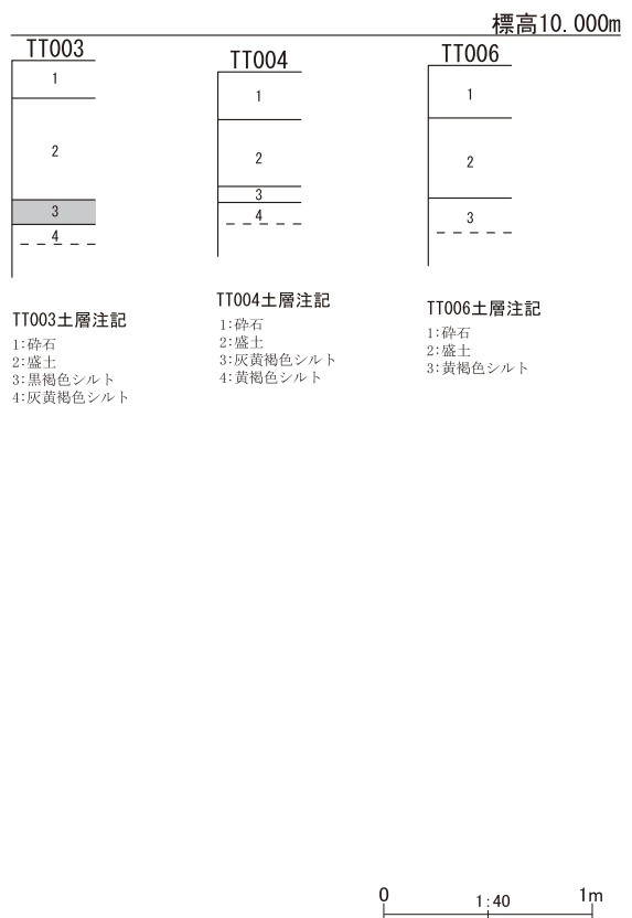
第 19 図 整理番号 22-2-301 試掘調査実施箇所及び土層断面模式図
