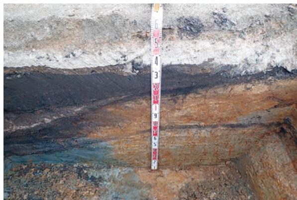
B TT11-11 土層断面
