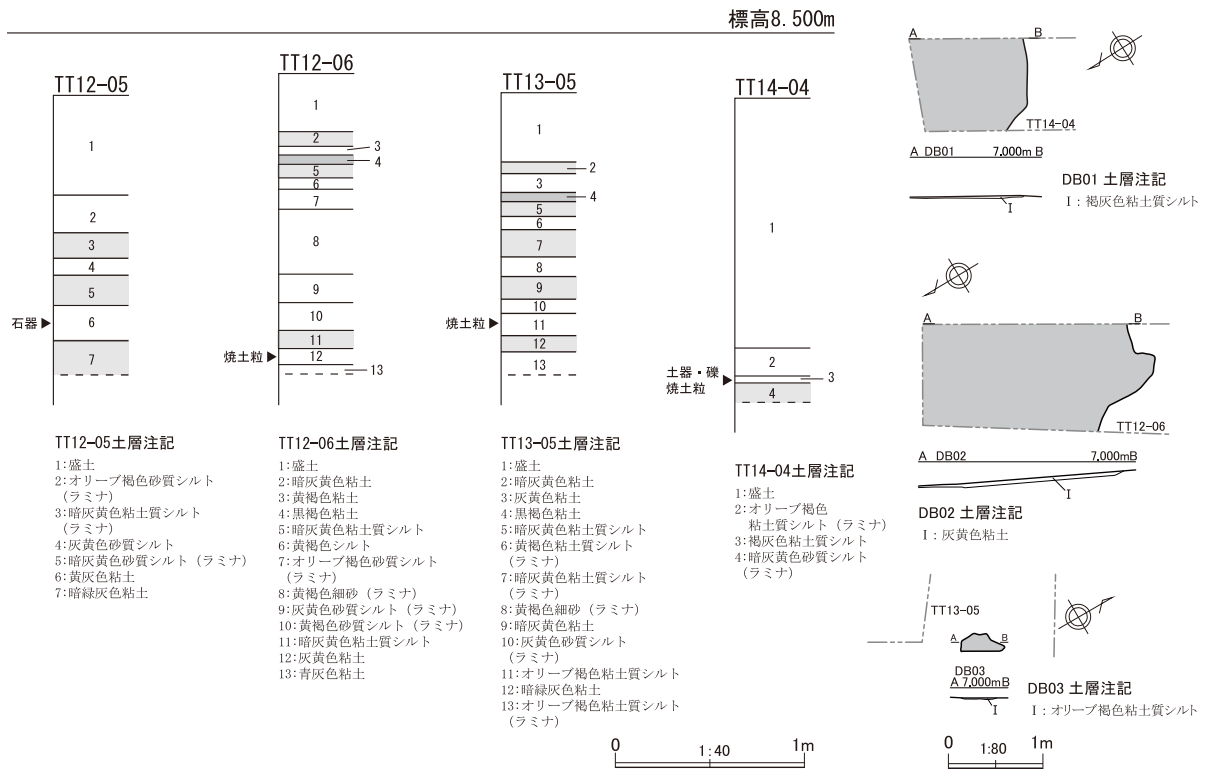
第11図 整理番号 21-3-325 試掘調査実施箇所及び土層断面模式図、焼土粒集中実測図
