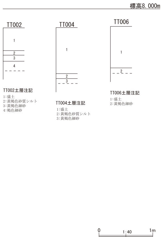
第 18 図 整理番号 21-2-316 試掘調査実施箇所及び土層断面模式図
