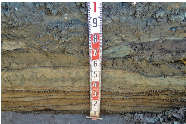
F TT06-07 土層断面
