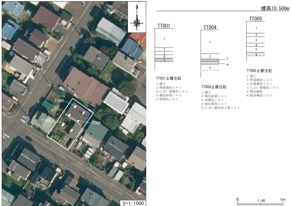
第27図 整理番号 22-2-309 試掘調査実施箇所及び土層断面模式図
