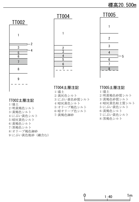
第19図 整理番号 20-2-319 試掘調査実施箇所及び土層断面模式図
