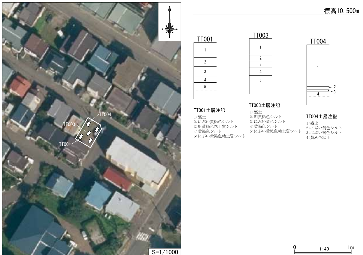
第26図 整理番号 21-2-306 試掘調査実施箇所及び土層断面模式図
