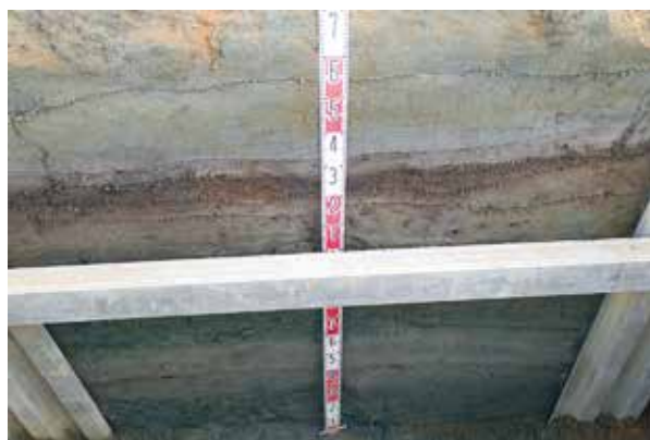
F TT06-09 土層断面
