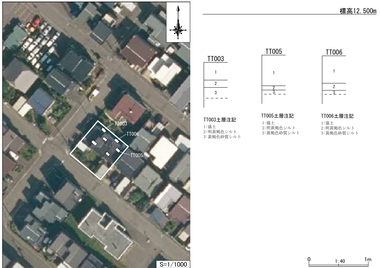
第25図 整理番号 21-2-305 試掘調査実施箇所及び土層断面模式図
