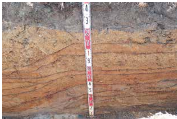
B TT07-06 土層断面
