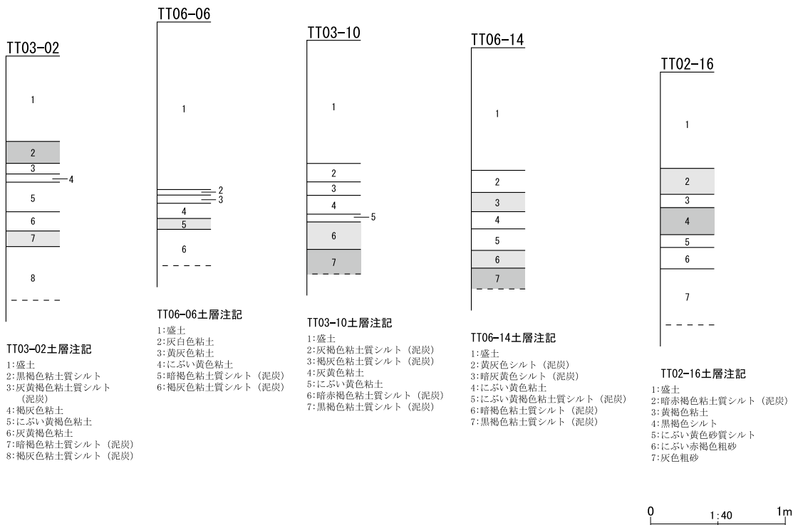
第 14 図 整理番号 20-3-320 試掘調査実施箇所及び土層断面模式図
