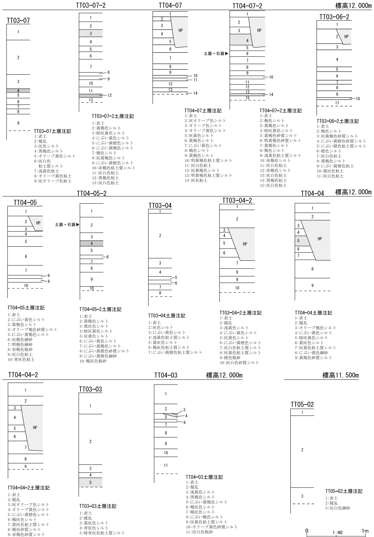
第22図 整理番号 21-2-302 土層断面模式図
