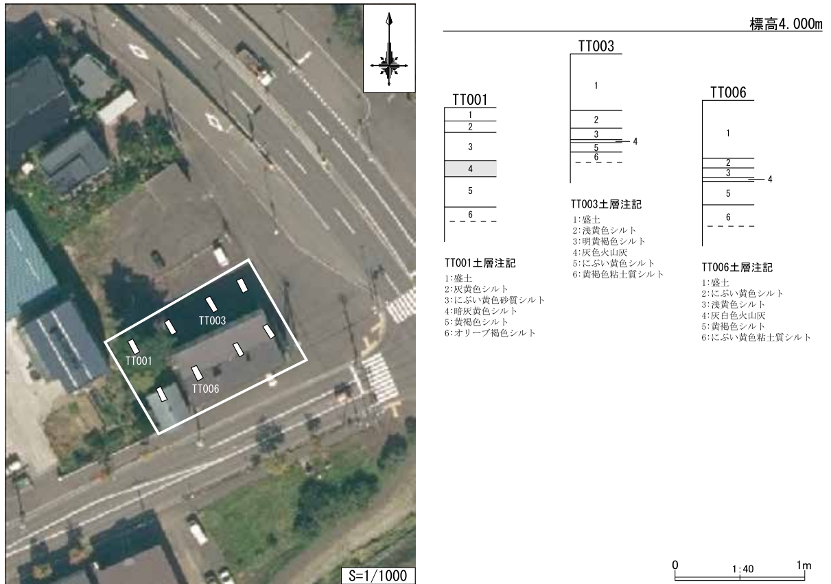
第 29 図 整理番号 21-2-309 試掘調査実施箇所及び土層断面模式図
