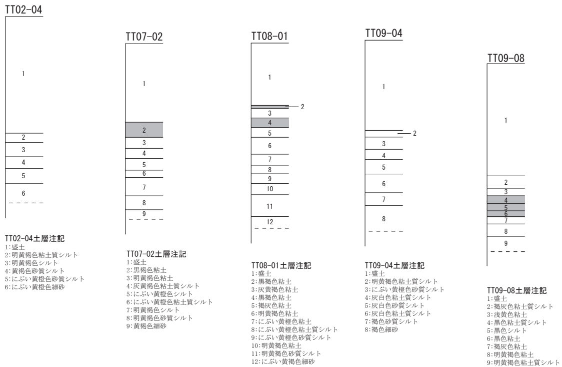
第 25 図 整理番号 18-2-303 試掘調査実施箇所及び土層断面模式図
