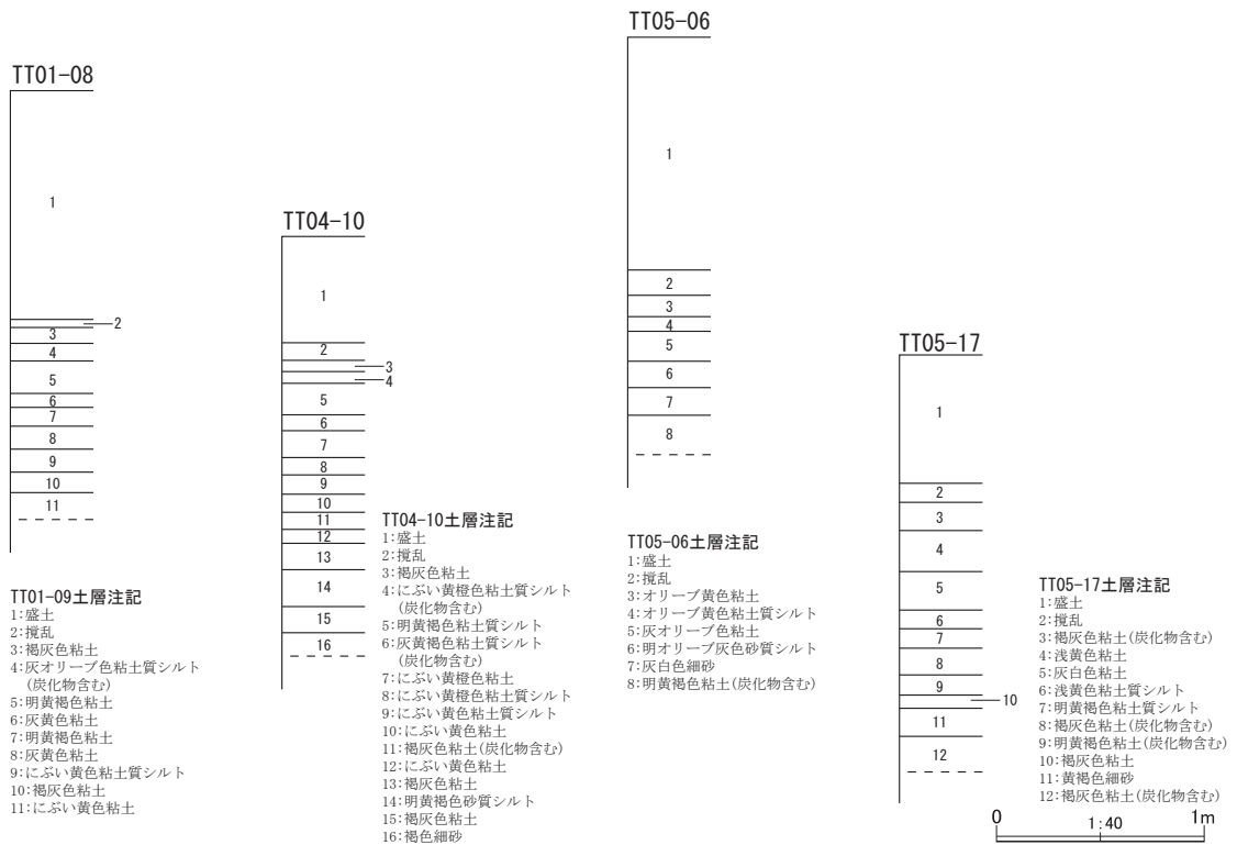
第 17 図 整理番号 18-3-303 試掘調査実施箇所及び土層断面模式図
