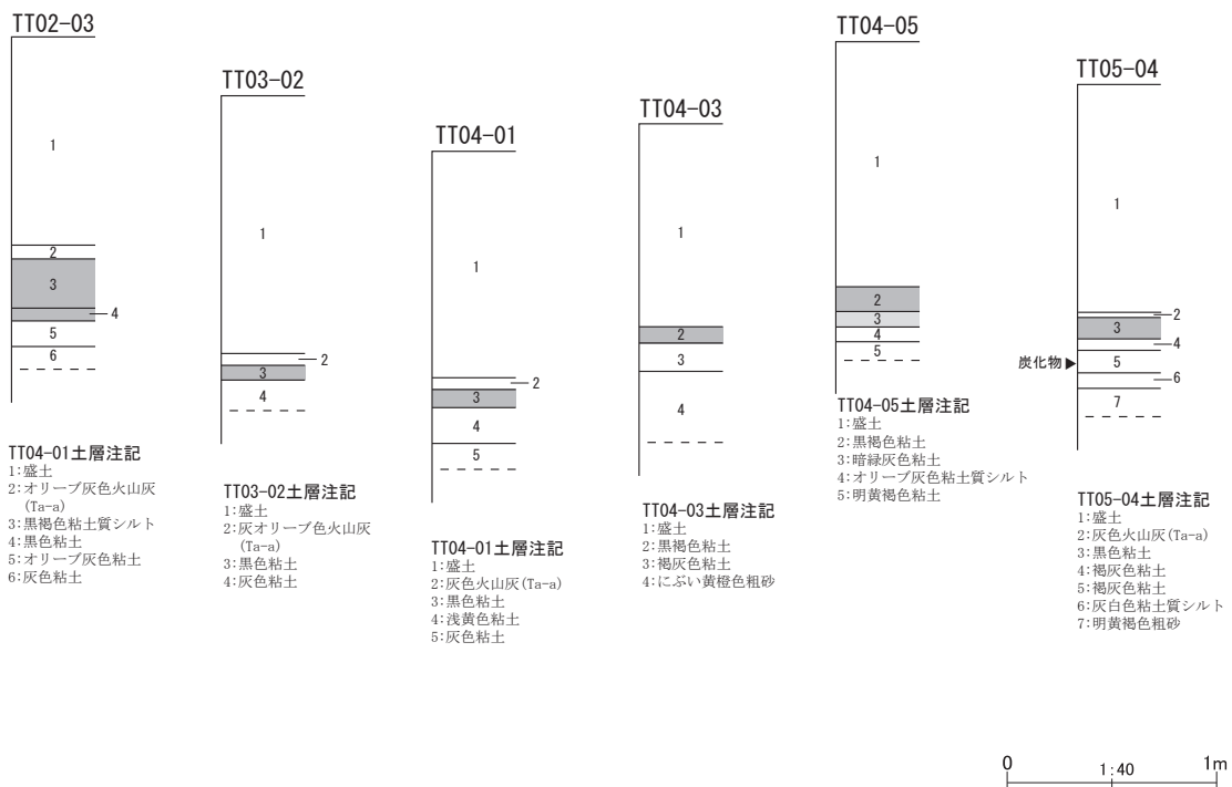
第 22 図 整理番号 17-2-317 試掘調査実施箇所及び土層断面模式図
