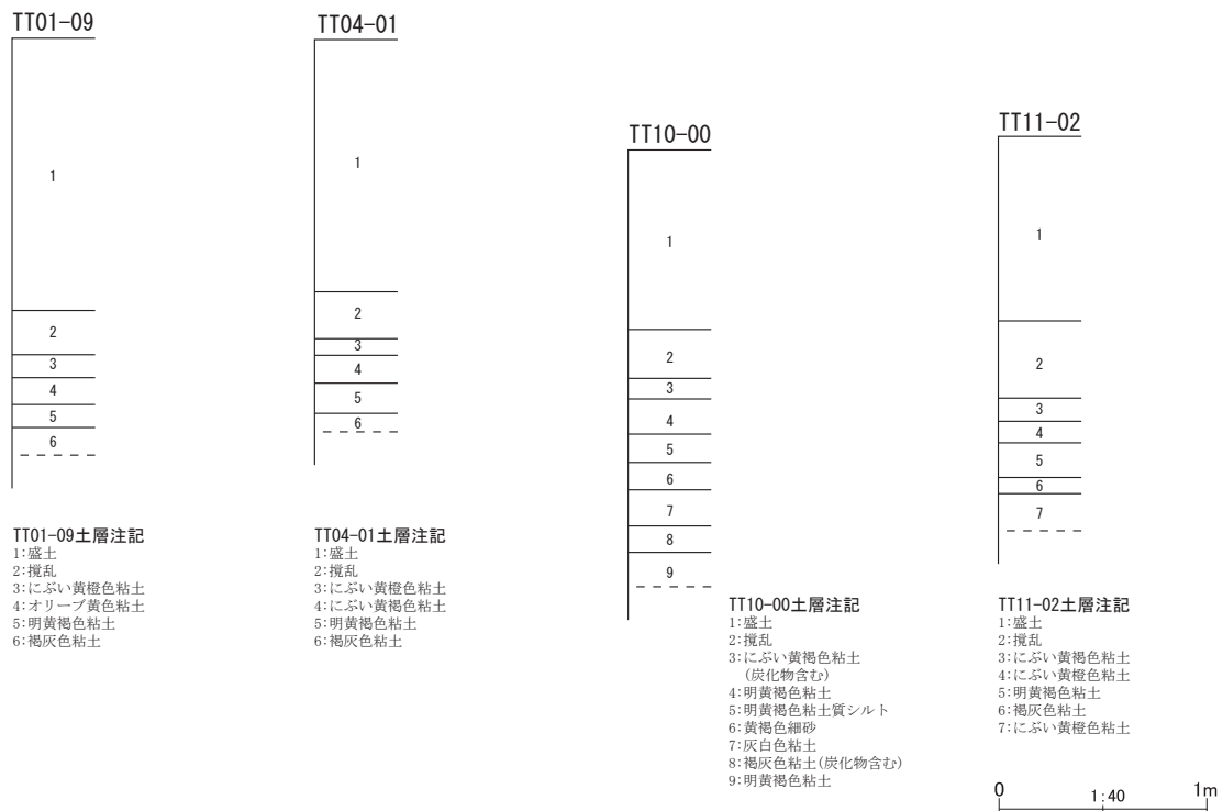
第16図 整理番号 18-3-301 試掘調査実施箇所及び土層断面模式図
