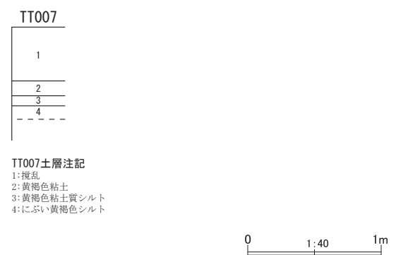
第23図 整理番号 18-2-301 試掘調査実施箇所及び土層断面模式図
