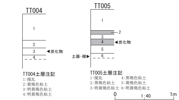
第 28 図 整理番号 18-2-307 試掘調査実施箇所及び土層断面模式図
