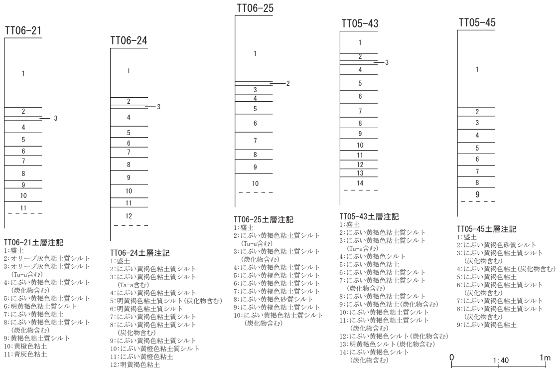
第12図 整理番号15-3-323 試掘調査実施箇所及び土層断面模式図
