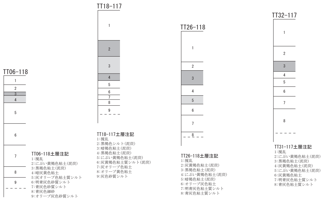
第7図 整理番号 07-3-325 試掘調査実施箇所及び土層断面模式図
