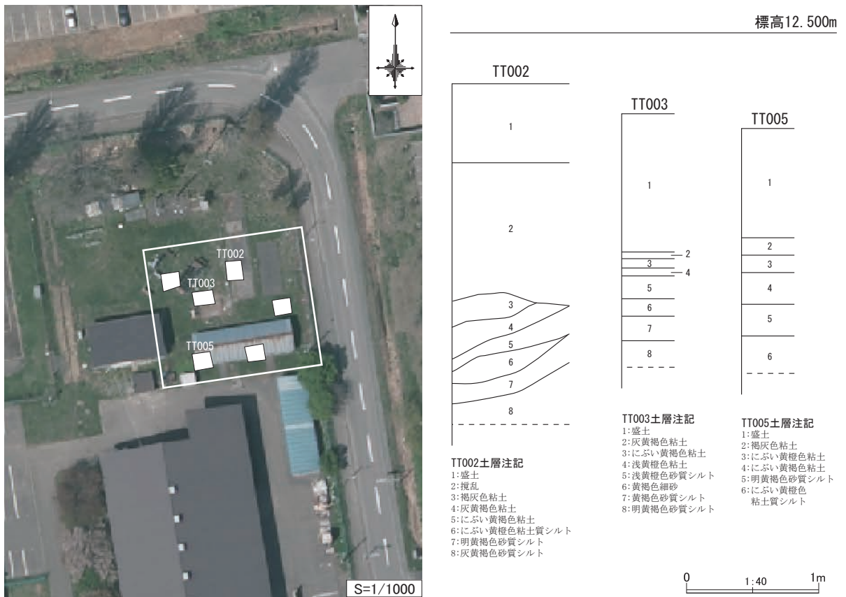
第20図 整理番号17-2-315 試掘調査実施箇所及び土層断面模式図
