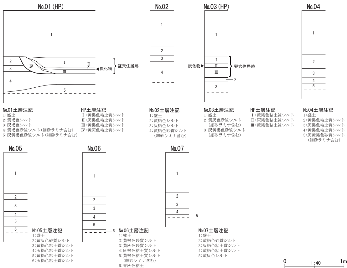
第33図 整理番号 18-3-003 工事立会実施箇所及び土層断面模式図
