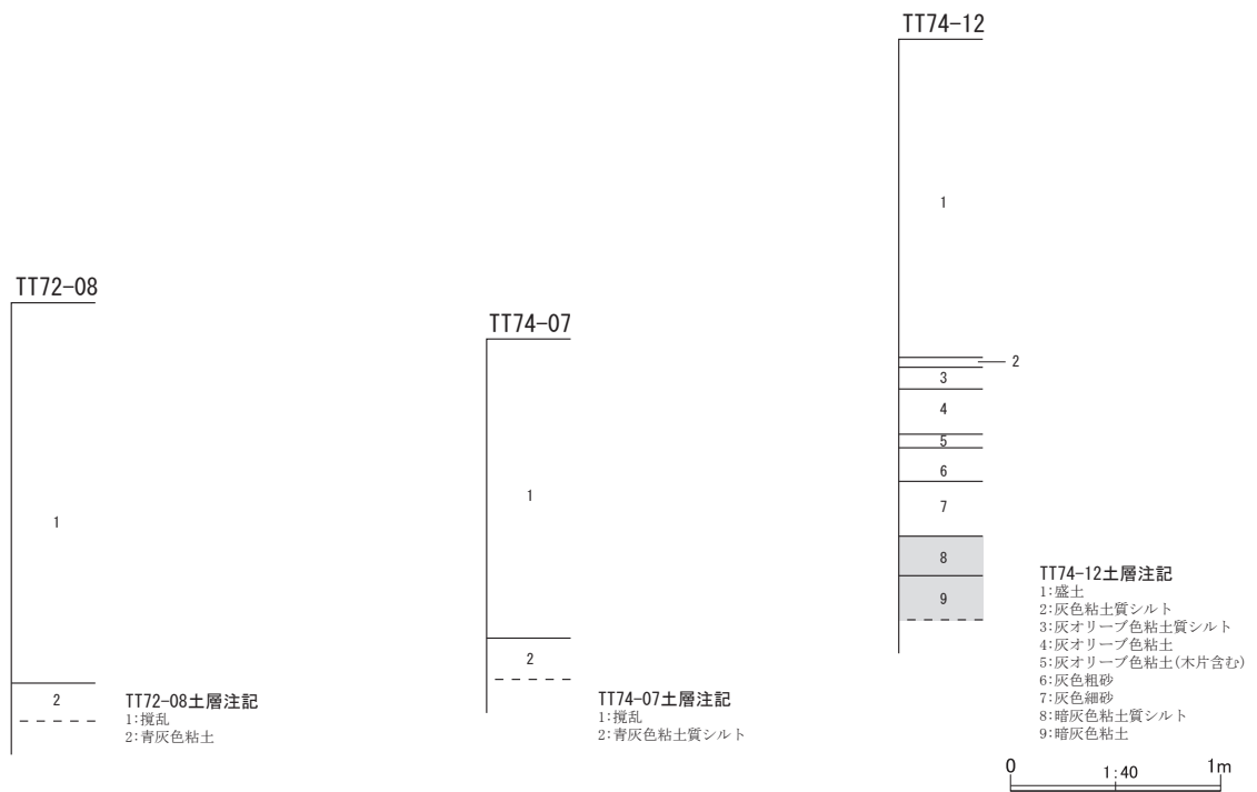
第8図 整理番号 14-3-312 試掘調査実施箇所及び土層断面模式図
