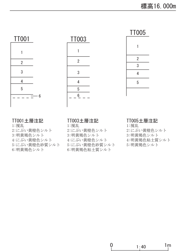
第 29 図 整理番号 18-2-308 試掘調査実施箇所及び土層断面模式図
