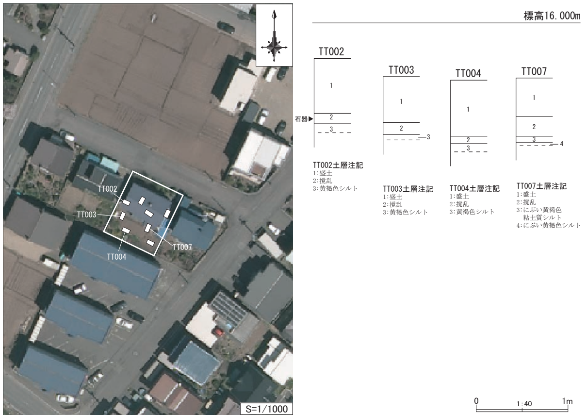
第21図 整理番号17-2-319 試掘調査実施箇所及び土層断面模式図
