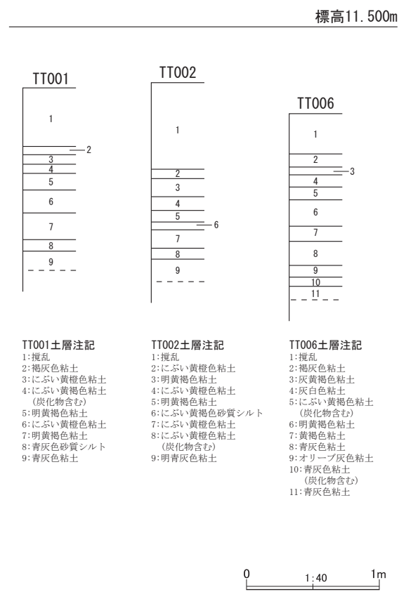
第24図 整理番号 18-2-302 試掘調査実施箇所及び土層断面模式図
