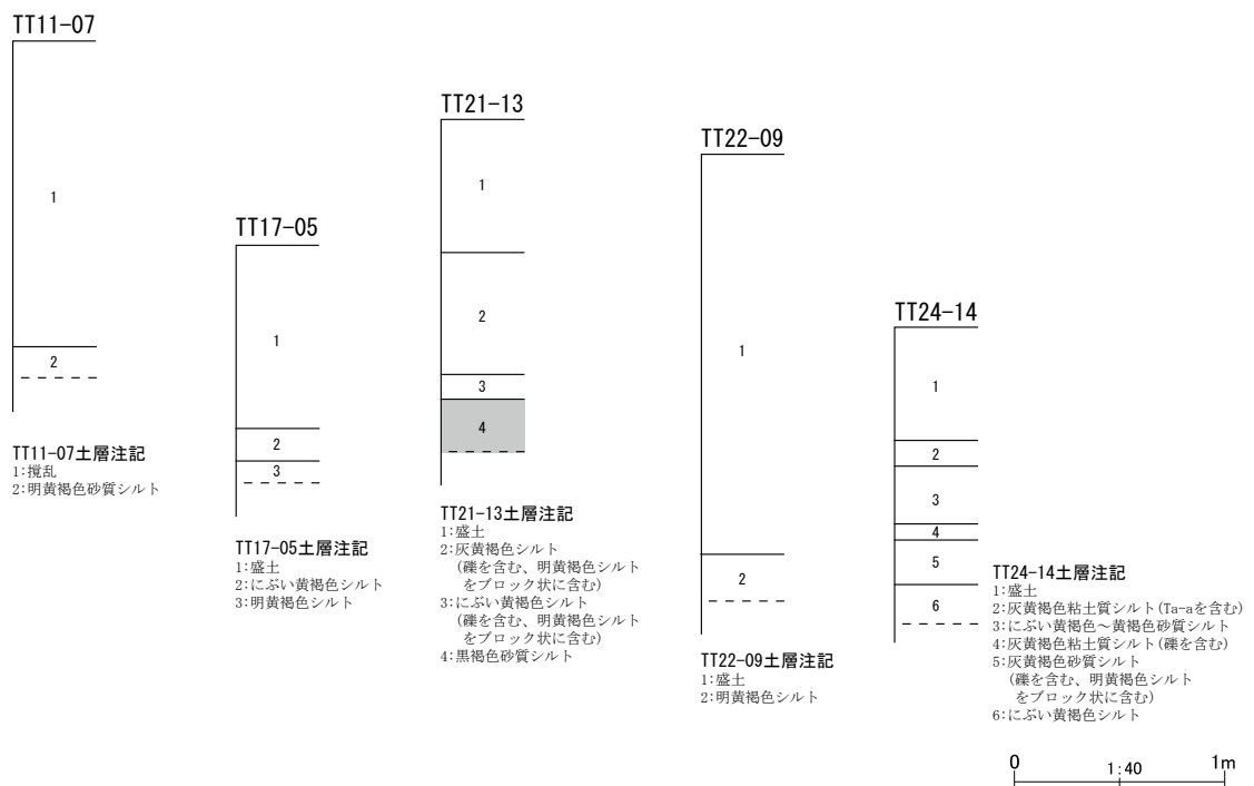
第16図 整理番号 16-3-304 試掘調査実施箇所及び土層断面模式図
