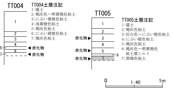
第 28 図 整理番号 16-2-317 試掘調査実施箇所及び土層断面模式図
