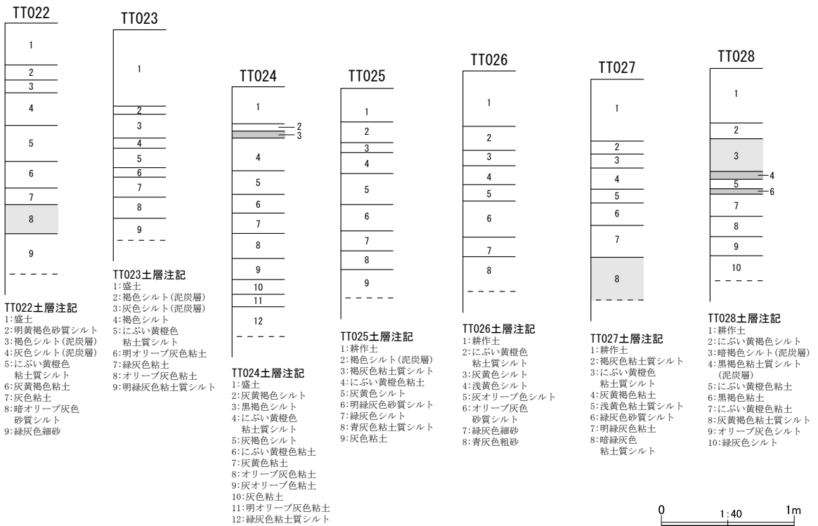
第7図 整理番号 10-3-318 試掘調査実施箇所及び土層断面模式図
