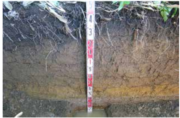
B TT35-94 土層断面
