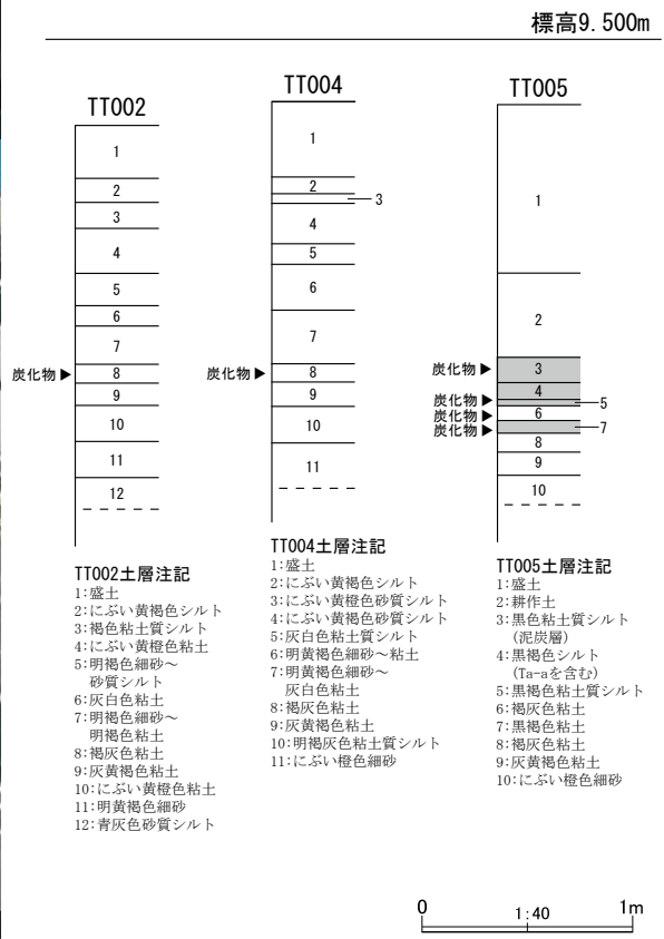
第 22 図 整理番号 17-3-303 試掘調査実施箇所及び土層断面模式図
