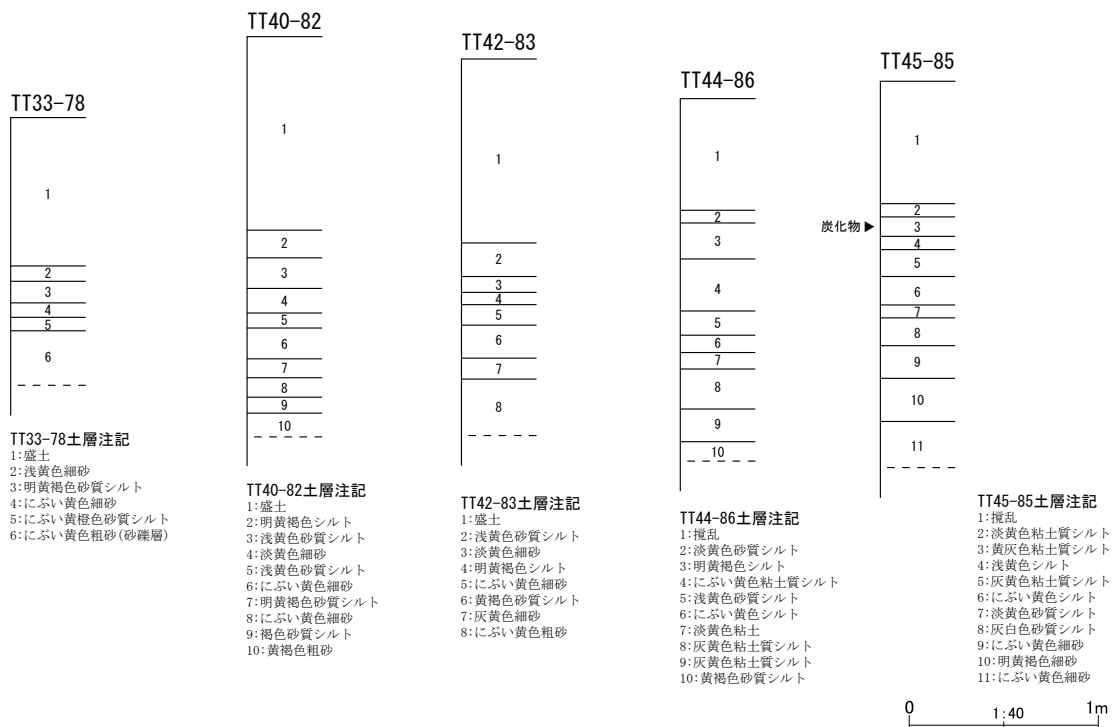
第12図 整理番号 14-3-321 試掘調査実施箇所及び土層断面模式図
