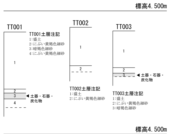
第 28 図 整理番号 16-2-317 試掘調査実施箇所及び土層断面模式図
