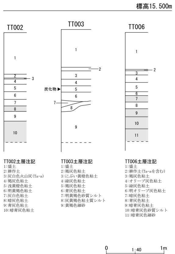
第 21 図 整理番号 17-3-302 試掘調査実施箇所及び土層断面模式図
