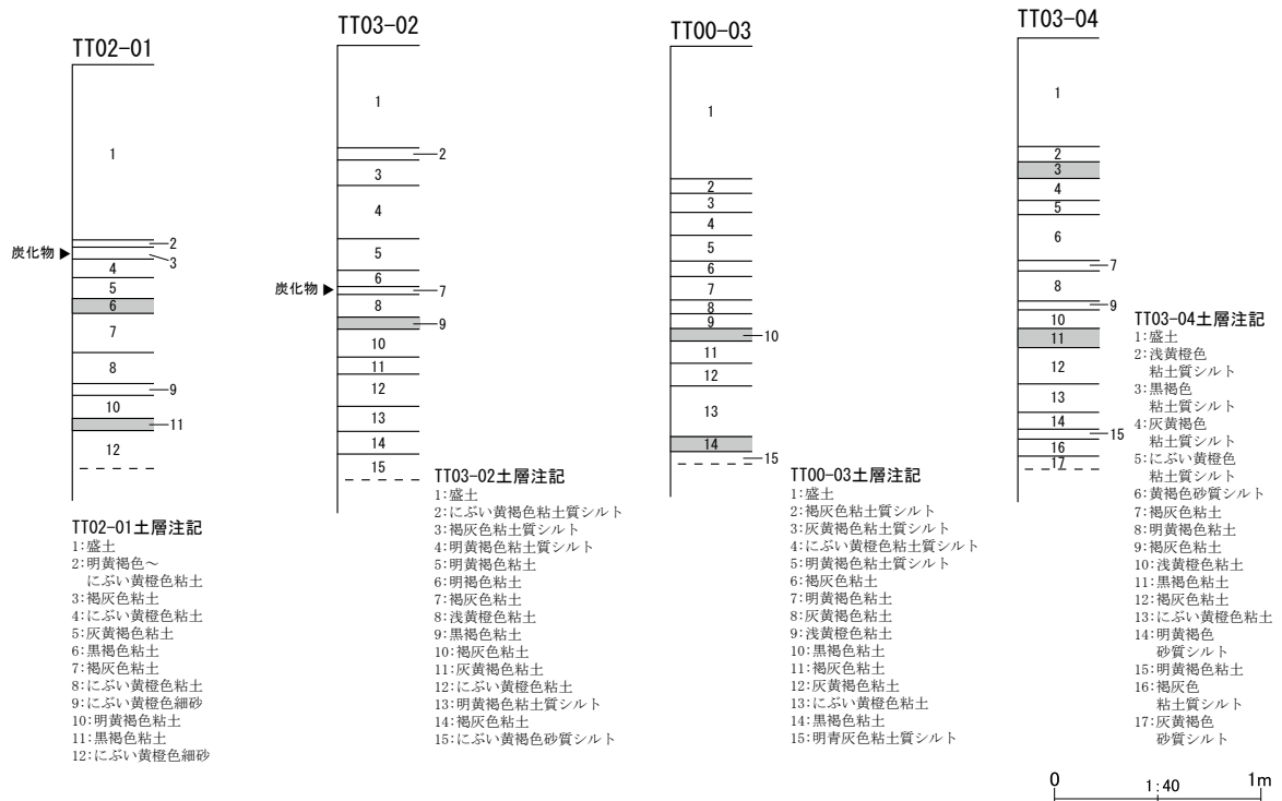
第27図 整理番号17-3-315 試掘調査実施箇所及び土層断面模式図
