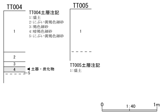
第 29 図 整理番号 16-2-318 試掘調査実施箇所及び土層断面模式図
