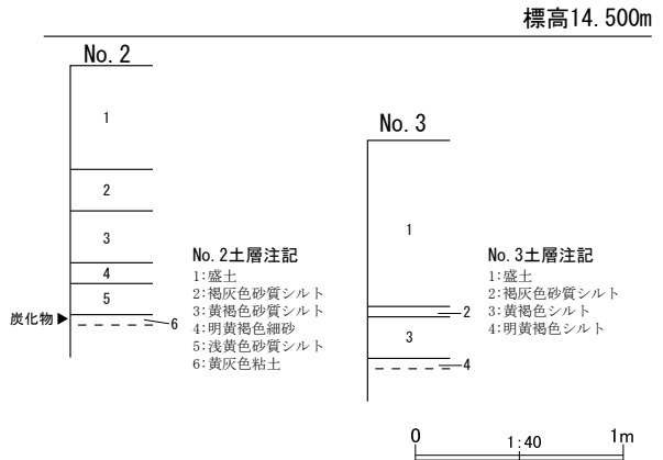
第 36 図 整理番号 17-3-003 工事立会実施箇所及び土層断面模式図
