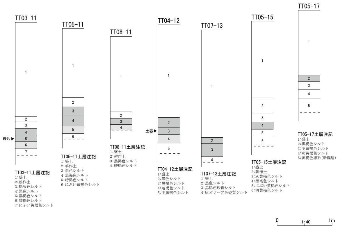
第25図 整理番号17-3-308 試掘調査実施箇所及び土層断面模式図
