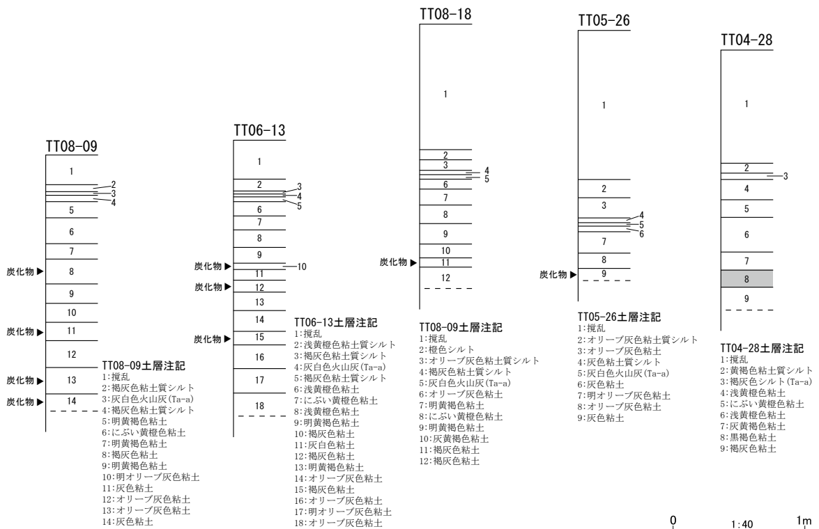
第14図 整理番号 15-3-319 試掘調査実施箇所及び土層断面模式図
