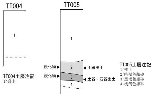
第31図 整理番号16-2-315 試掘調査実施箇所及び土層断面模式図
