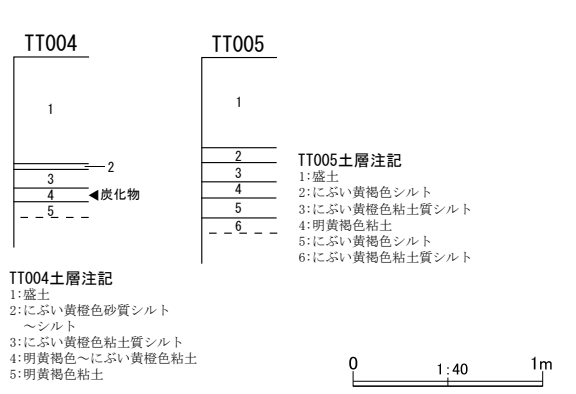
第16図 整理番号15-2-315 試掘調査実施箇所及び土層断面模式図
