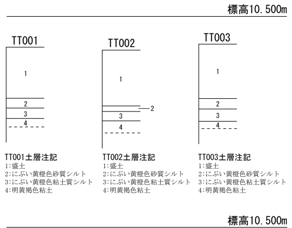
第15図 整理番号15-2-314 試掘調査実施箇所及び土層断面模式図
