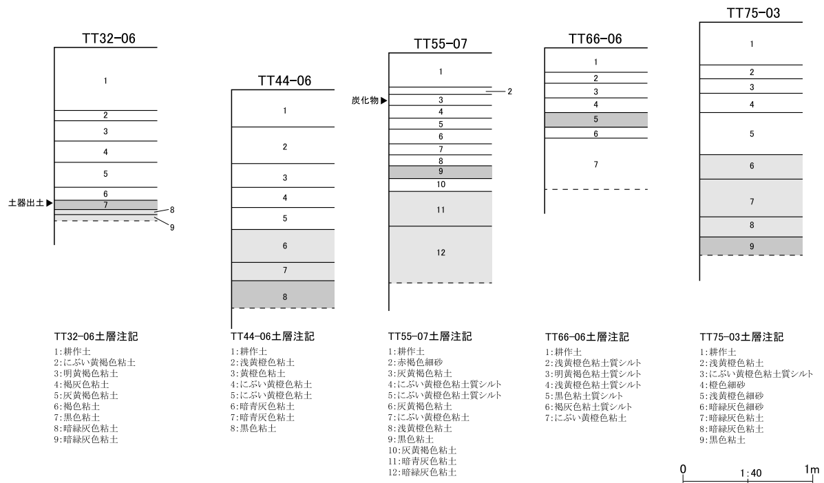
第19図 整理番号10-3-321 試掘調査土層断面模式図
