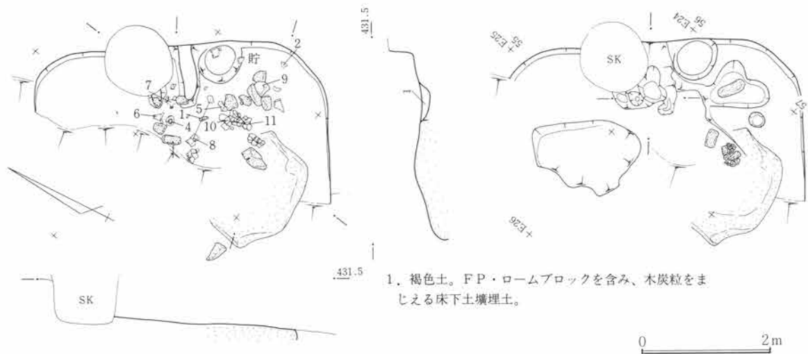
第286図 SJ80遺構図 1:80
