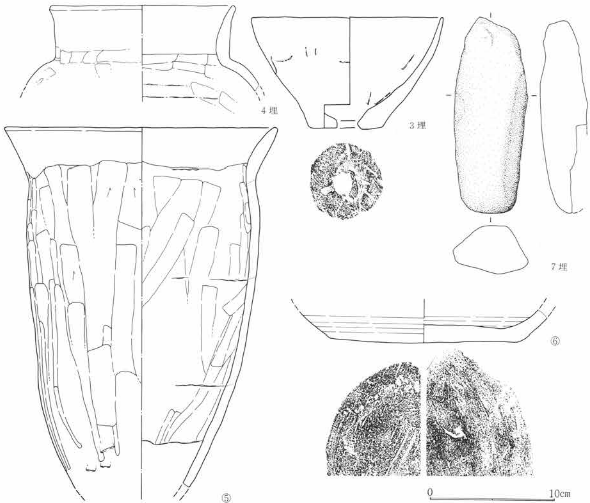
第482図 SJ157出土遺物図 1:3
