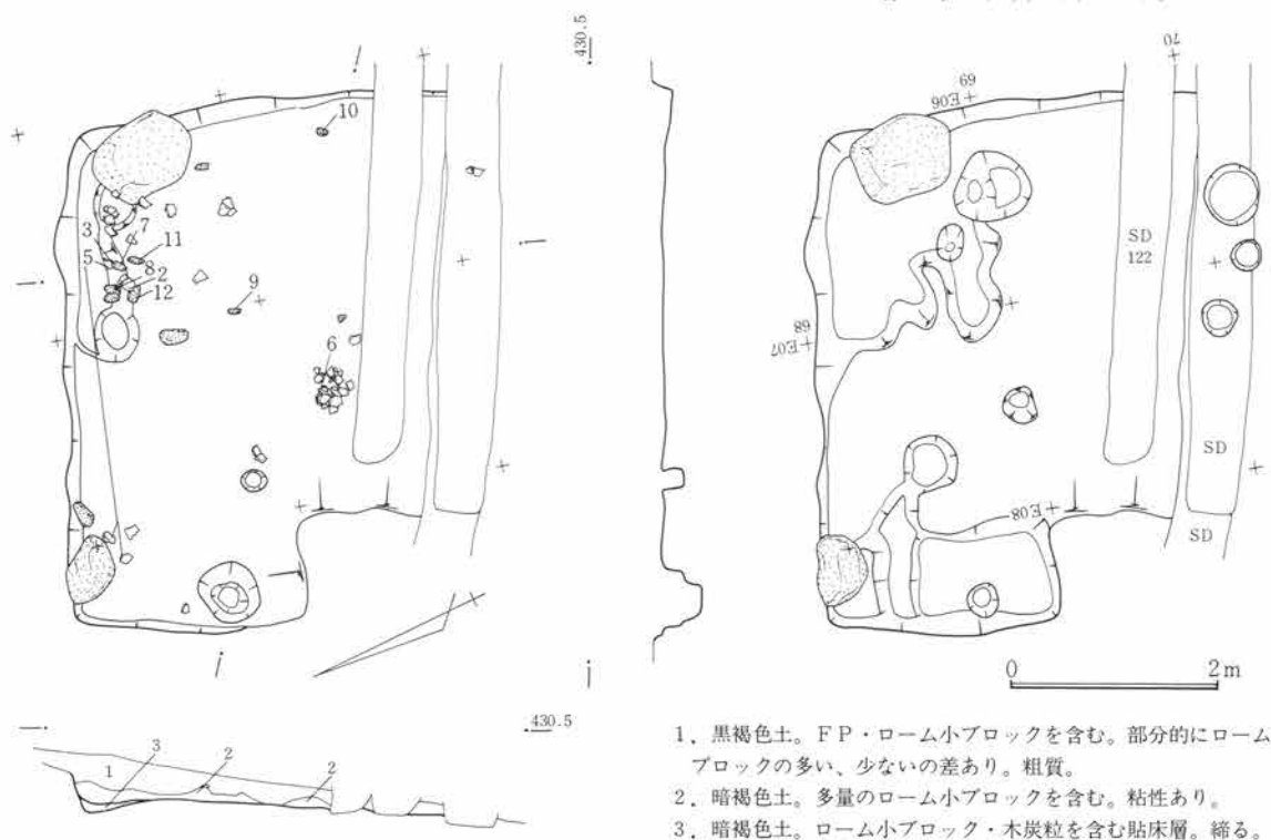
第264図 SJ71遺構図 1:80
