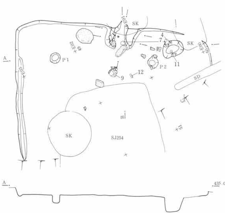
第296図 SJ83遺構図 1:80
