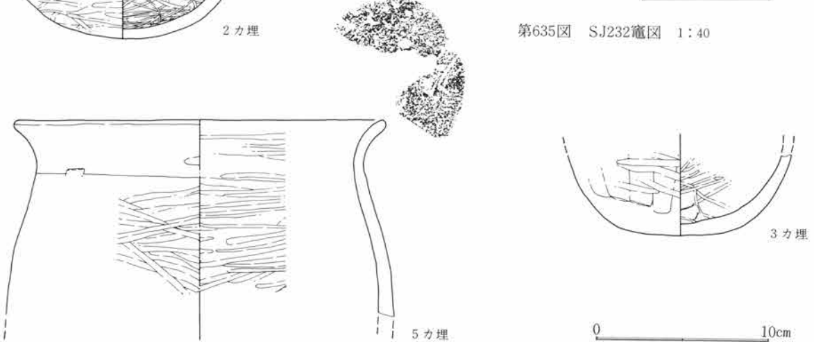
第636図 SJ232出土遺物図 1:3
