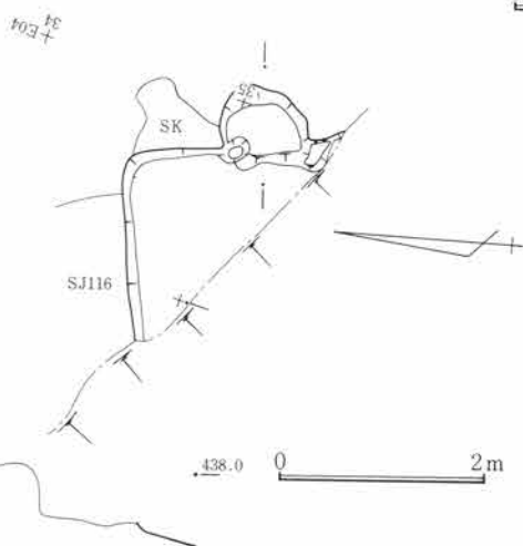
第394図 SJ115遺構図 1:80
