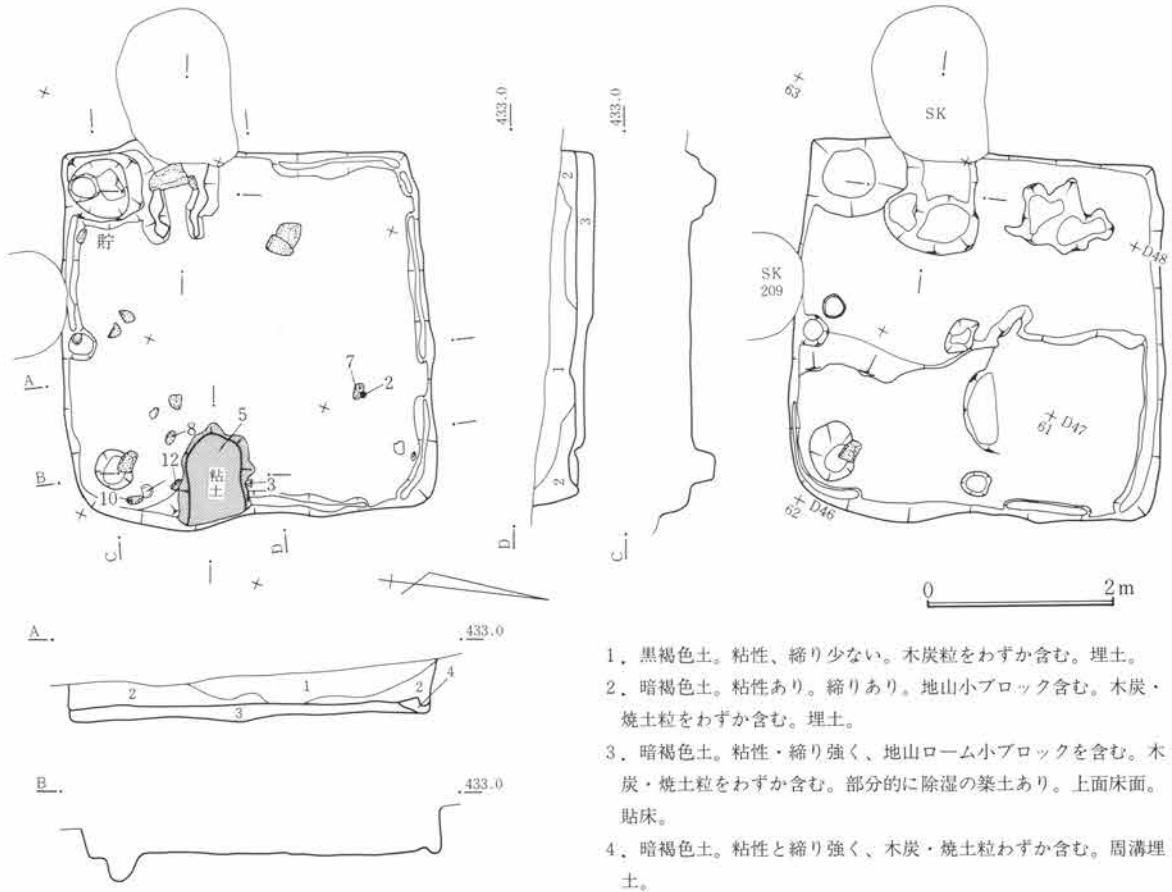
第115図 SJ27遺構図 1:80
