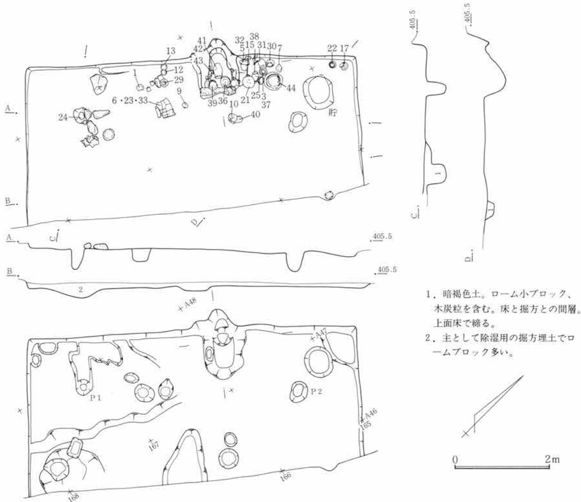
第467図 SJ149遺構図 1 : 80
