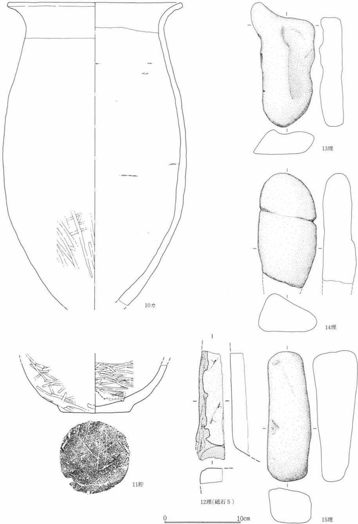
第300図 SJ83出土遺物図 1:3
