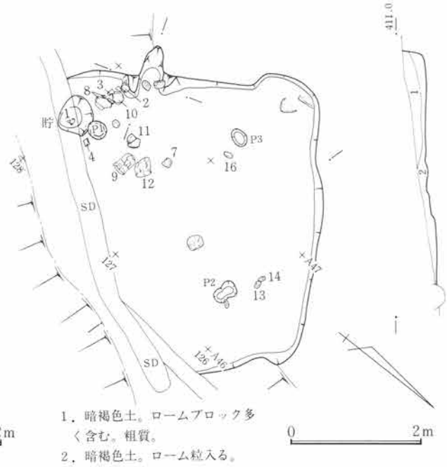
第519図 SJ174遺構図 1:80
