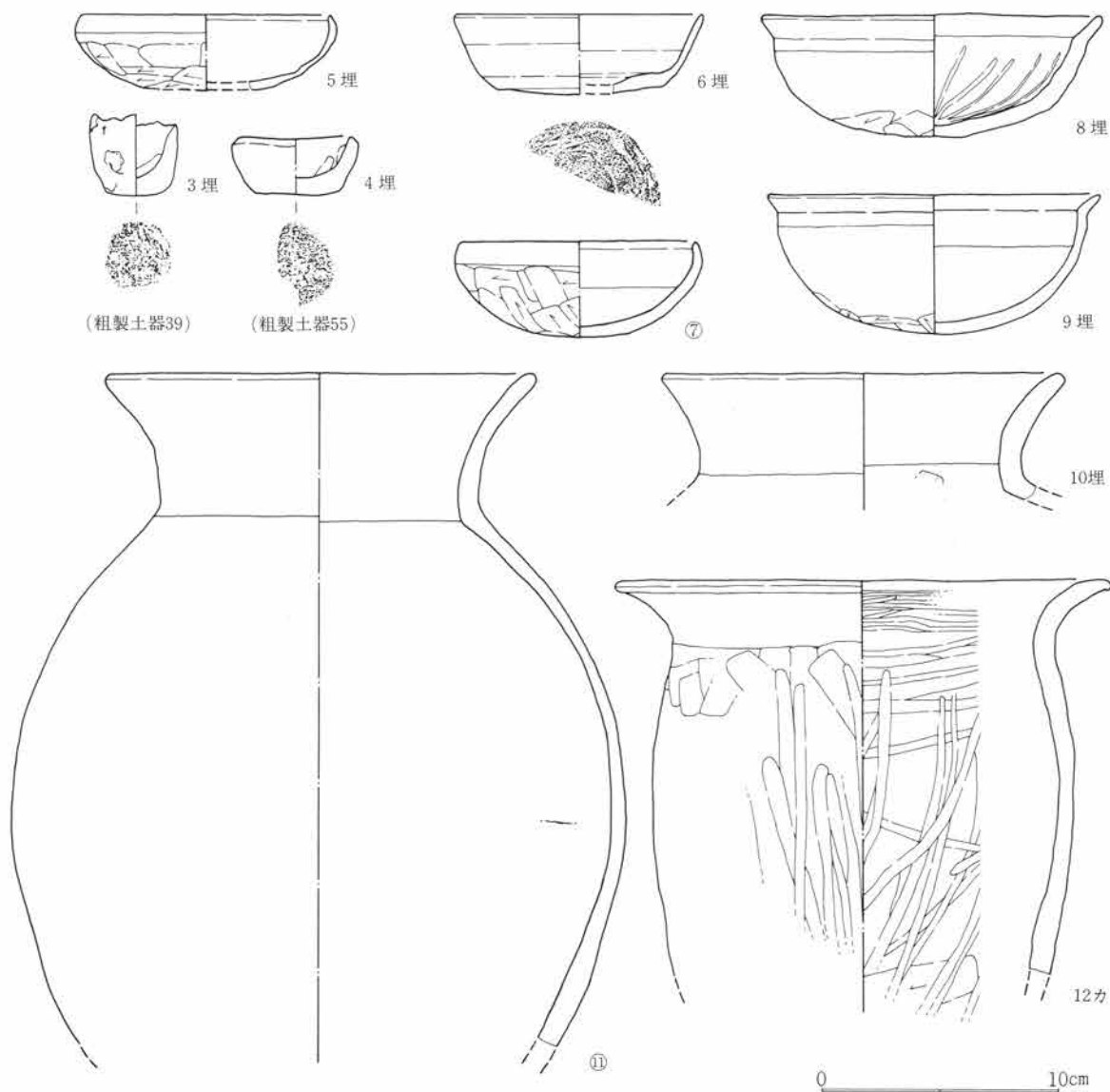
第189図 SJ48出土遺物図 1:3
