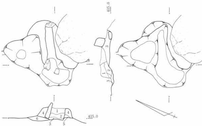
第589図 SJ211竈図 1:40
