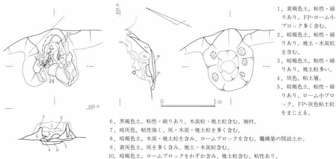
第141図 SJ34竈図 1:40
