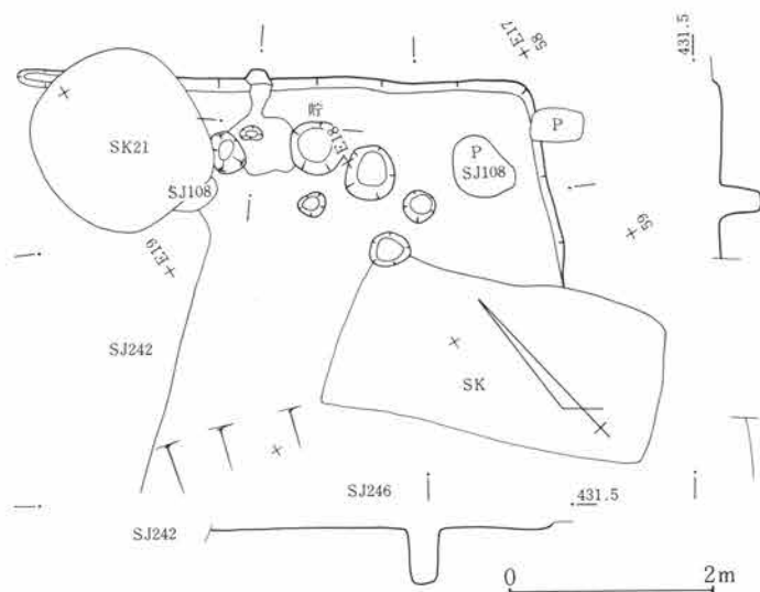
第660図 SJ240遺構図 1:80
