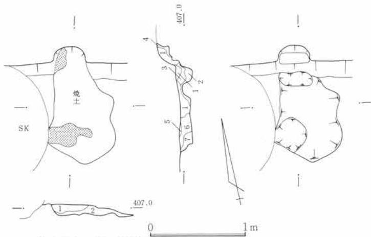
第487図 SJ160旧竈図 1:40
