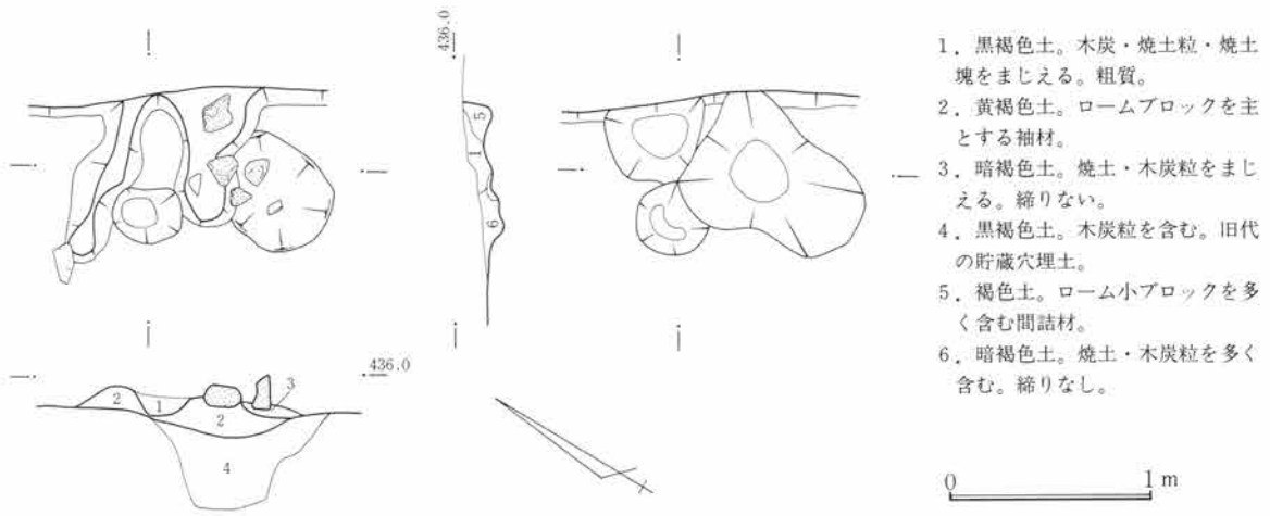
第249図 SJ65竈図 1:40
