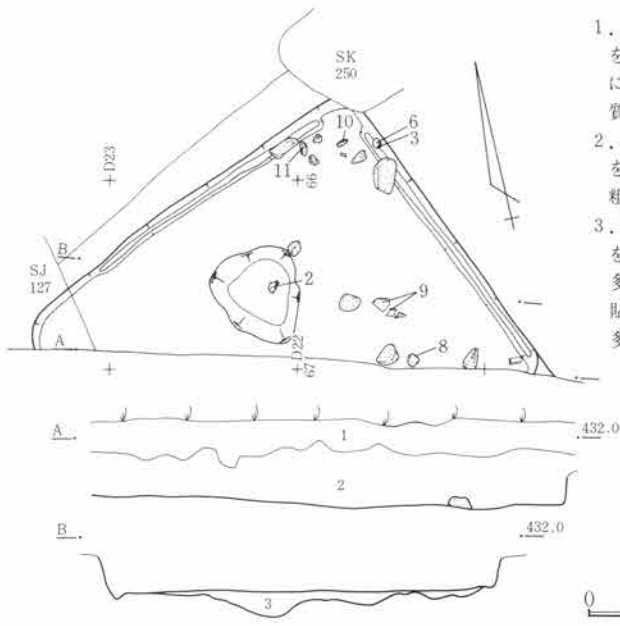
第422図 SJ128遺構図 1:80
