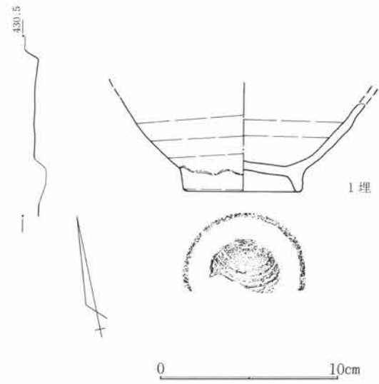
第736図 SJ274出土遺物図 1:3
