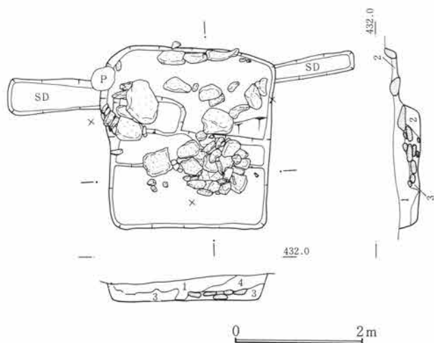
第696図 SJ260遺構図 1:80
