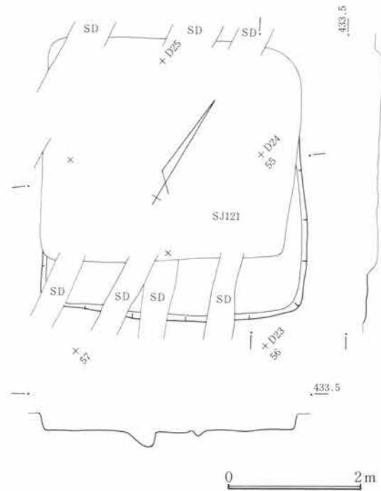
第689図 SJ255遺構図 1:80
