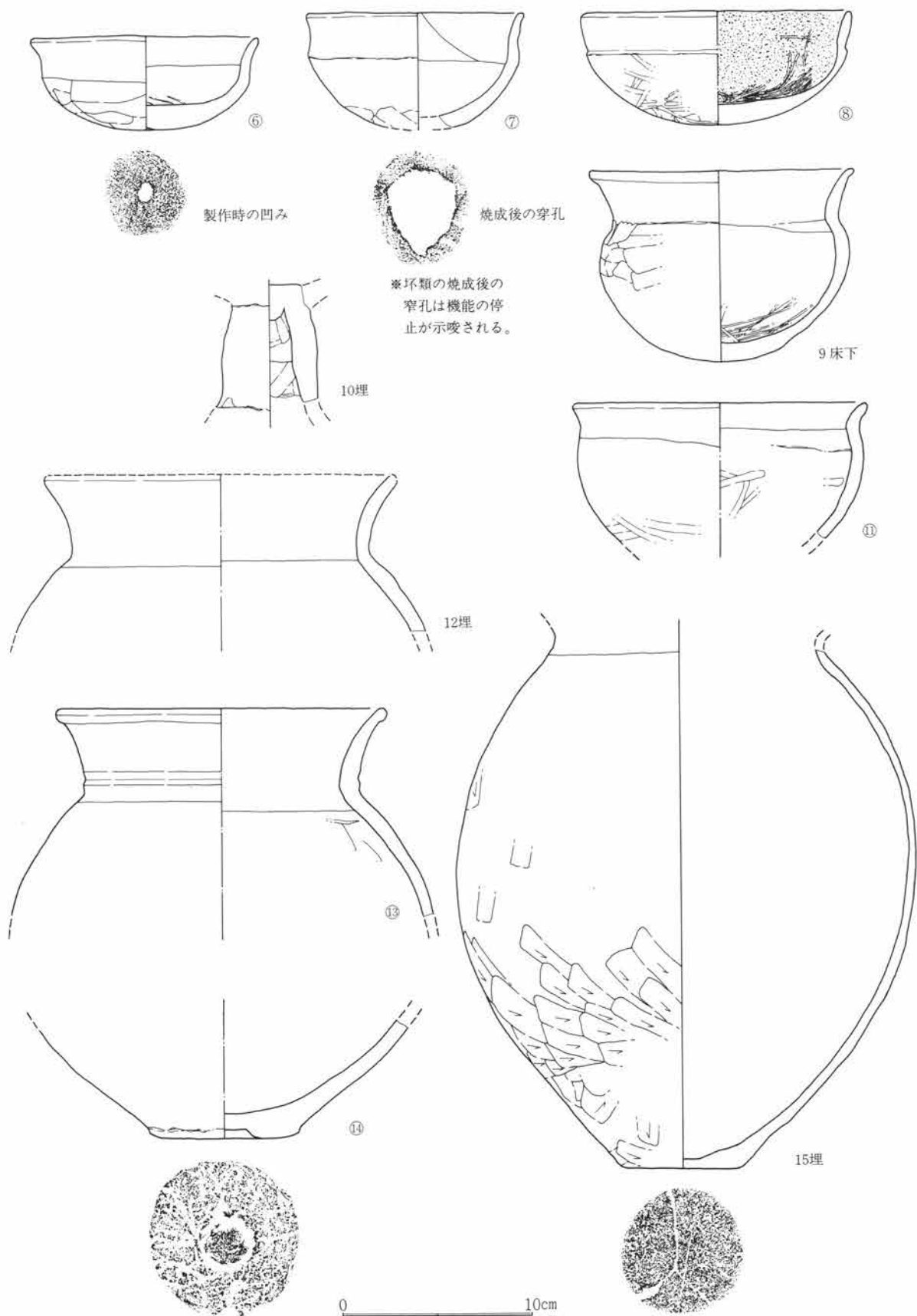
第335図 SJ93出土遺物図 1:3
