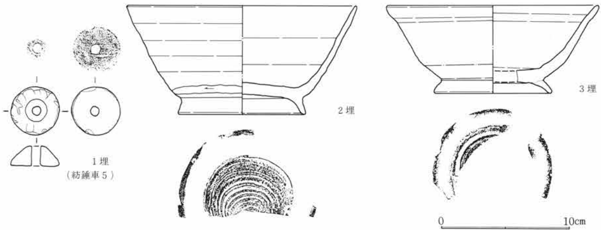
第692図 SJ257出土遺物図 1:3
