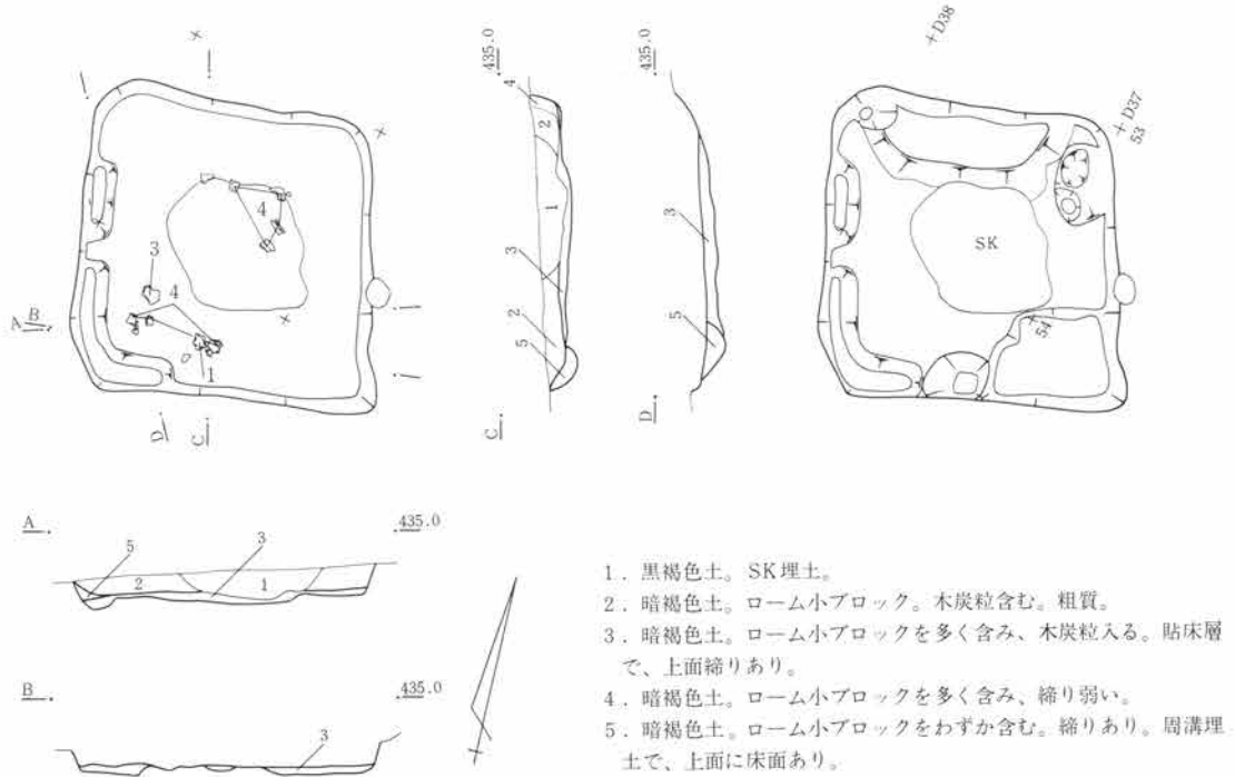
第686図 SJ253遺構図 1:80
