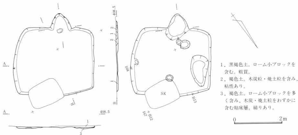
第491図 SJ161遺構図 1:80
