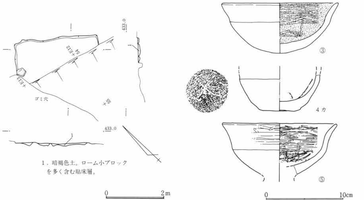
第622図 SJ225遺構図 1:80
