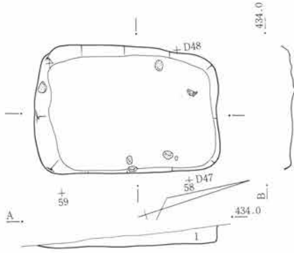
第138図 SJ33遺構図 1:80
