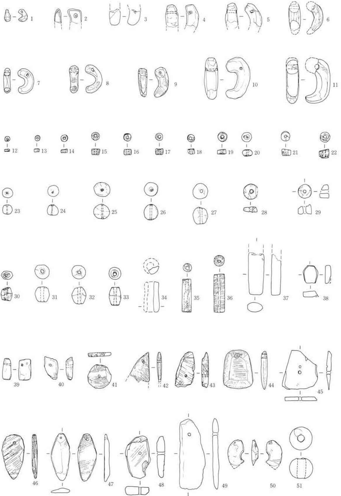
第871図 玉類・石製模造品 1:2 1~36玉類、37・38石墨、39~49石製模造品、50块状耳飾、51数珠
