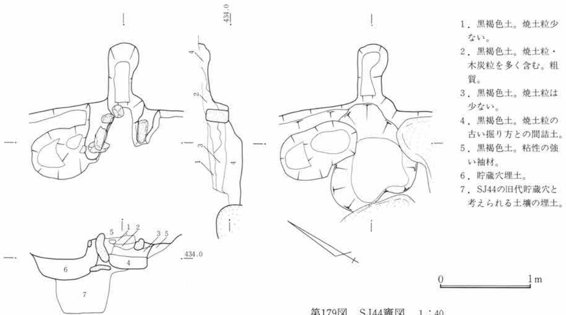
第179図 SJ44竈図 1:40
