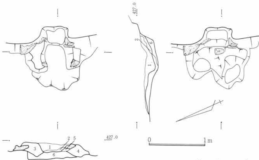
第227図 SJ59竈図 1 : 40
