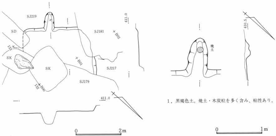
第613図 SJ220竈図 1:40
