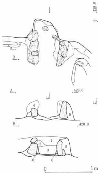
第217図 SJ56竈図 1:40
