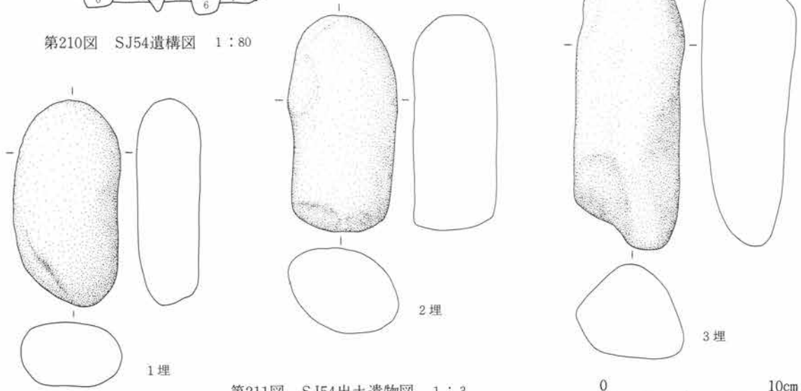
第211図 SJ54出土遺物図 1 : 3
