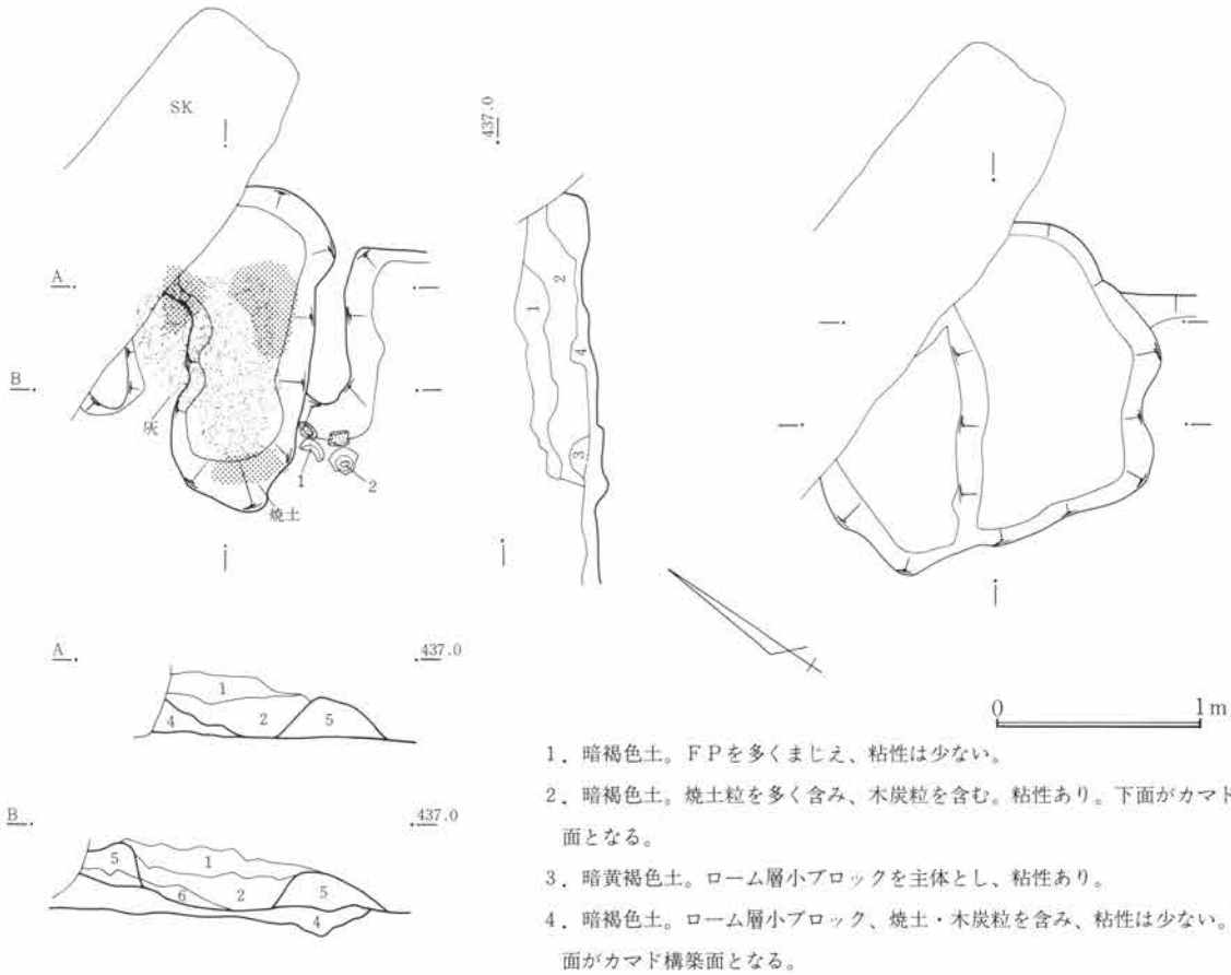
第84図 SJ16竈図 1:40
