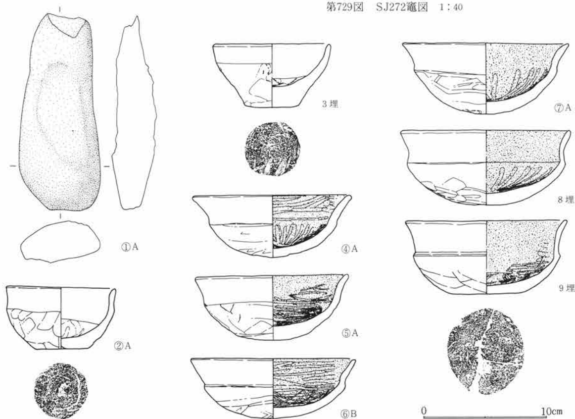
第730図 SJ272出土遺物図 1:3
