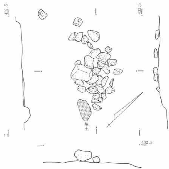
第415図 SJ125集石図 1:40
