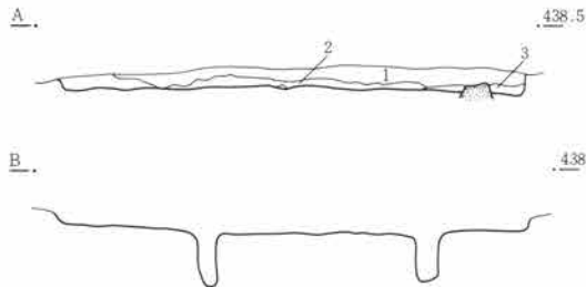
第88図 SJ18遺構図 1 : 80
