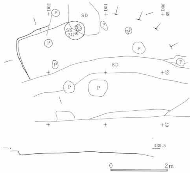
第735図 SJ274遺構図 1:80
