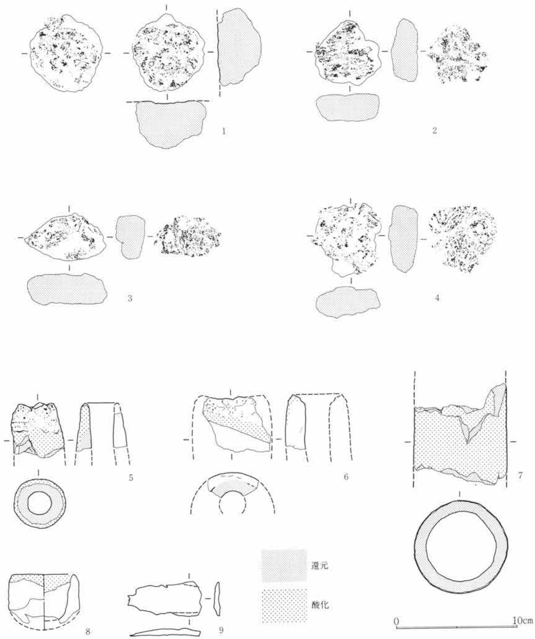
第887図 壁体・羽口・溶解金属 1:3
