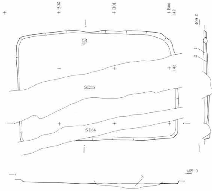
第501図 S J 166遺構図 1:80
