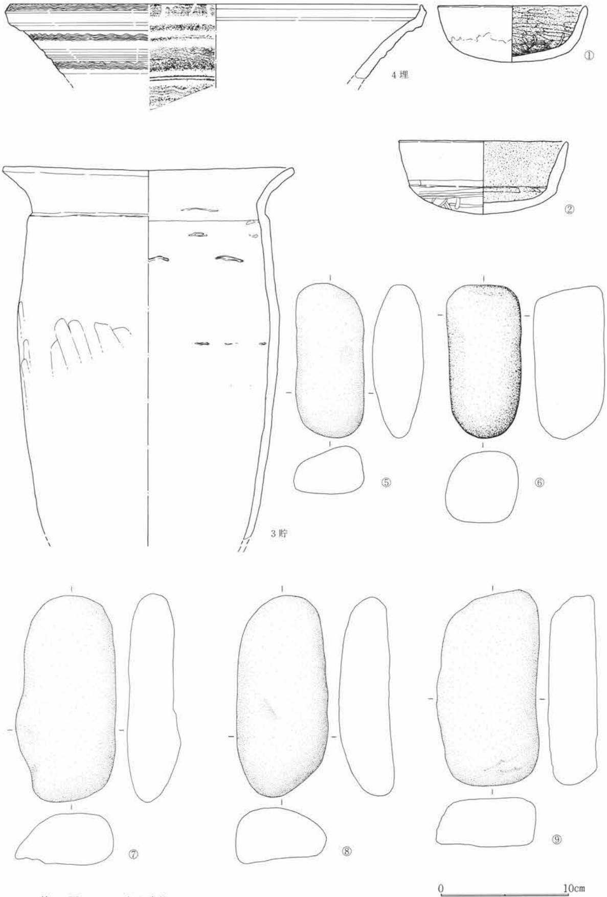
第417図 SJ125出土遺物図 1:3
