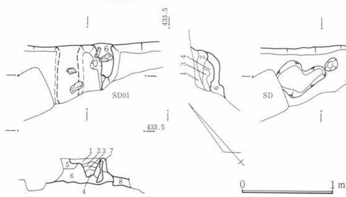
第184図 SJ47竈図 1 : 40
