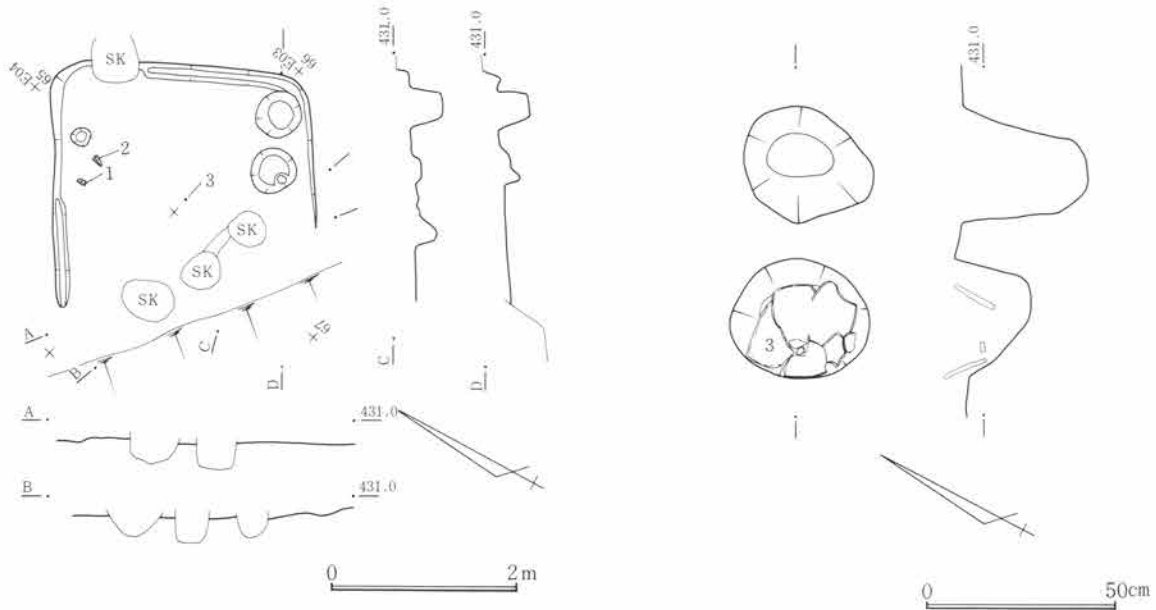
第856図 SJ90遺構図 (住居図1:80 炉跡図1:20)
