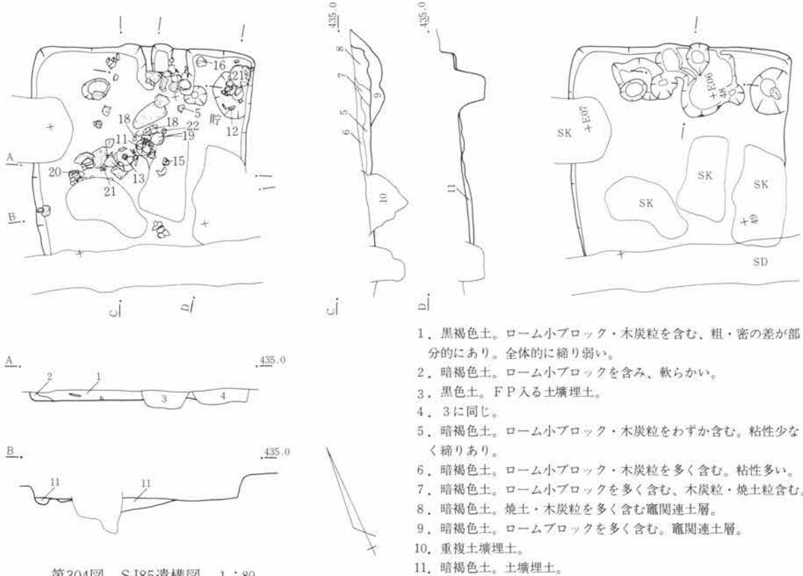
第304図 SJ85遺構図 1:80
