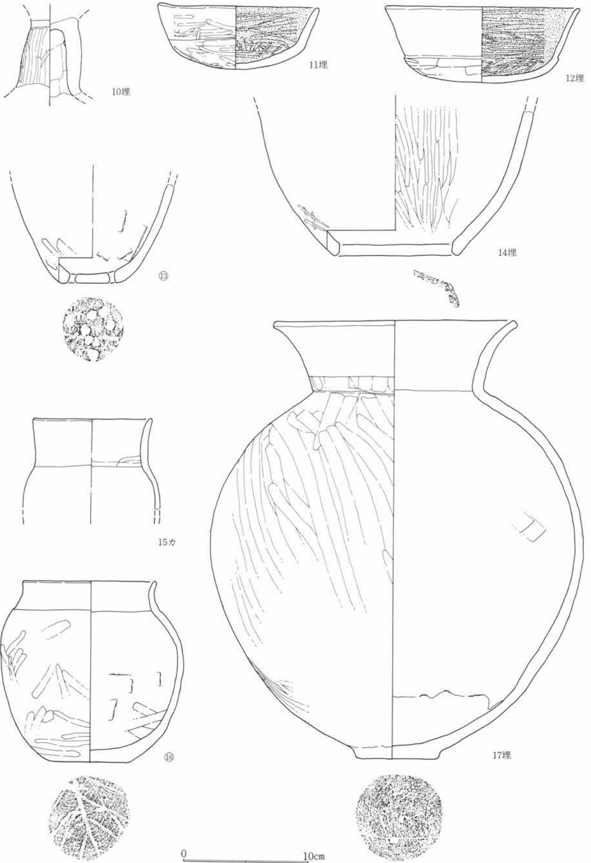
第158図 SJ37出土遺物図 1 : 3
