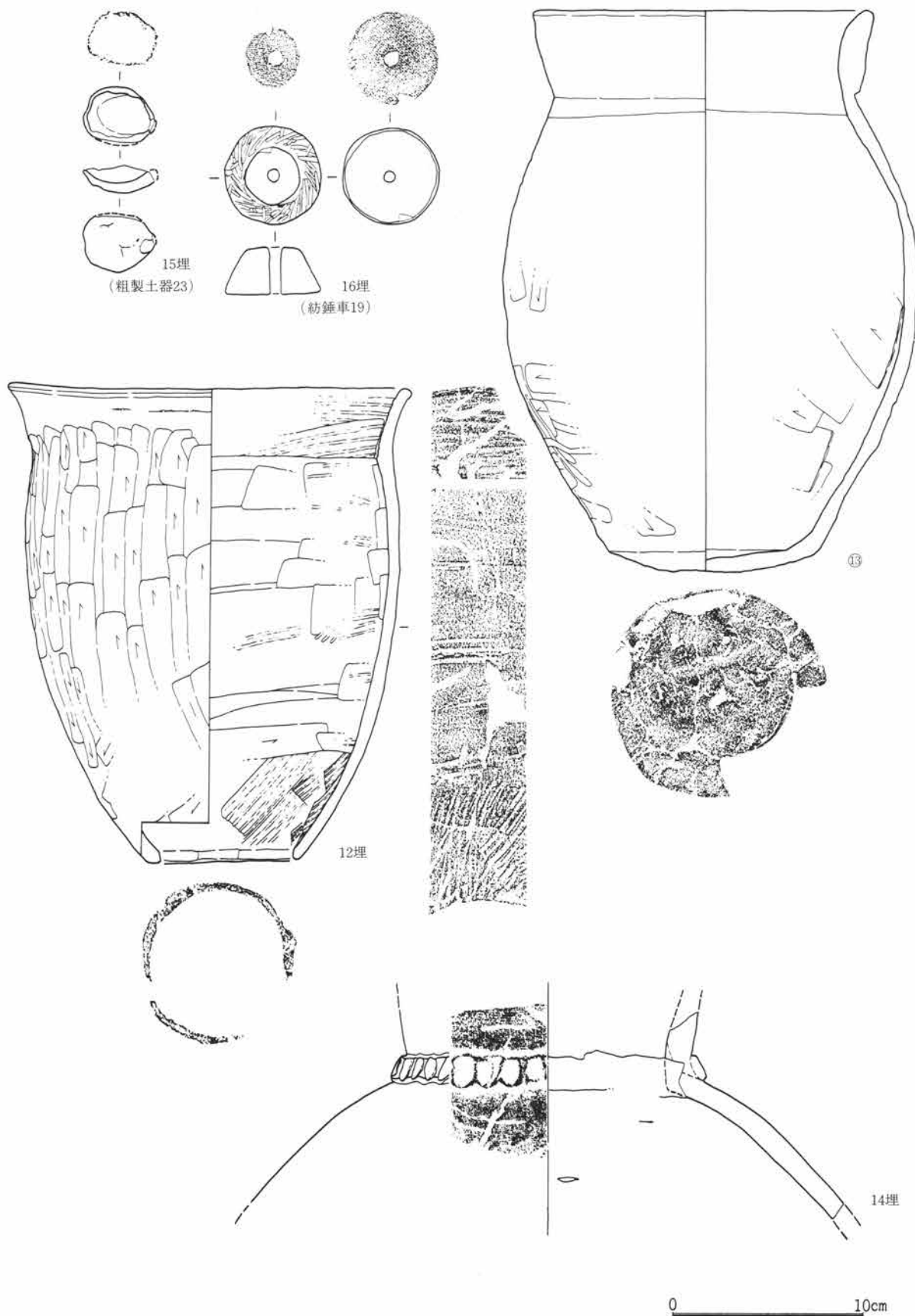
第392図 SJ114出土遺物図 1:3
