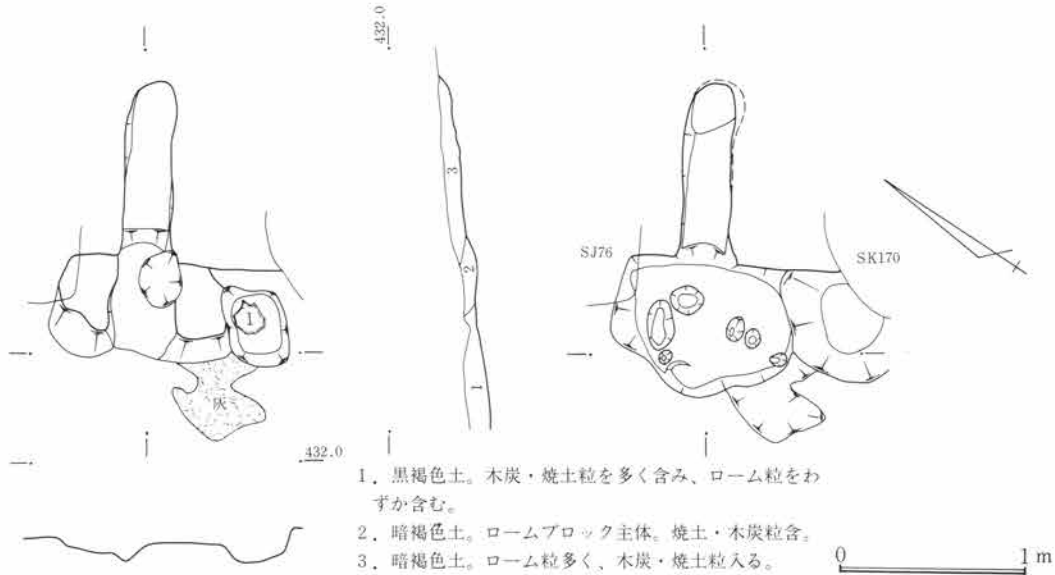
第769図 S J 288-1竈図 1:40
