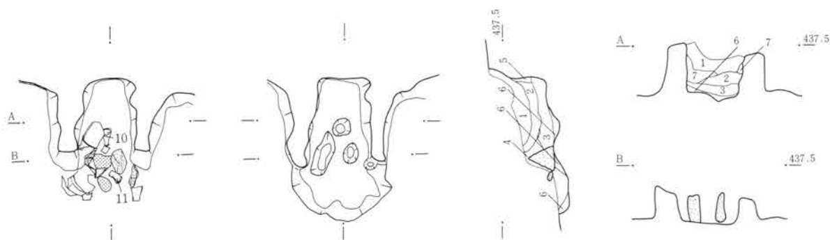
第47図 SJ08遺構図 1:80
