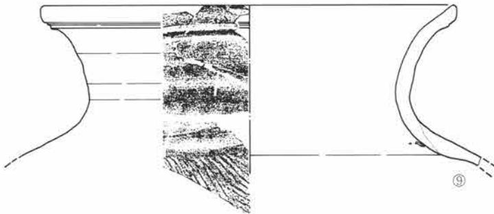
第423図 SJ128出土遺物図 1:3
