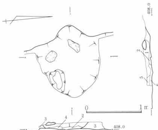
第476図 SJ155竈図 1:40
