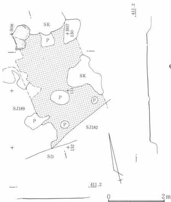
第570図 SJ193遺構図 1:80
