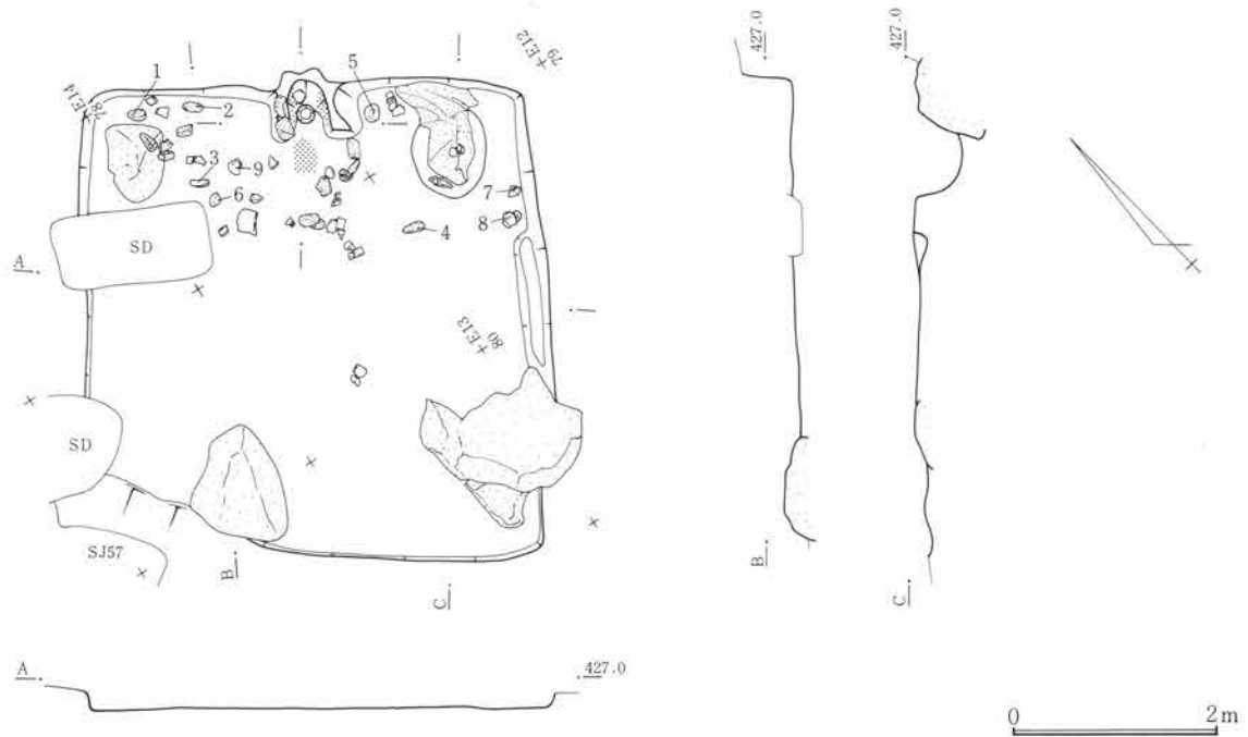
第224図 SJ58遺構図 1:80
