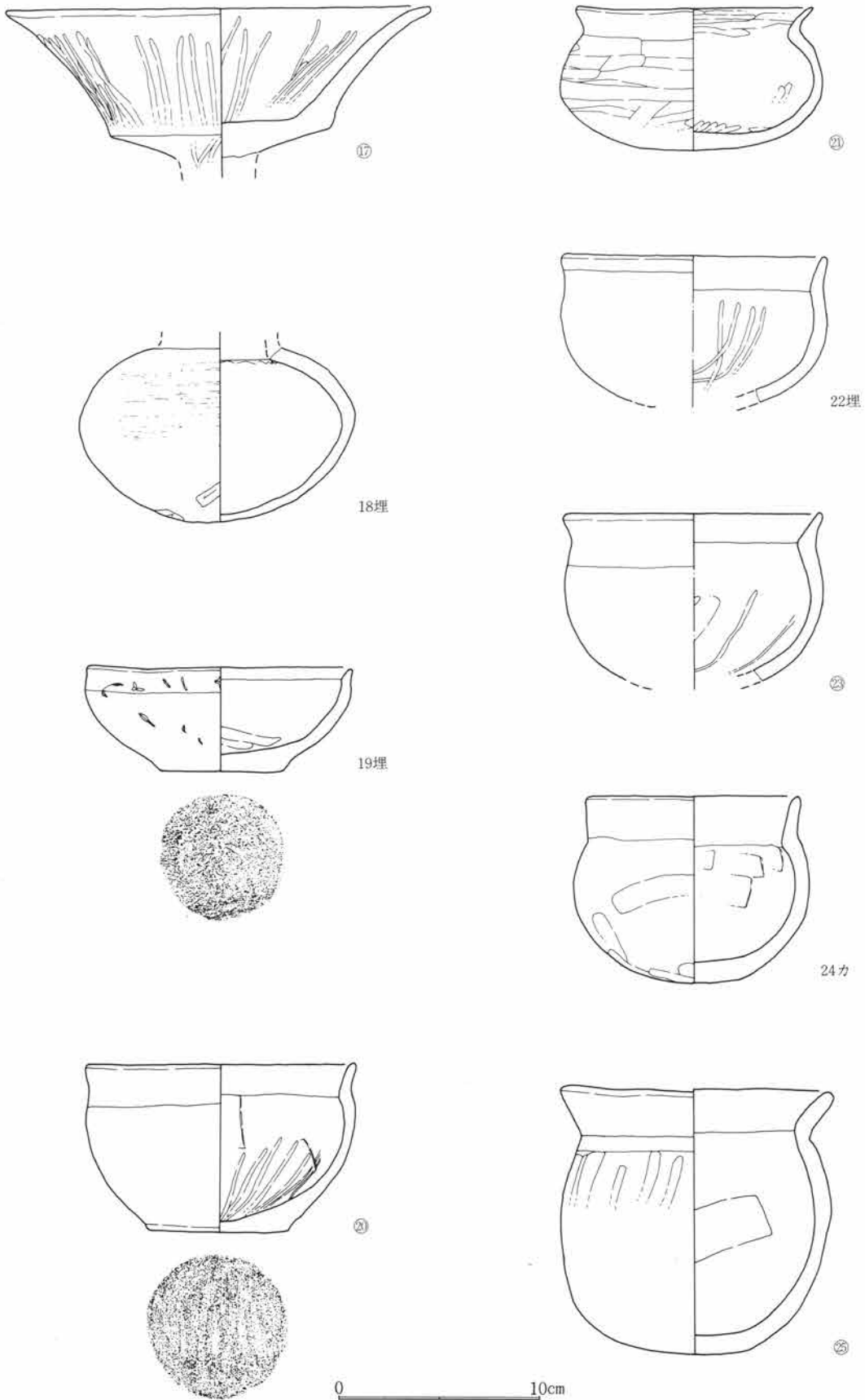
第78図 SJ14出土遺物図 1:3
