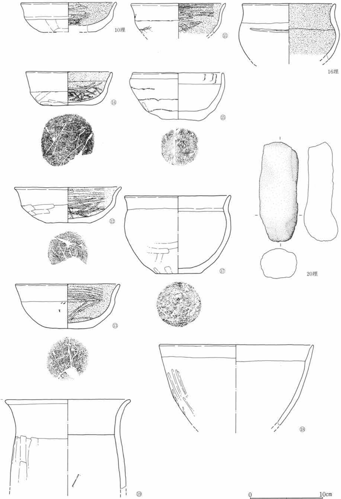
第101図 SJ20出土遺物図 1 : 3
