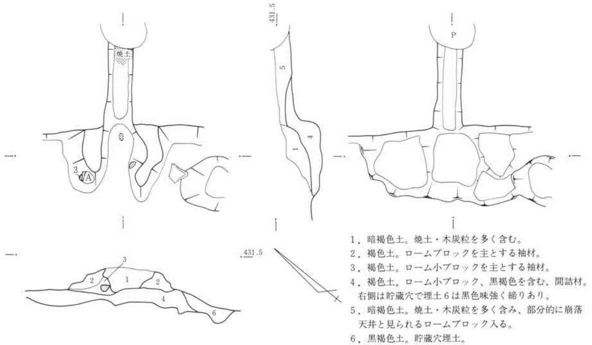
第276図 SJ75竈図 1:40
