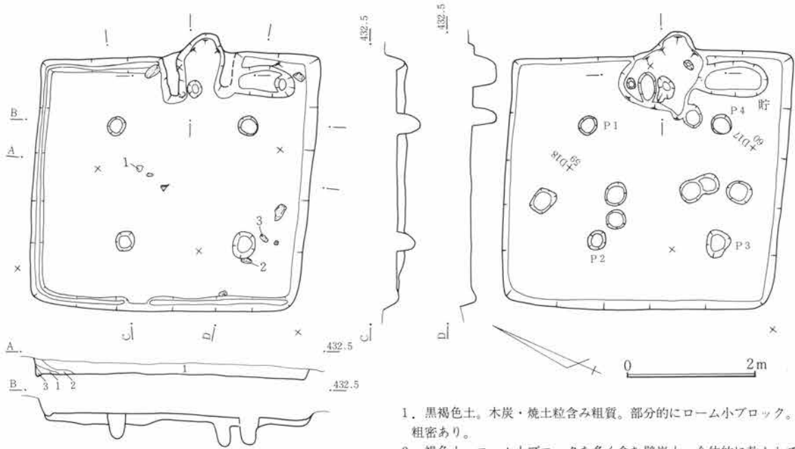
第411図 SJ124遺構図 1:80
