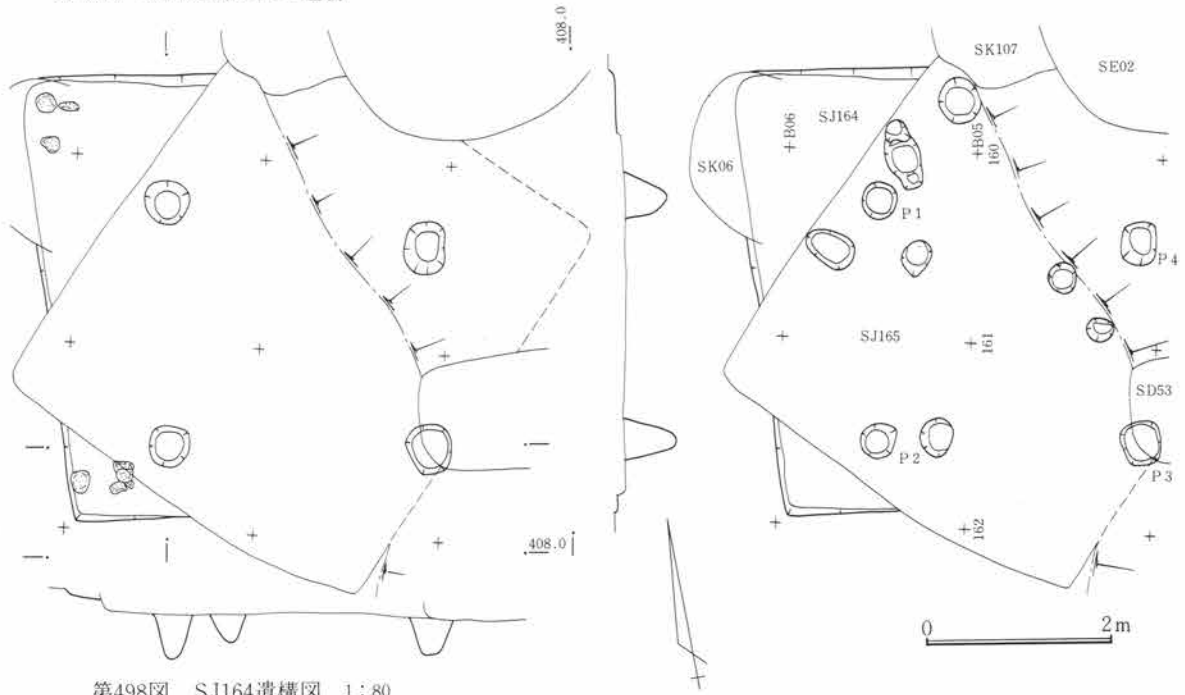
第498図 SJ164遺構図 1:80
