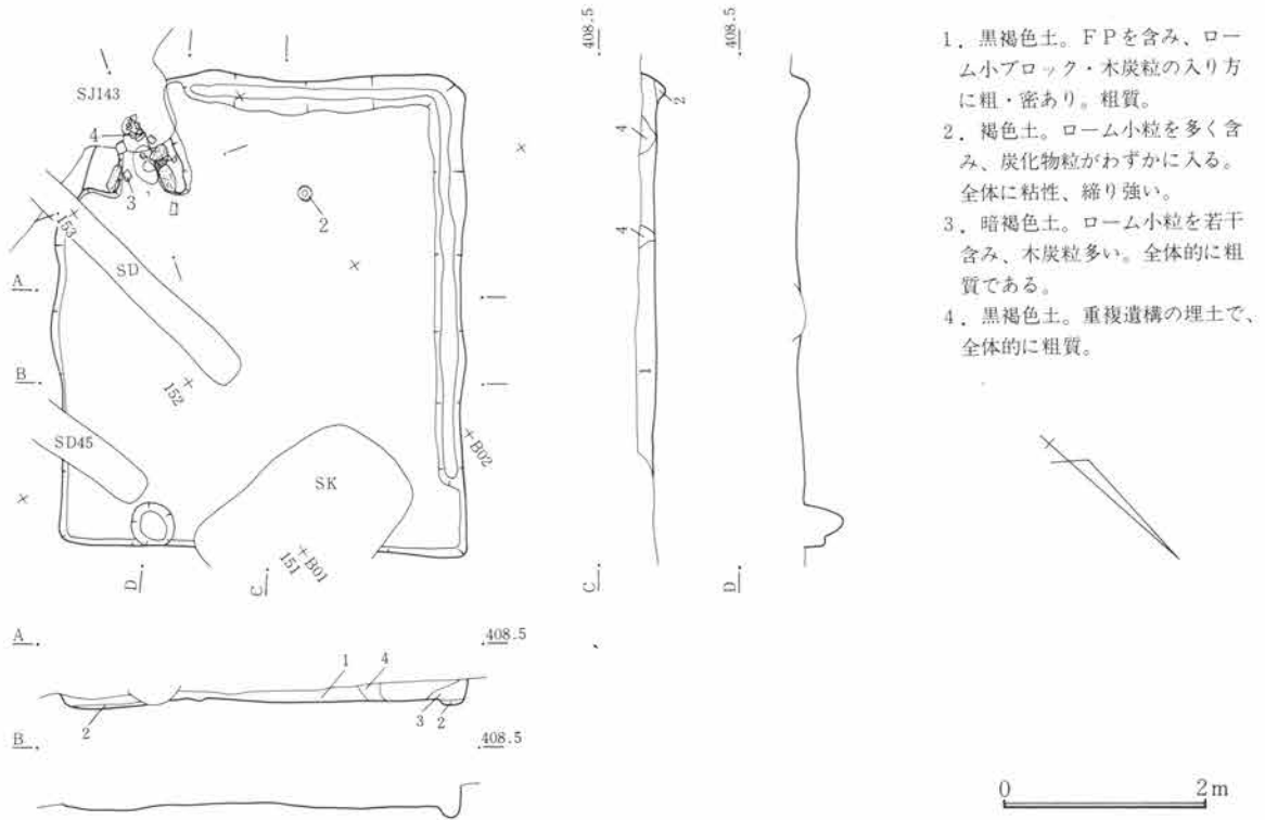
第503図 SJ167遺構図 1:80
