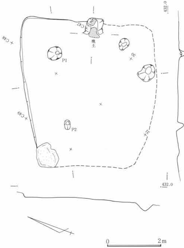
第679図 SJ248遺構図 1:80
