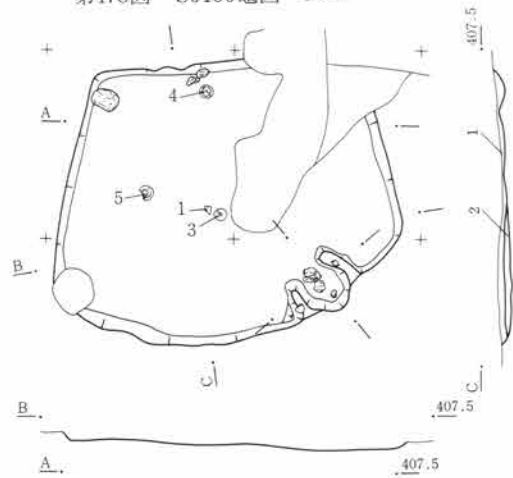
第478図 SJ156竈図 1:40
