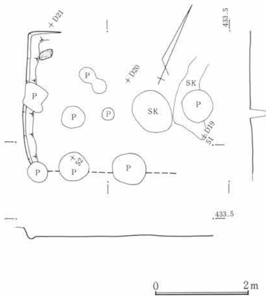
第628図 SJ228遺構図 1:80
