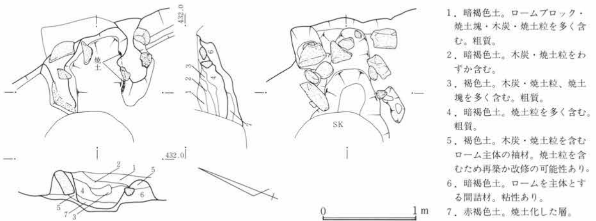
第372図 SJ108竈図 1:40
