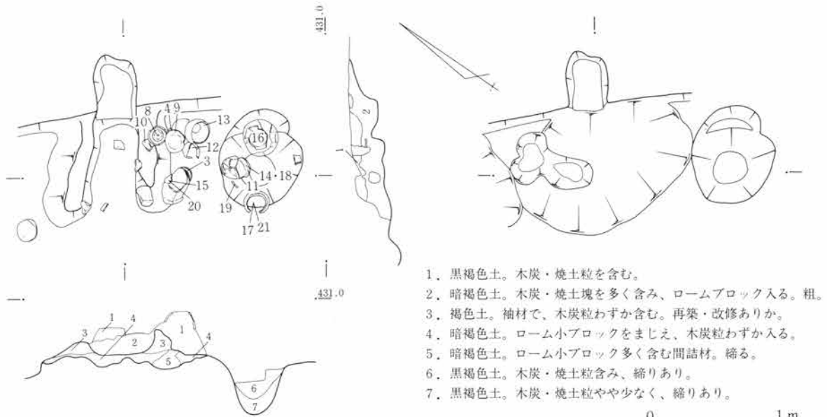
第630図 SJ231竈図 1:40
