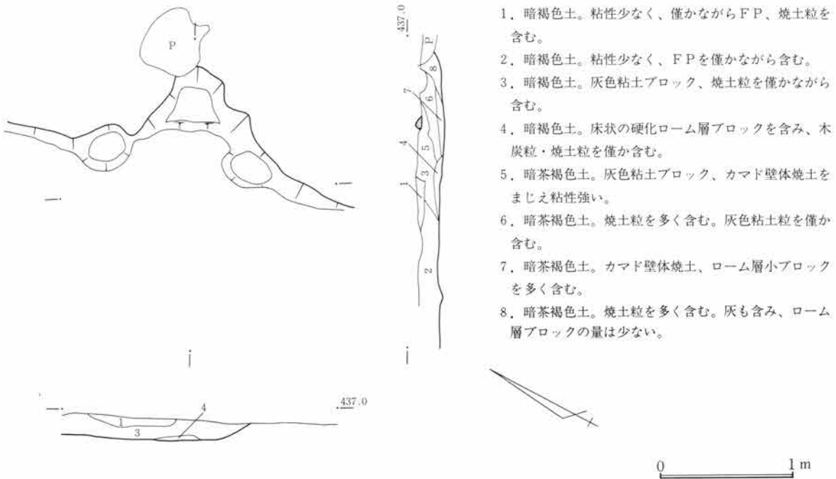
第85図 SJ17竈図 1:40
