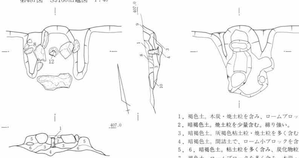
第488図 SJ160竈図 1:40
