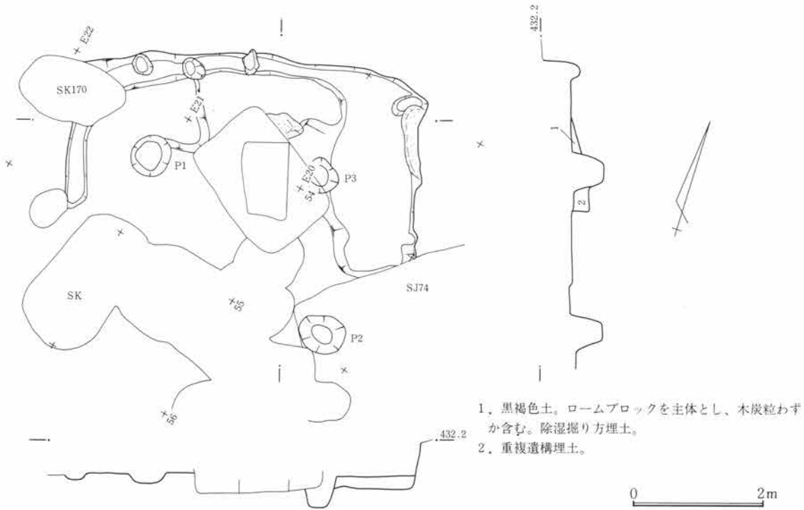
第773図 SJ289-1遺構図 1:80
