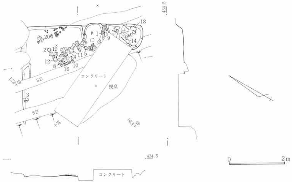
第310図 SJ86遺構図 1:80
