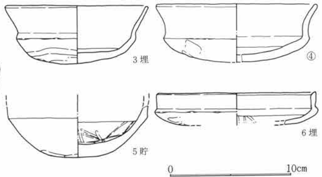
第388図 SJ113出土遺物図 1 : 3
