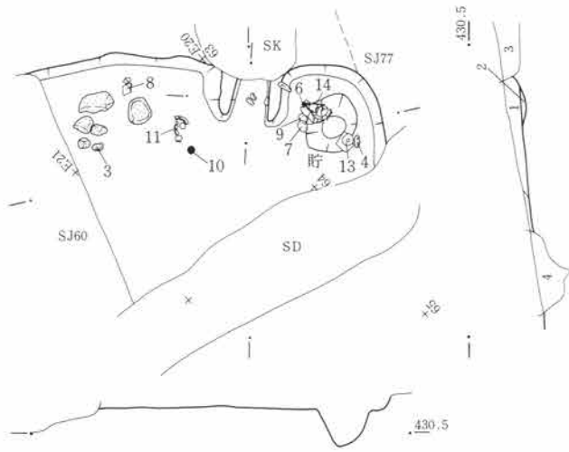
第332図 SJ93遺構図 1:80
