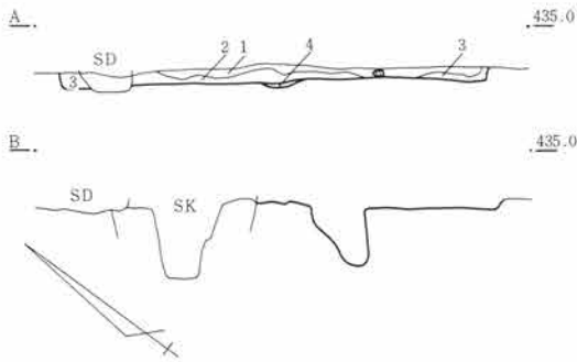
第186図 SJ48遺構図 1:80
