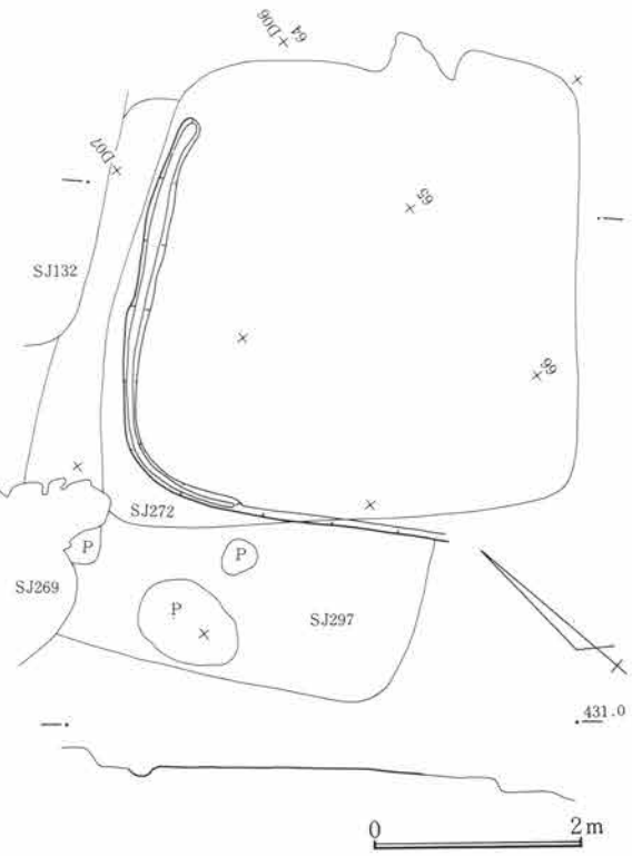
第795図 SJ301遺構図 1:80
