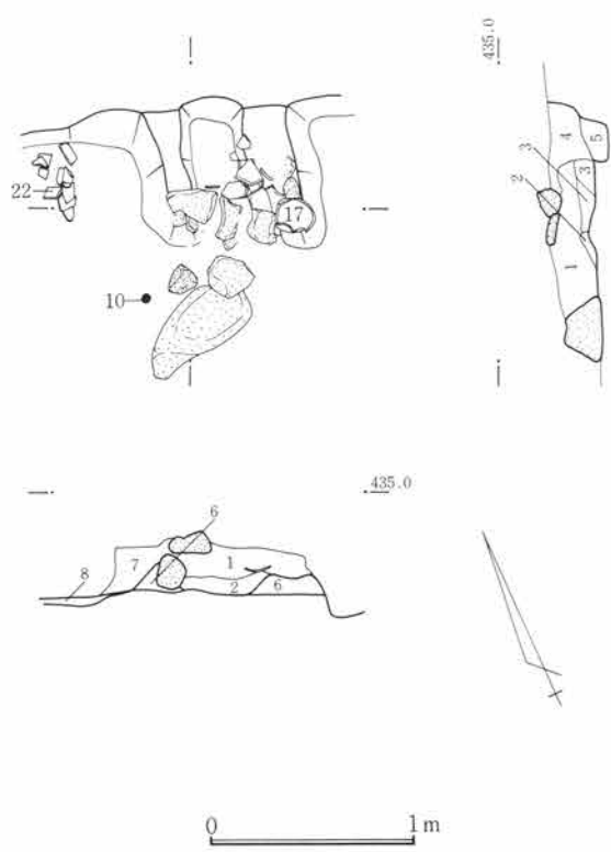
第305図 SJ85竈図 1:40
