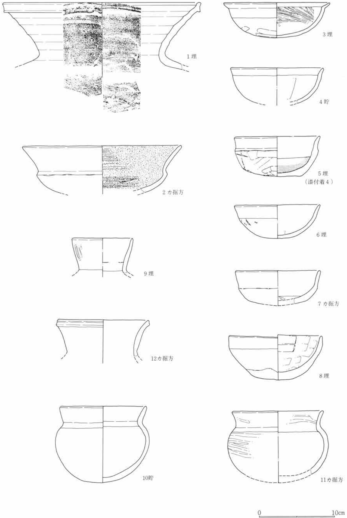
第382図 SJ111出土遺物図 1 : 3
