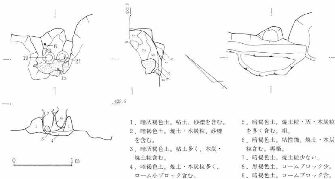
第155図 SJ37竈図 1:40
