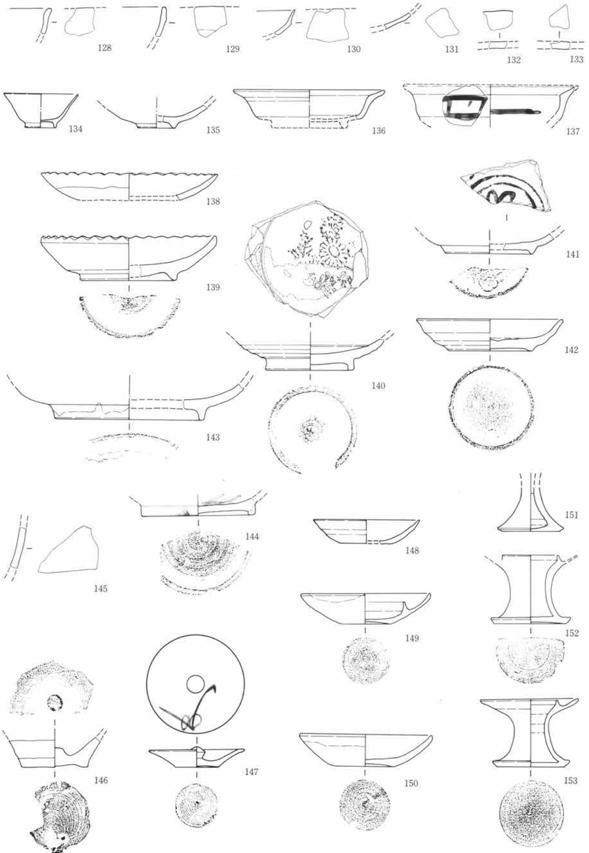
第920図 近世陶・磁器 1 : 3
