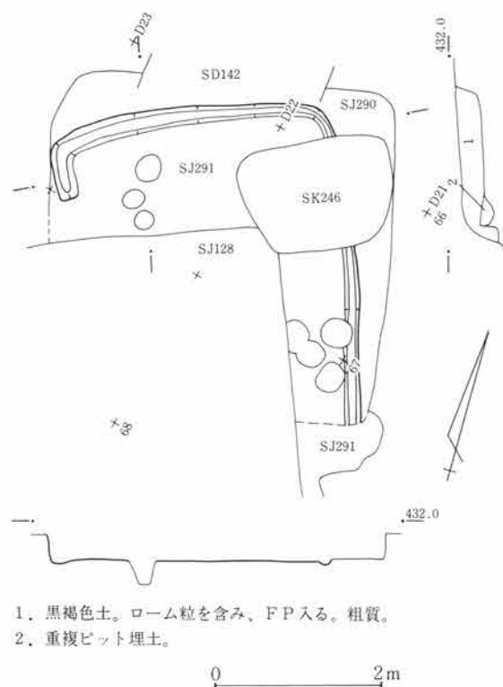
第586図 SJ204遺構図 1:80
