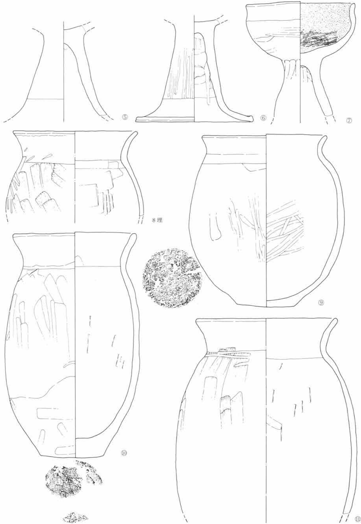
第289図 SJ80出土遺物図 1:3
