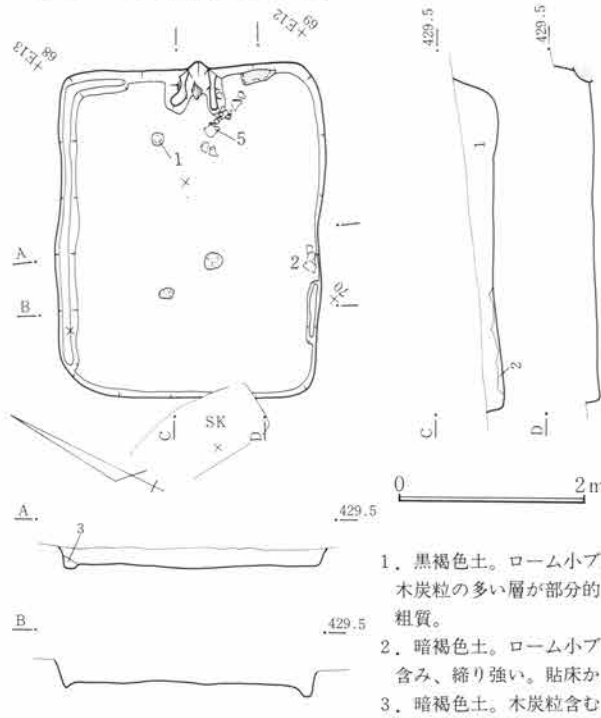
第290図 SJ81遺構図 1:80
