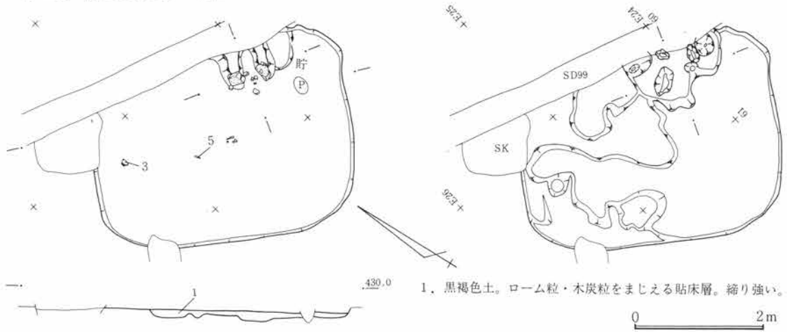
第619図 SJ224遺構図 1:80
