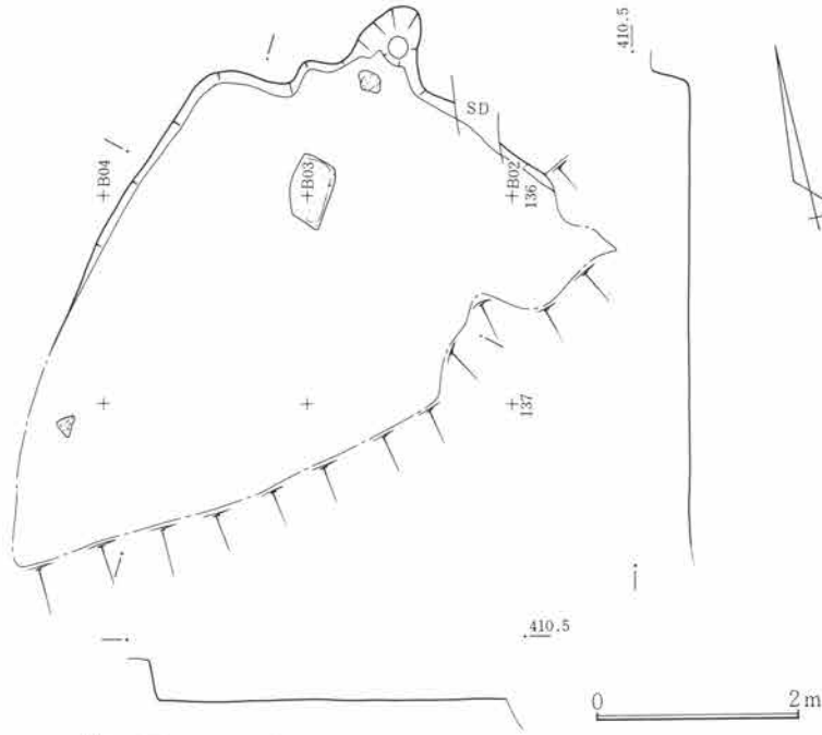
第566図 SJ190遺構図 1:80
