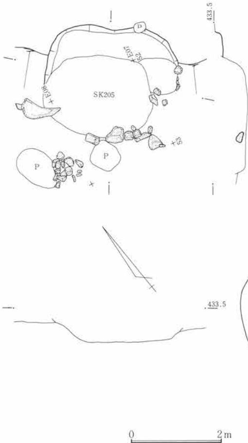
第684図 SJ251遺構図 1:80
