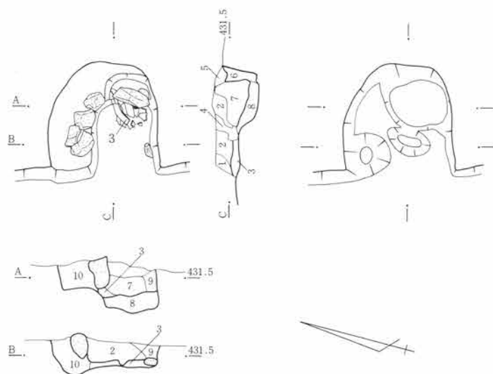
第426図 SJ129竈図 1:40
