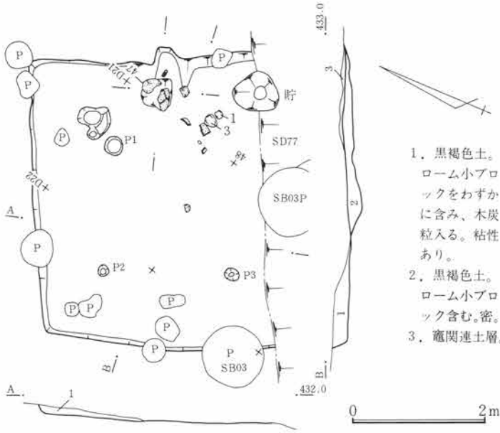
第575図 SJ196遺構図 1:80
