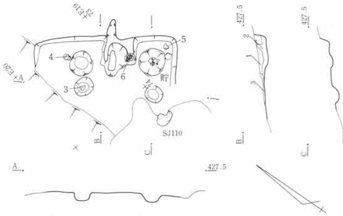
第375図 SJ109遺構図 1:80
