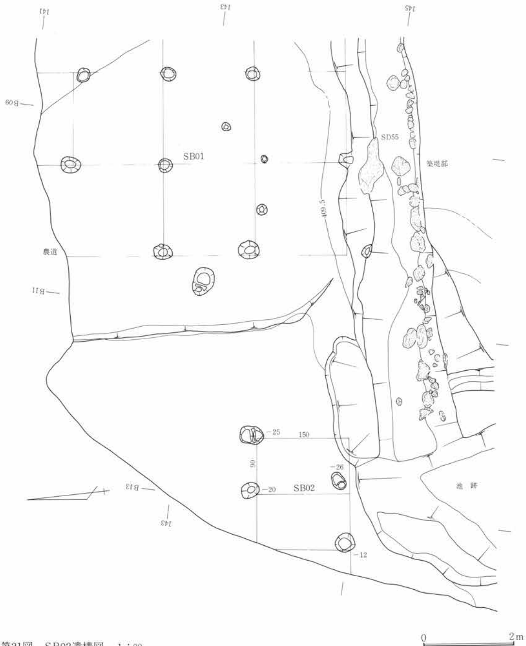
第21図 SB02遺構図 1:80
