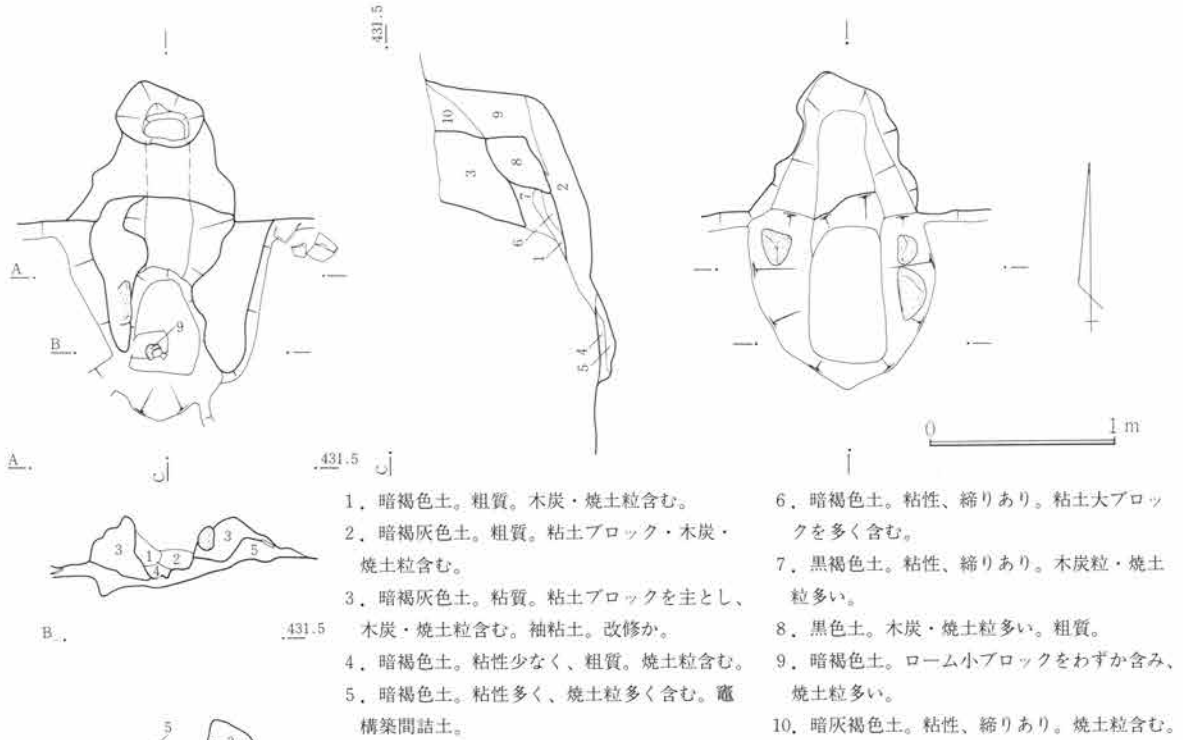
第134図 SJ32竈図 1:40
