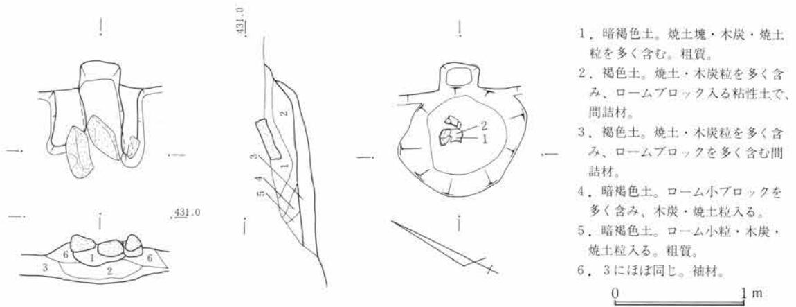
第658図 SJ239竈図 1:40
