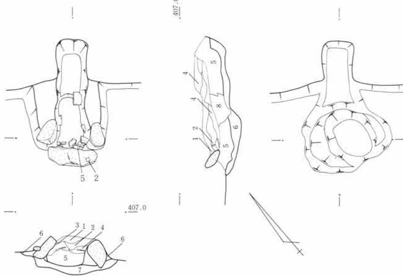
第506図 SJ168遺構図 1:80
