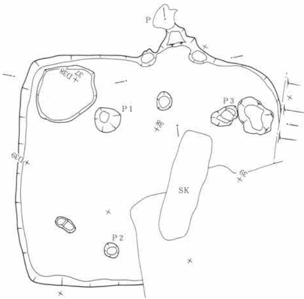
第86図 SJ17遺構図 1:80
