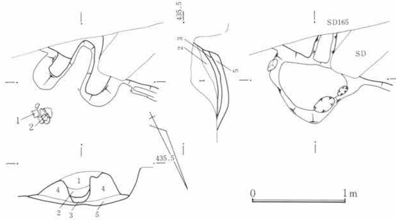
第801図 SJ303竈図 1:40
