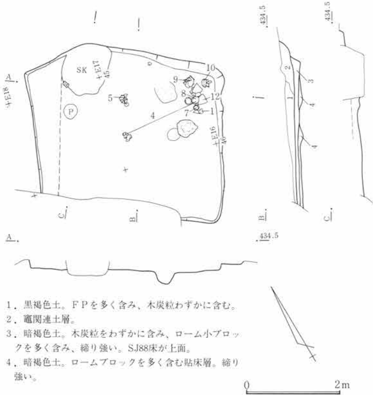
第840図 SJ324遺構図 1:80
