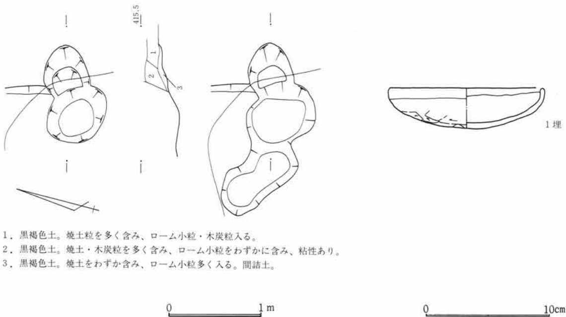
第594図 SJ212出土遺物図 1:3
