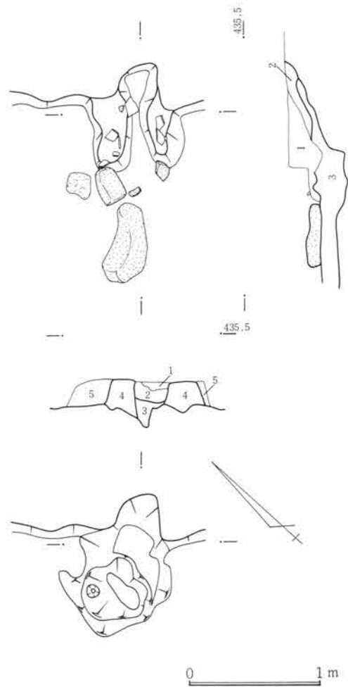
第237図 SJ61竈図 1:40
