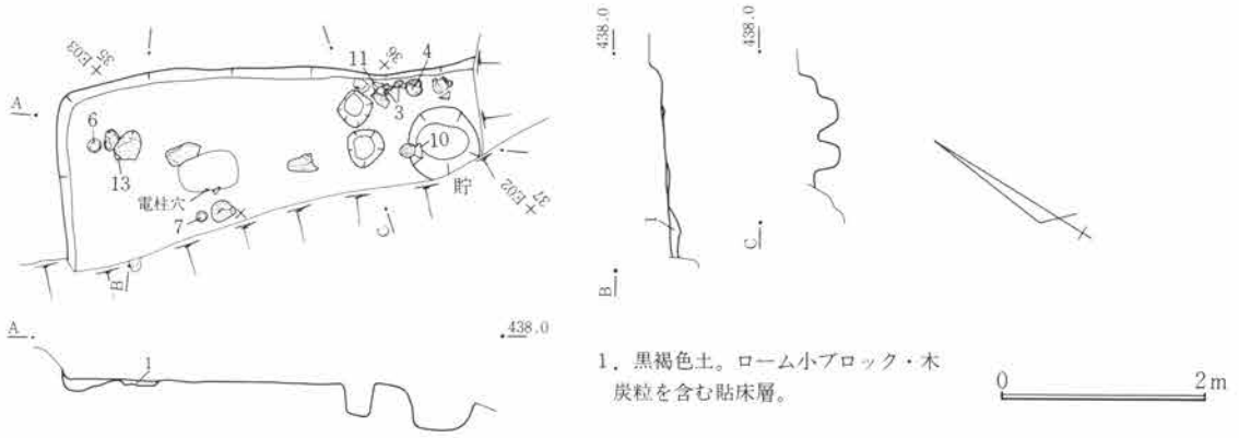
第390図 SJ114遺構図 1:80
