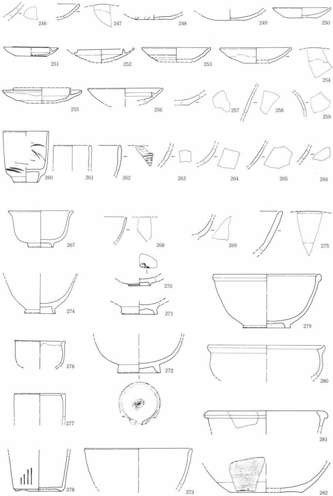
第926図 近世陶・磁器 1 : 3
