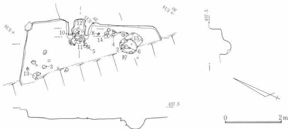
第47図 SJ08遺構図 1:80
