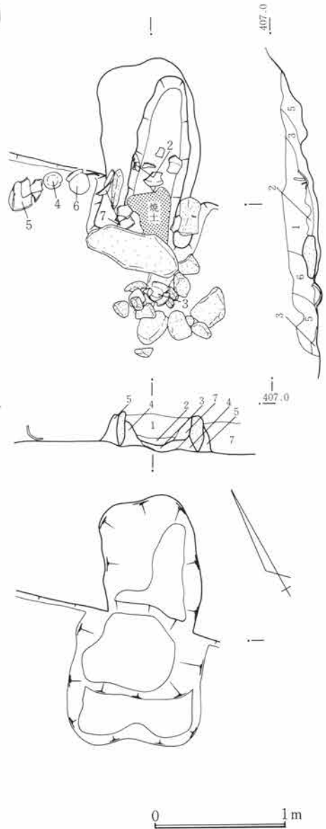
第461図 SJ145竈図 1:40
