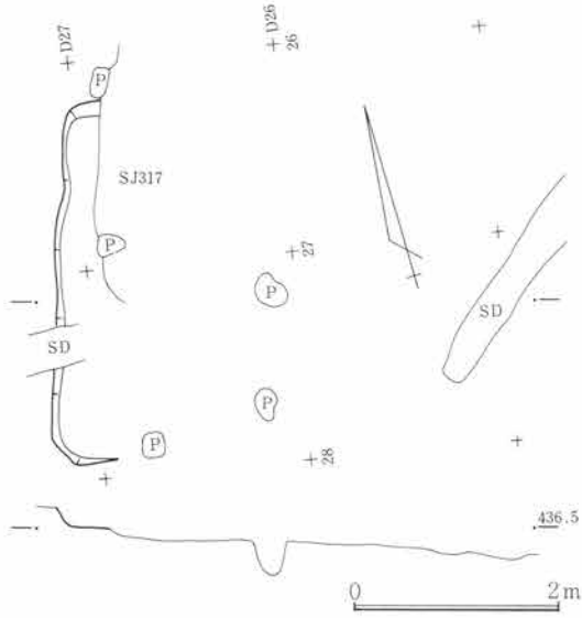
第828図 SJ316遺構図 1:80
