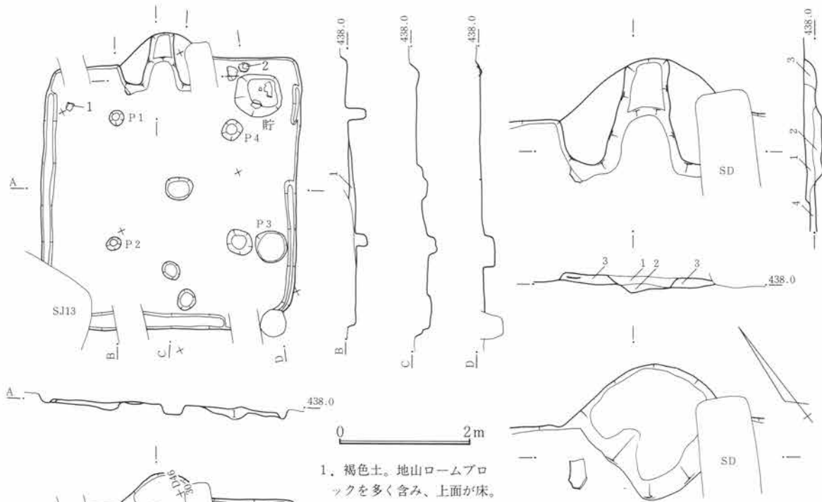
第162図 SJ38竈図 1:40
