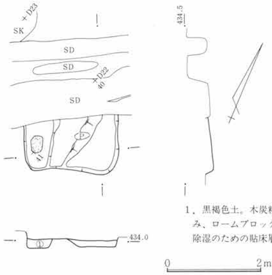
第830図 SJ318遺構図 1:80
