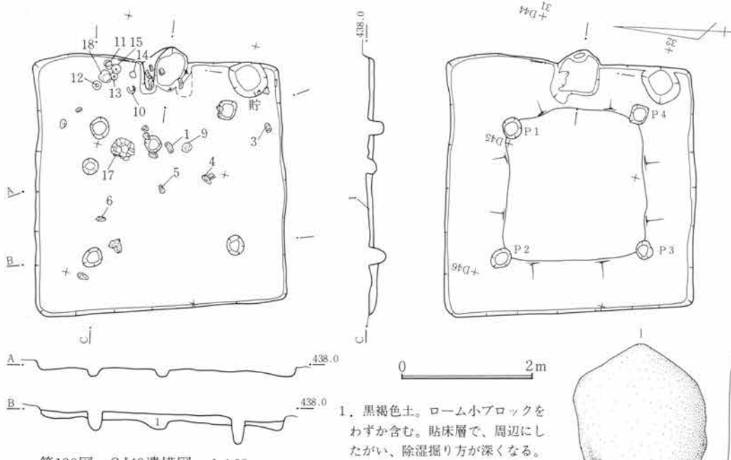
第190図 SJ49遺構図 1:80
