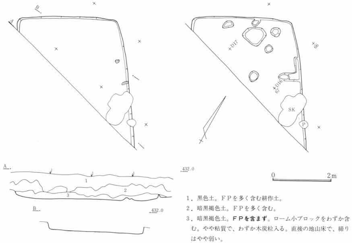
第428図 SJ130遺構図 1:80
