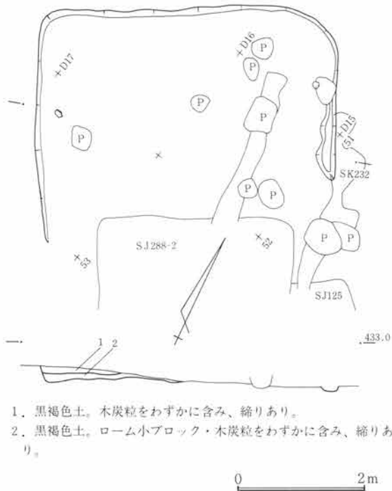
第767図 SJ287遺構図 1:80
