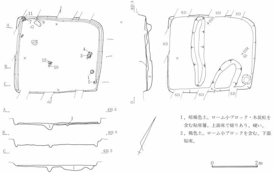
第401図 SJ121遺構図 1 : 80
