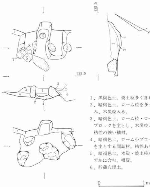
第816図 SJ307竈図 1:40
