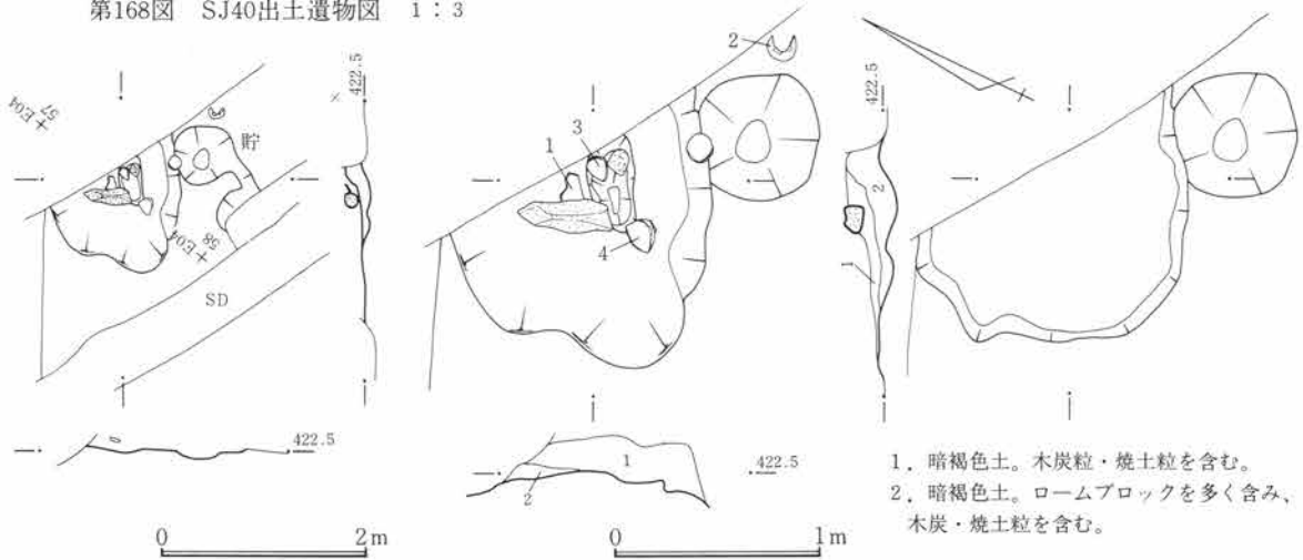
第169図 SJ41遺構図 1:80
