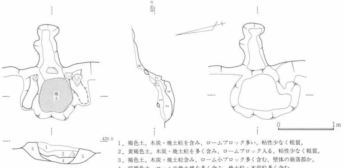
第209図 SJ54竈図 1 : 40
