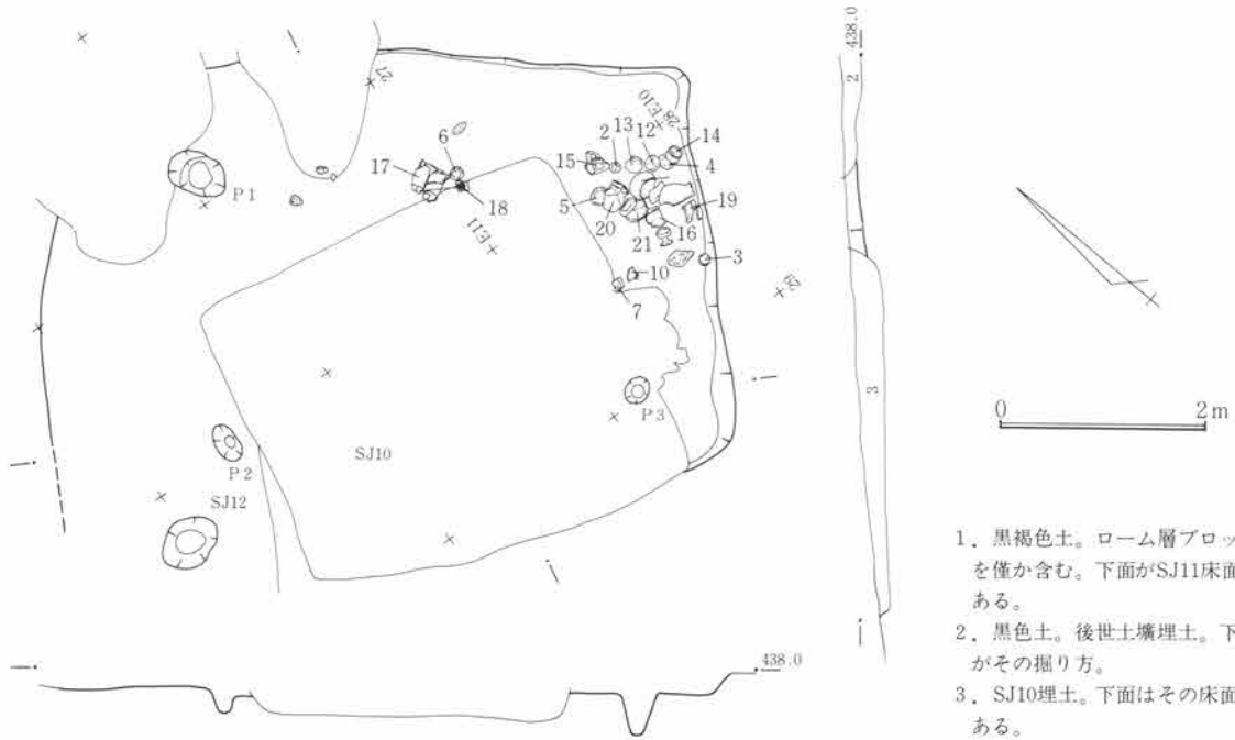
第60図 SJ11遺構図 1:80
