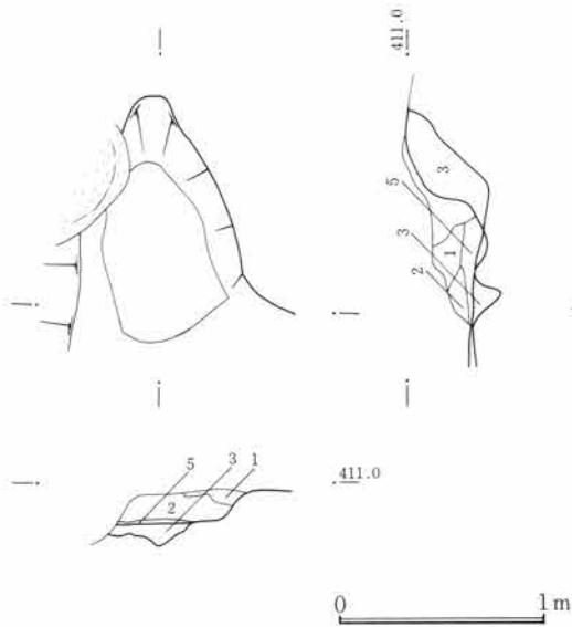
第536図 SJ178竈図 1:40
