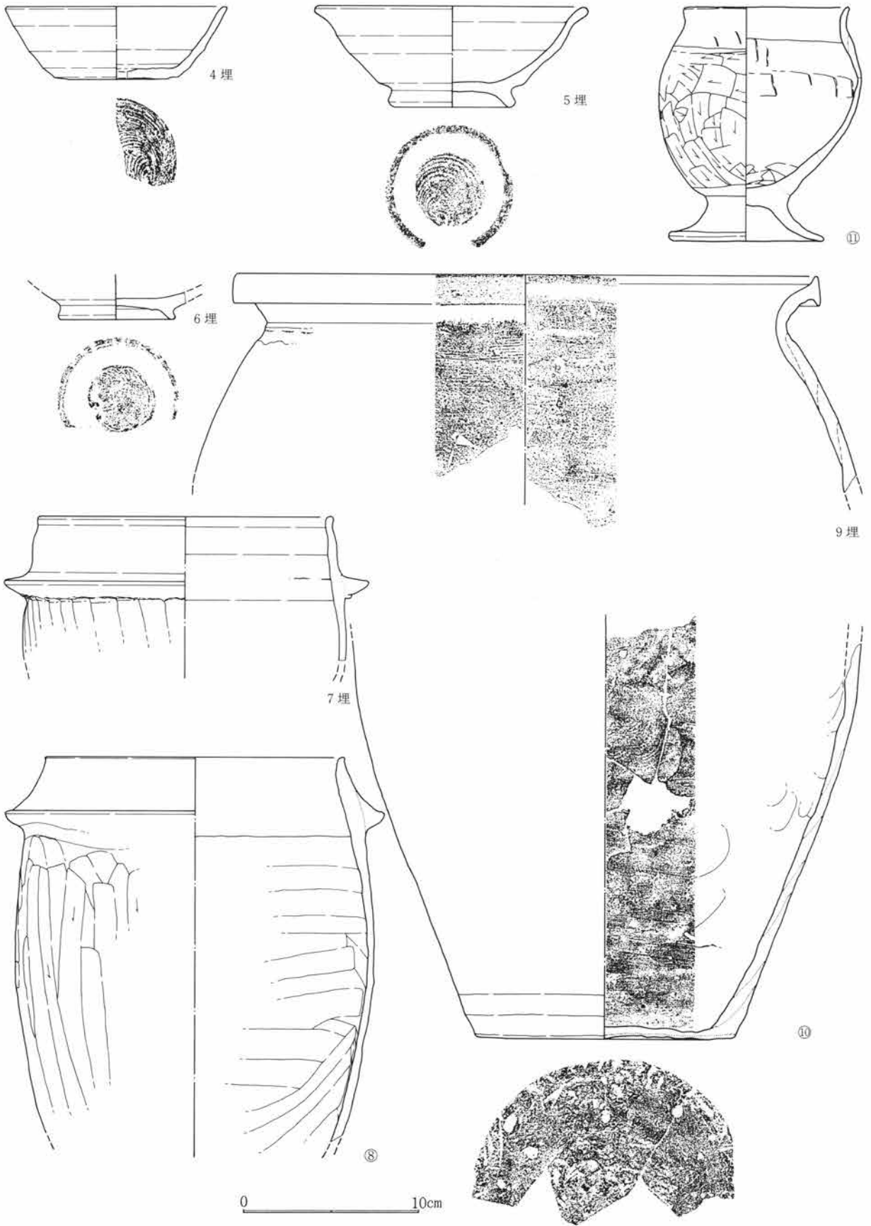
第652図 SJ236出土遺物図 1:3
