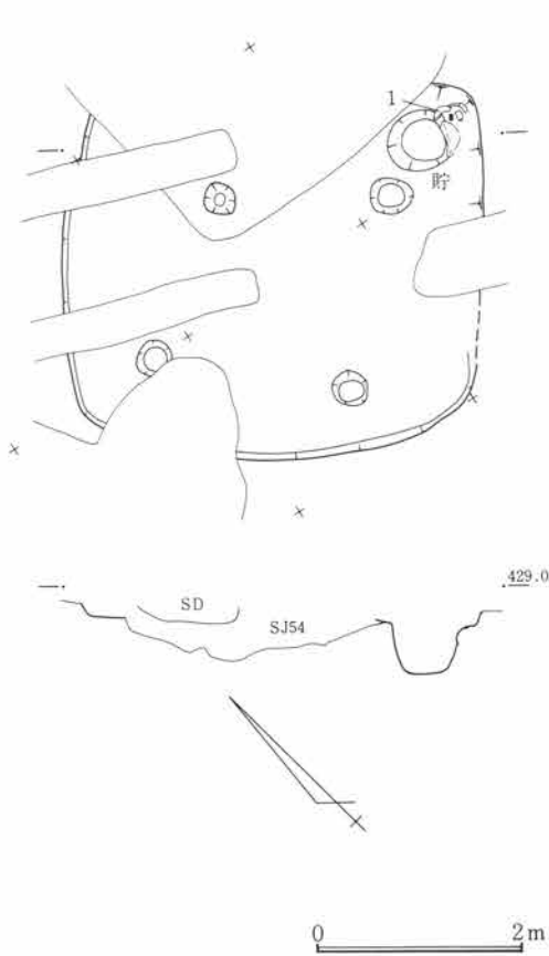
第668図 SJ243遺構図 1:80
