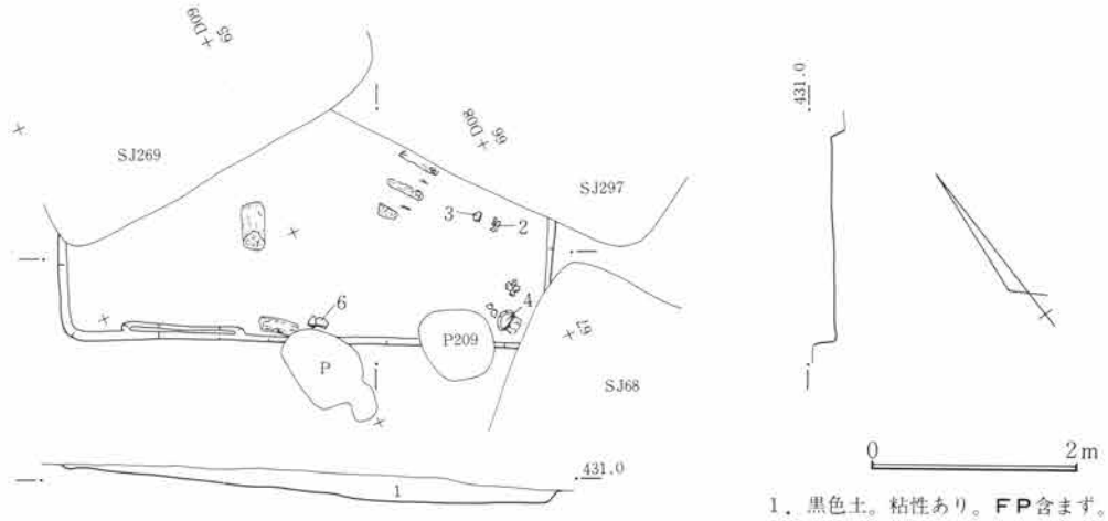
第785図 SJ296遺構図 1:80
