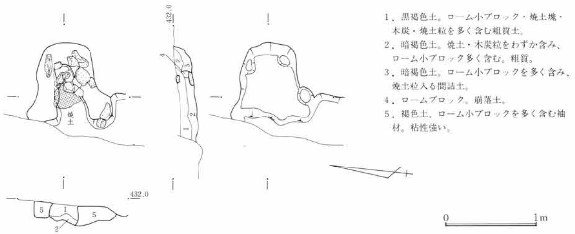
第691図 SJ257竈図 1:40
