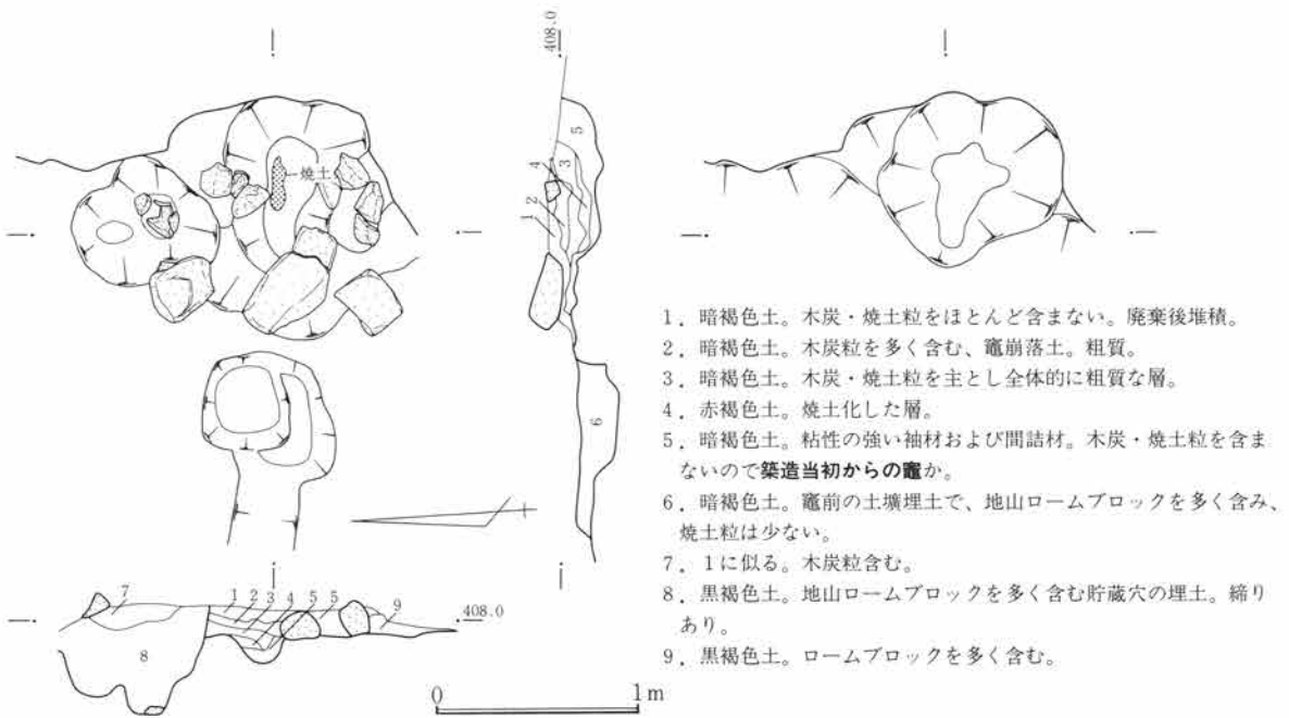
第465図 SJ148竈図 1:40
