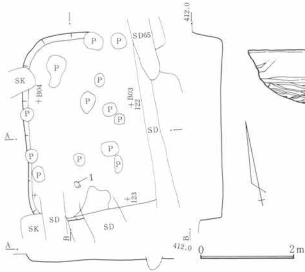
第513図 SJ171遺構図 1:80
