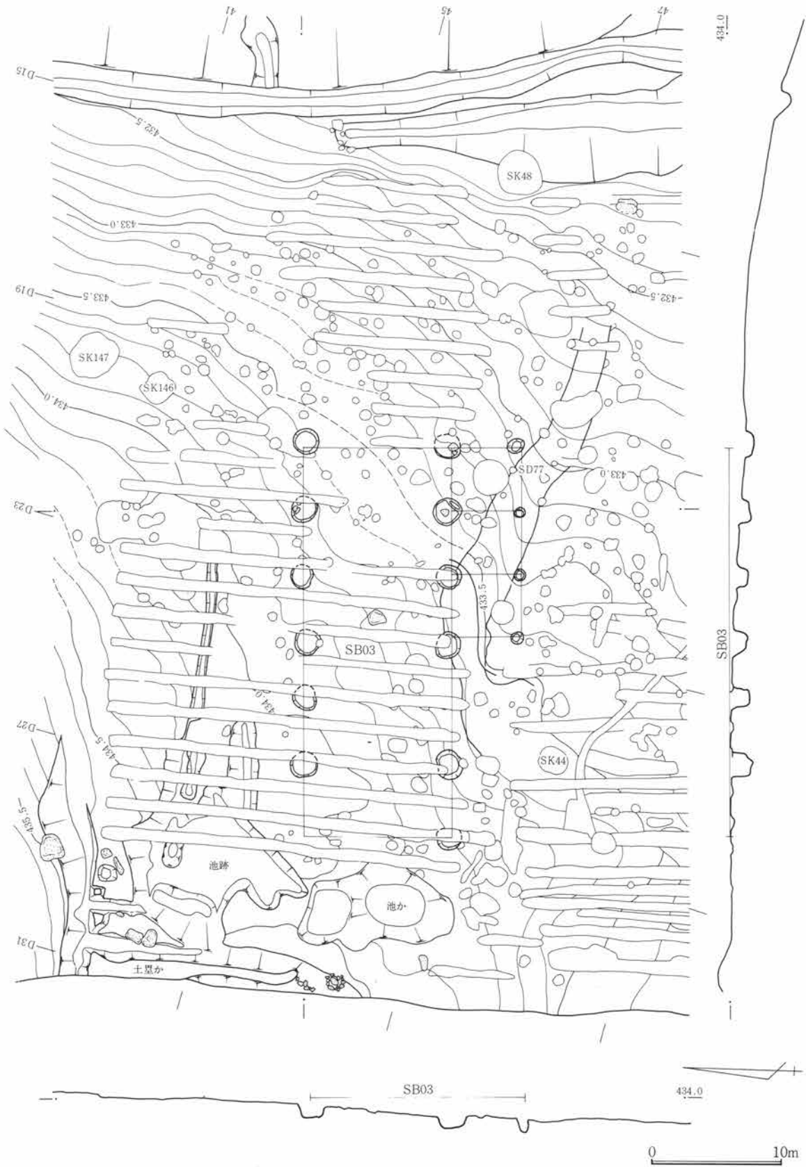
第22図 SB03と周辺遺構図 1:200
