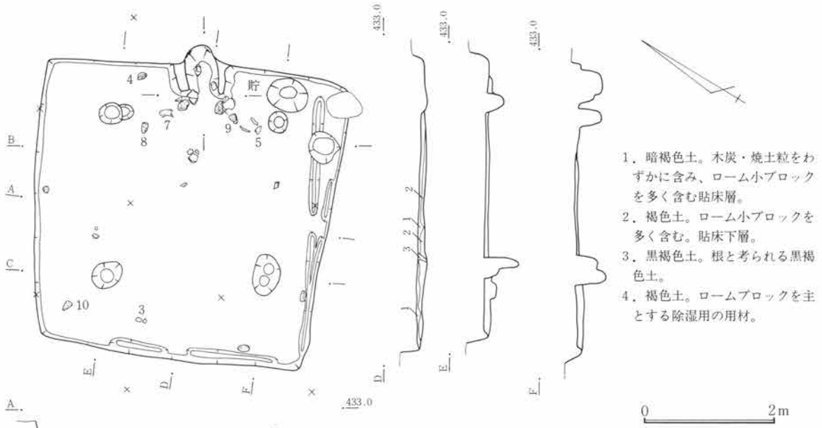
第404図 SJ122遺構図 1 : 80
