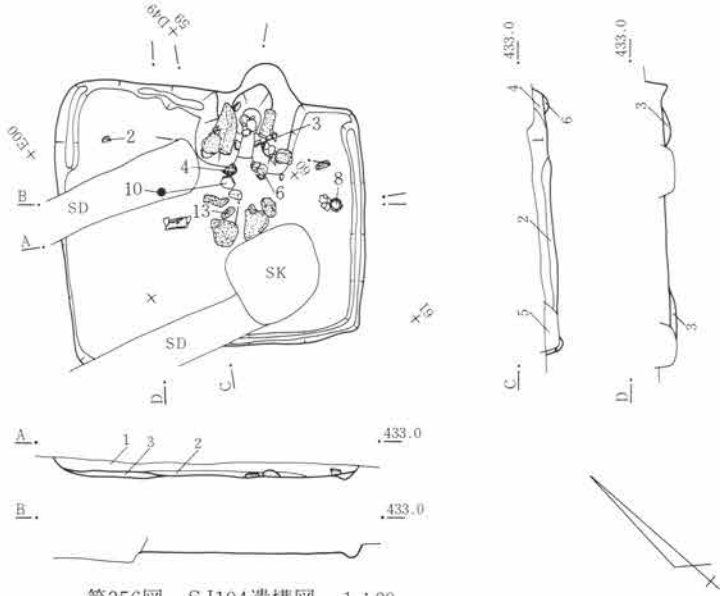
第356図 SJ104遺構図 1:80
