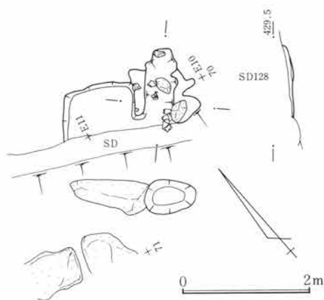
第670図 SJ244遺構図 1:80
