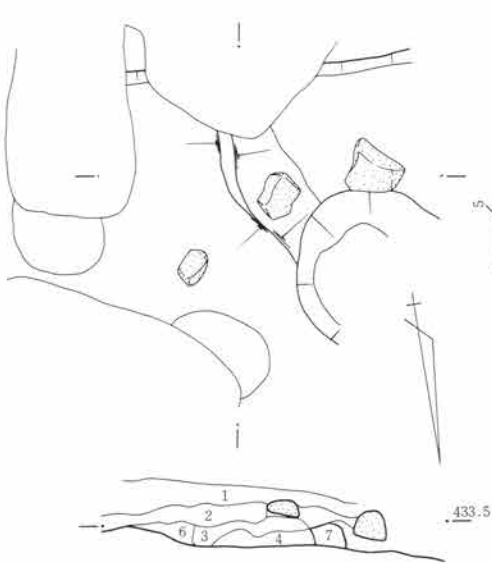
第176図 SJ43竈図 1:40
