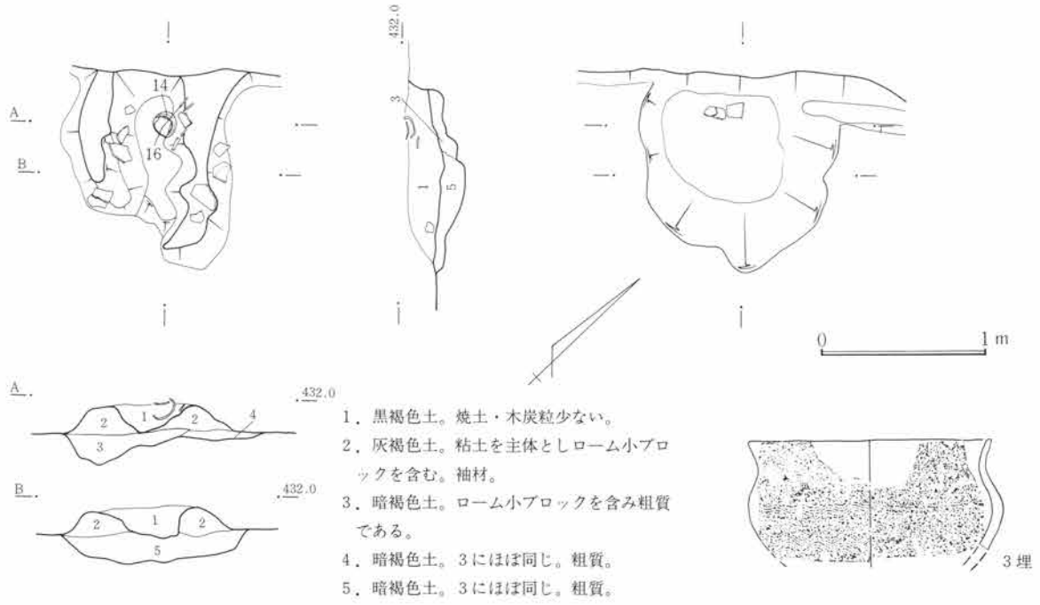
第150図 SJ36竈図 1:40
