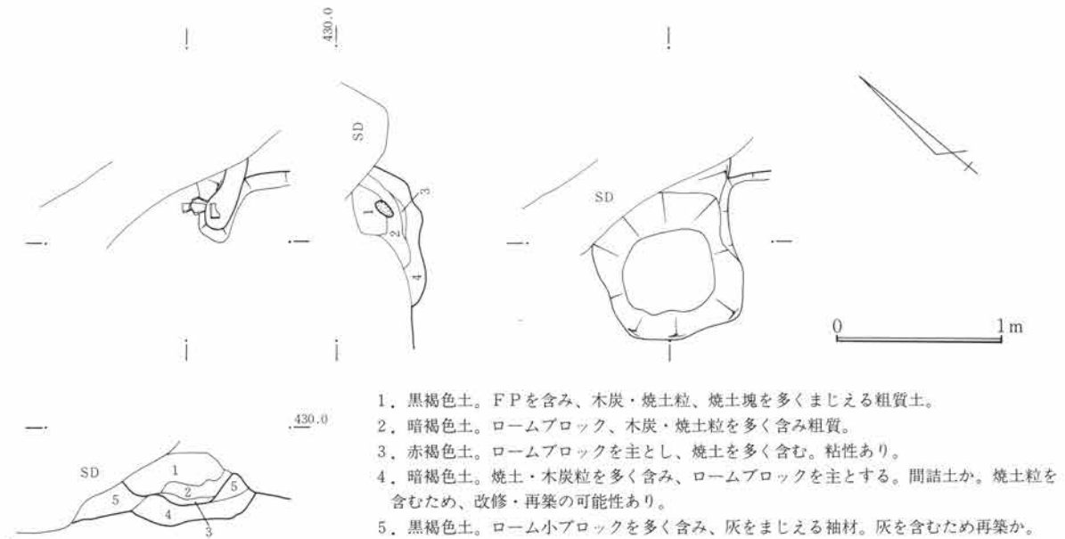
第316図 SJ87竈図 1:40
