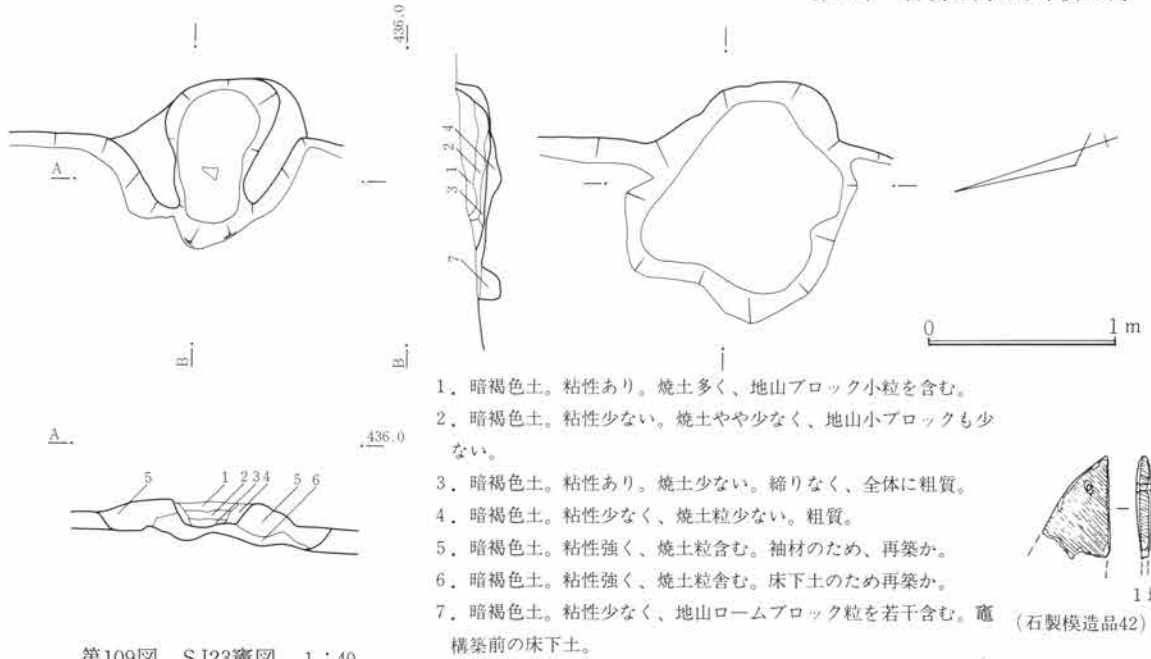
第109図 SJ23竈図 1:40
