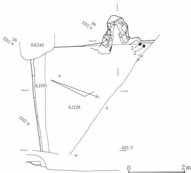
第777図 SJ291遺構図 1:80
