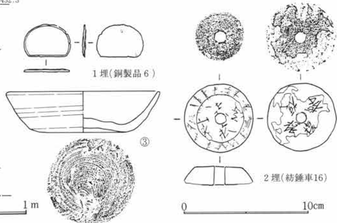
第285図 SJ79出土遺物図 1:3
