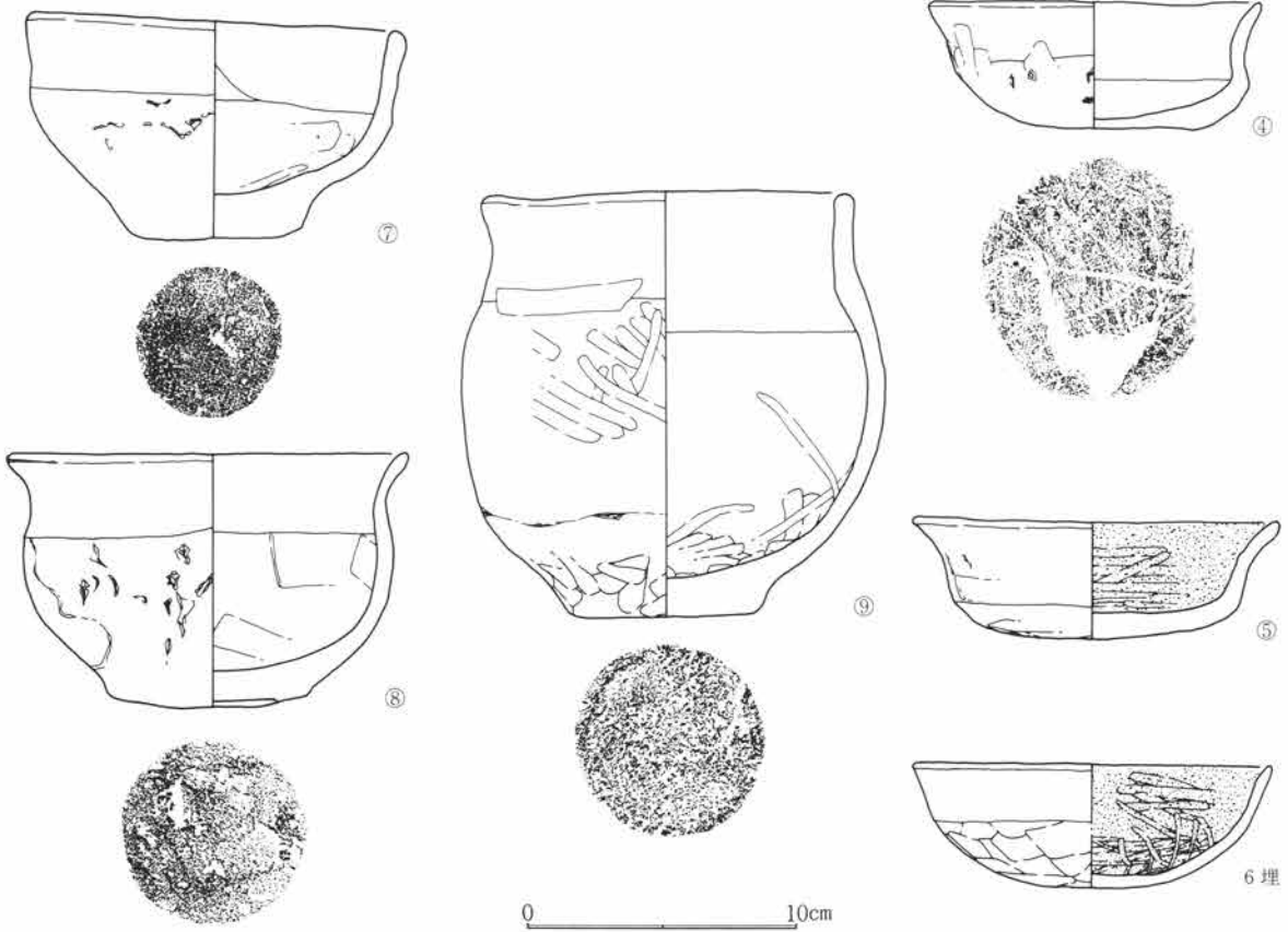
第841図 SJ324出土遺物図 1:3
