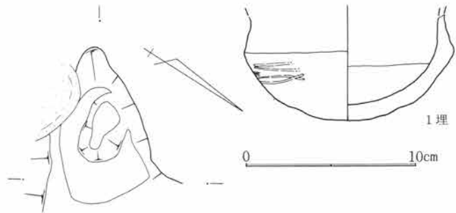
第537図 SJ178出土遺物図 1:3
