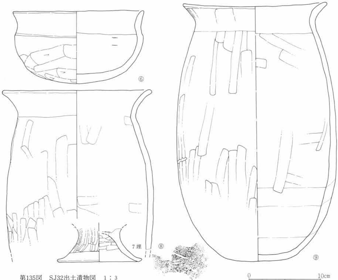
第135図 SJ32出土遺物図 1:3
