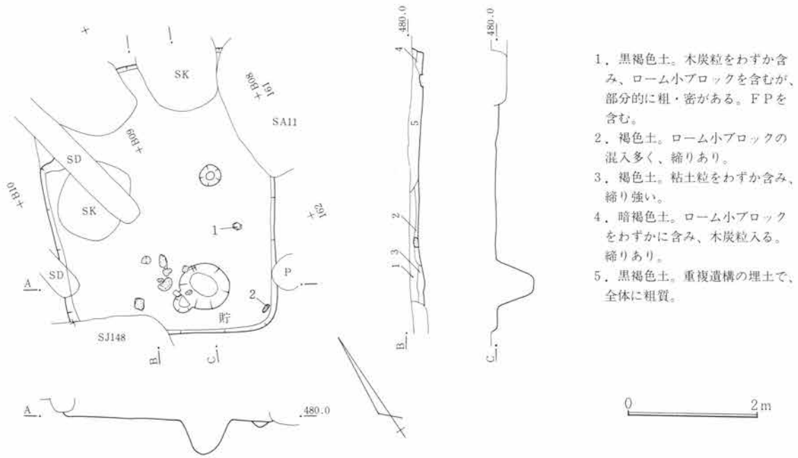
第496図 SJ163遺構図 1:80
