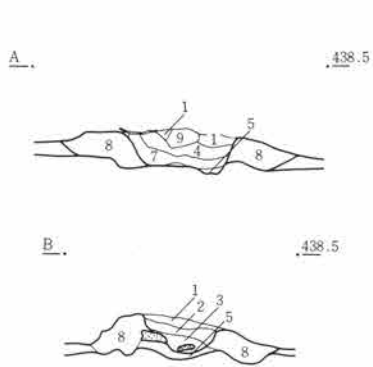
第89図 SJ18竈図 1 : 40
