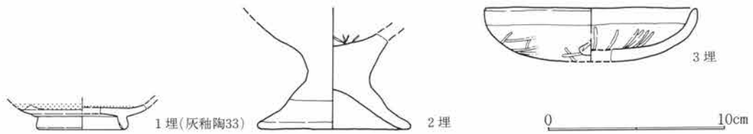
第75図 SJ14出土遺物図 1:3
