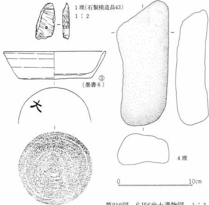
第218図 SJ56出土遺物図 1:3
