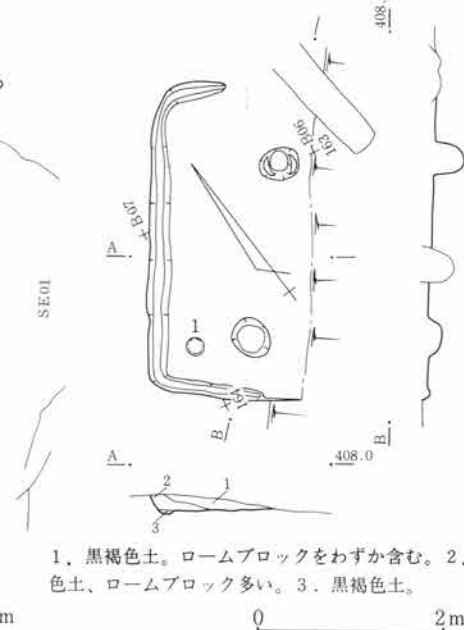
第446図 SJ137遺構図 1 : 80
