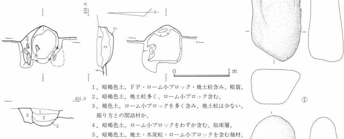
第191図 SJ49竈図 1:40
