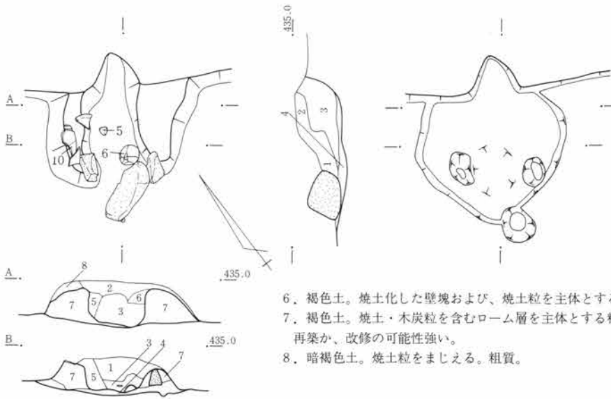
第297図 SJ83竈図 1:40
