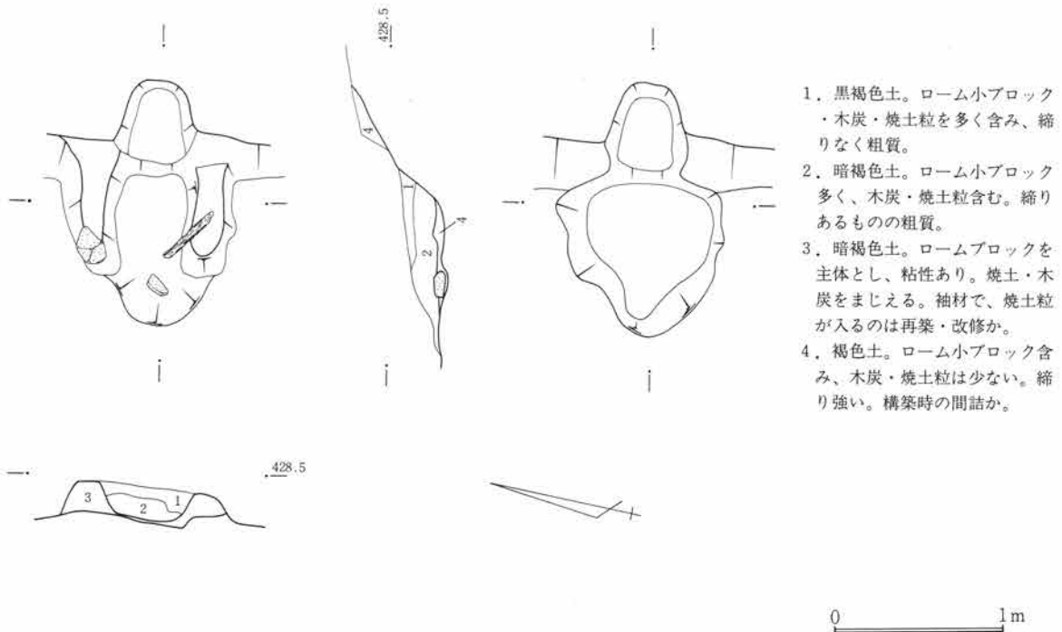
第206図 SJ53竈図 1:40
