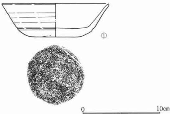
第574図 S J 195出土遺物図 1:3
