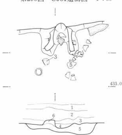
第290図 SJ81遺構図 1:80
