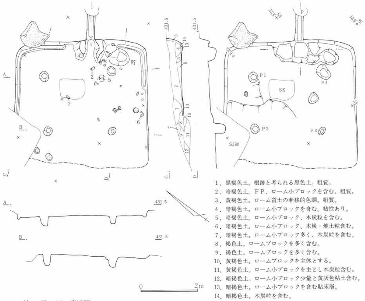
第275図 SJ75遺構図 1:80
