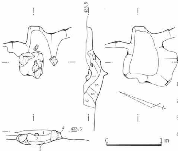
第576図 SJ196竈図 1:40
