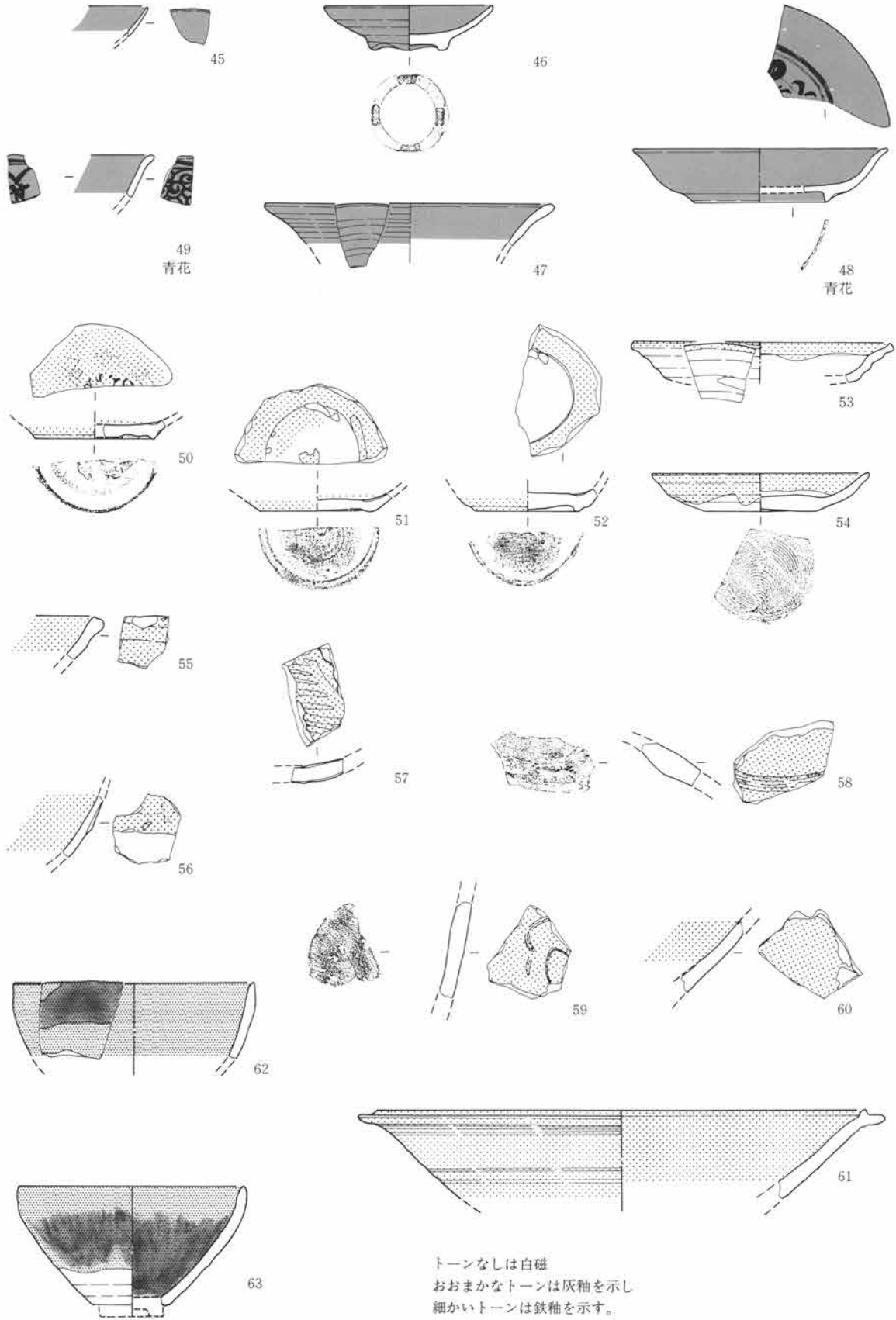
第901図 舶載陶・磁器と国産施釉陶器 1:3
