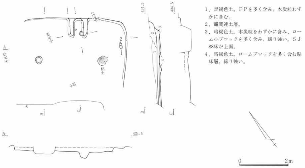
第318図 SJ88遺構図 1:80
