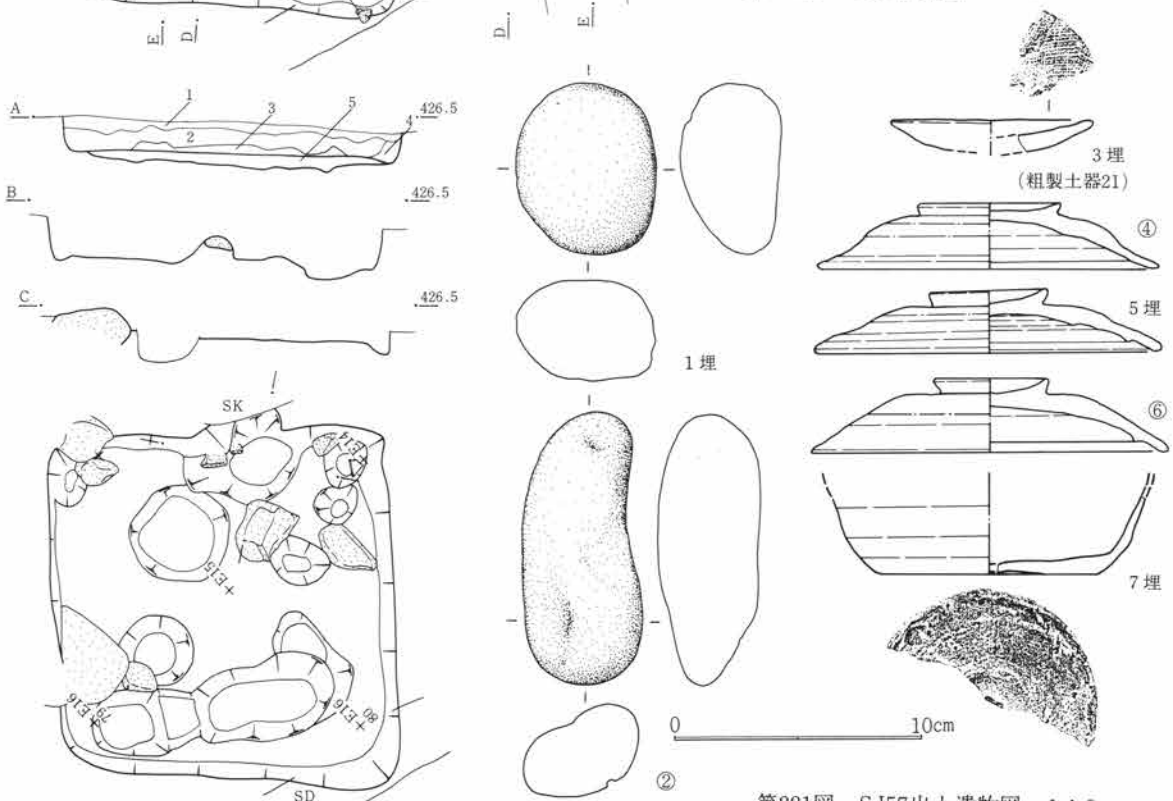
第221図 SJ57出土遺物図 1:3
