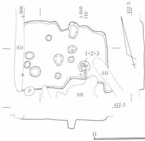
第509図 SJ169遺構図 1:80
