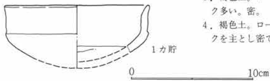
第379図 SJ110出土遺物図 1:3
