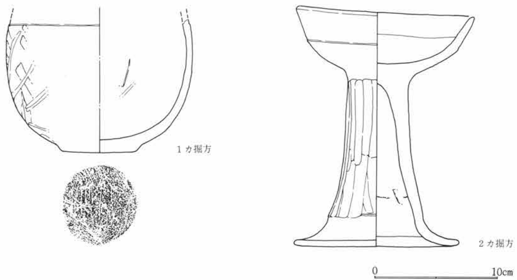
第659図 SJ239出土遺物図 1:3
