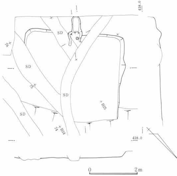
第554図 SJ185遺構図 1:80
