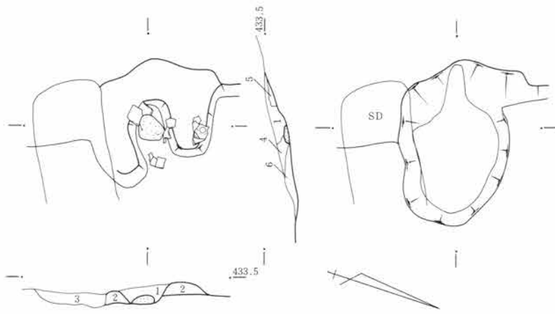
第834図 SJ320竈図 1:40
