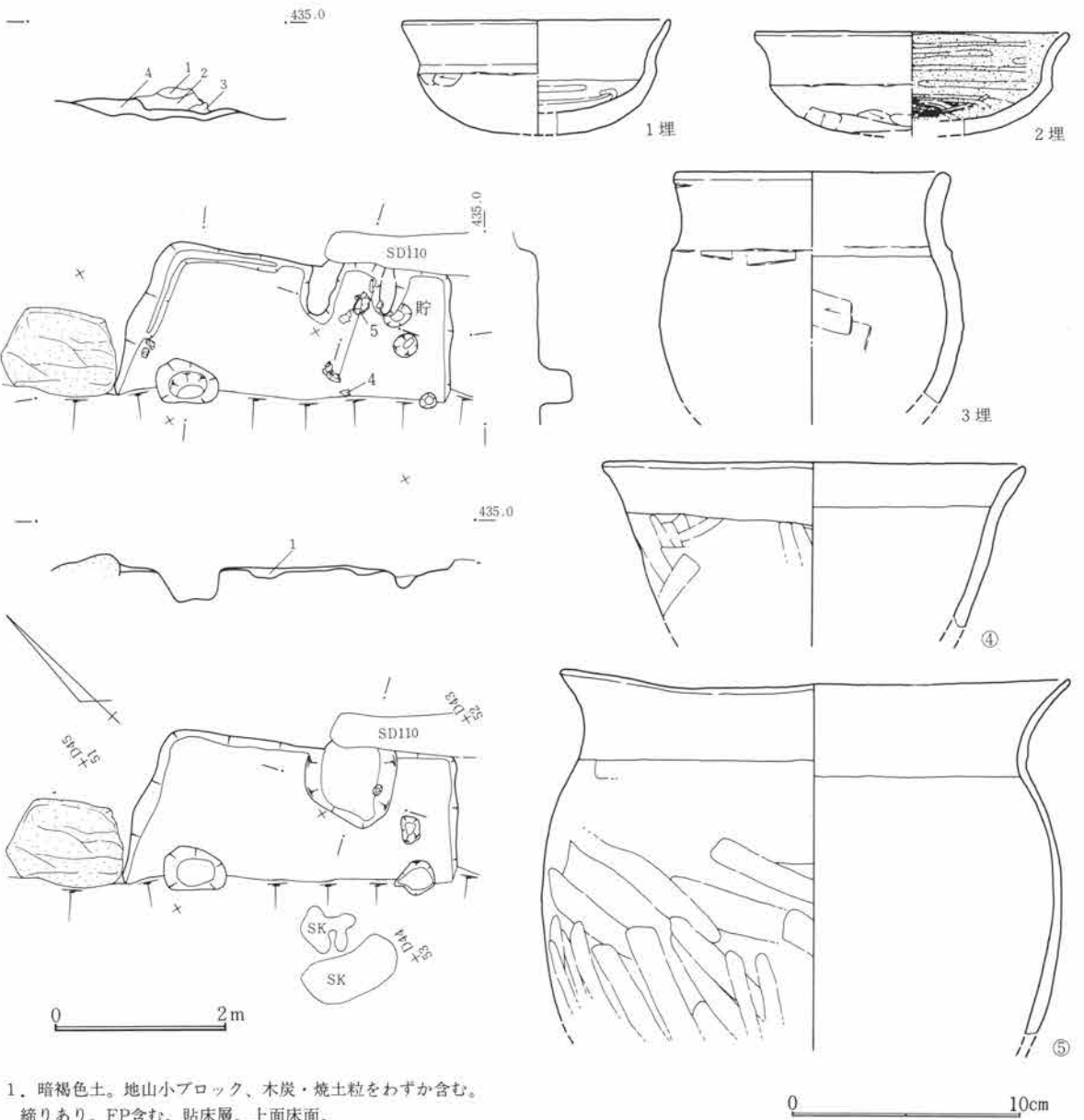
第123図 SJ29遺構図 1:80
