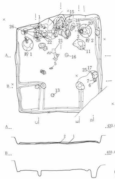
第138図 SJ33遺構図 1:80
