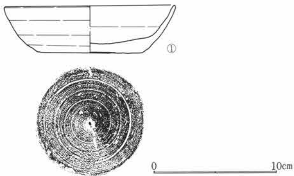
第122図 SJ28出土遺物図 1:3
