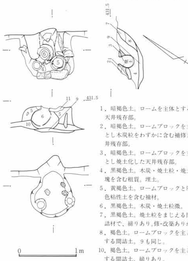
第763図 SJ286竈図 1:40
