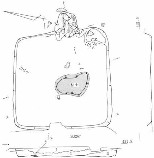
第707図 SJ265遺構図 1:80
