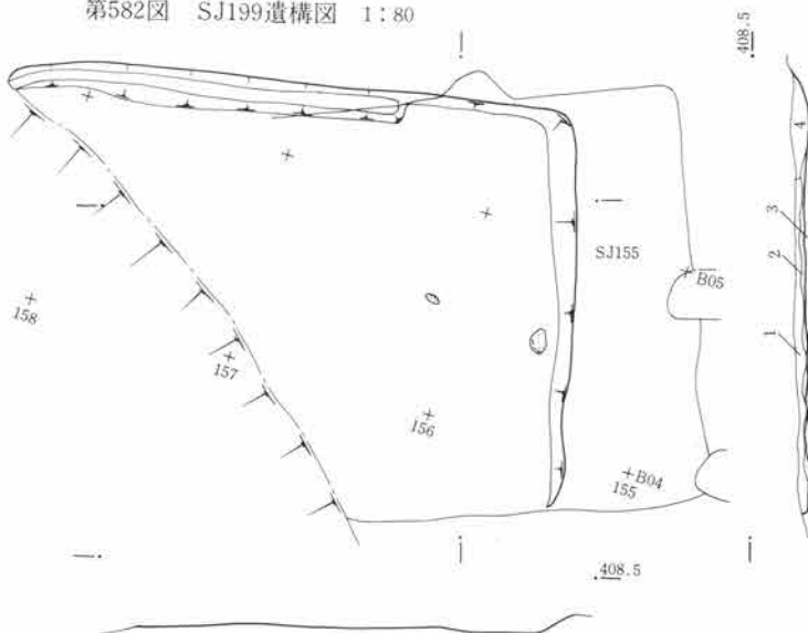
第582図 SJ199遺構図 1:80
