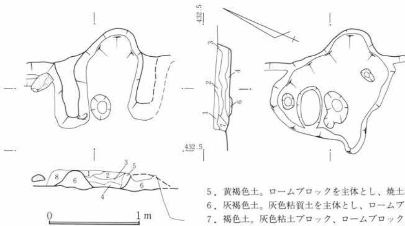
第412図 SJ124竈図 1:40
