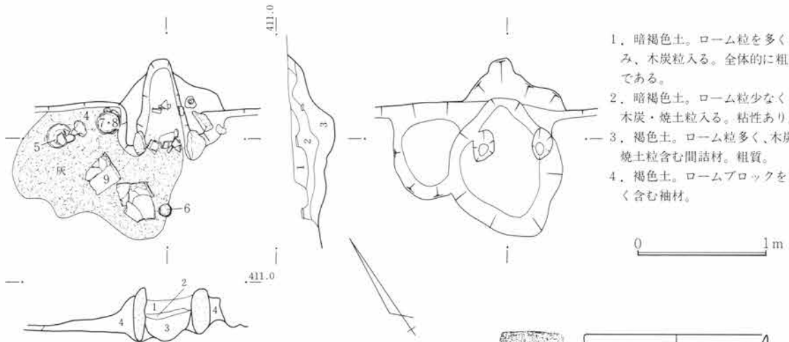
第543図 SJ181竈図 1:40
