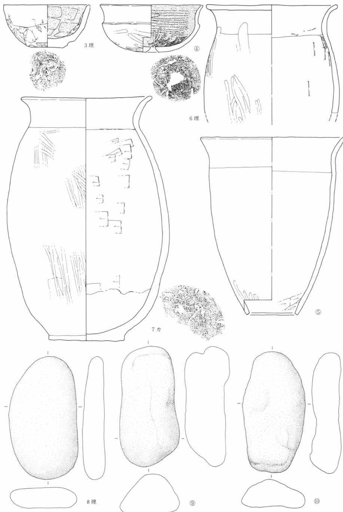
第407図 SJ122出土遺物図 1:3
