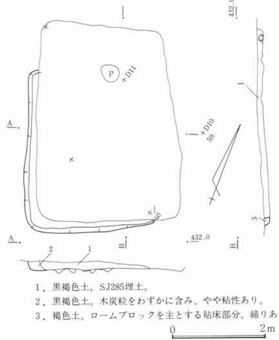
第784図 SJ294遺構図 1:80
