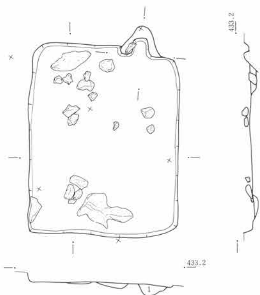
第677図 SJ247遺構図 1:80
