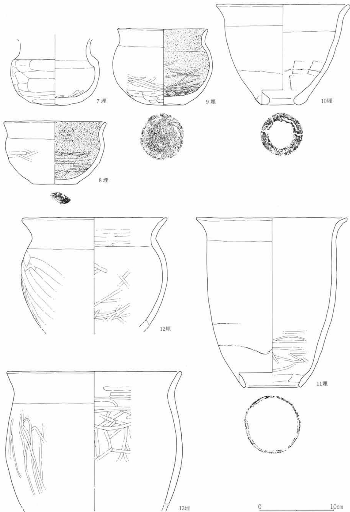
第313図 SJ86出土遺物図 1:3
