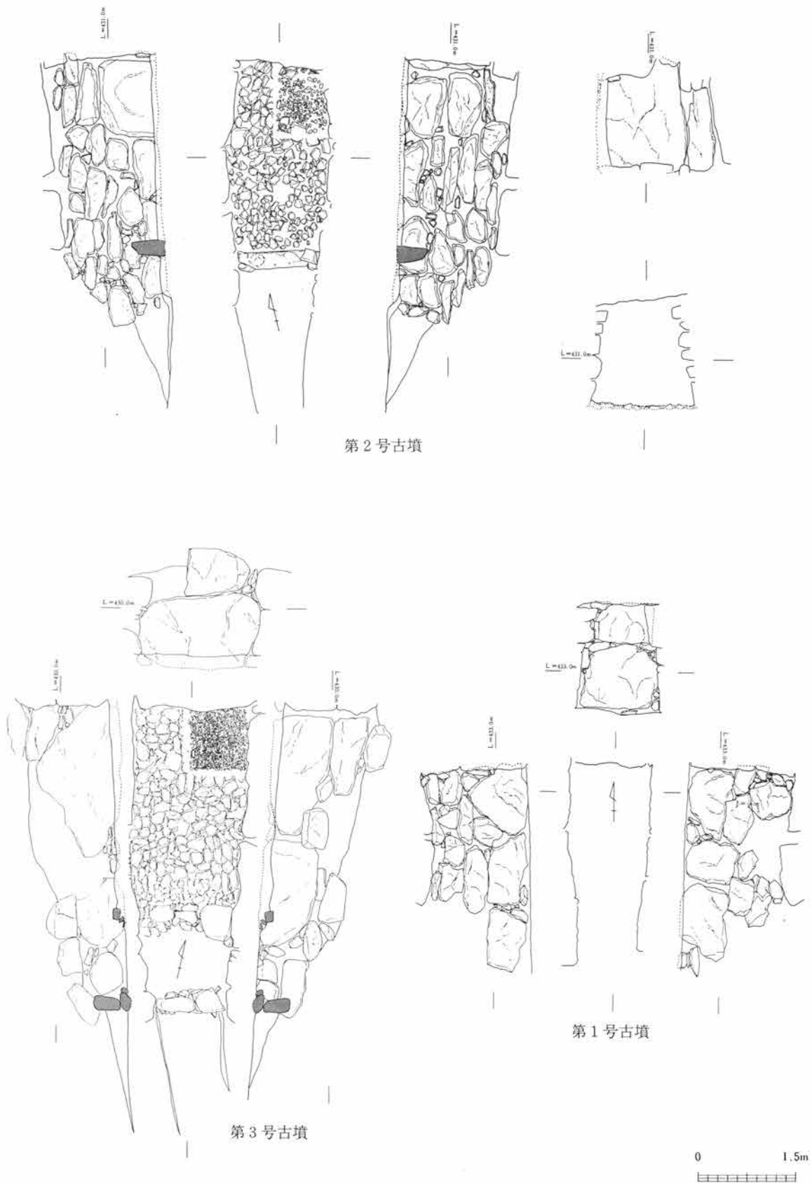
第10図 金山古墳群1・2・3号古墳石室実測図 1:80
