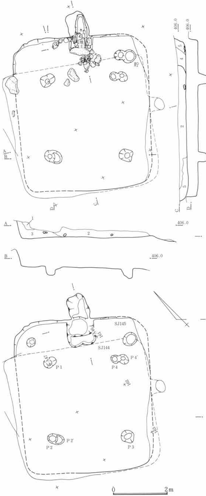
第460図 SJ145遺構図 1:80
