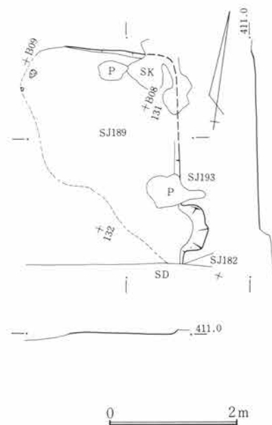
第565図 SJ189遺構図 1:80
