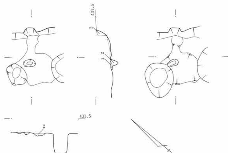
第661図 SJ240竈図 1:40
