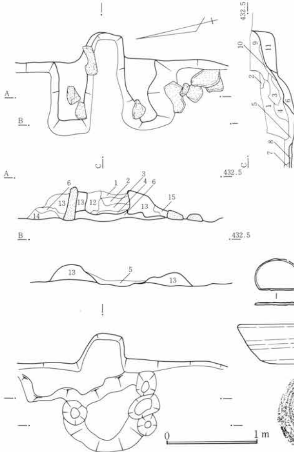
第284図 SJ79竈図 1:40
