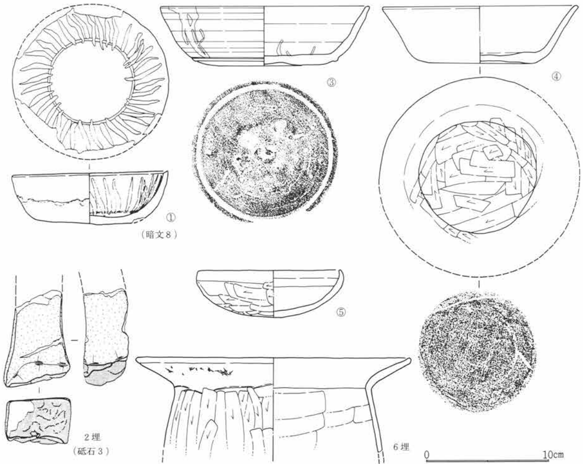
第402図 SJ121出土遺物図 1 : 3
