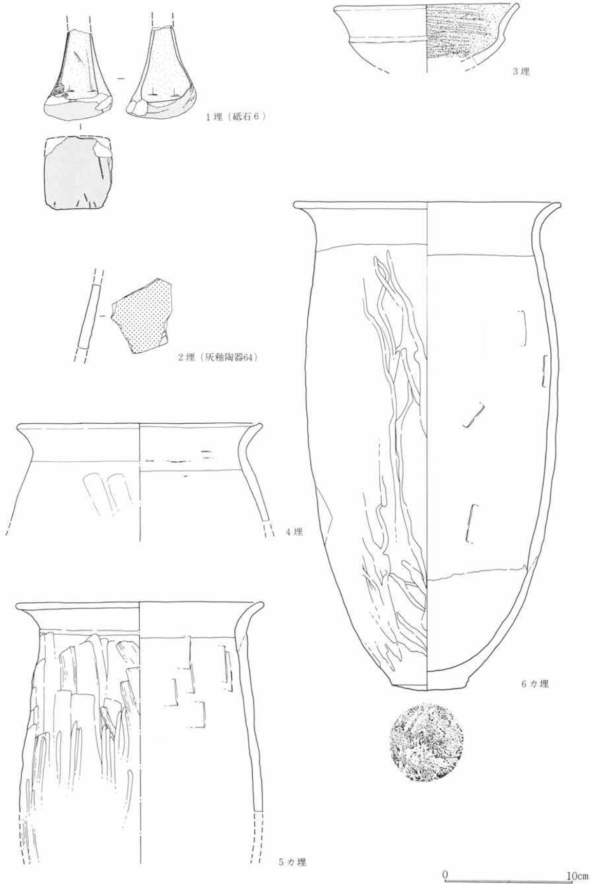
第526図 SJ175出土遺物図 1:3
