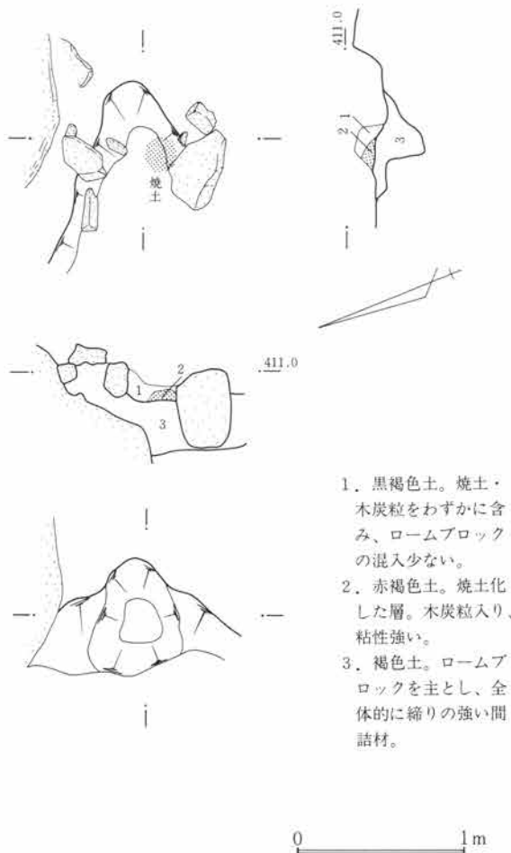
第606図 SJ217竈図 1:40
