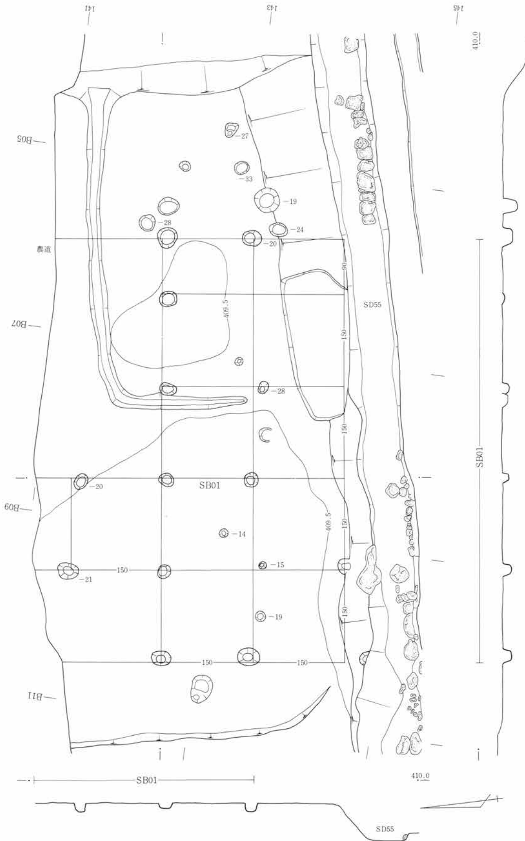
第20図 SB01遺構図 1 : 80
