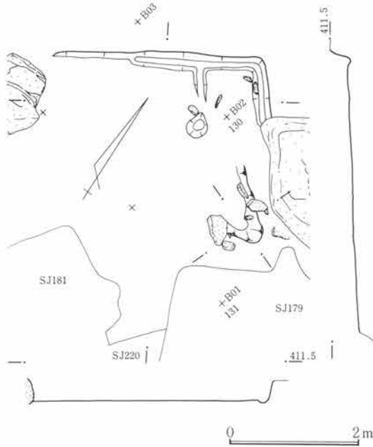
第605図 SJ217遺構図 1:80
