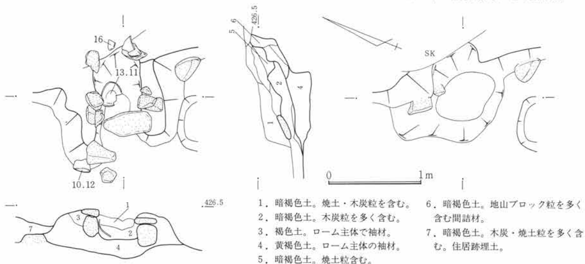
第219図 SJ57竈図 1:40
