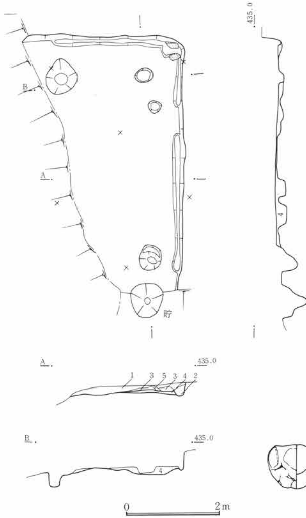
第112図 SJ25遺構図 1:80
