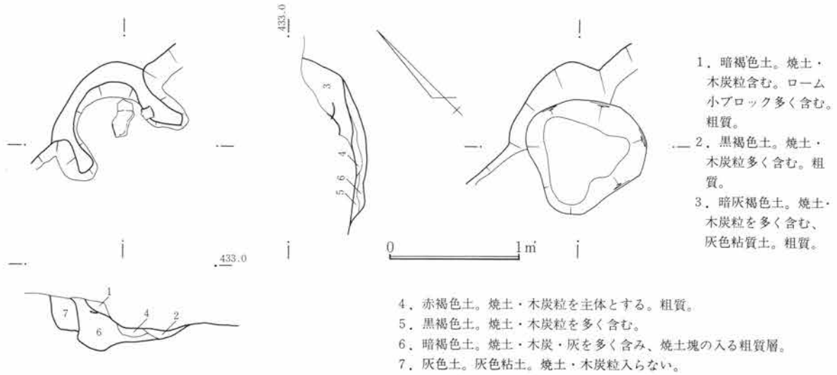
第162図 SJ38竈図 1:40
