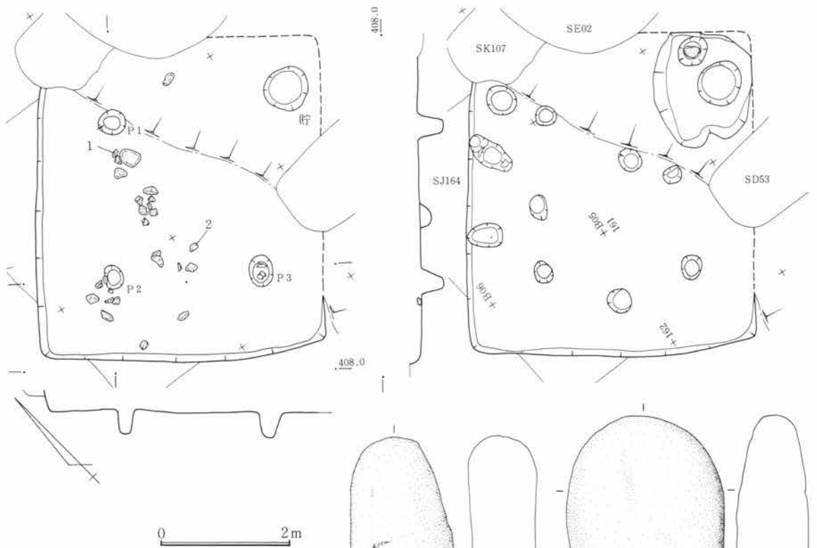
第499図 SJ165遺構図 1:80
