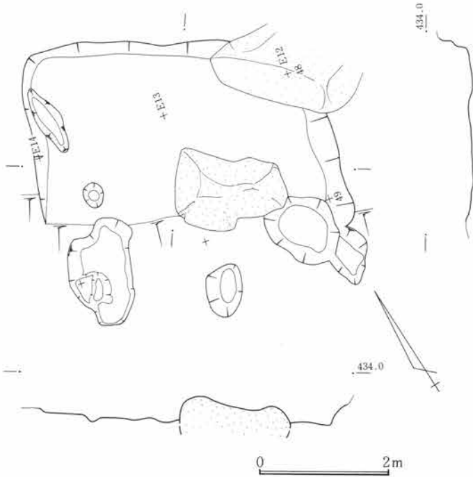
第617図 SJ223遺構図 1:80
