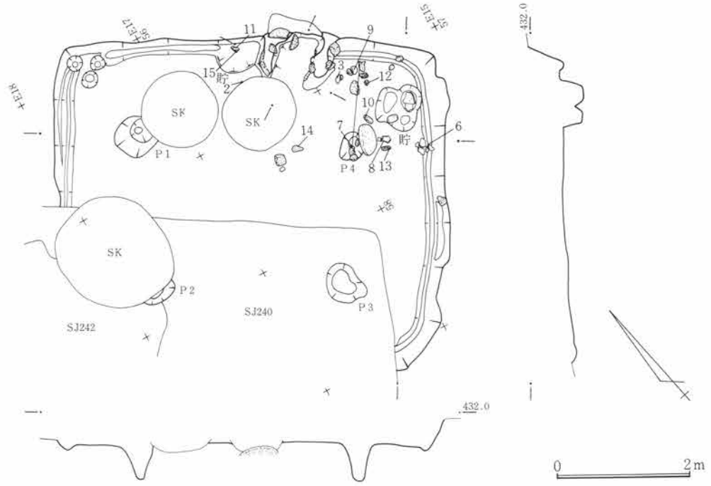
第371図 SJ108遺構図 1:80
