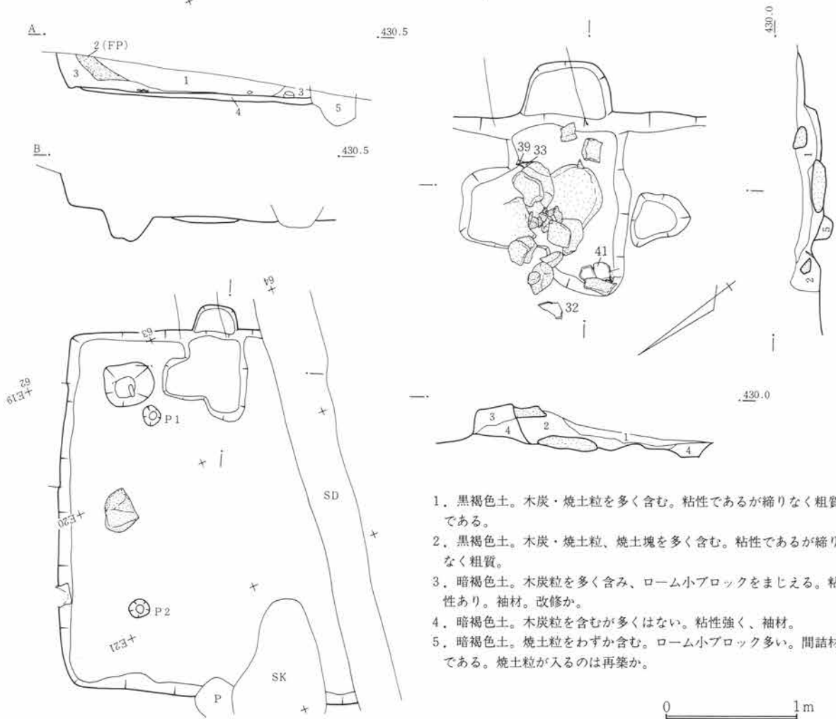
第229図 SJ60遺構図 1:80
