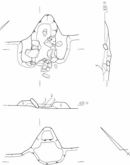
第415図 SJ125集石図 1:40
