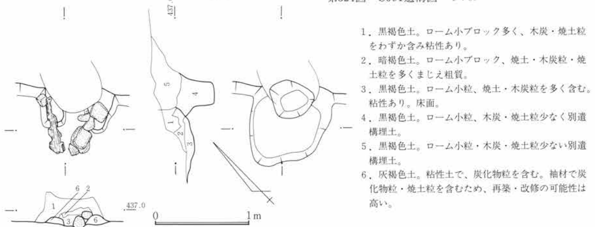
第325図 SJ91竈図 1:40
