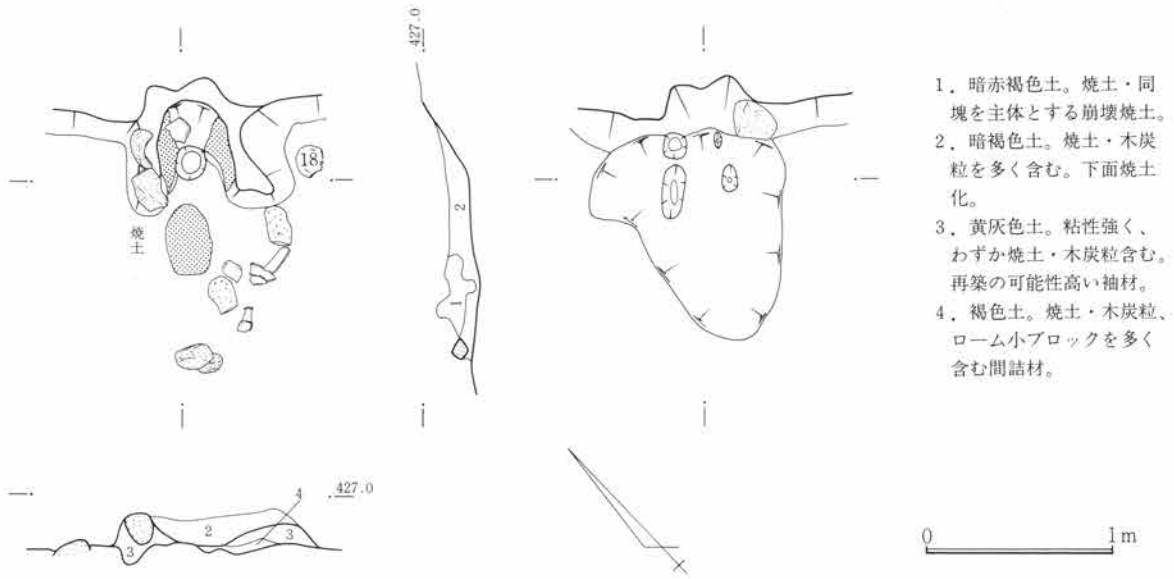
第223図 SJ58竈図 1:40
