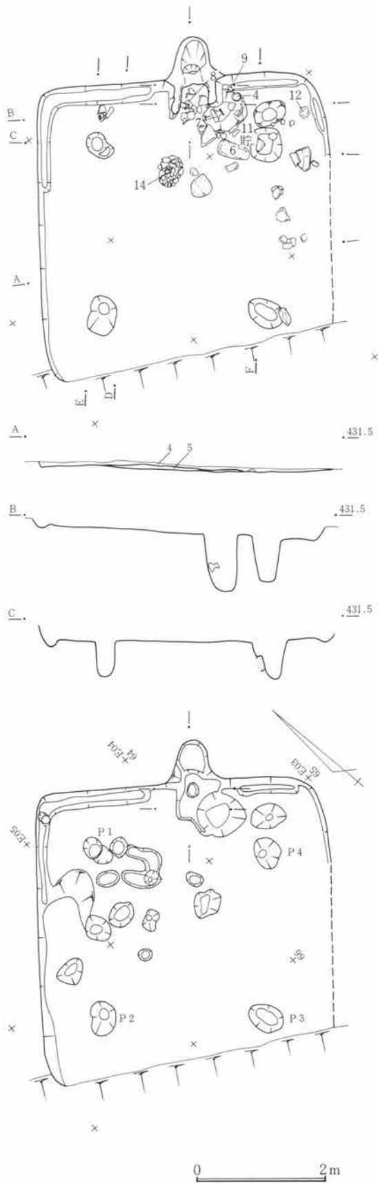
第321図 SJ89遺構図 1:80
