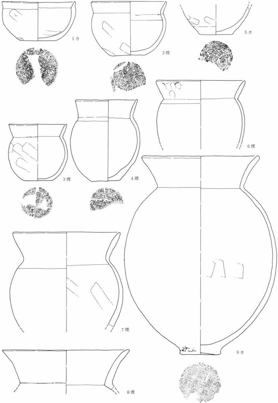
第247図 SJ64出土遺物図 1:3
