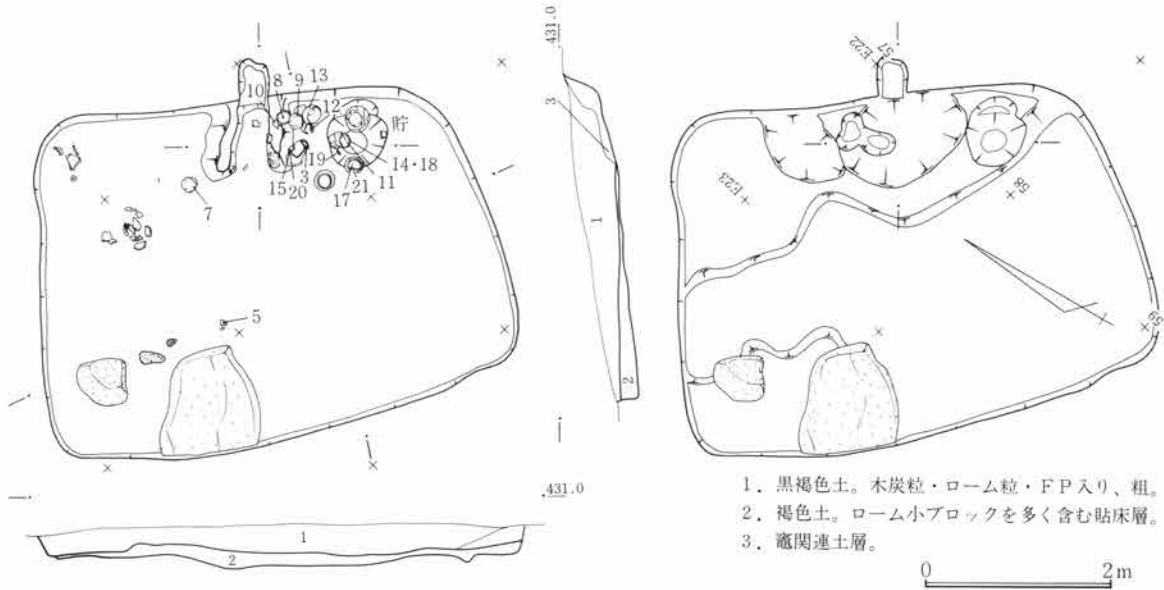
第629図 SJ231遺構図 1:80
