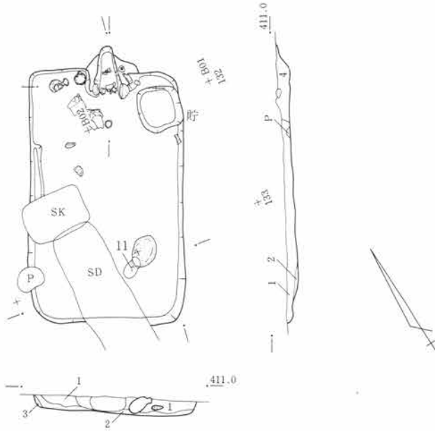
第542図 SJ181遺構図 1:80
