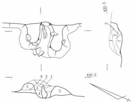
第787図 SJ297遺構図 1:80
