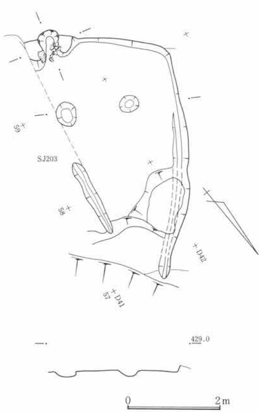
第792図 SJ299遺構図 1:80
