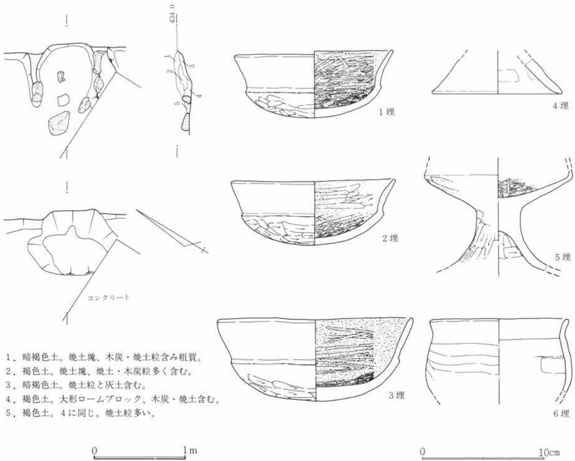
第311図 SJ86竈図 1:40
