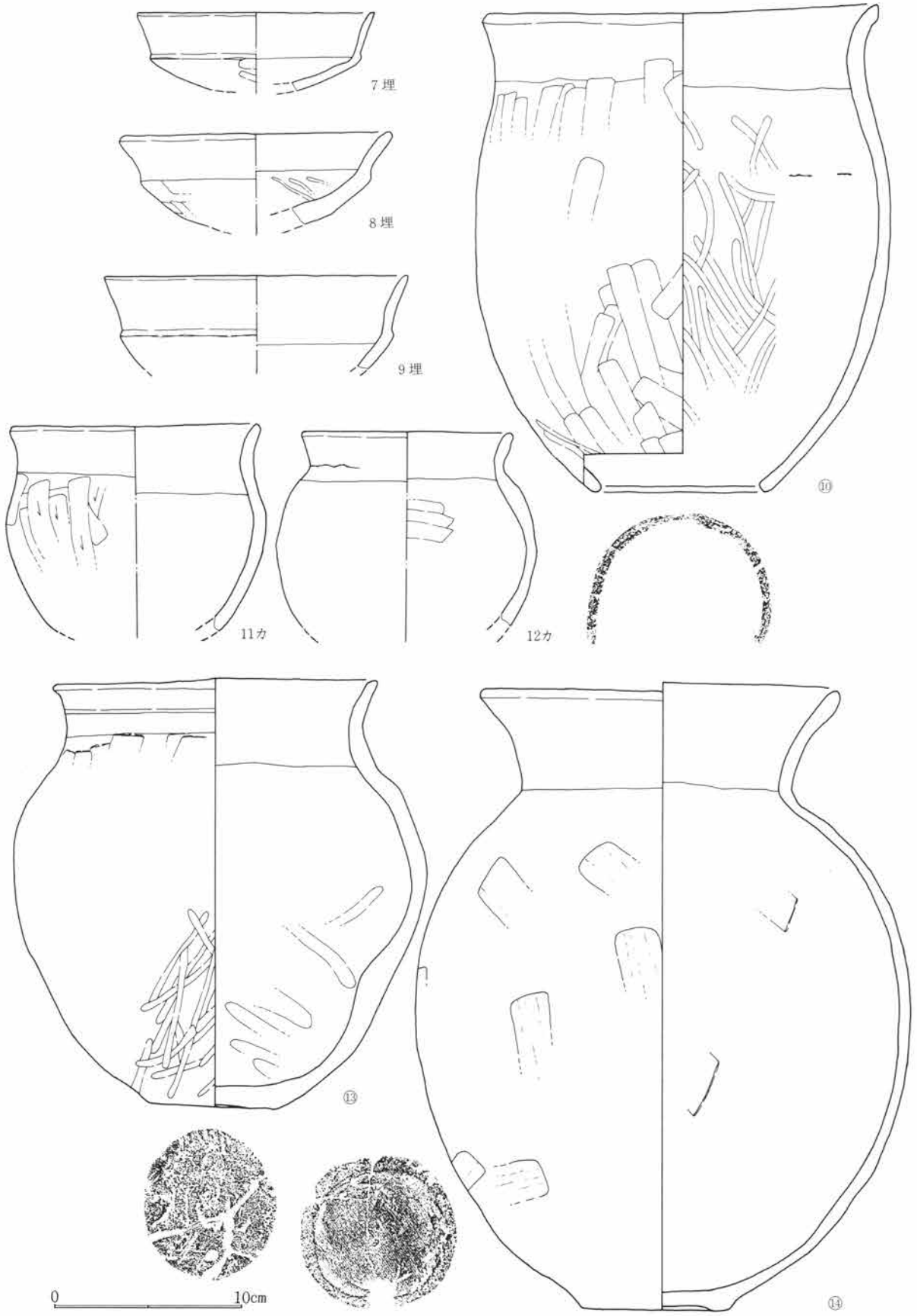
第97図 SJ19出土遺物図 1 : 3
