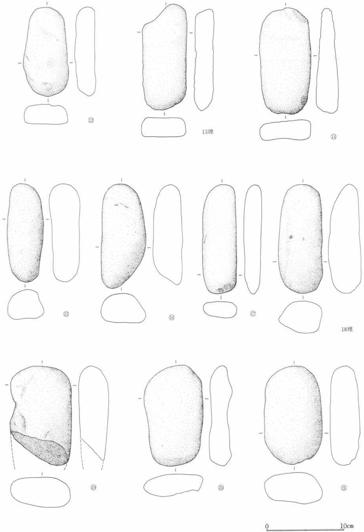
第811図 SJ305出土遺物図 1:3
