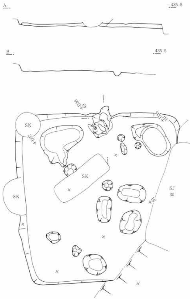
第236図 SJ61遺構図 1:80
