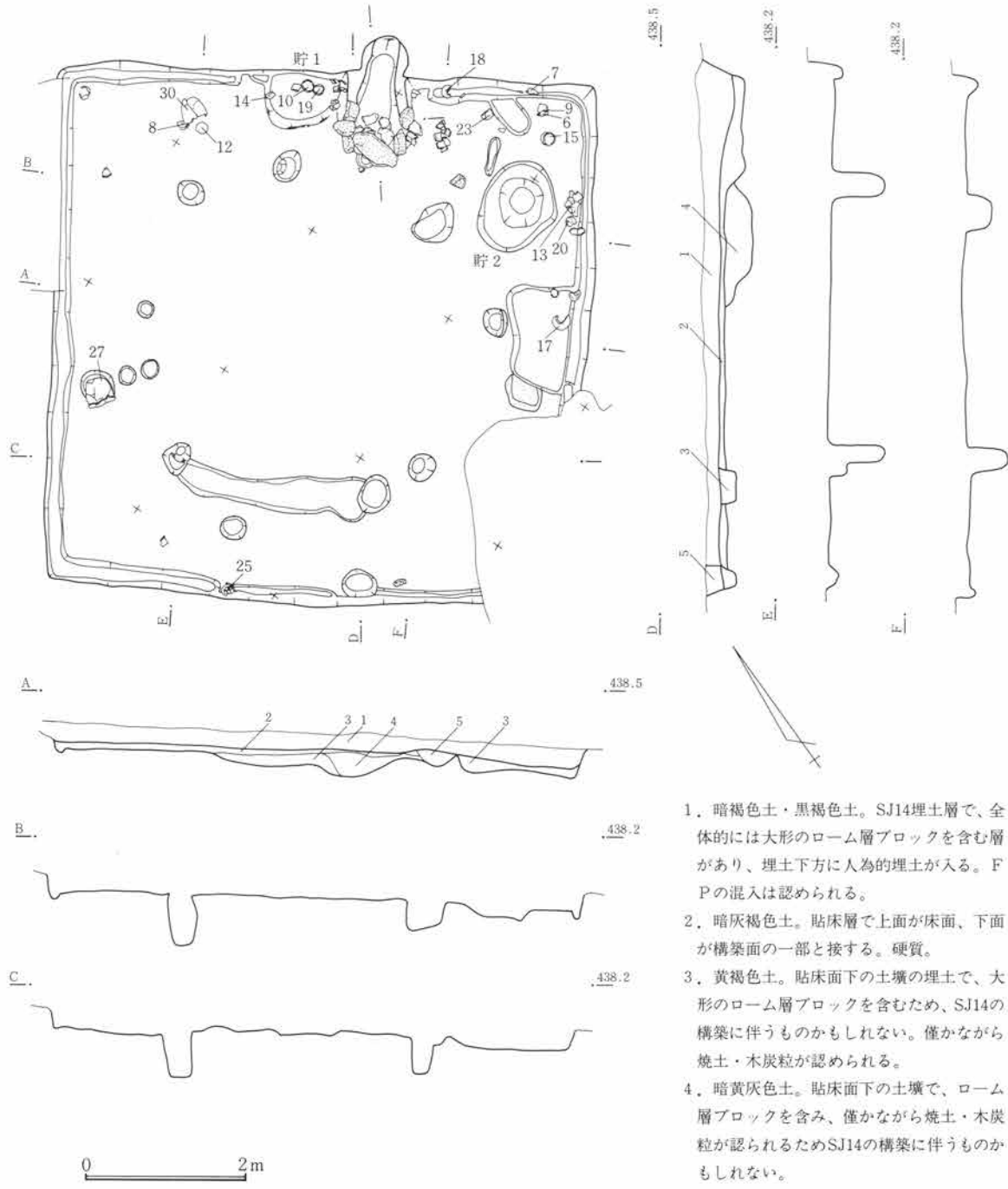
第74図 SJ14遺構図 1:80
