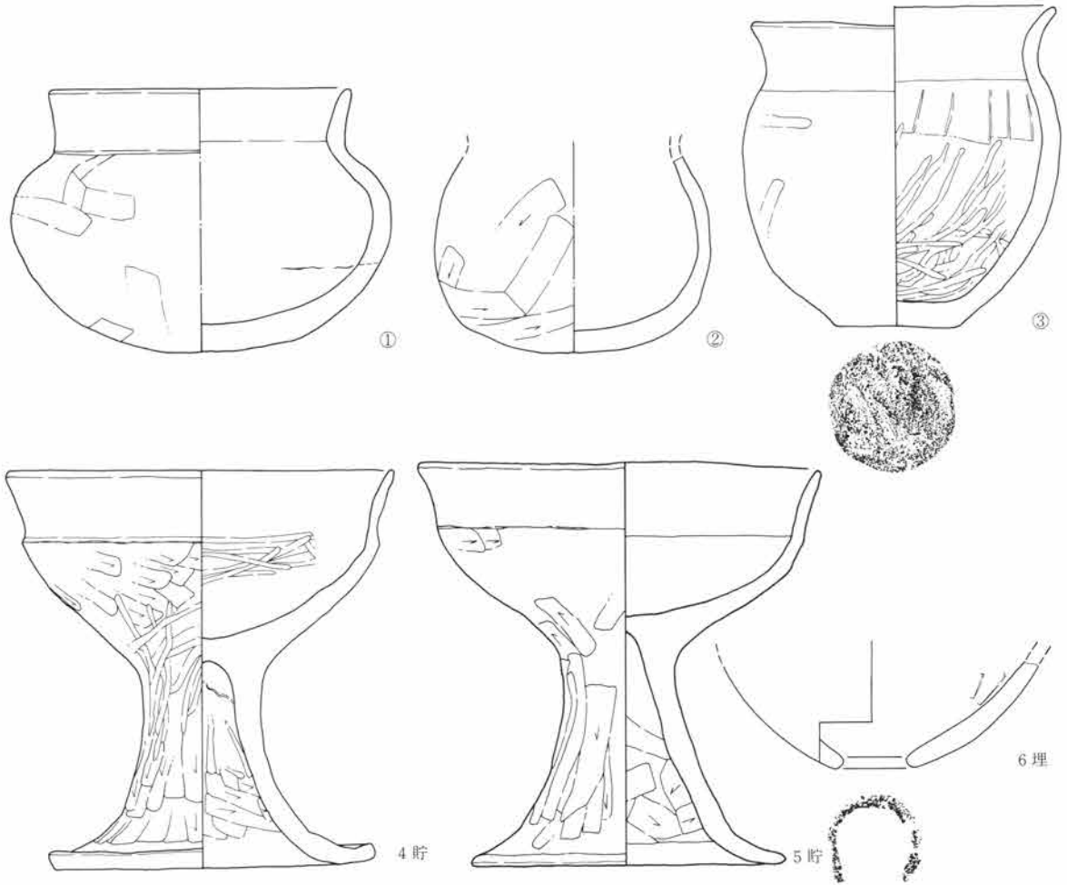
第782図 SJ292出土遺物図 1:3
