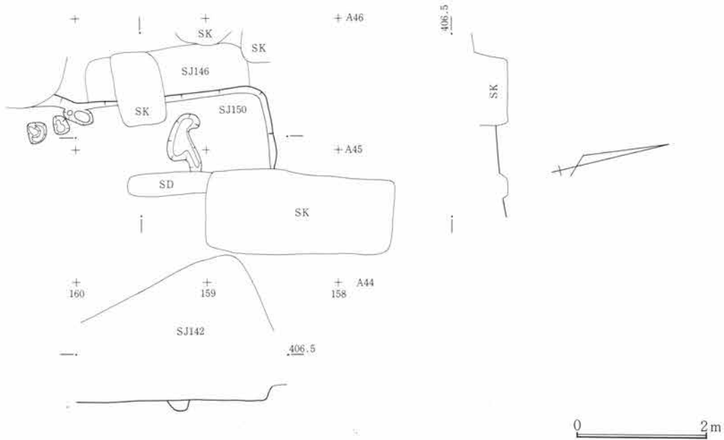
第474図 SJ150遺構図 1:80
