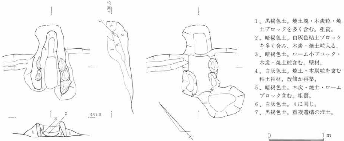
第268図 SJ72竈図 1:40
