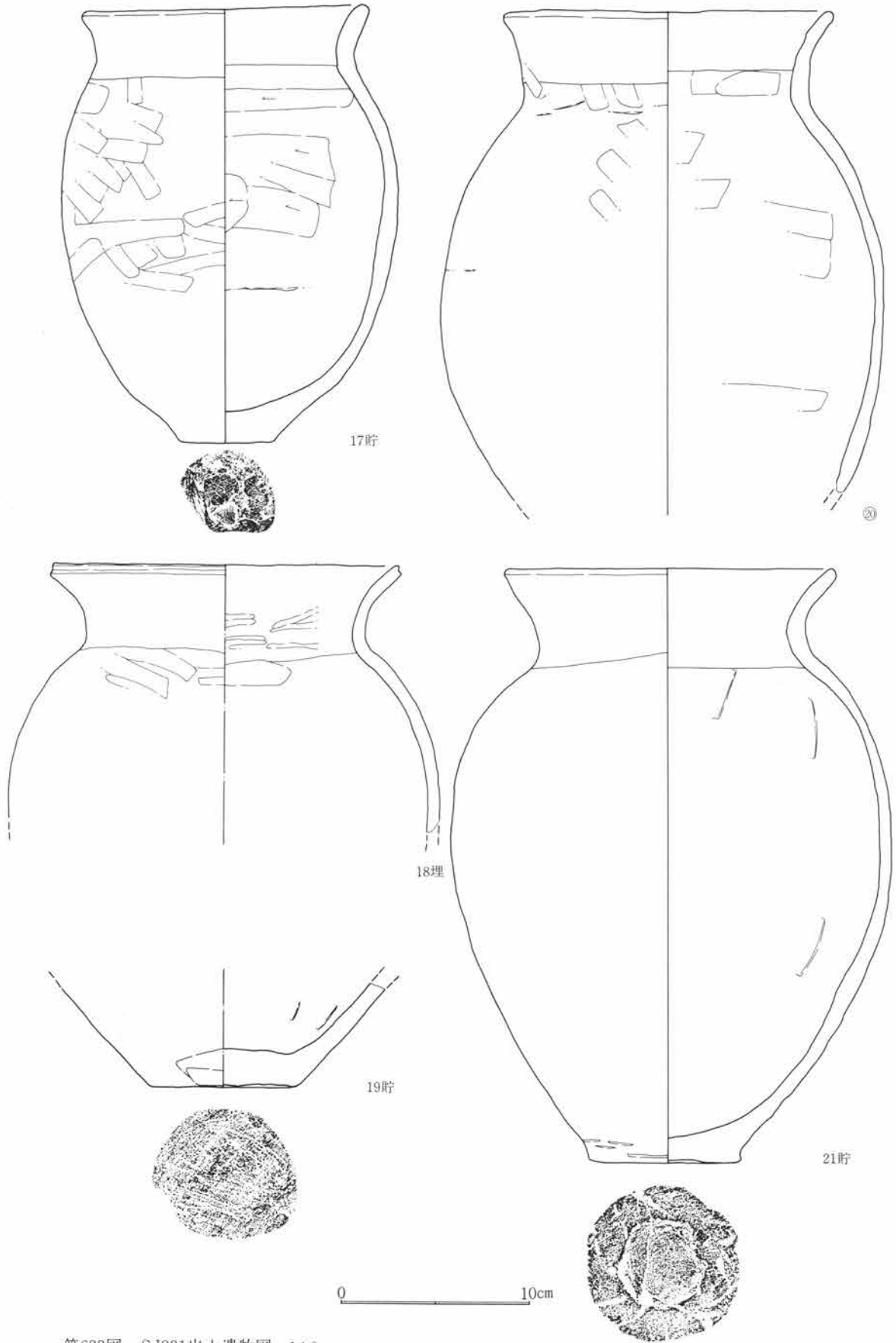
第633図 SJ231出土遺物図 1:3
