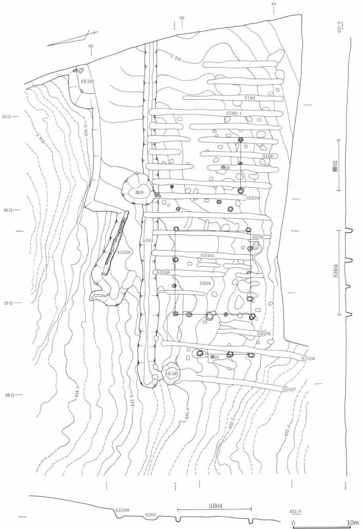
第24図 SB04・柵01・柵02と周辺遺構図 1:200
