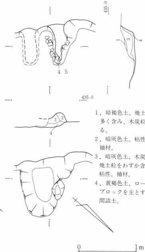
第813図 SJ306竈図 1:40
