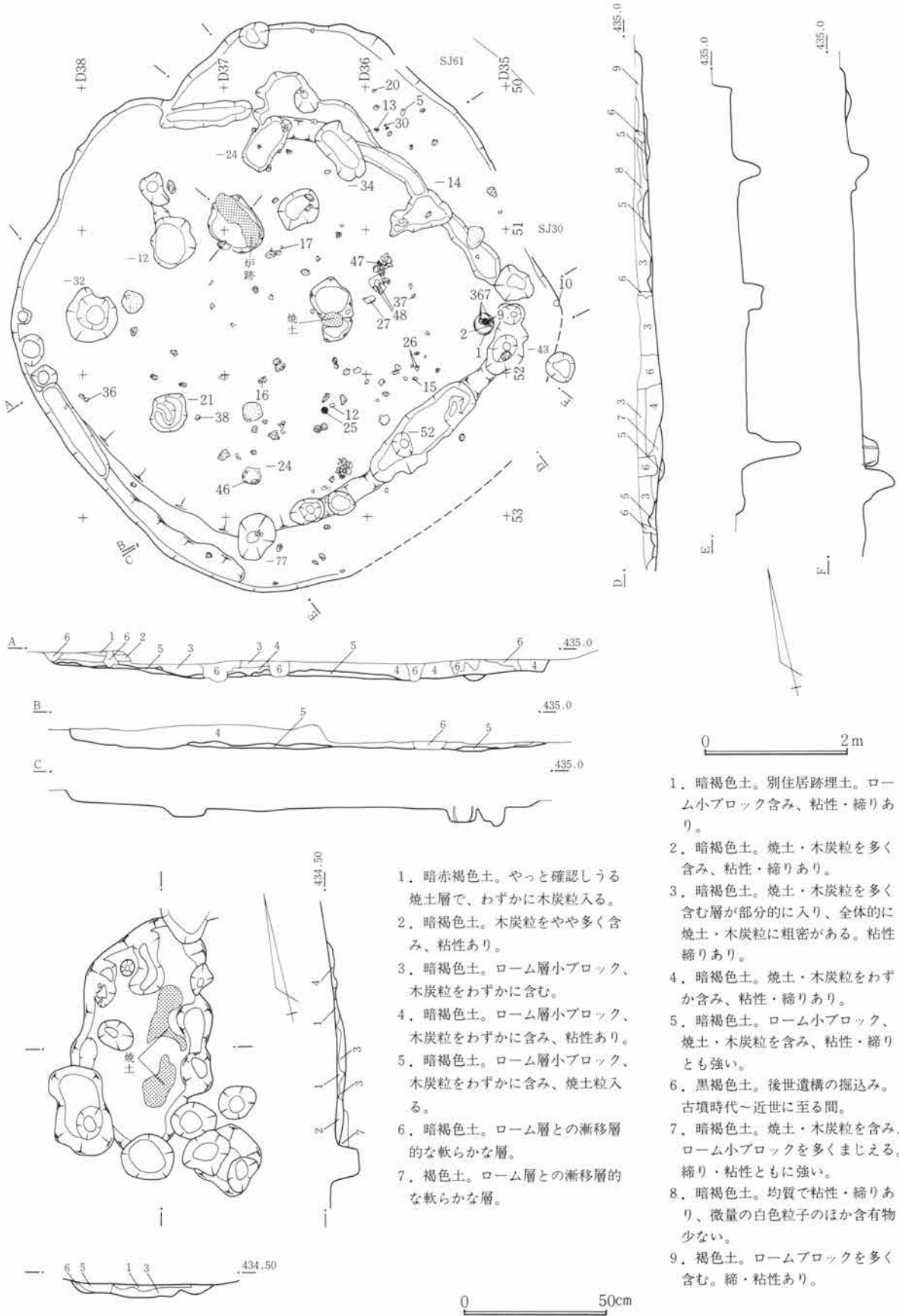
第849図 SJ67遺構図（住居図1：80 炉跡図1：20）
