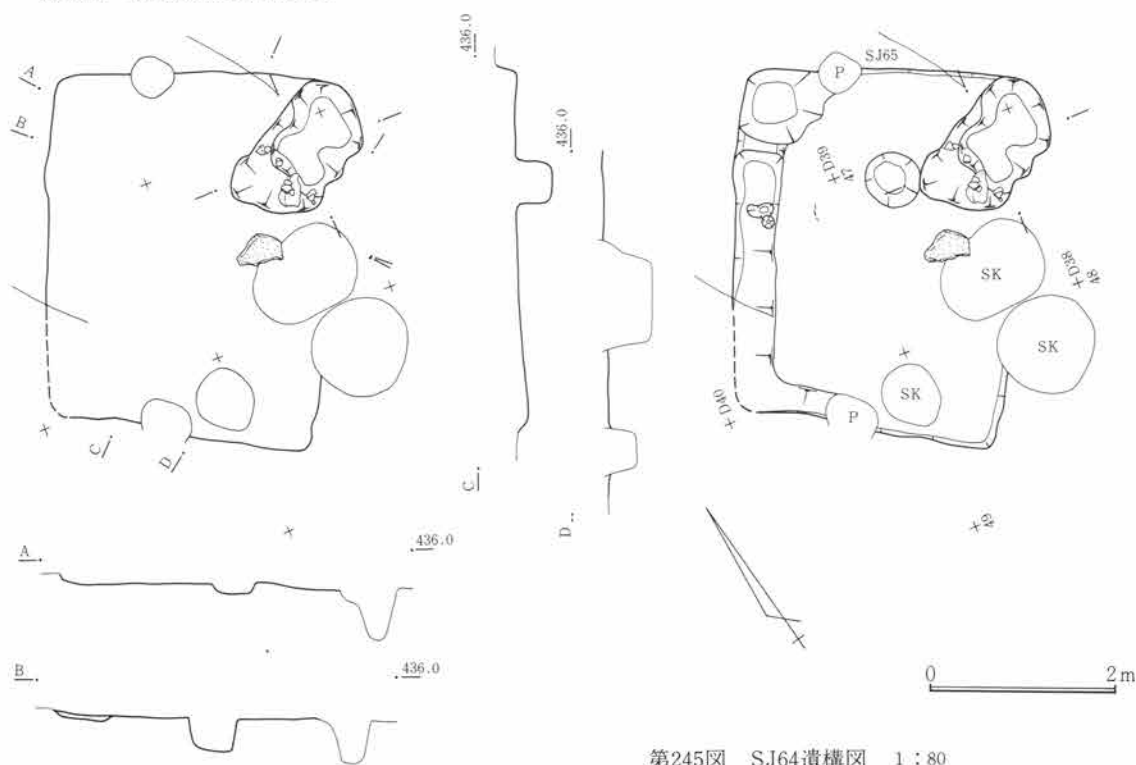
第245図 SJ64遺構図 1:80
