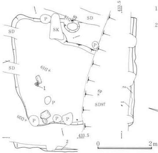
第580図 SJ198遺構図 1:80
