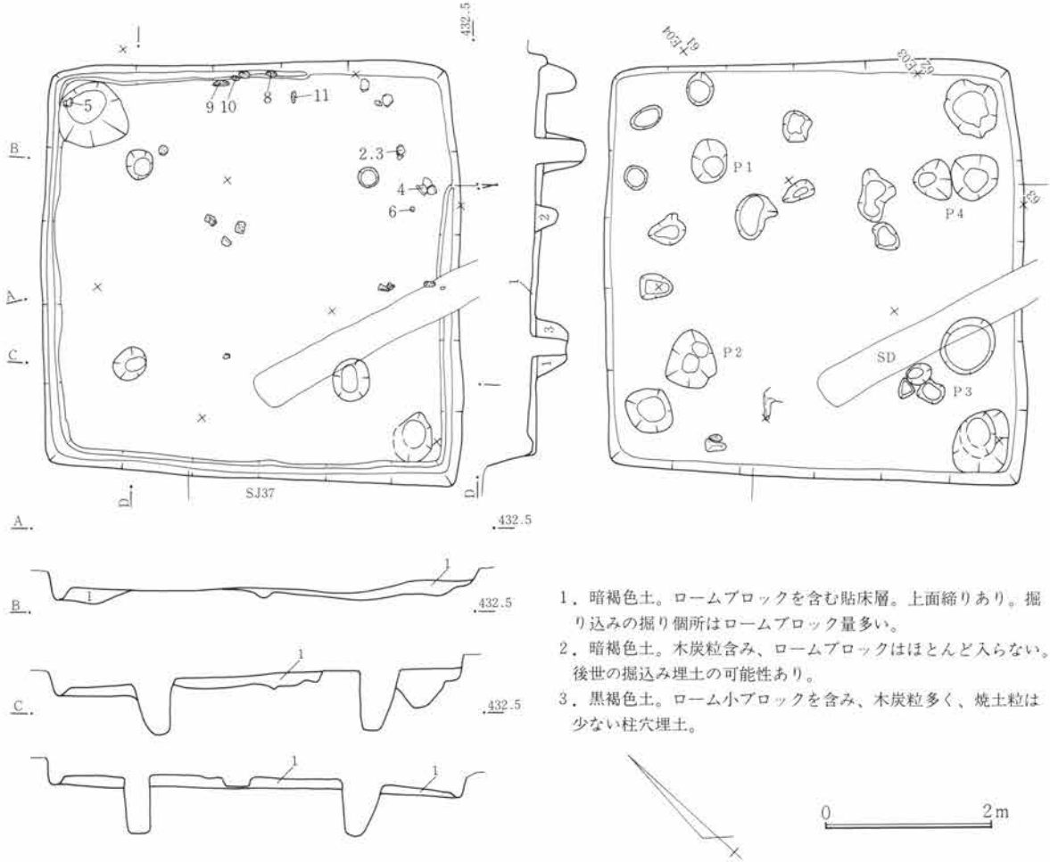
第336図 SJ94遺構図 1 : 80
