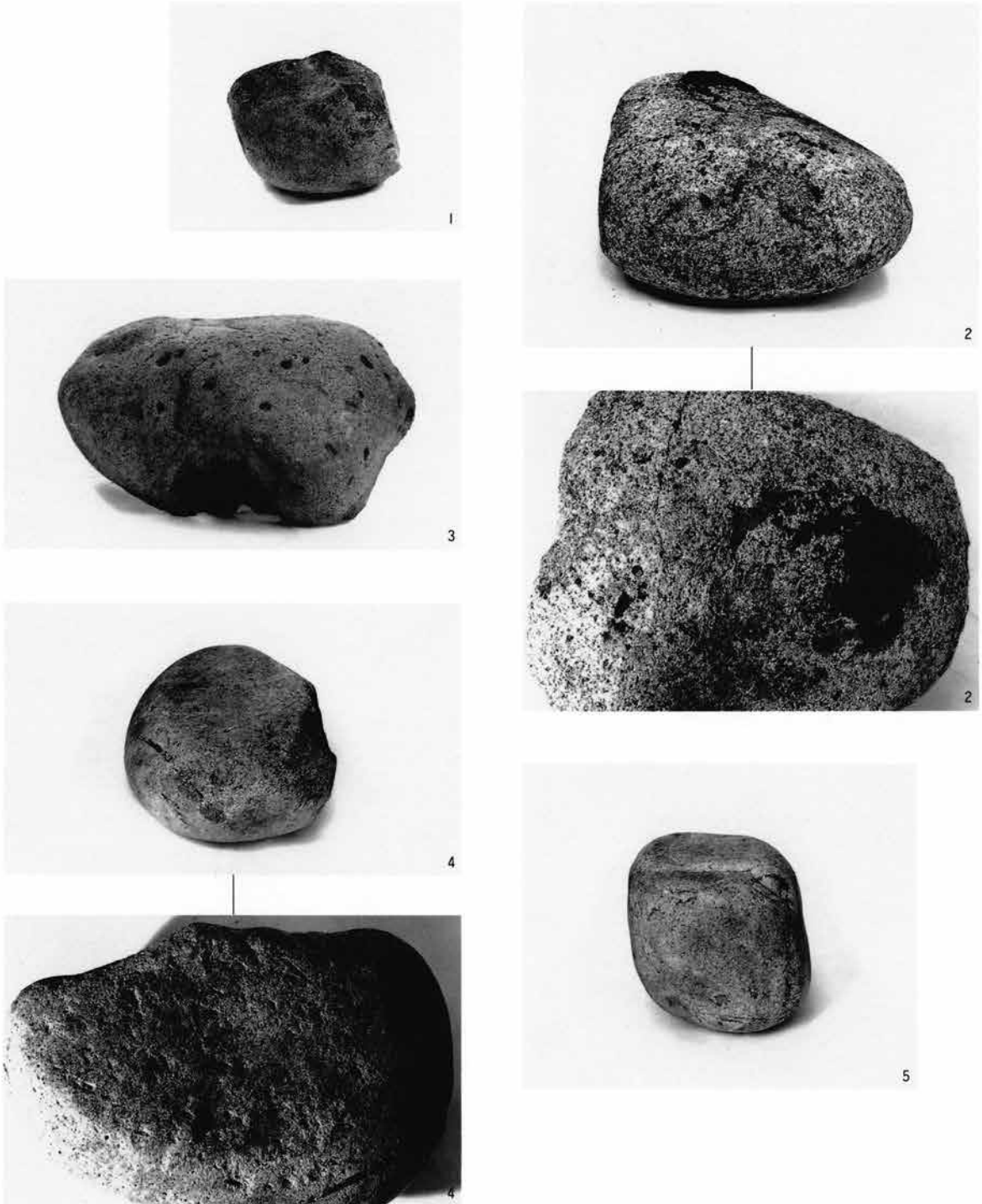
I区鍛冶工房跡出土台石（鉄床）
