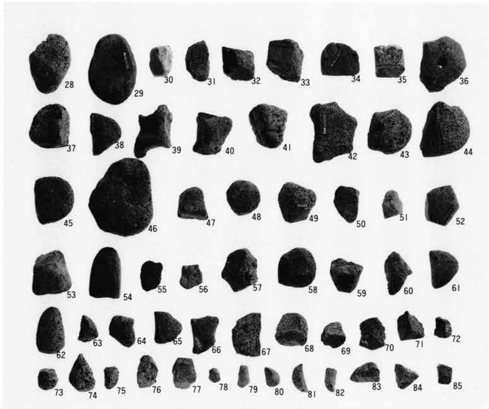
ⅠⅠ号鍛冶工房跡出土遺物
