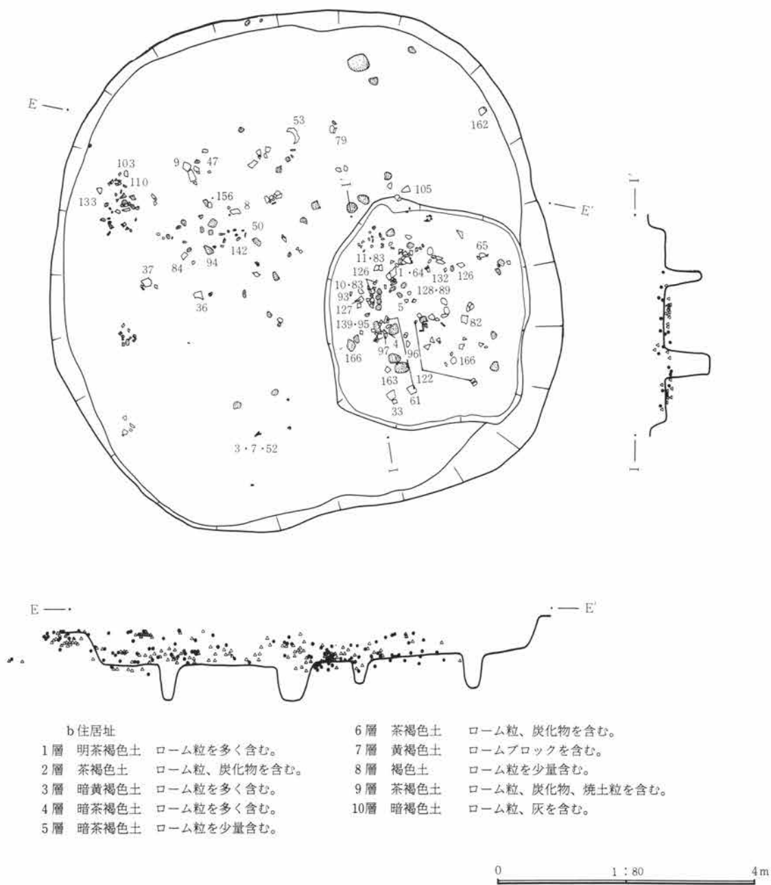
第57図 66号住居址遺物出土状態実測図
