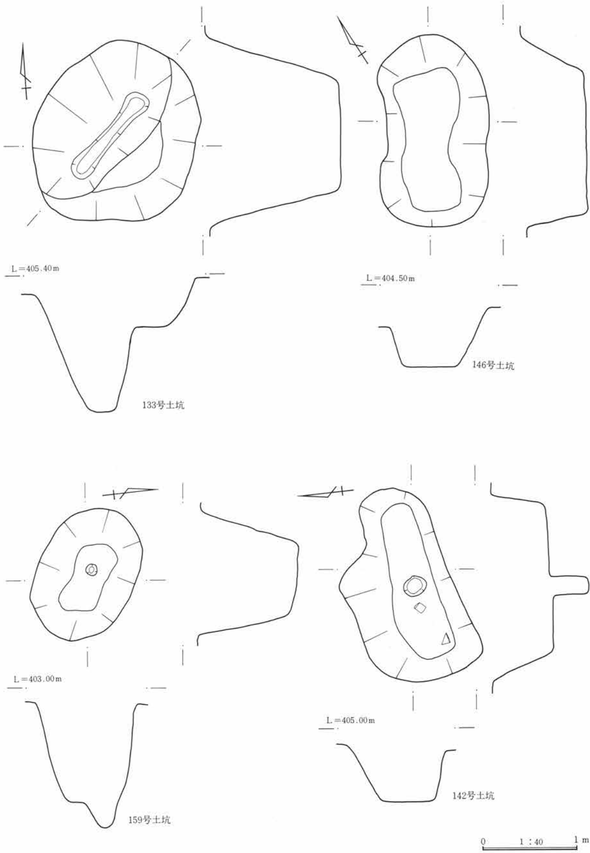
第486图 土坑实测图
