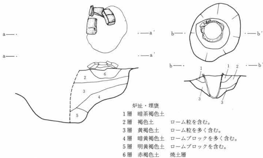
第376図 131号a・b住居址・炉址実測図
