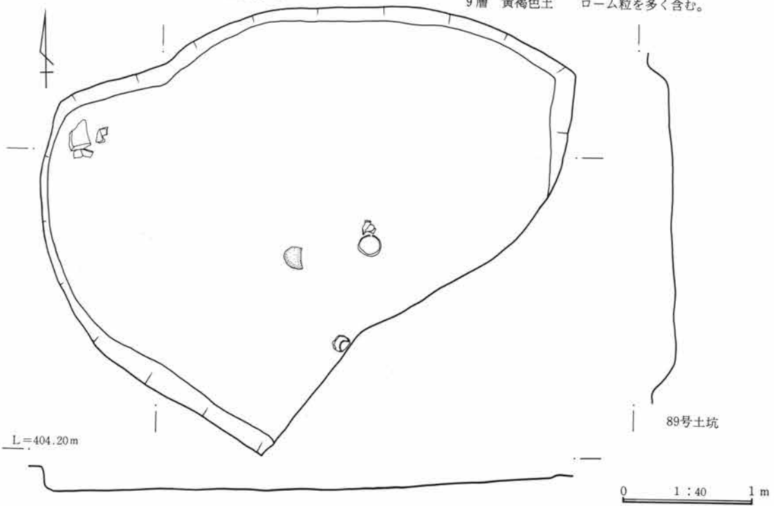
第545図 土坑実測図
