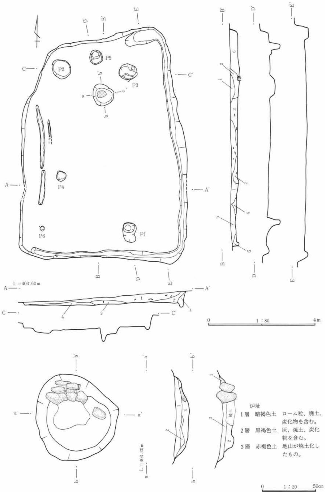
第90図 72号住居址・炉址実測図
