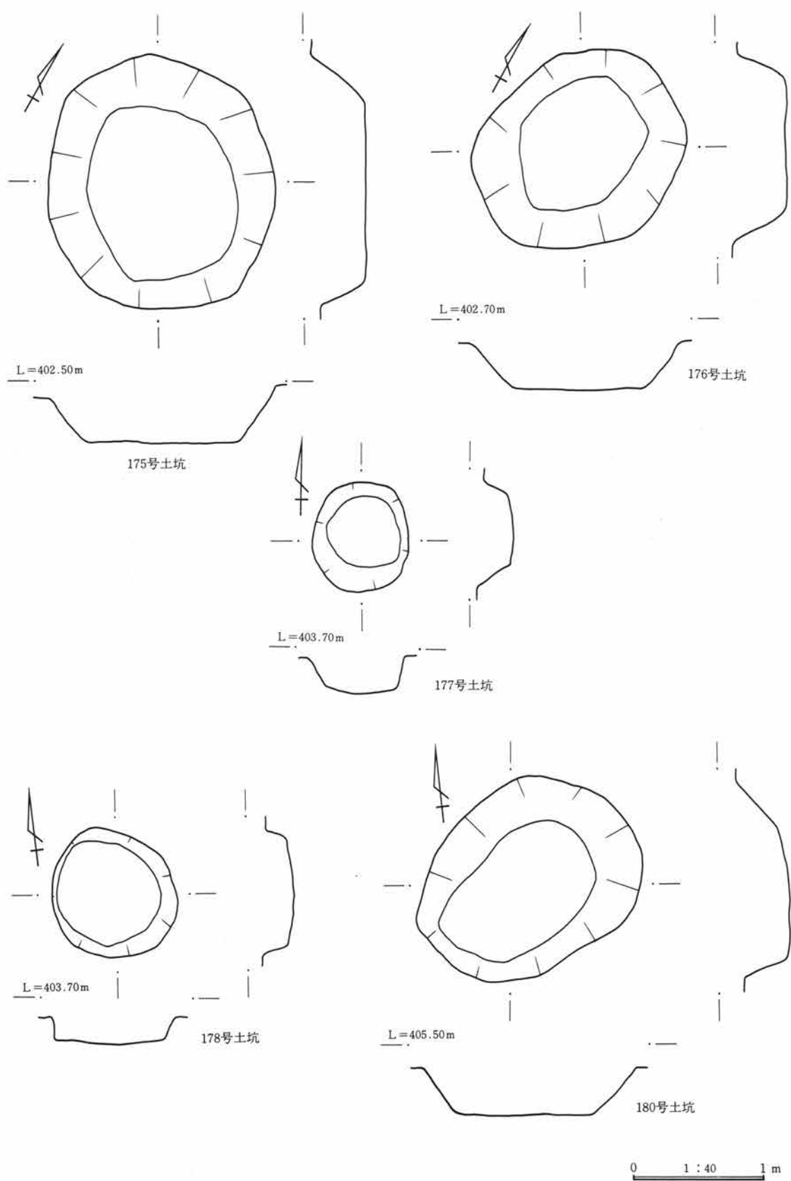
第521图 土坑实测图
