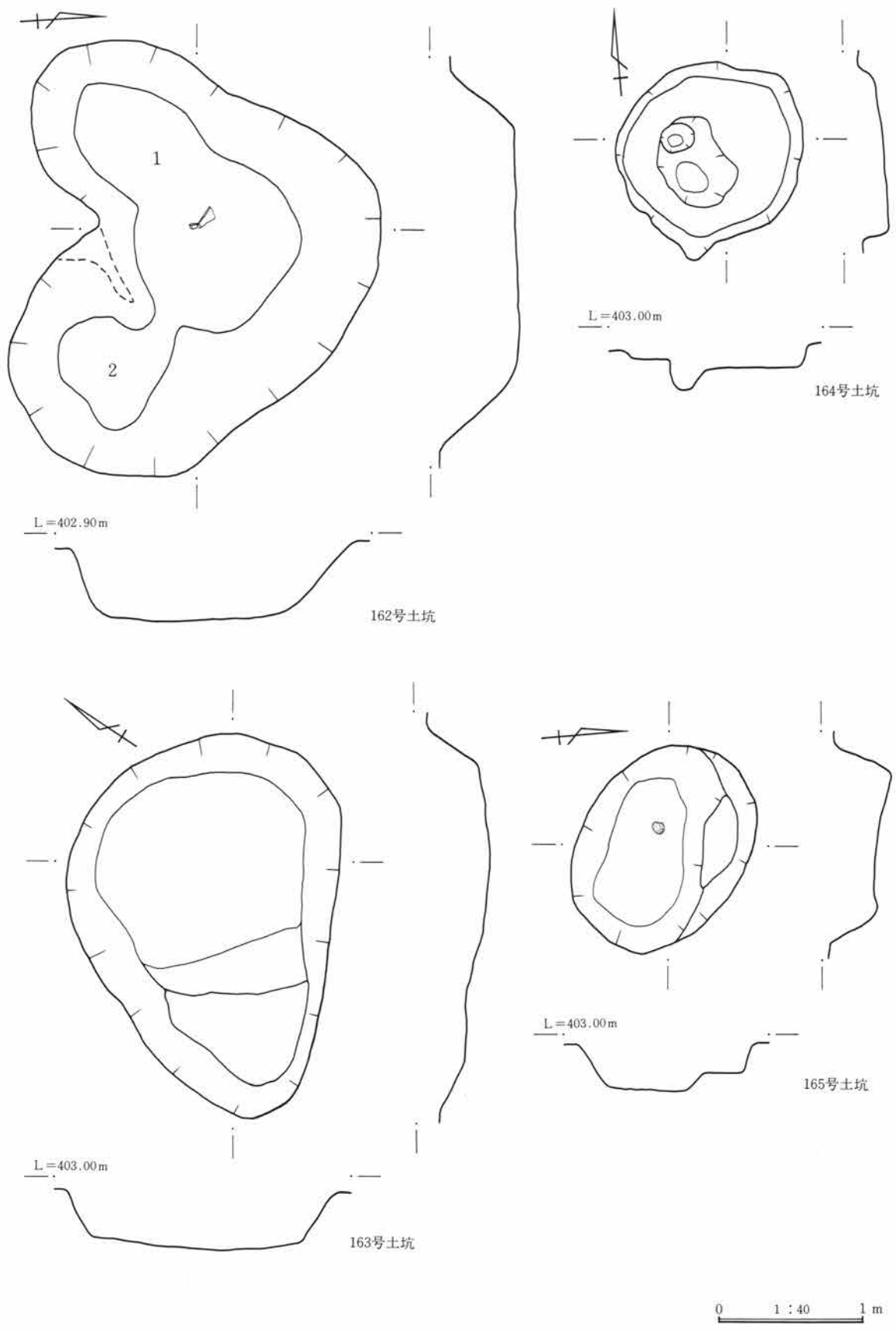
第518图 土坑实测图
