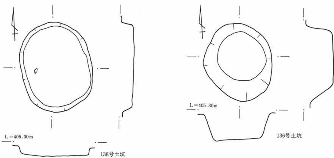
第513图 土坑实测图
