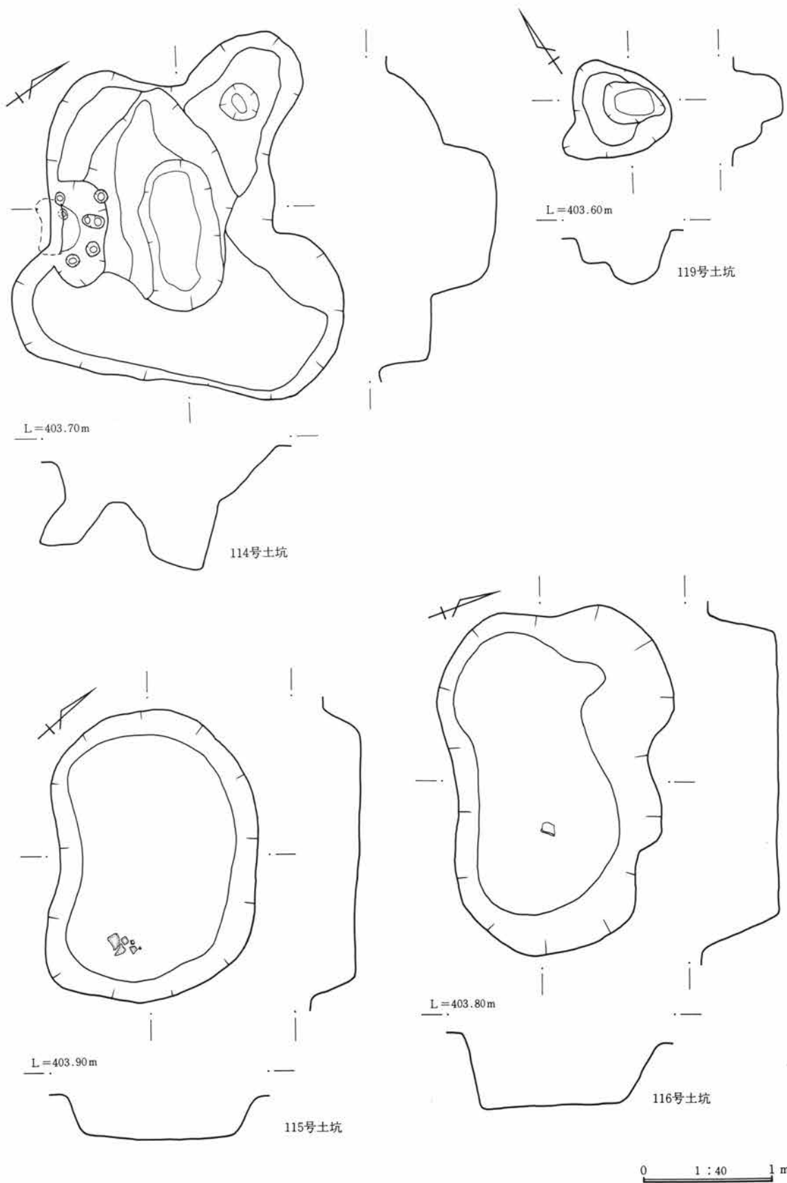
第509图 土坑实测图
