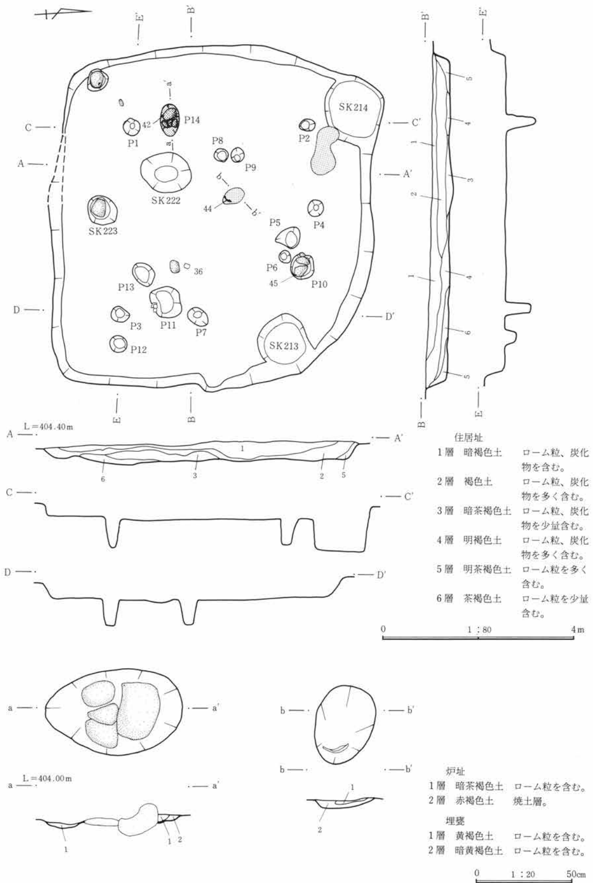
第410図 136号住居址・炉址実測図
