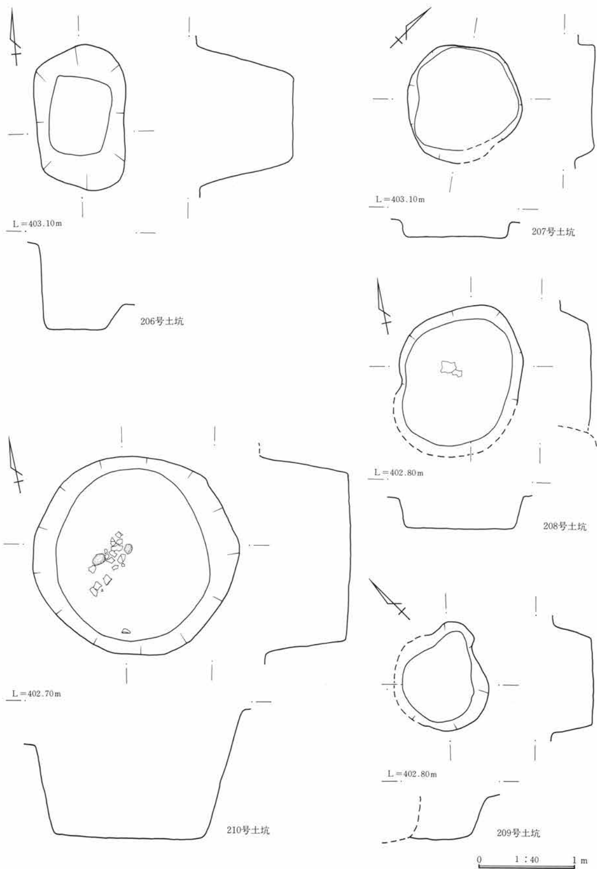
第527图 土坑实测图
