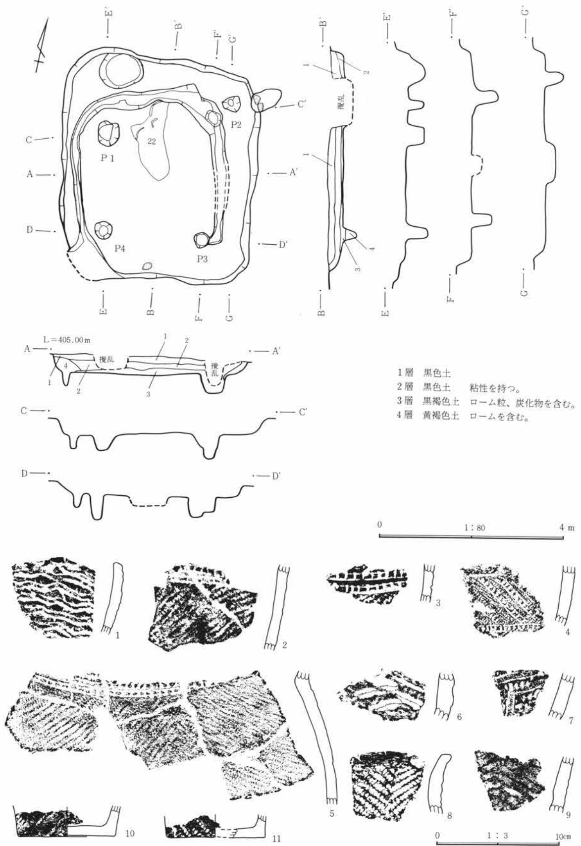
第2図 2号住居址実測図・出土遺物図
