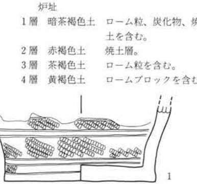
第335図 121号a・b住居址・炉址実測図・出土遺物図
