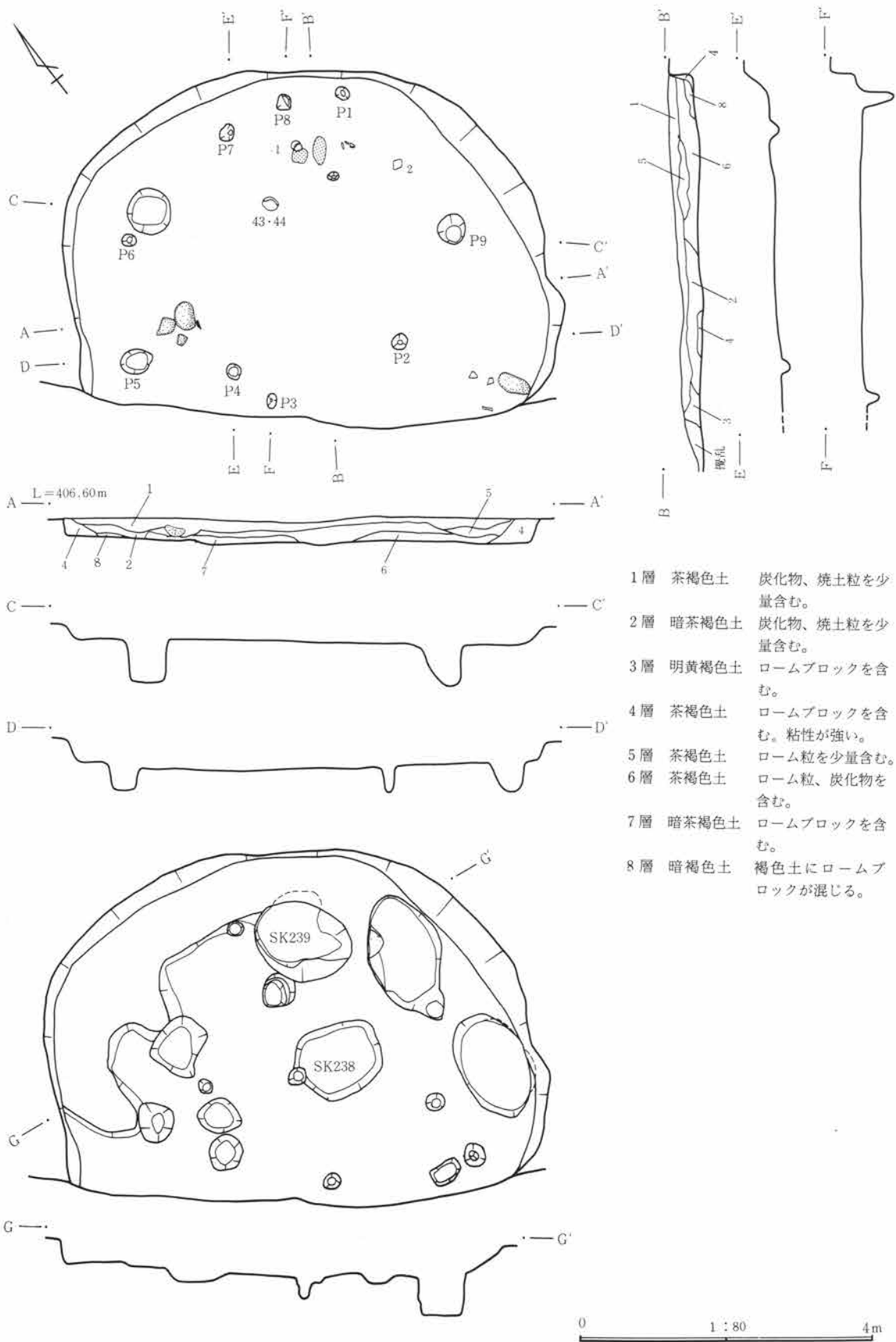
第52図 65号住居址実測図
