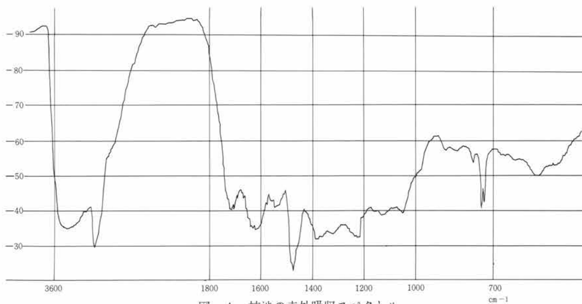
図-4 柿渋の赤外吸収スペクトル
