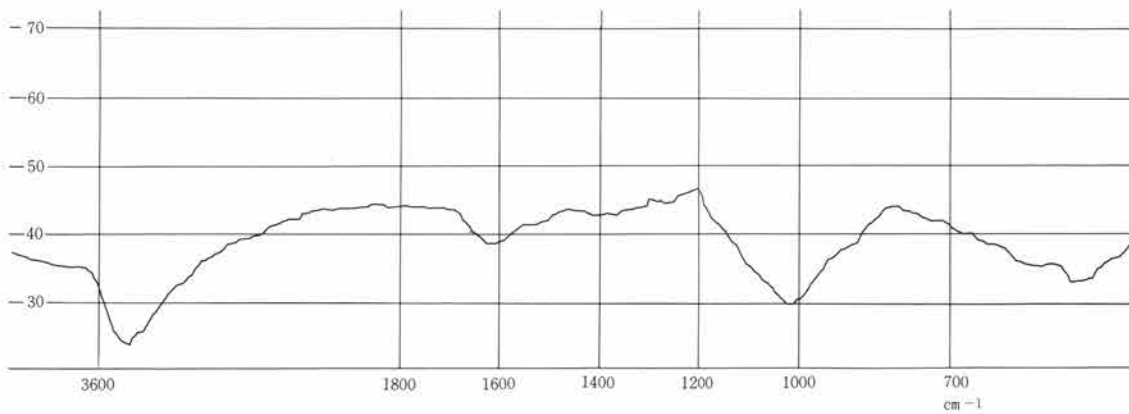
図-2 褐色膜状部分の表面を削りとった試料の赤外吸収スペクトル
