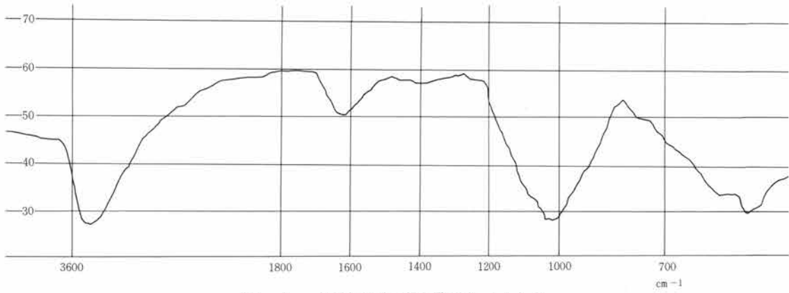
図-1 土器素地の赤外吸収スペクトル
