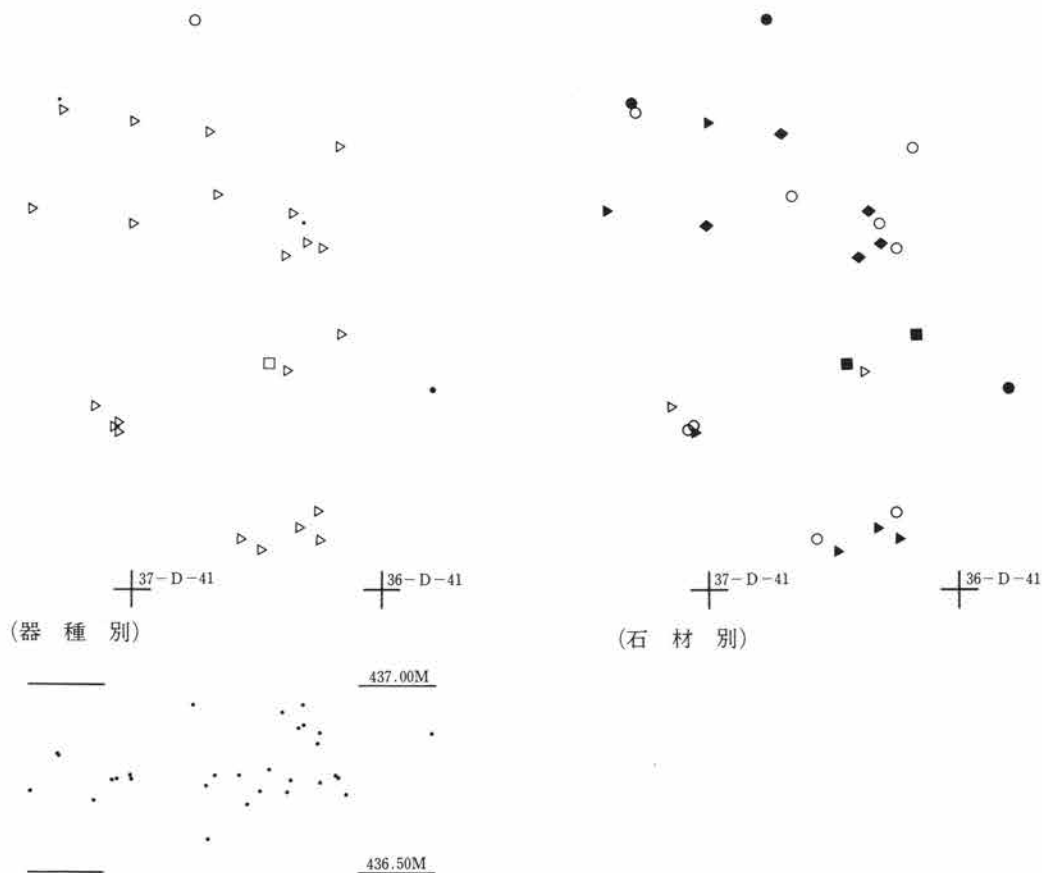
第195図 第31ブロック水平・垂直分布図 (1/60)
