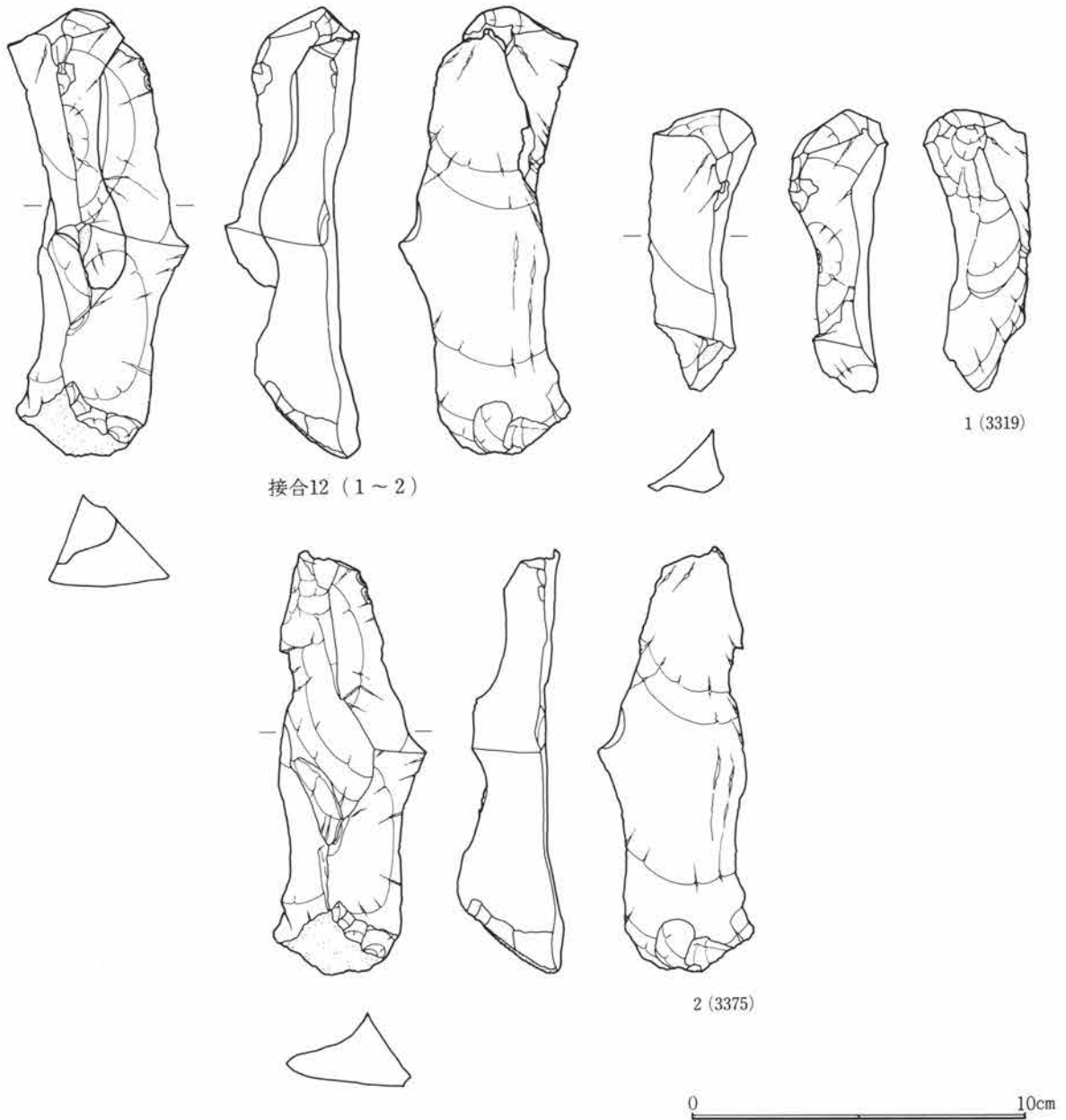
第123図 接合資料12
