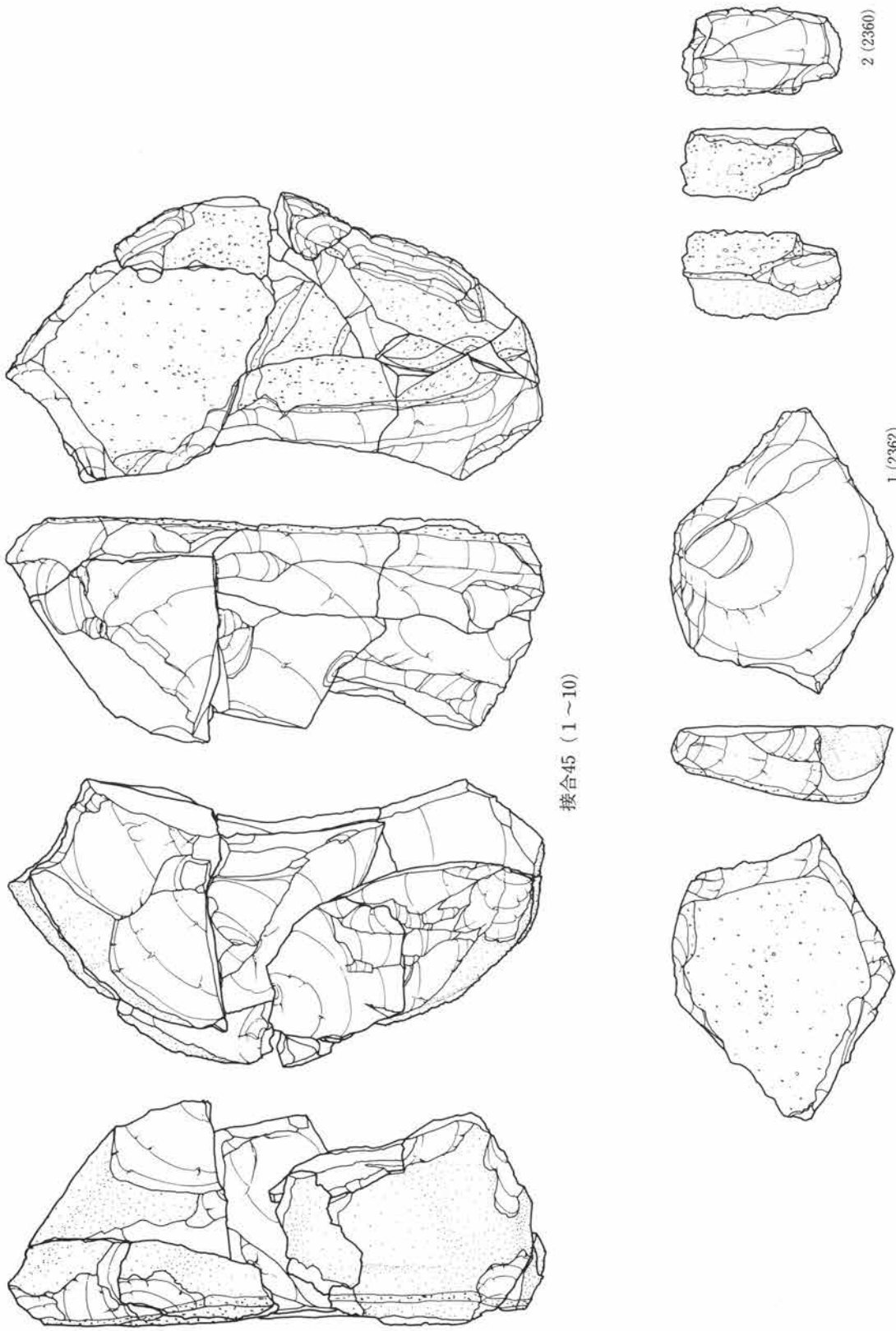
第170図 接合資料45-①
