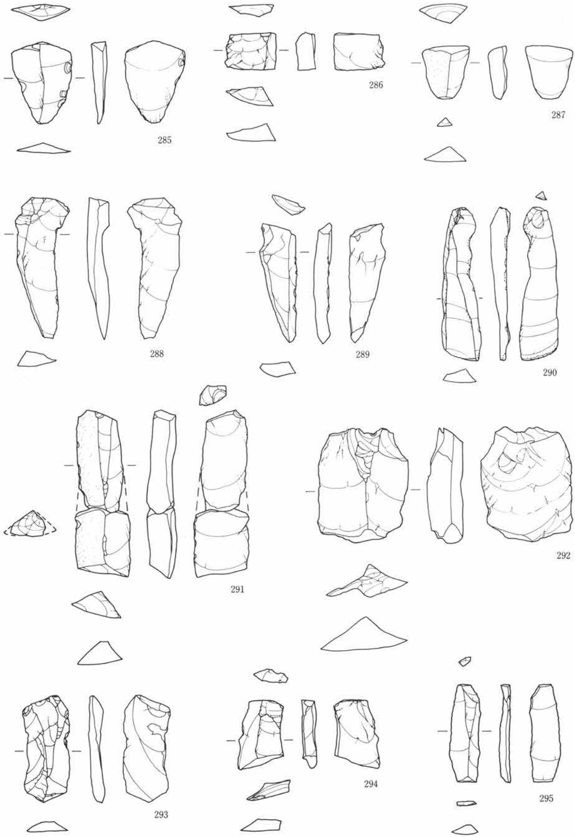
第52図 石刃状剥片(7)
