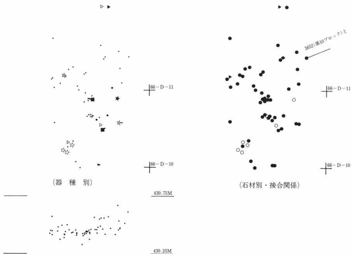
第120図 第11ブロック水平・垂直分布図（1/60）
