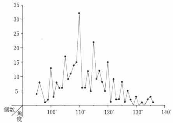
第270図 打角分布図
