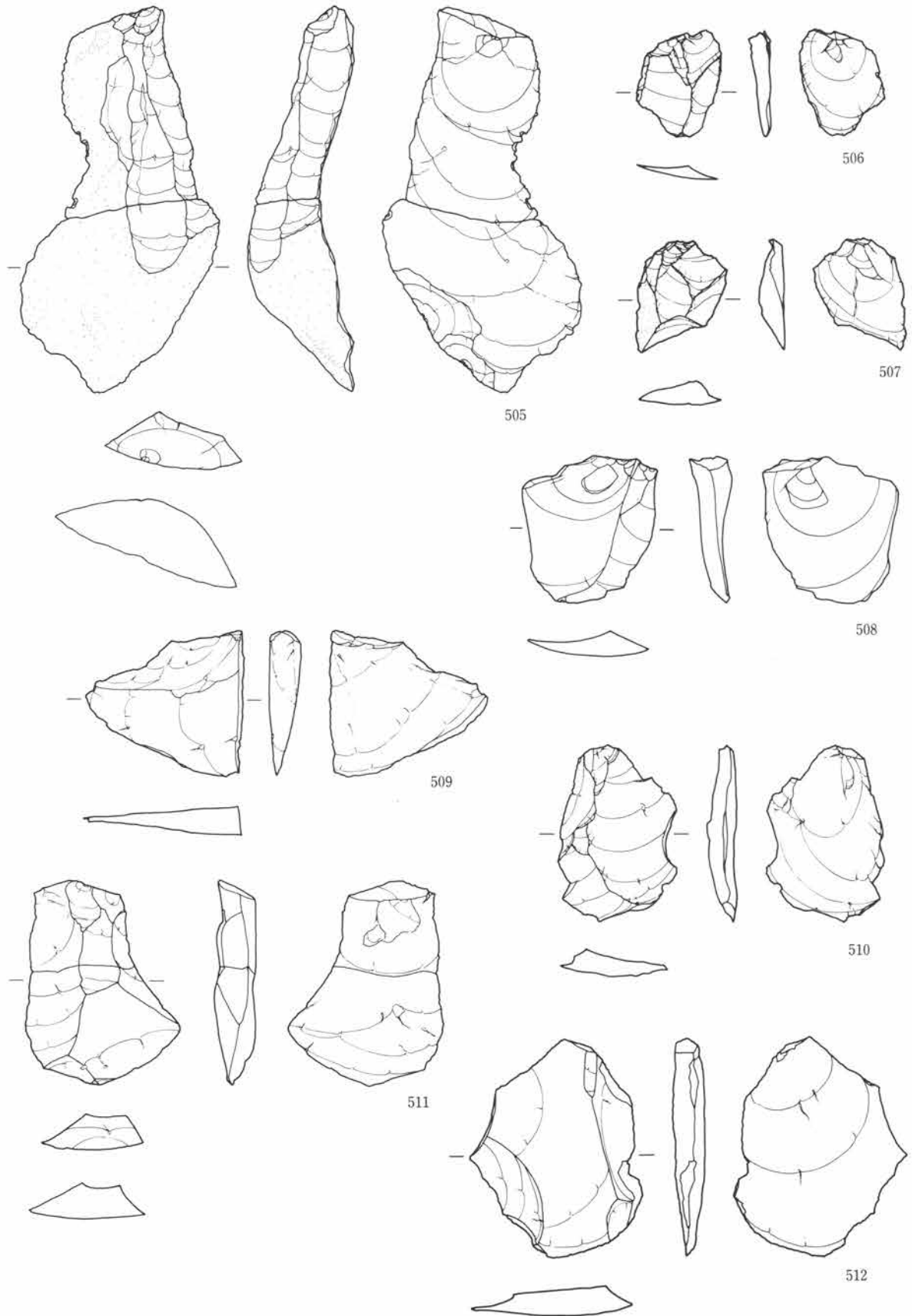
第75図 剥片 (3)
