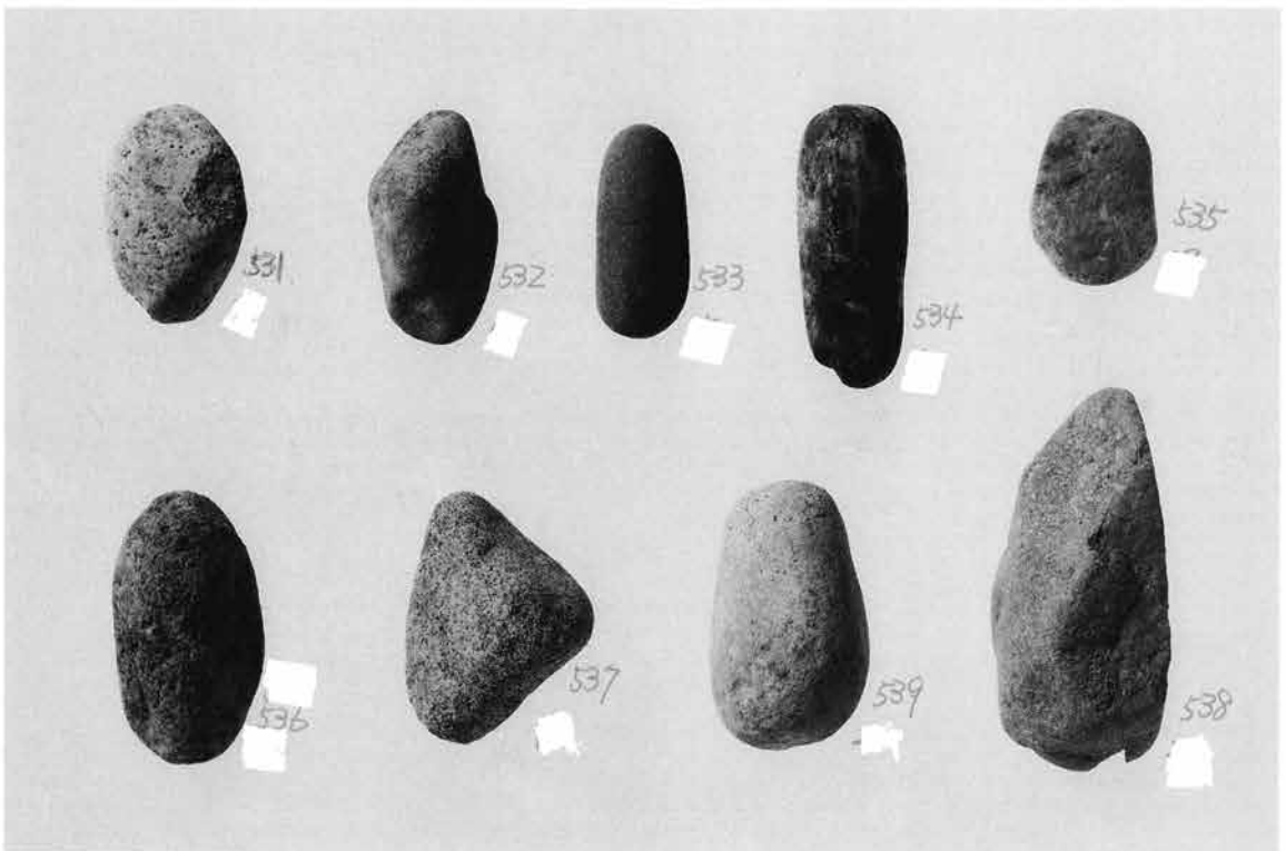
2. 敲石 (1)
