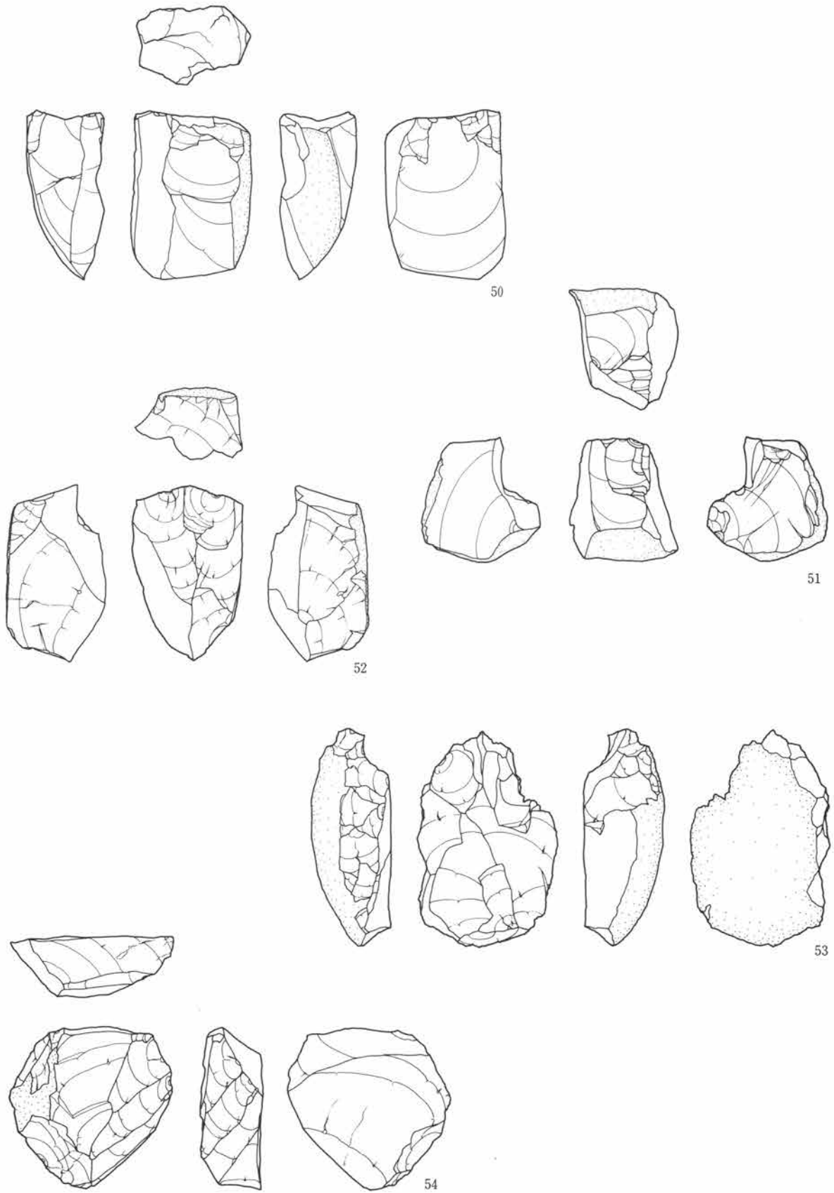
第20図 石核 (1)
