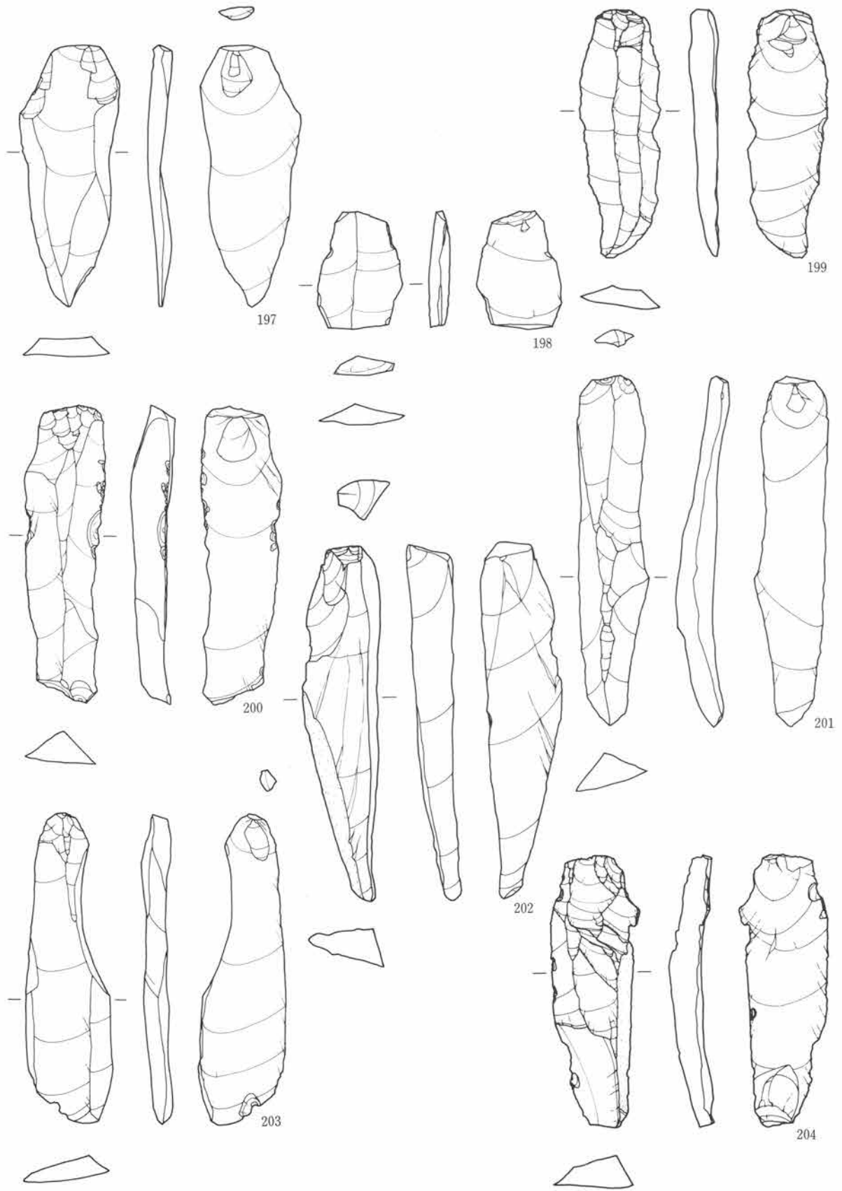
第43図 石 刃 (4)
