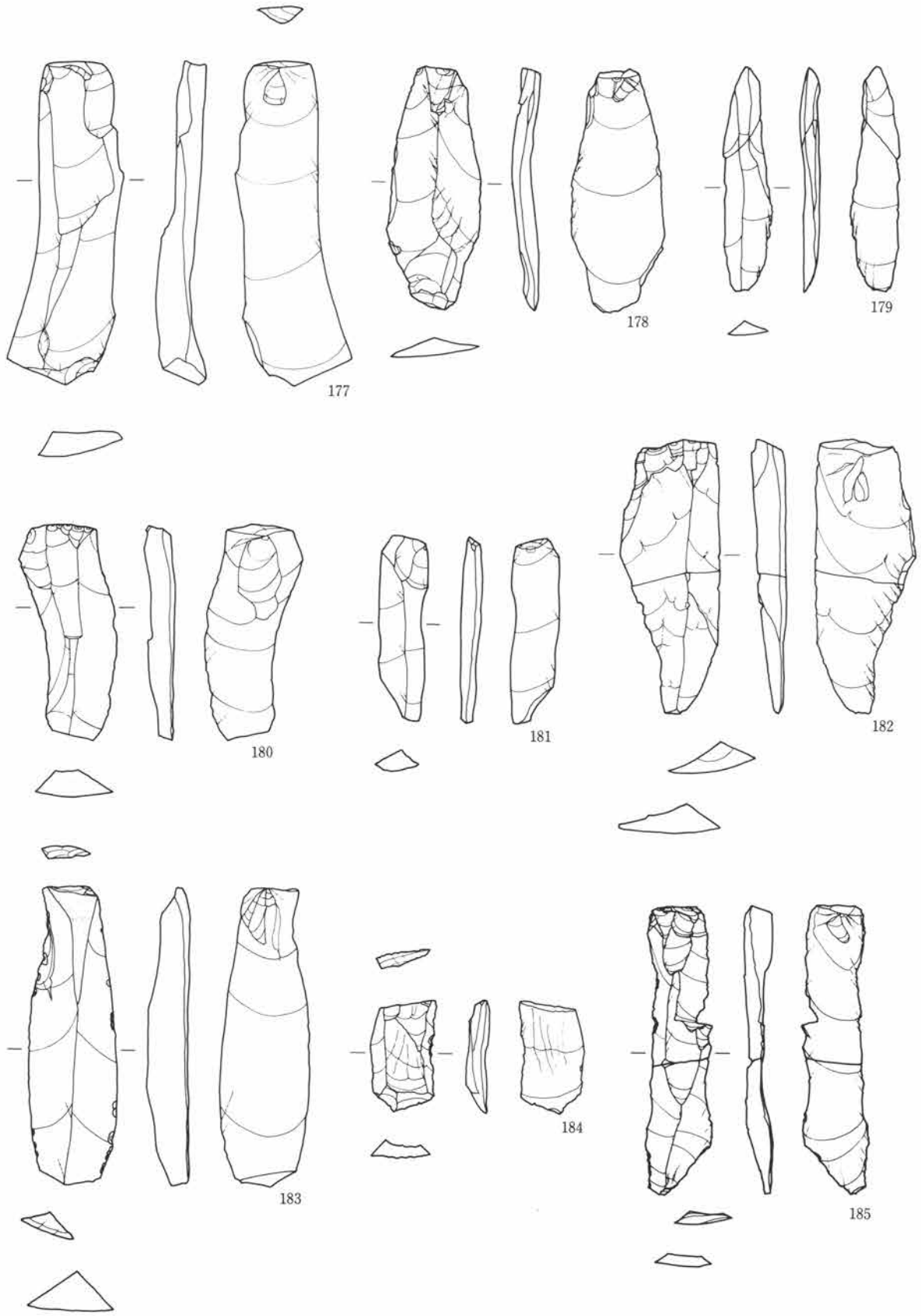
第41図 石刃 (2)
