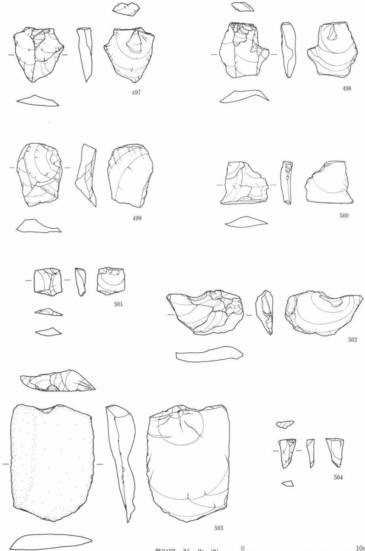
第74図 剥片 (2)
