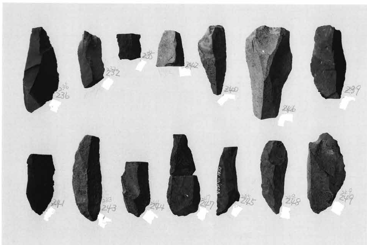
1. 石刃状剥片 (2)
