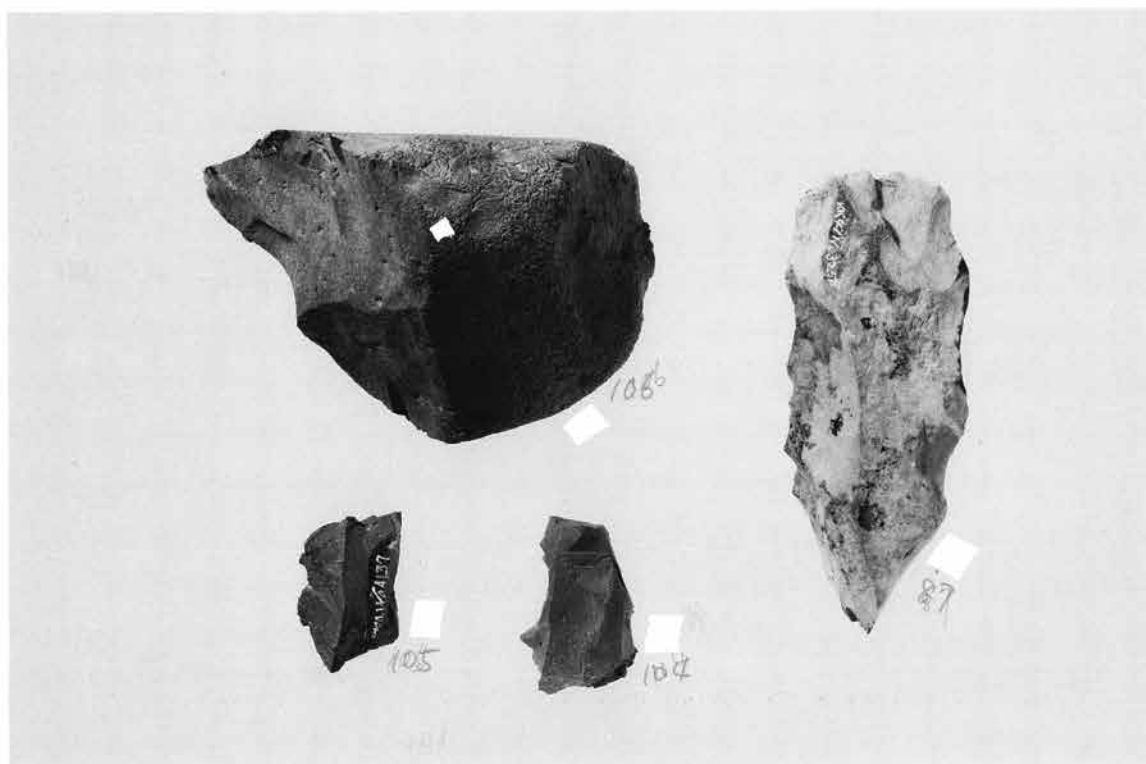
2. 石核 (9)
