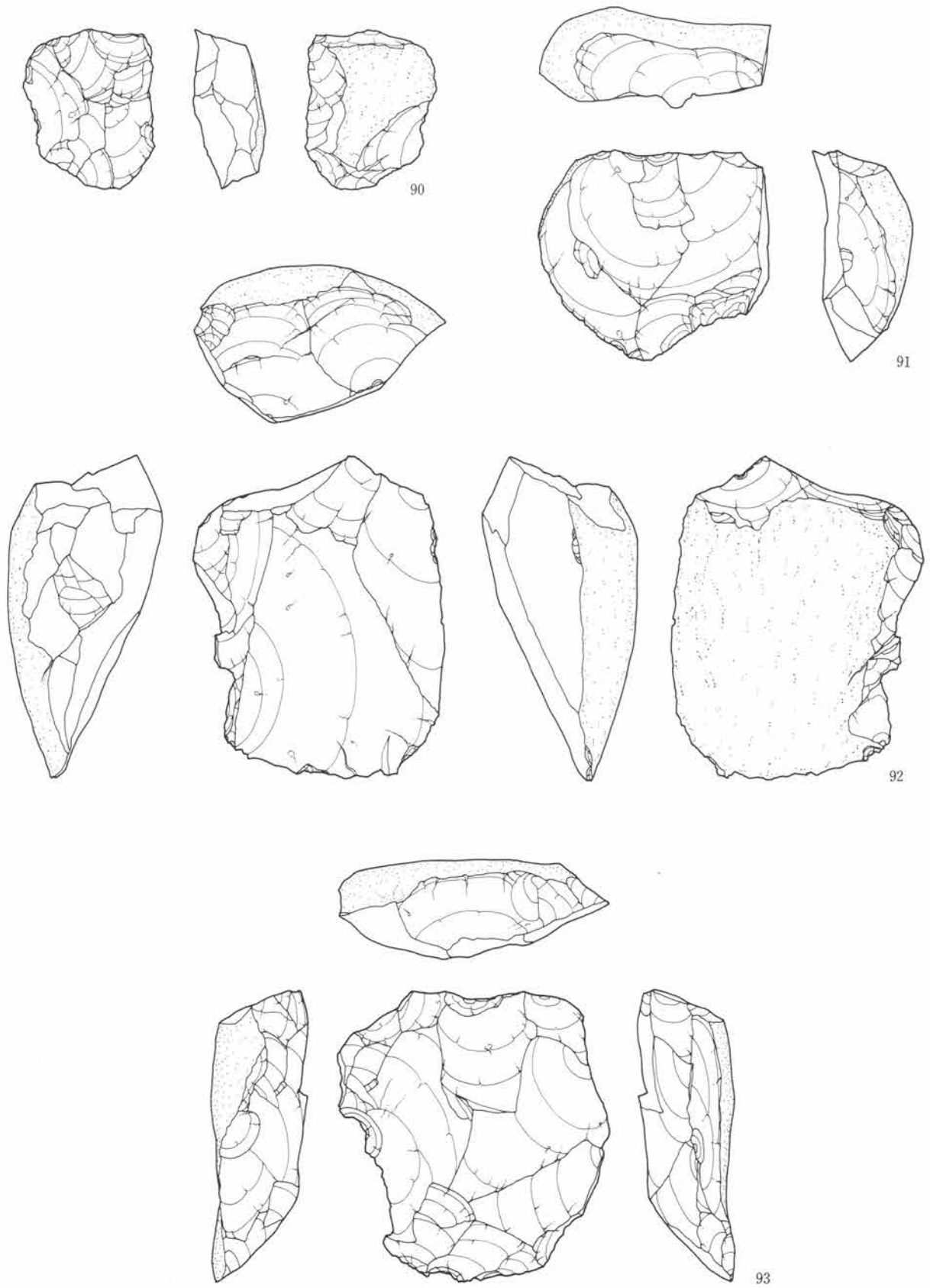
第29図 石核 (10)
