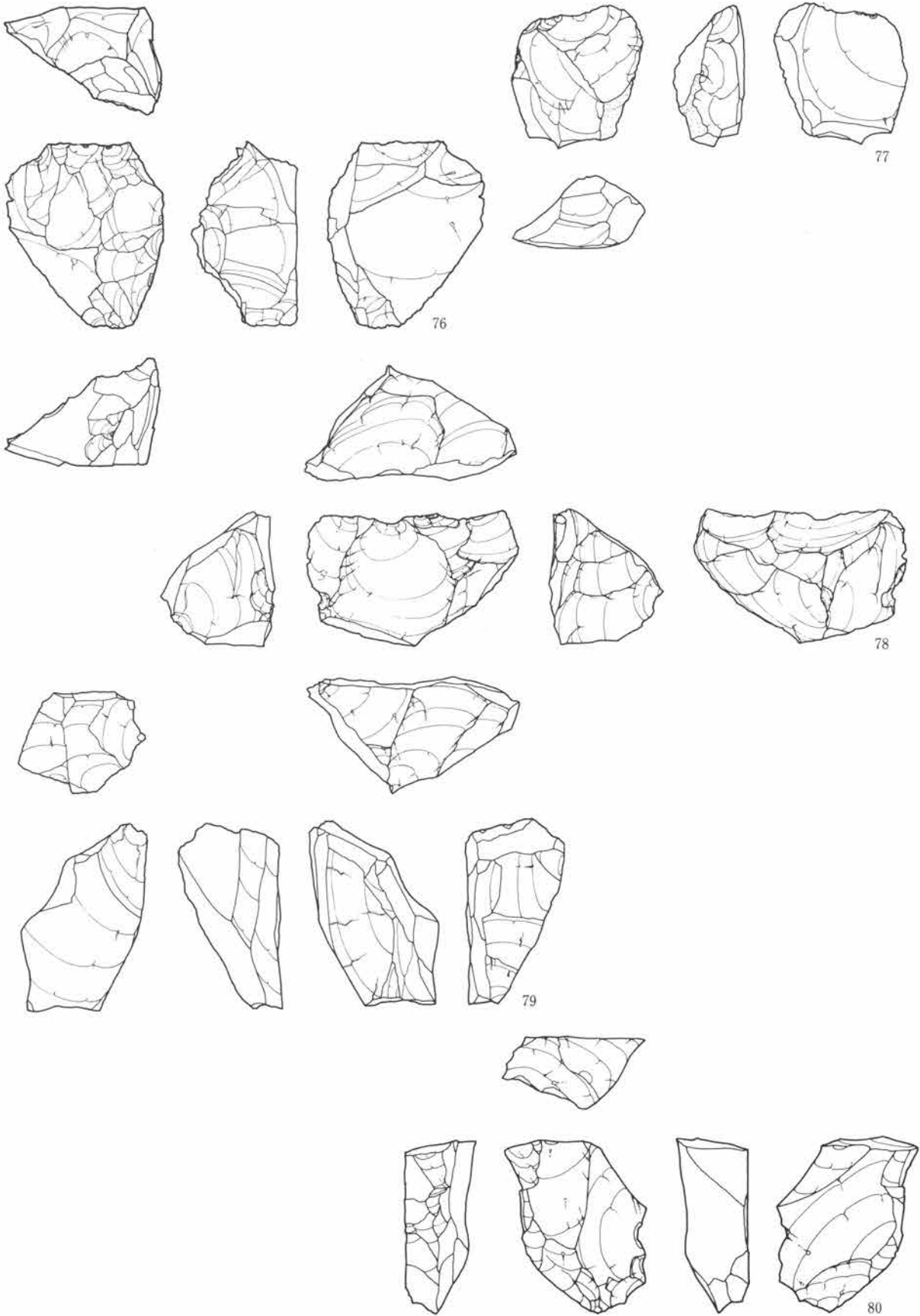
第26図 石核 (7)
