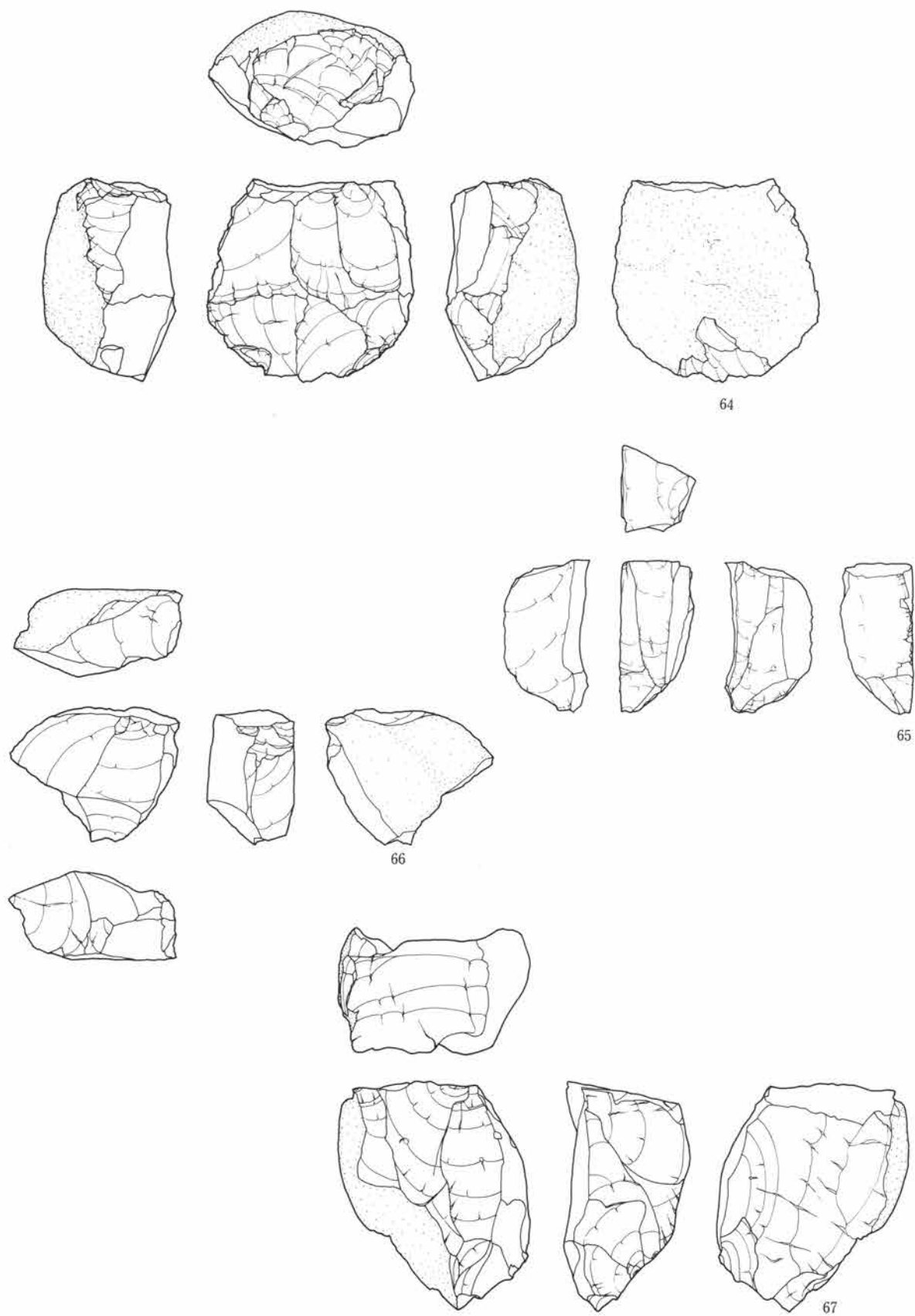
第23図 石核 (4)
