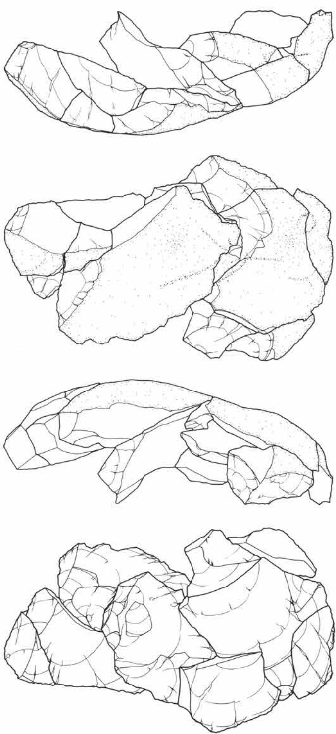
接合17 (1~10)
