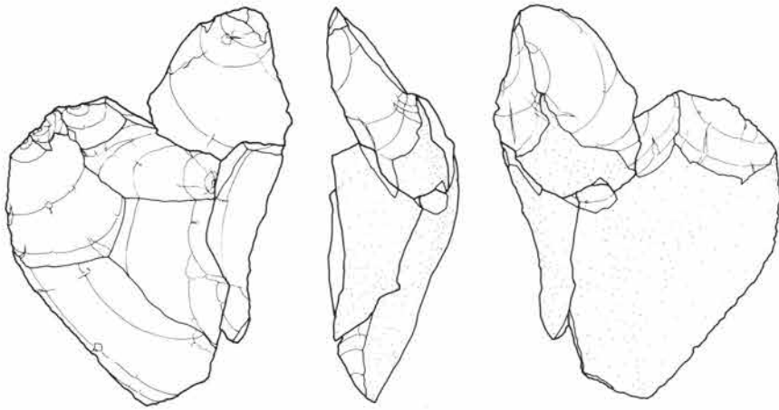
接合30 (1~3)
