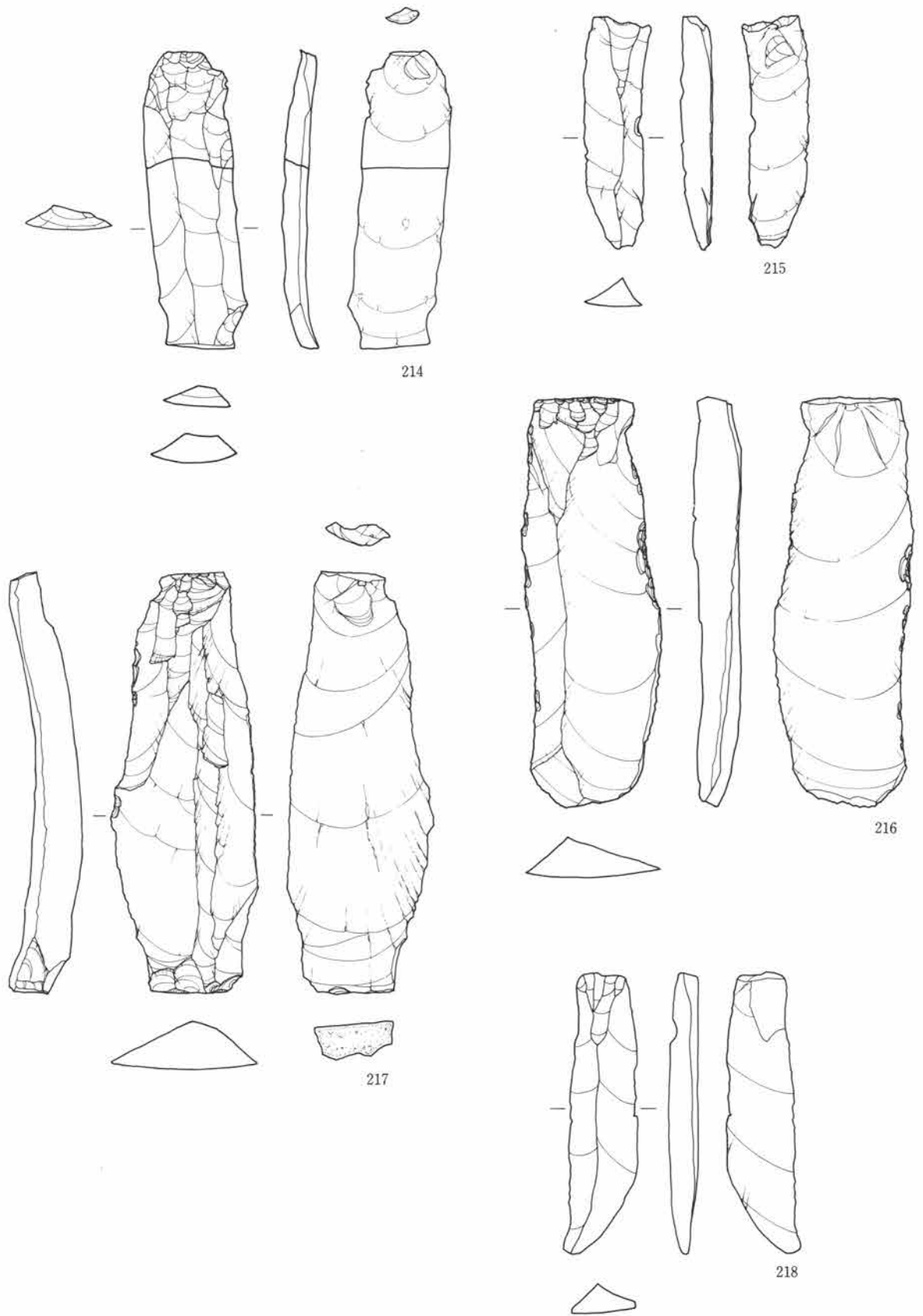
第45図 石 刃 (6)
