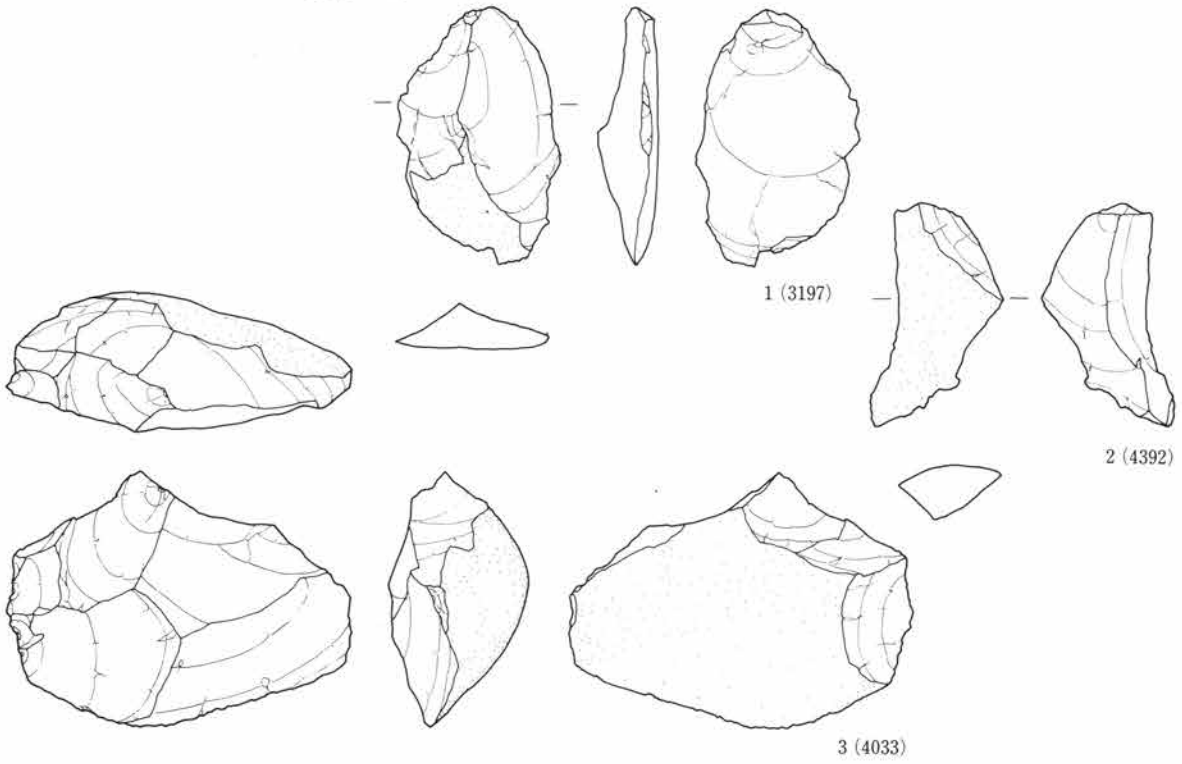
接合30 (1~3)
