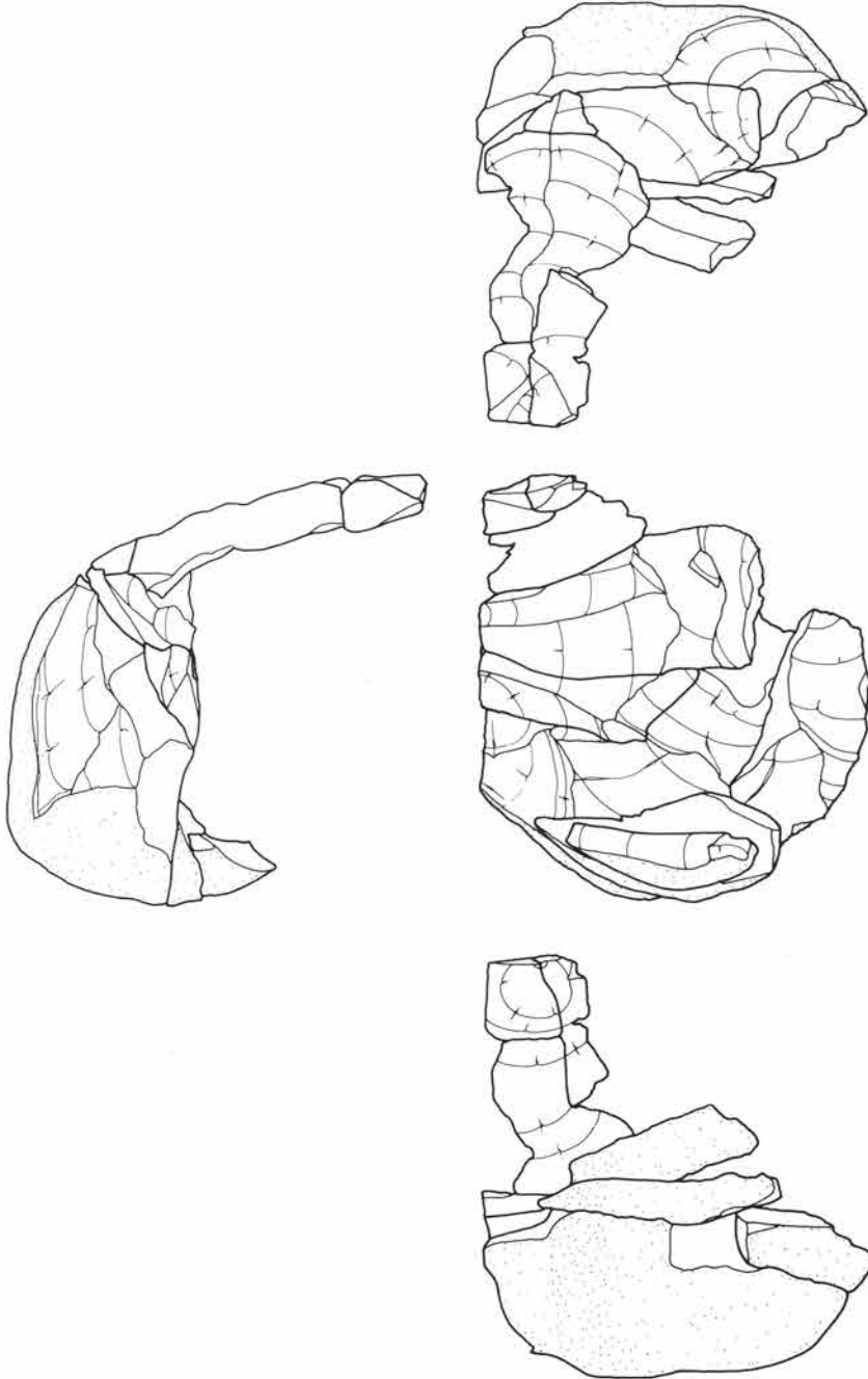
接合58 (1~10)
