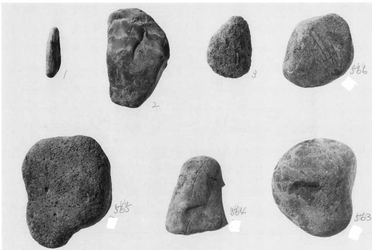
1. 敲石 (4) ・原石
