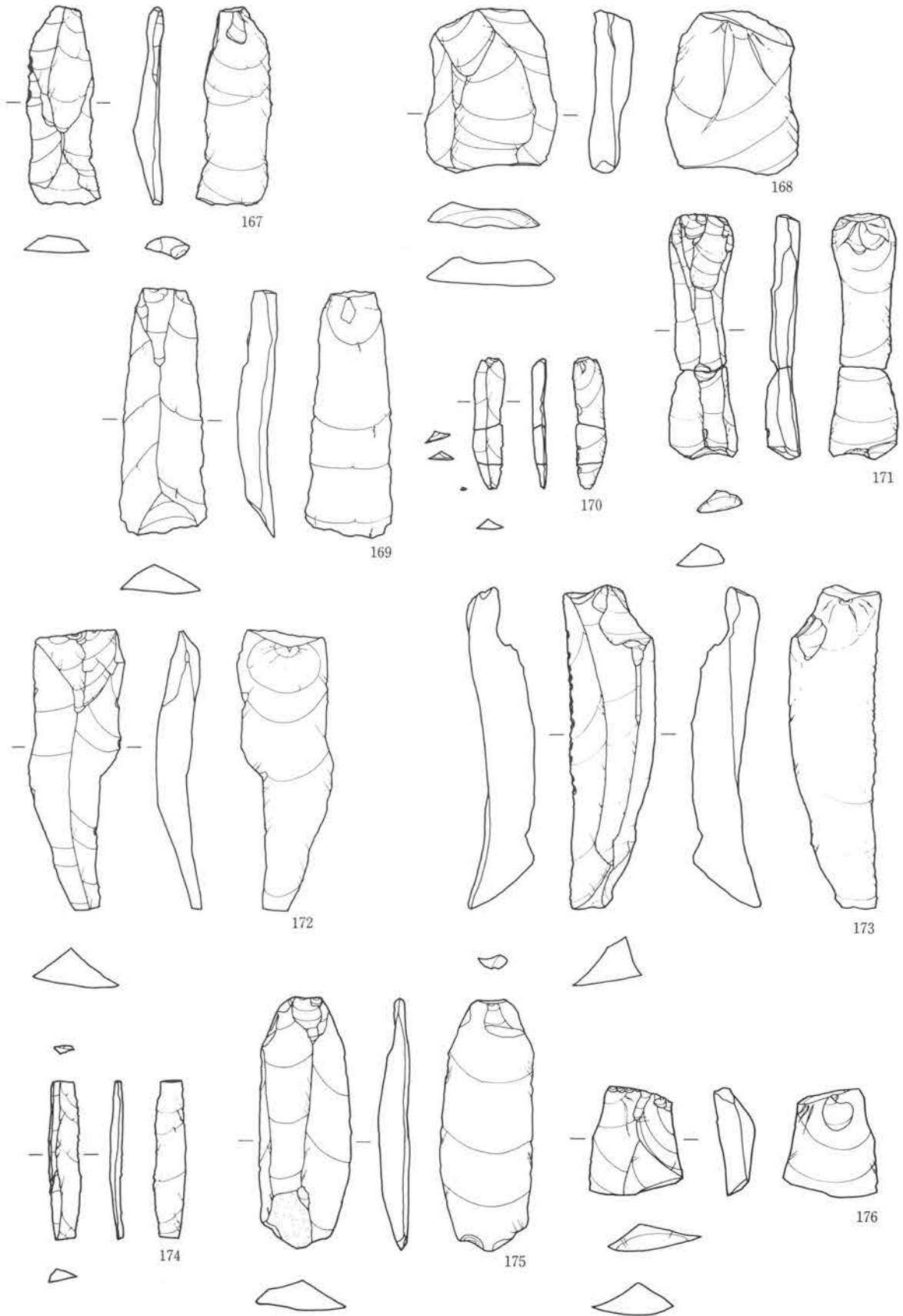
第40図 石 刃 (1)
