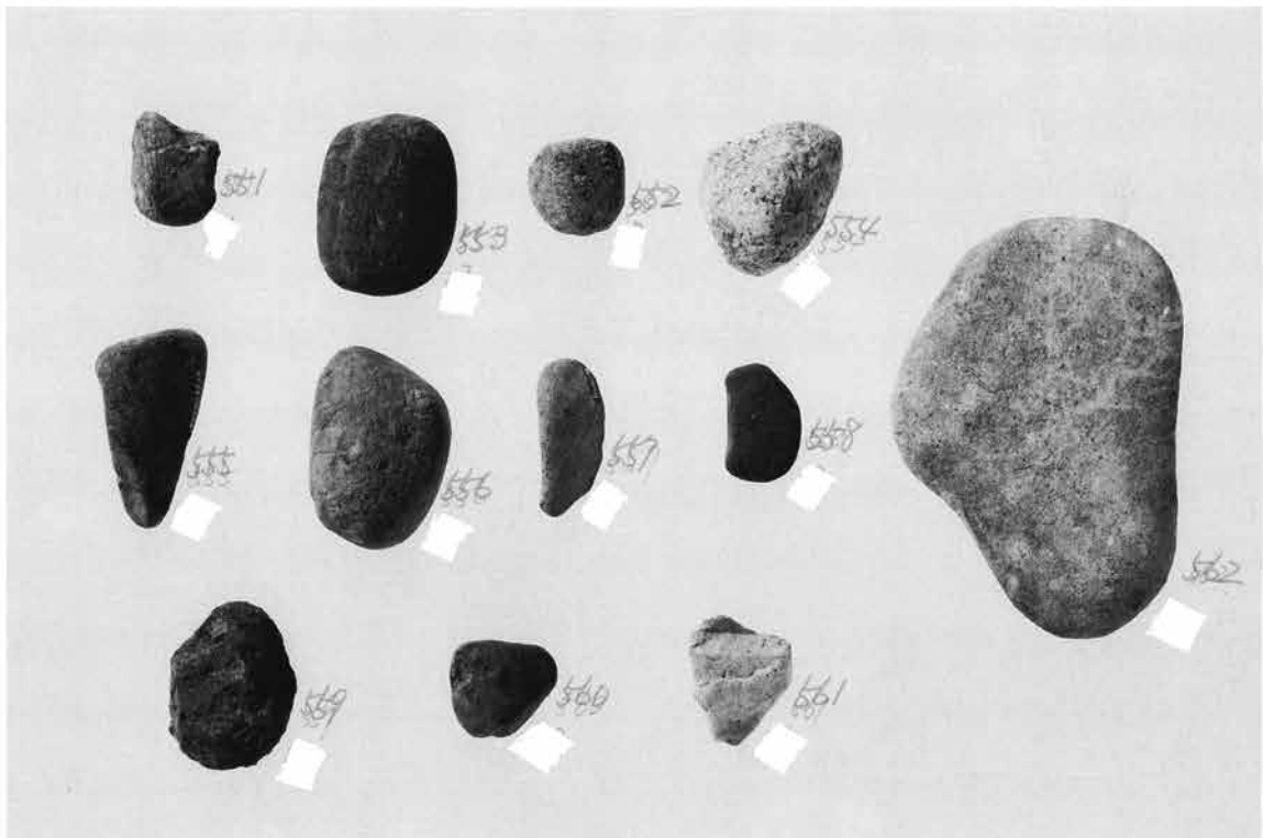
2. 敲石 (3)
