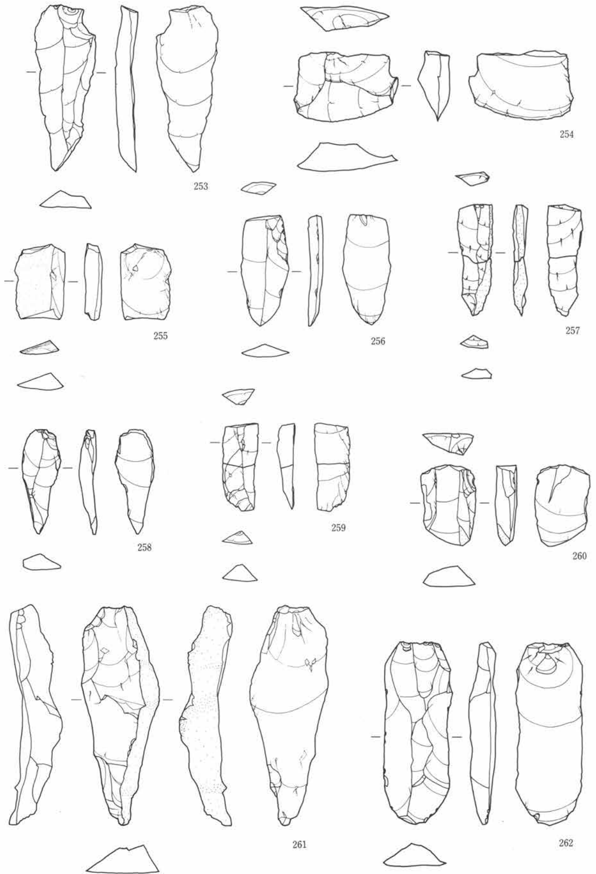
第49図 石刃状剥片(4)
