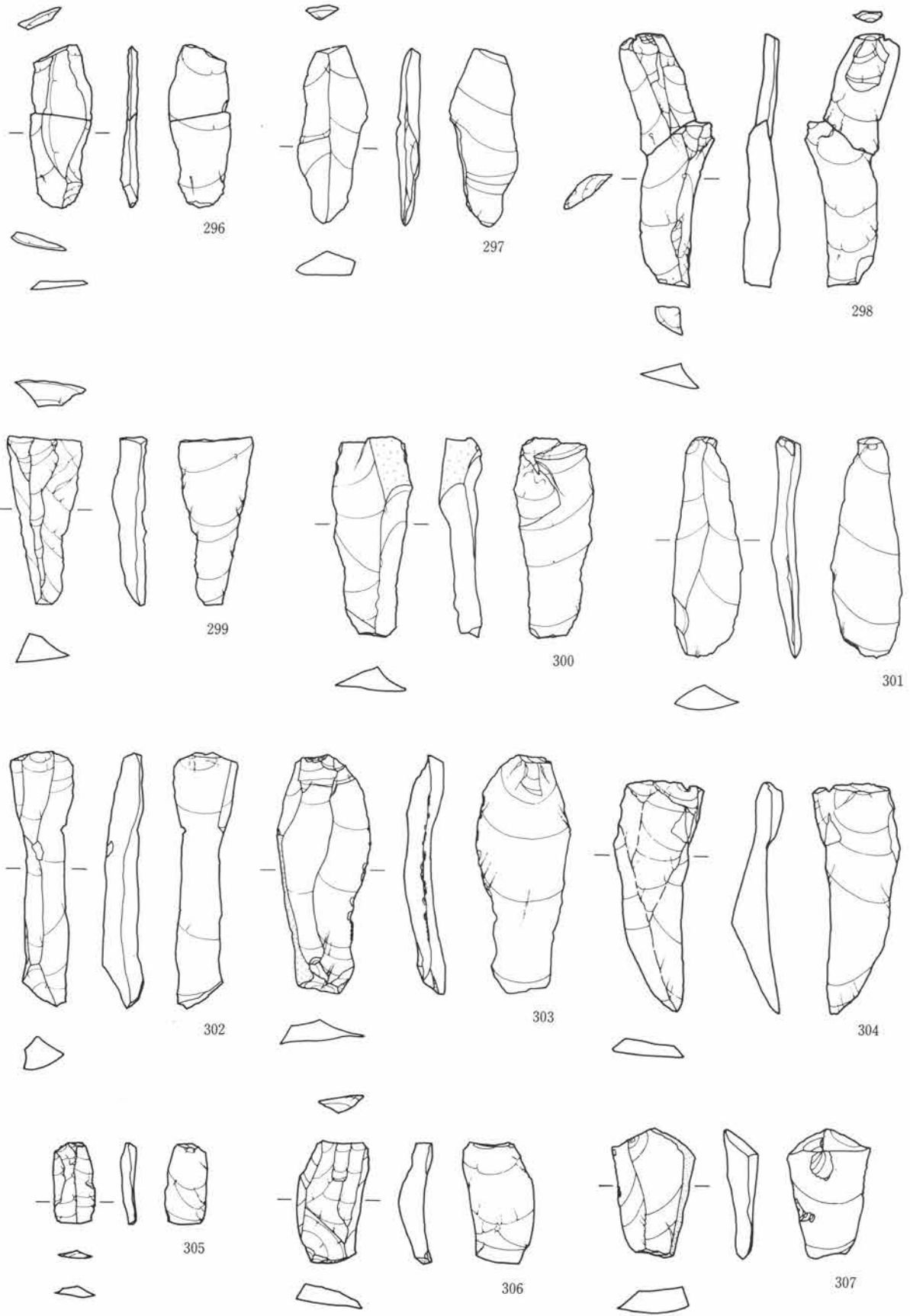
第53図 石刃状剥片(8)
