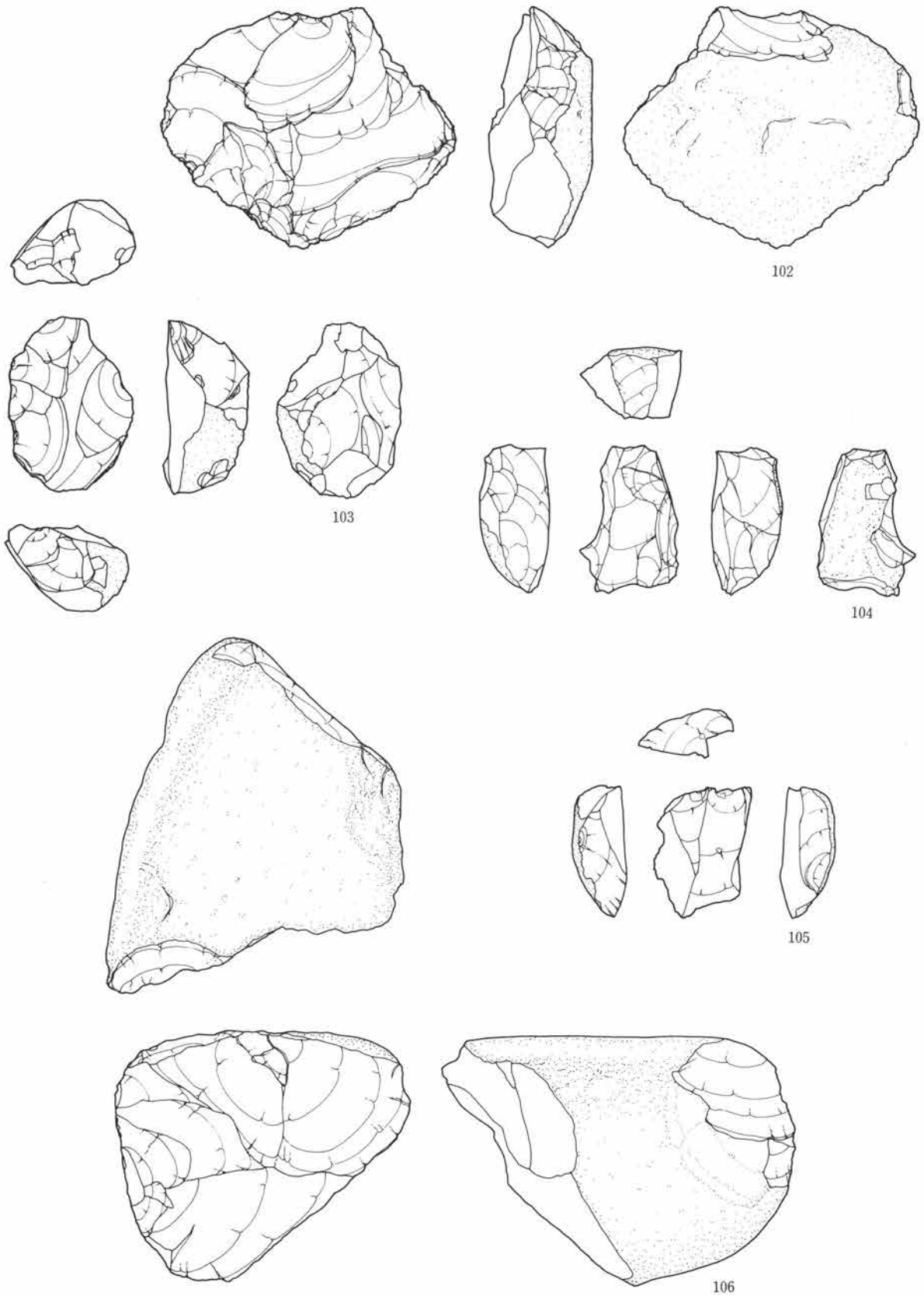
第32図 石核 (13)
