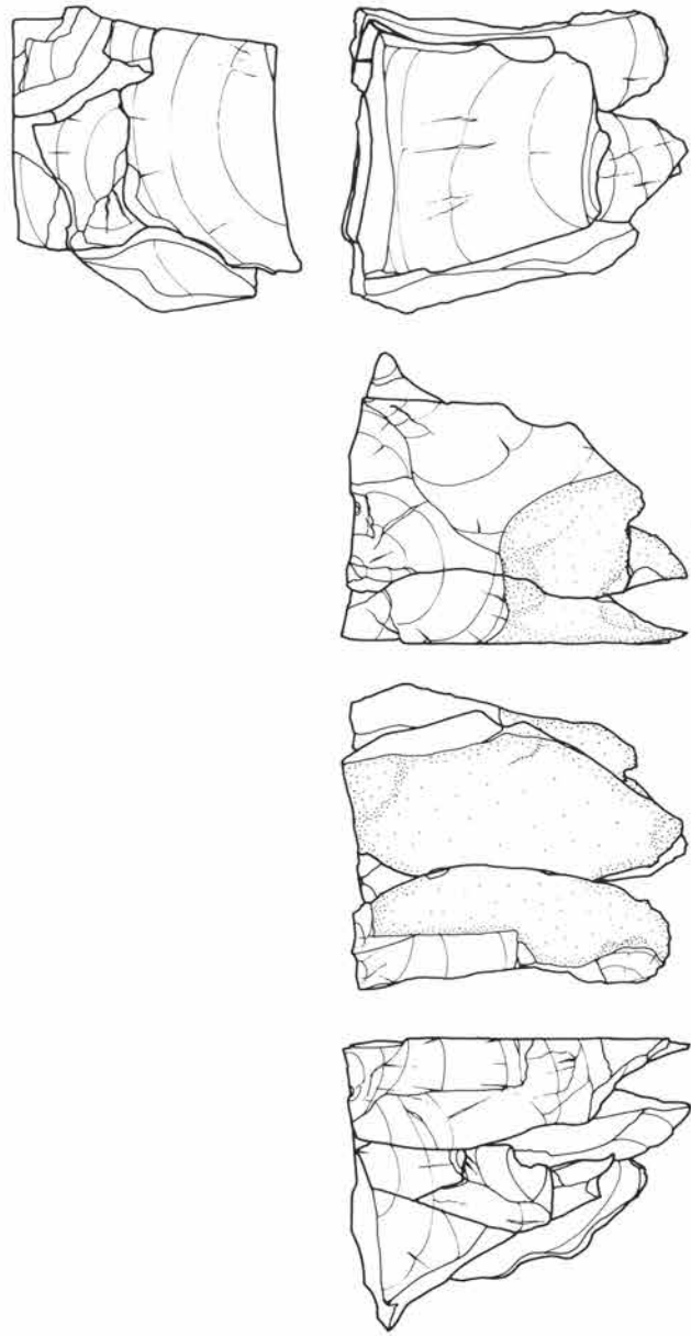
接合87 (1~7)
