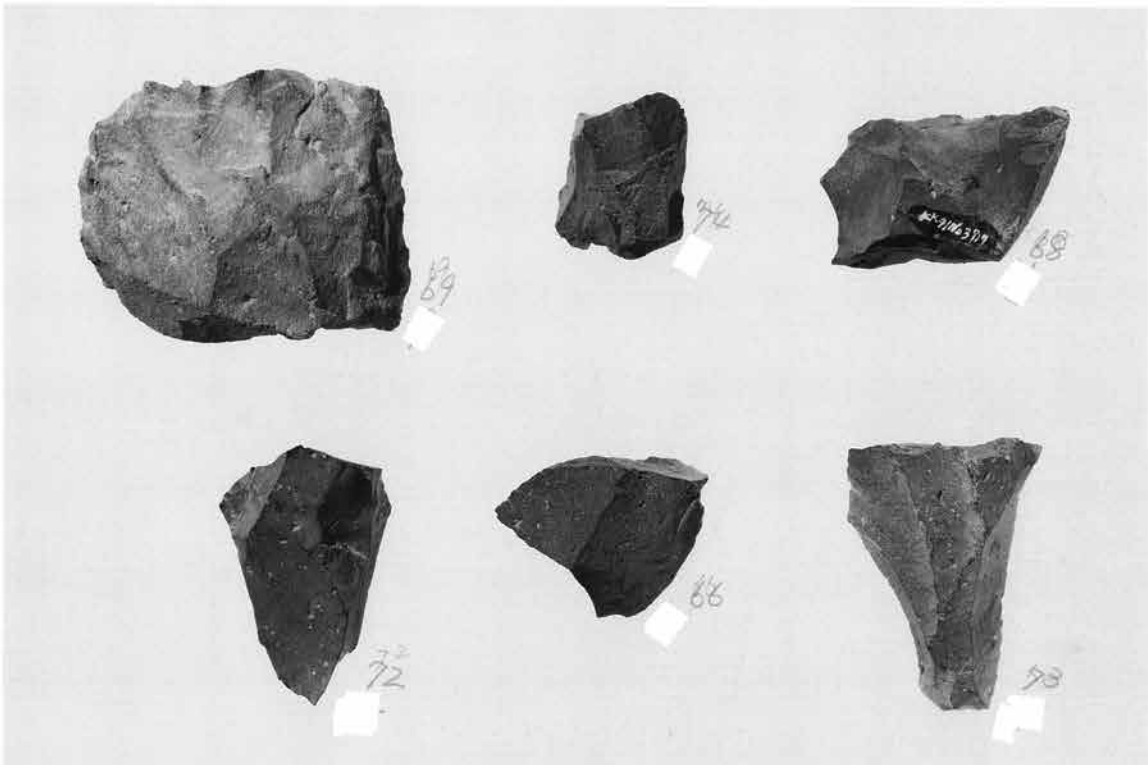
2. 石核 (3)
