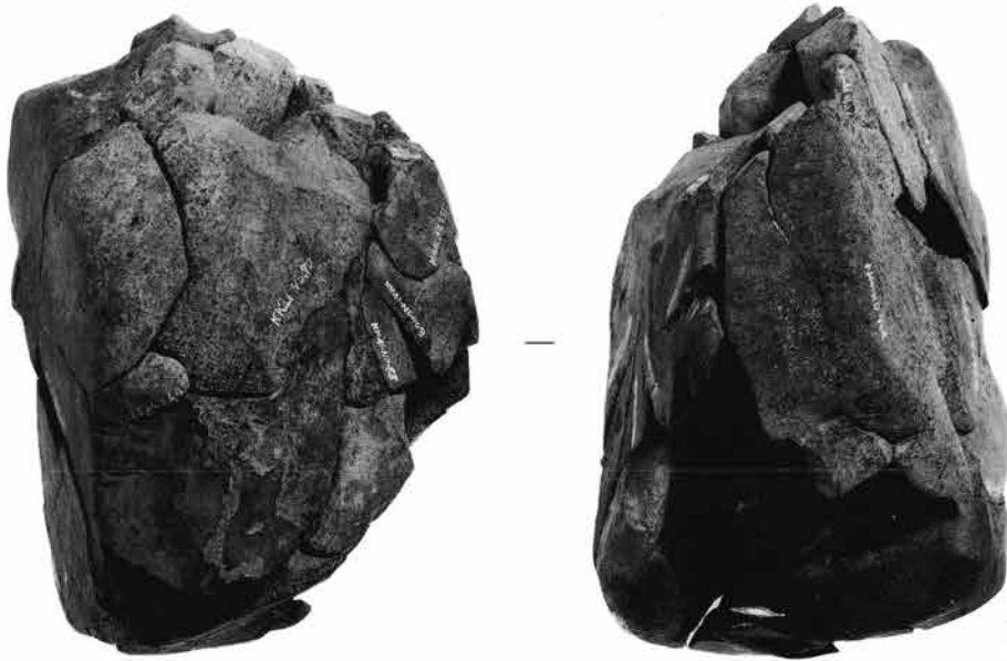
接合資料68
