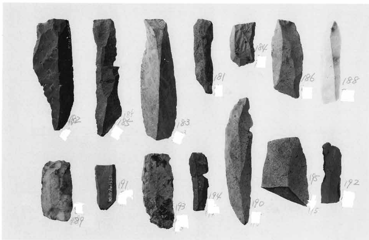
1. 石 刃 (2)
