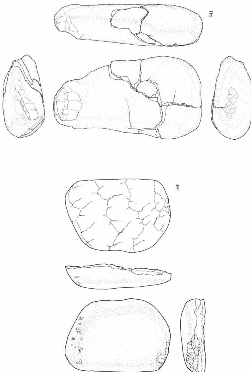
第83図 敲石 (6)
