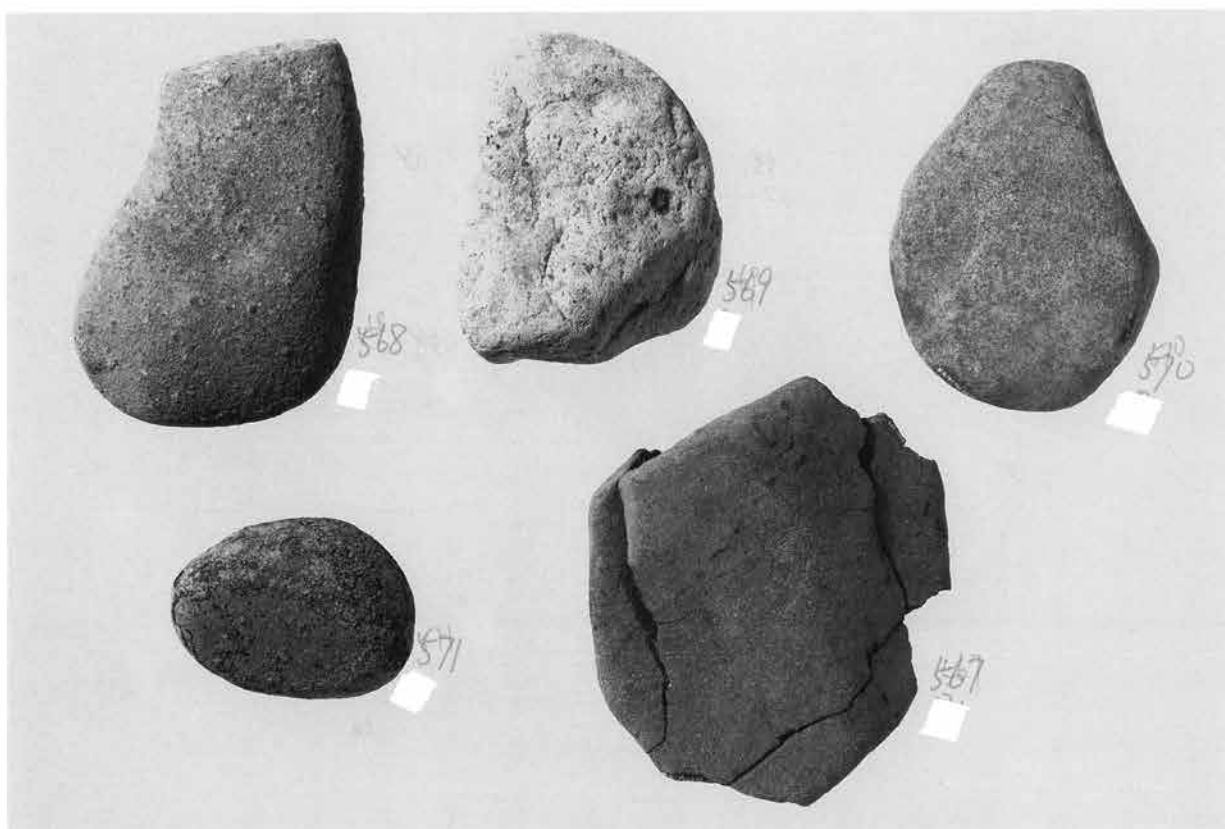
2. 台石・磨石
