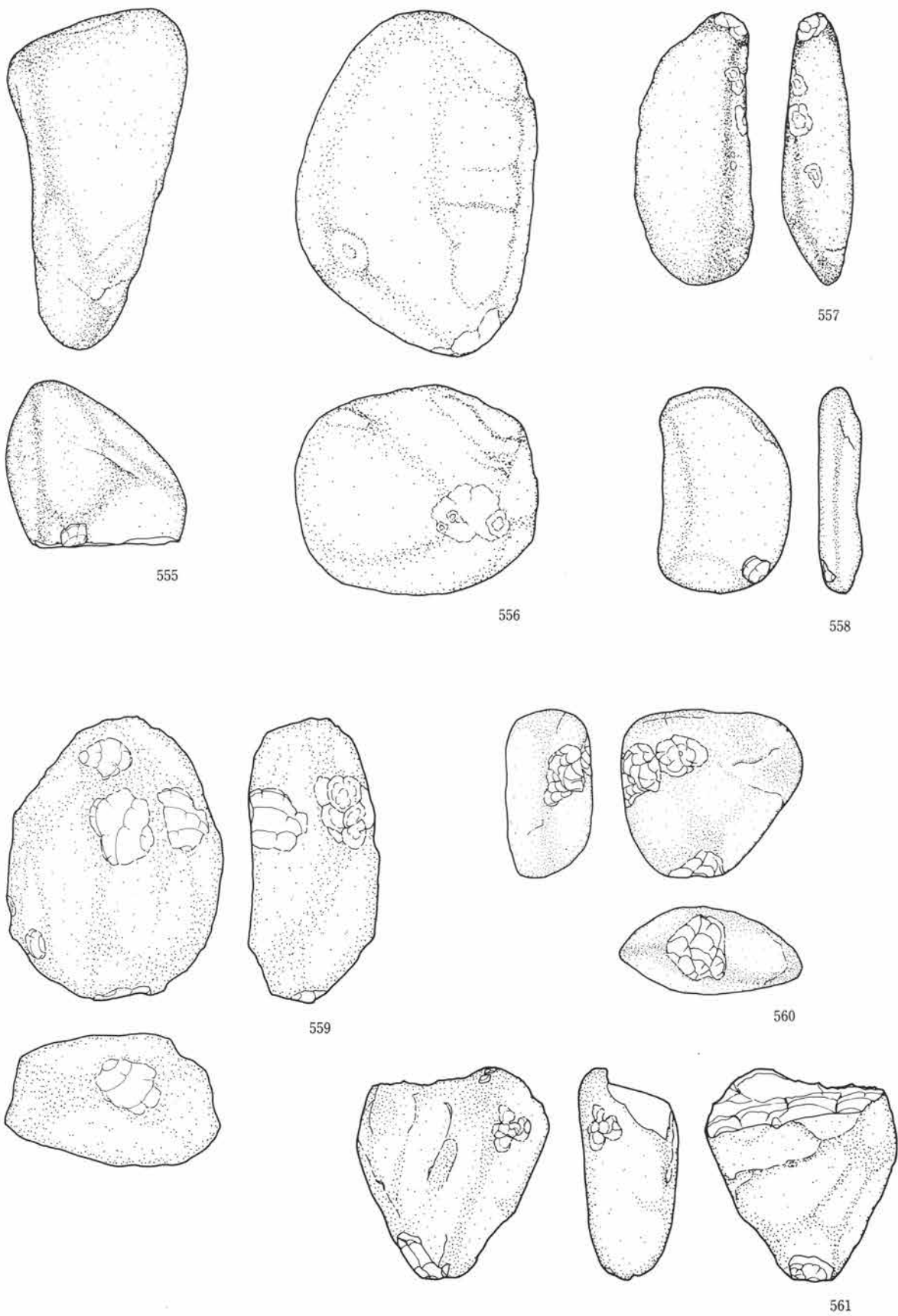
第89図 敲石 (12)
