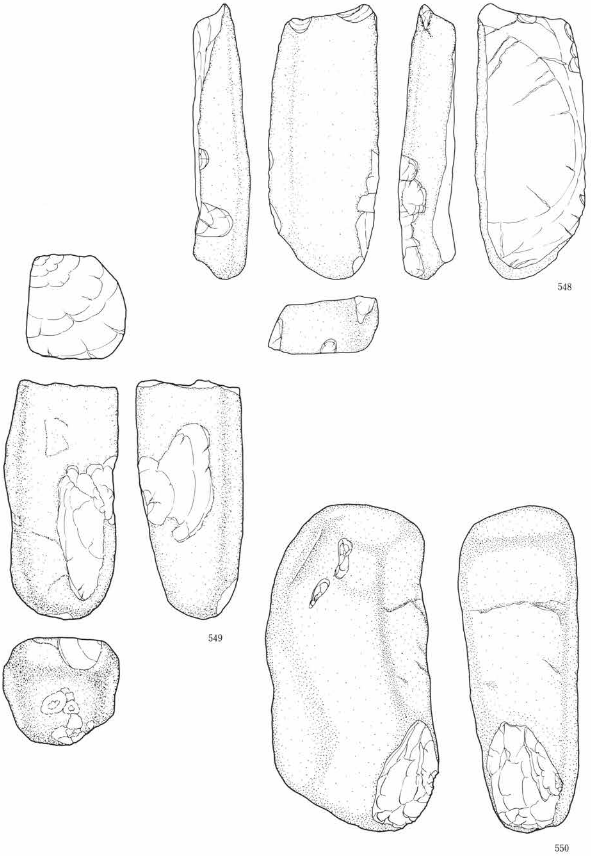
第87図 敲石 (10)
