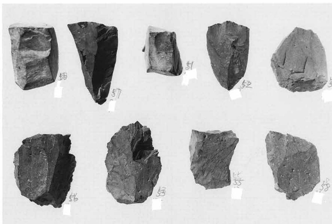
2. 石核 (1)
