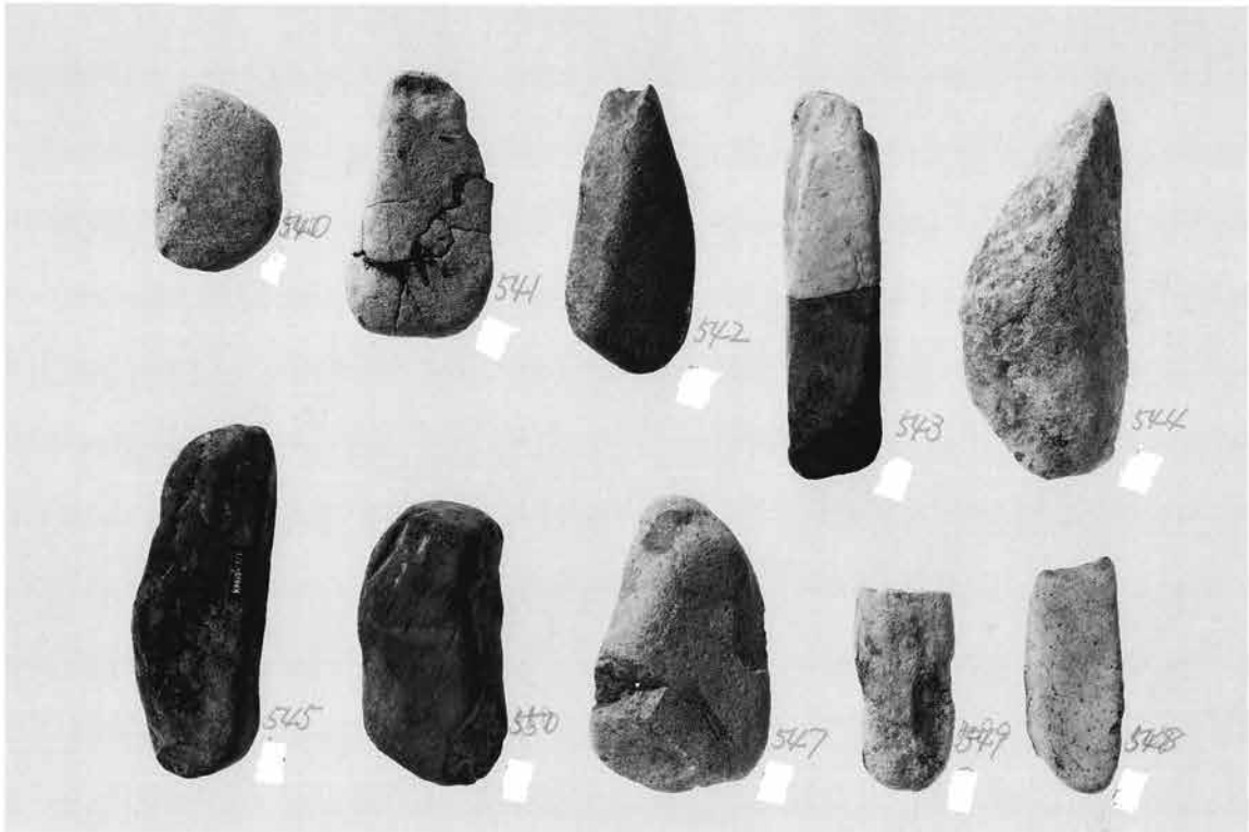
1. 敲石 (2)
