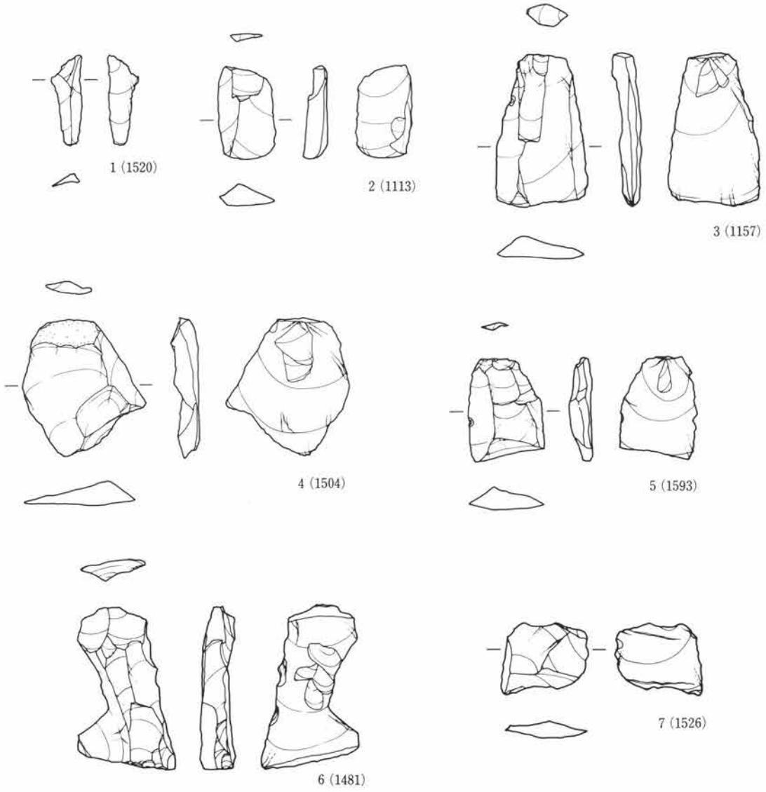
接合95 (1~7)
