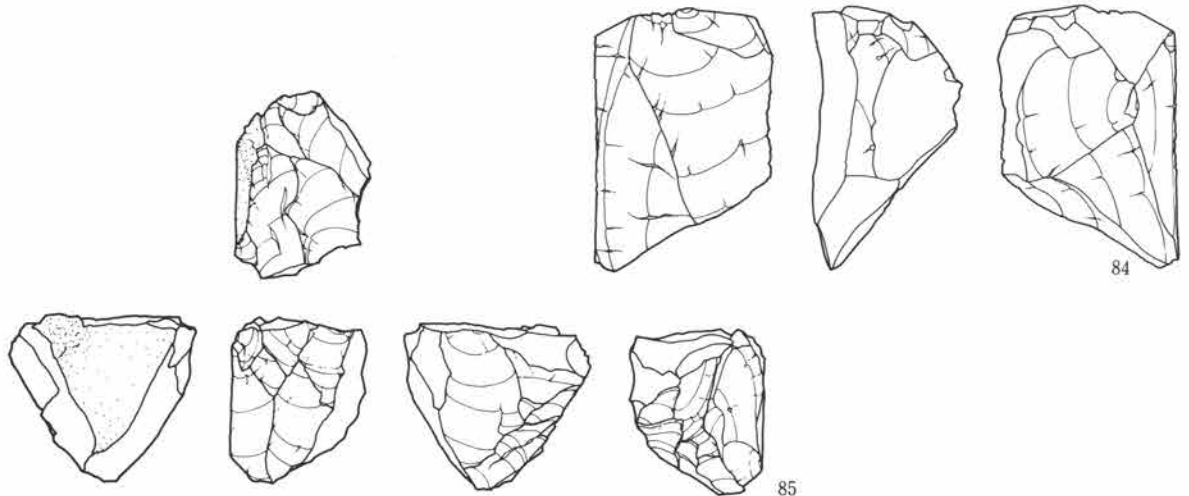
第27図 石核 (8)
