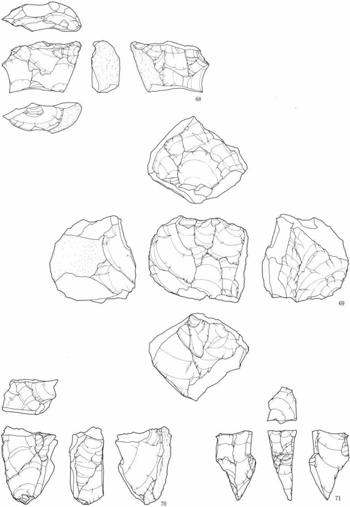
第24図 石核 (5)
