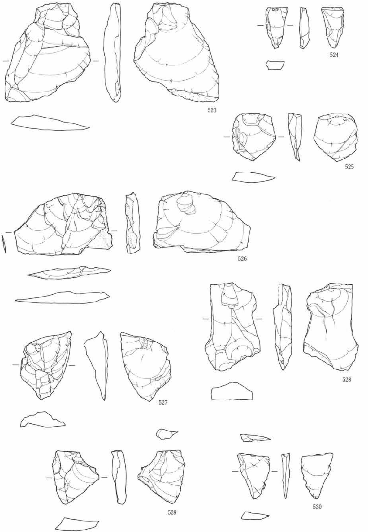
第77図 剥片 (5)
