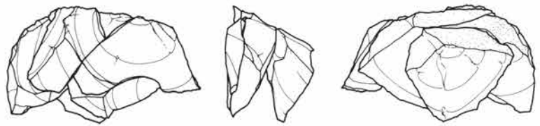
接合31 (1~5)
