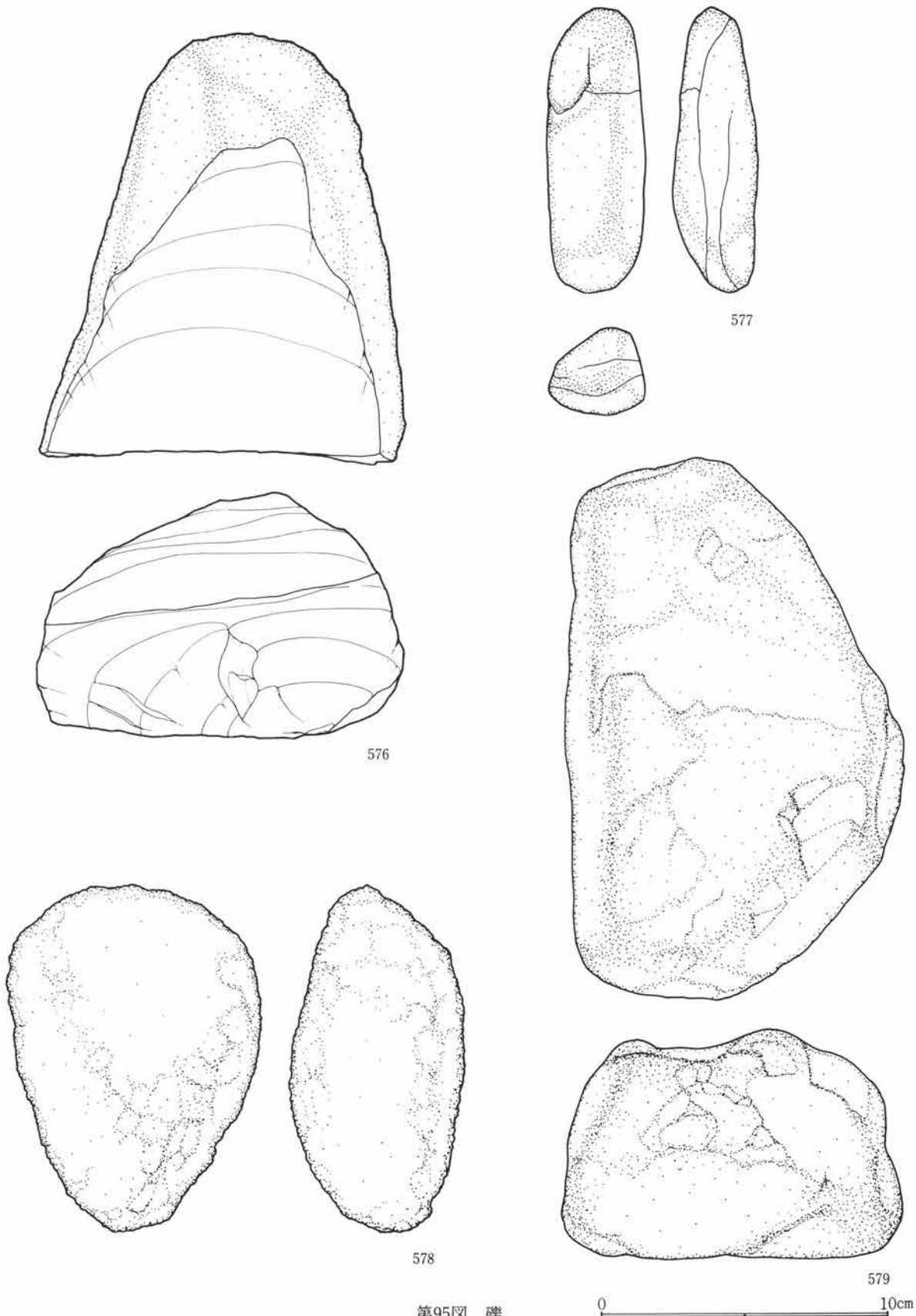
第95図 磔
