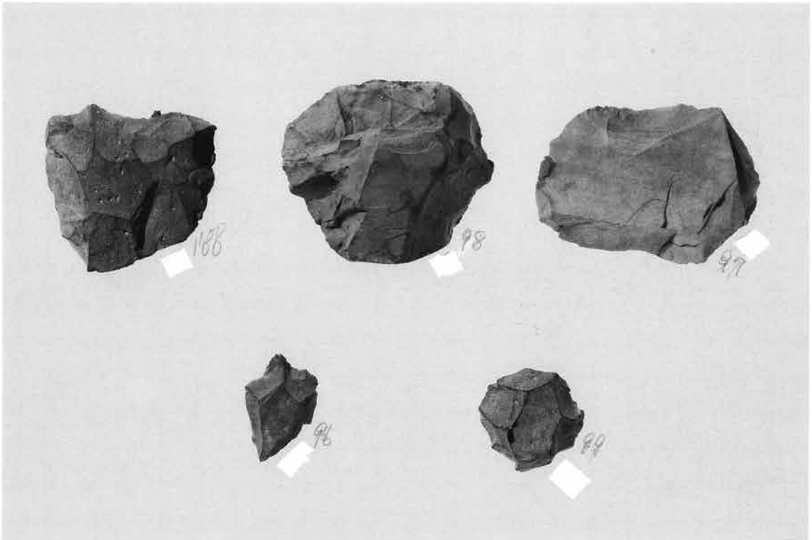
2. 石核 (7)
