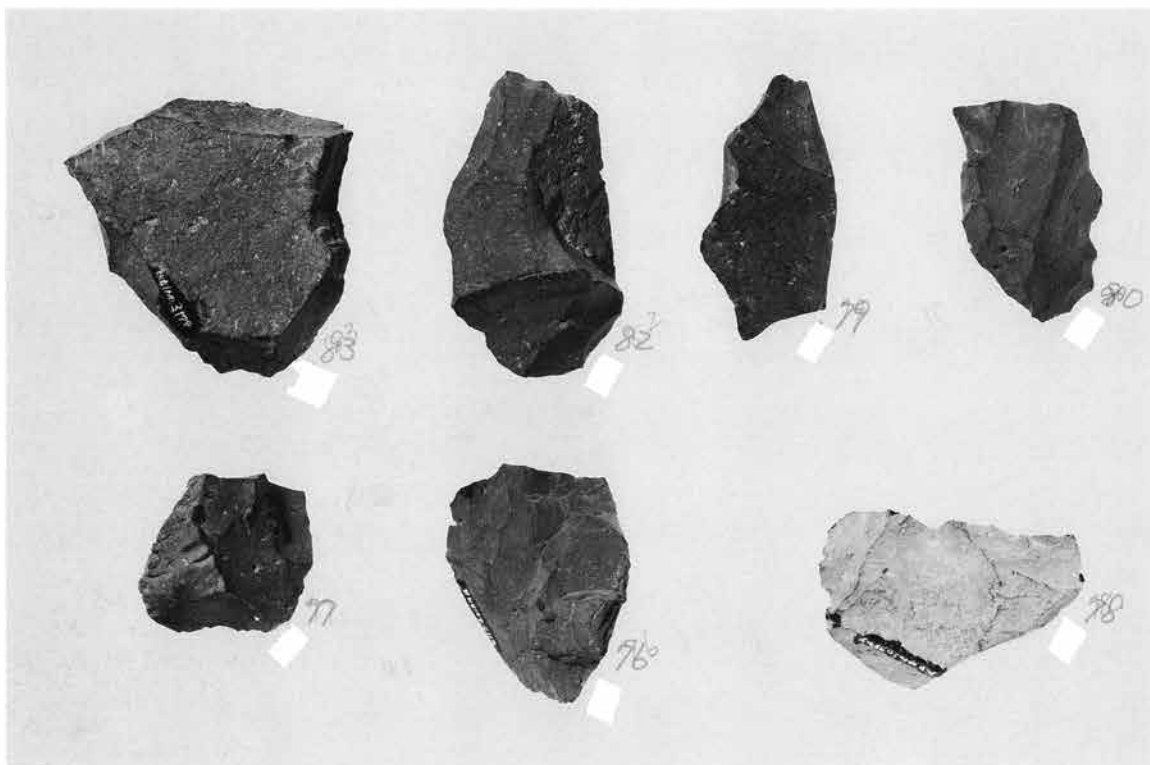
1. 石核 (4)
