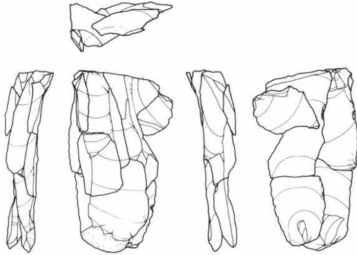
接合95 (1~7)
