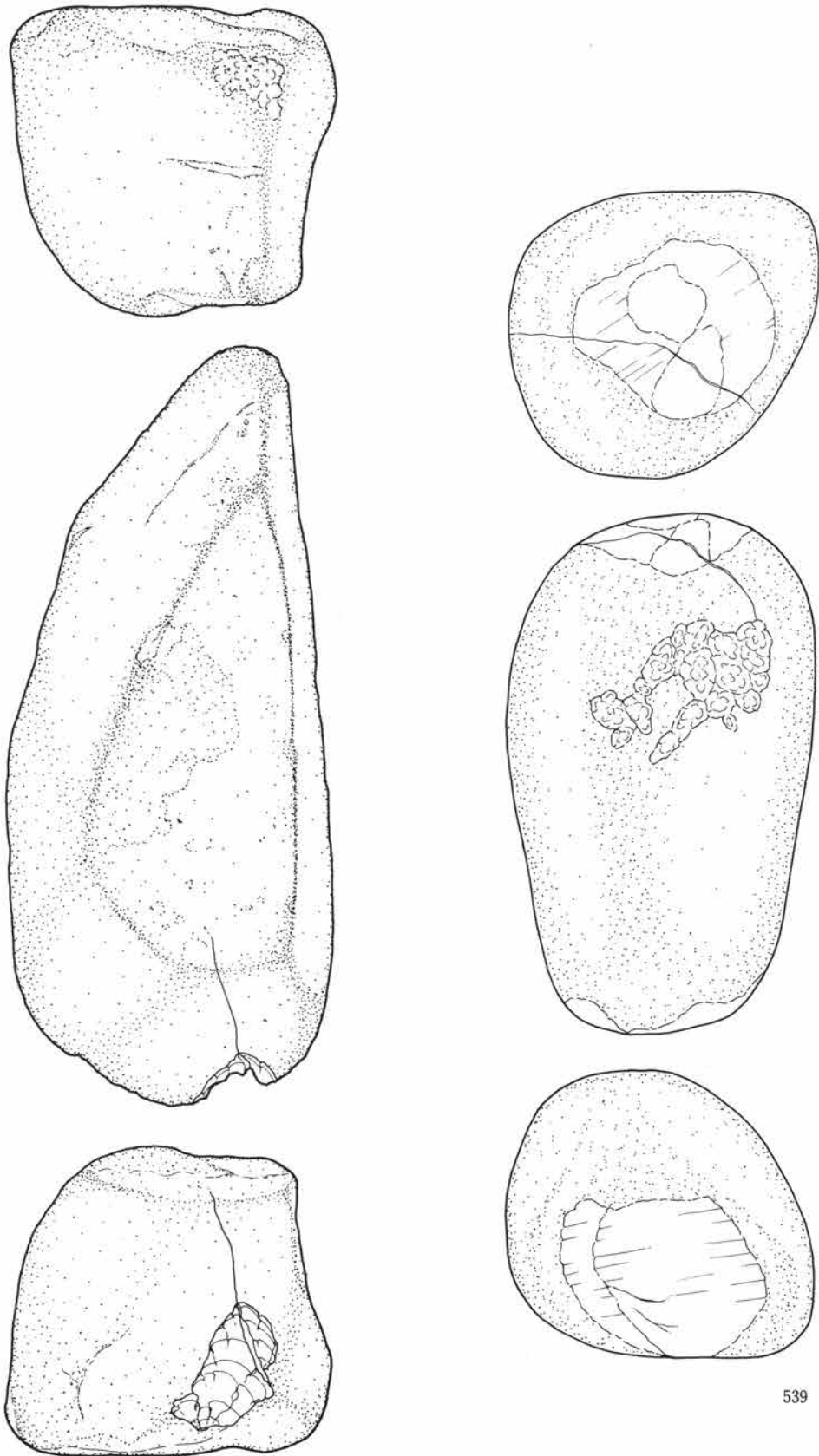
第82図 敲石 (5)
