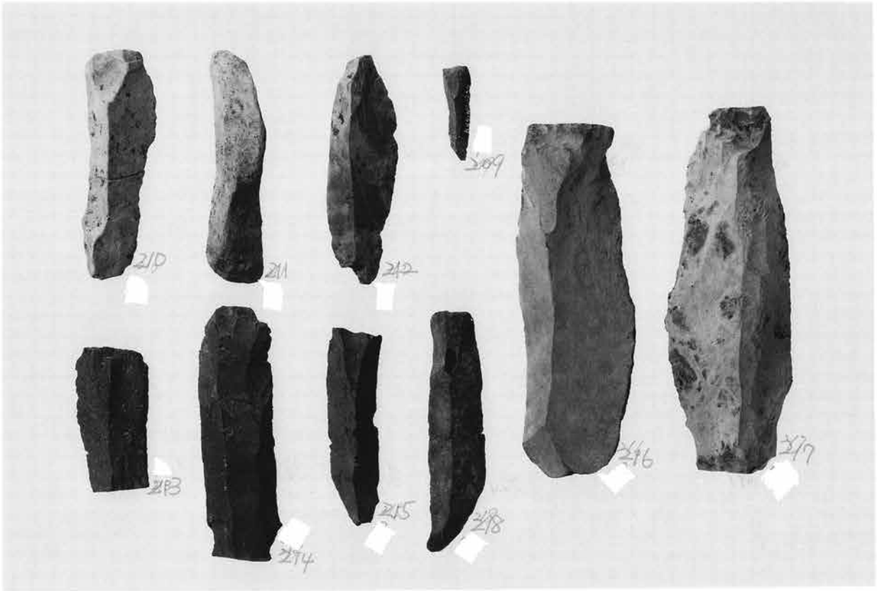
1. 石刃 (4)
