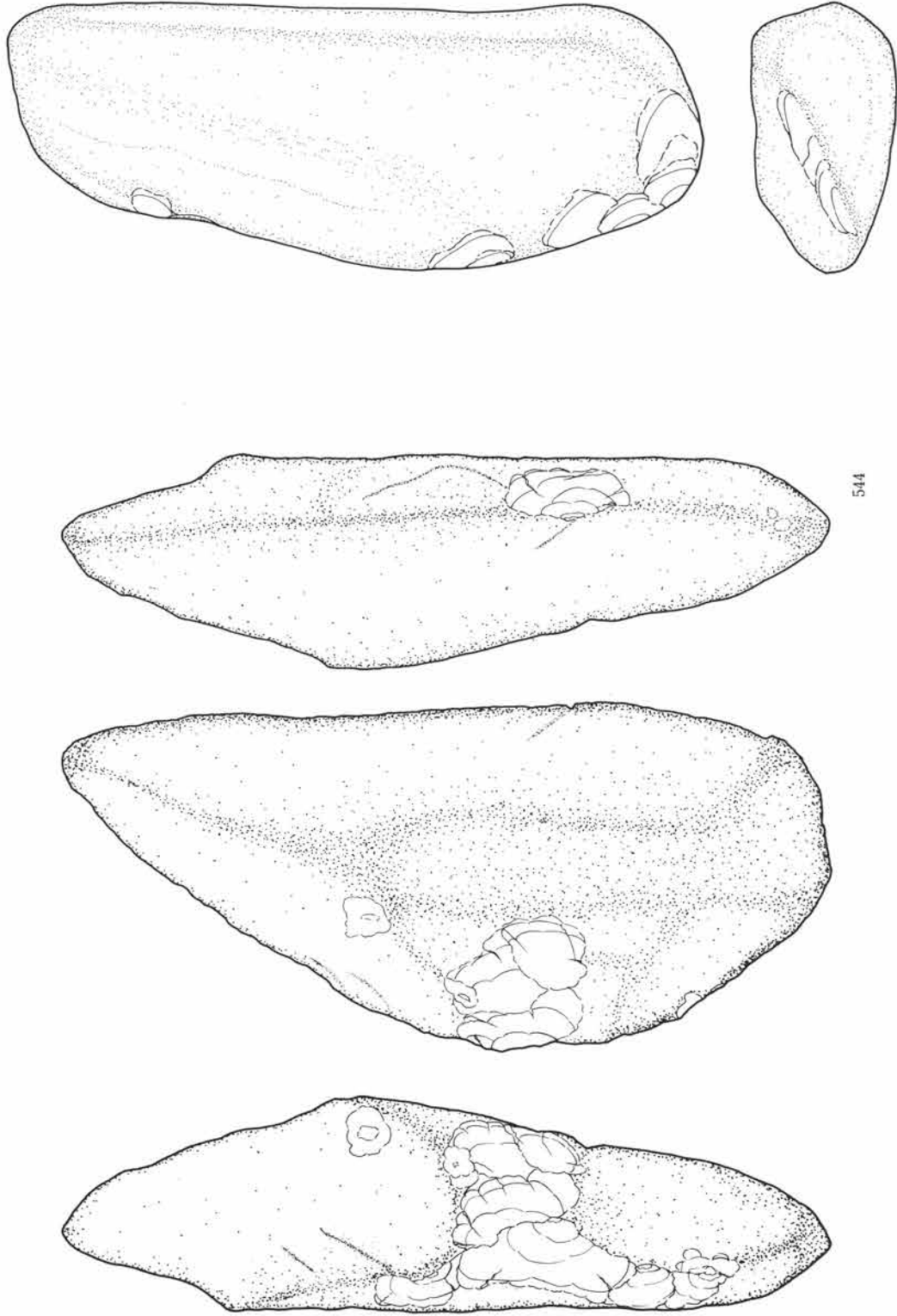
第85図 敲石 (8)
