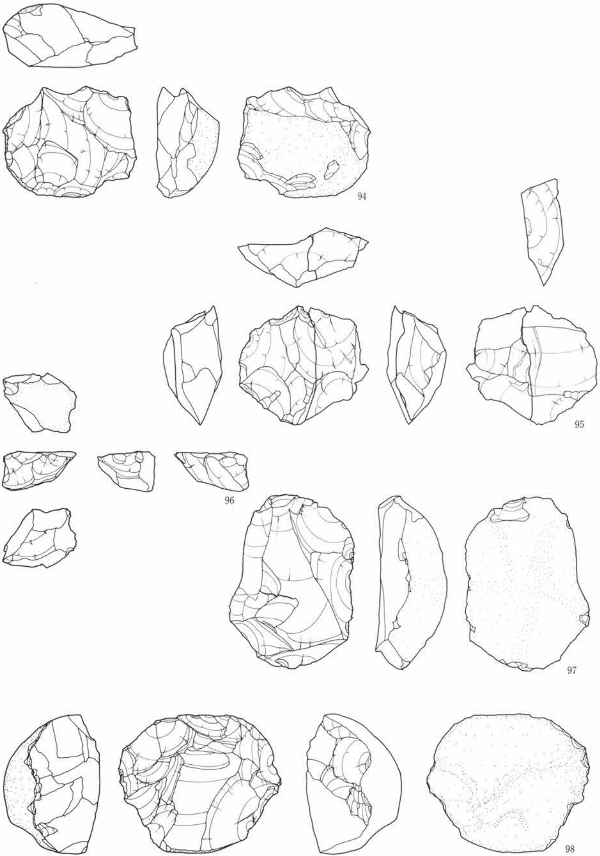
第30図 石核 (II)
