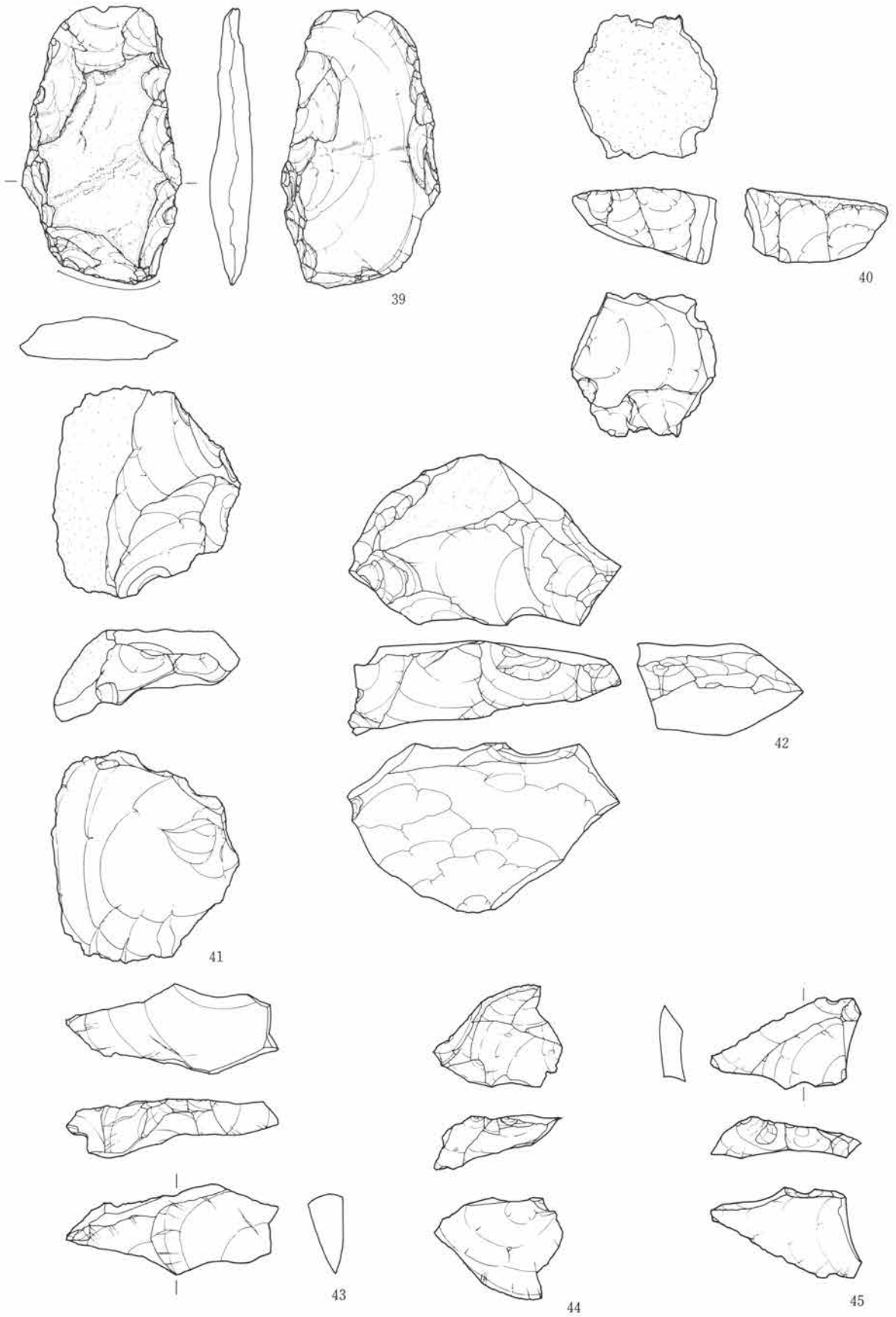
第18図 石斧・打面再生剥片
