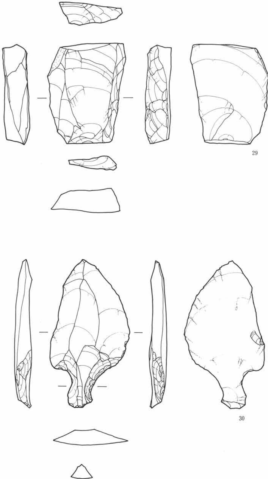
第16図 ナイフ形石器(7)
