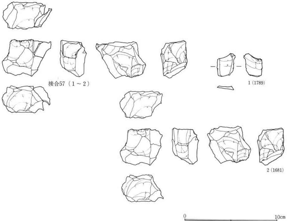
第185図 接合資料57
