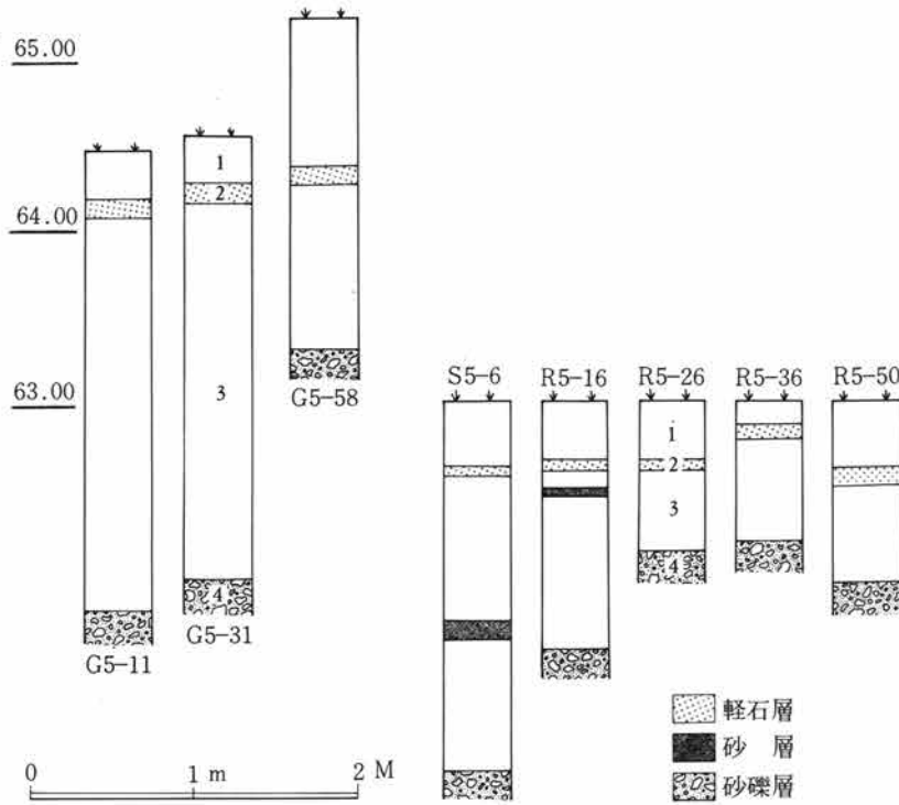
第5図 I. II区グリッド土層断面図
