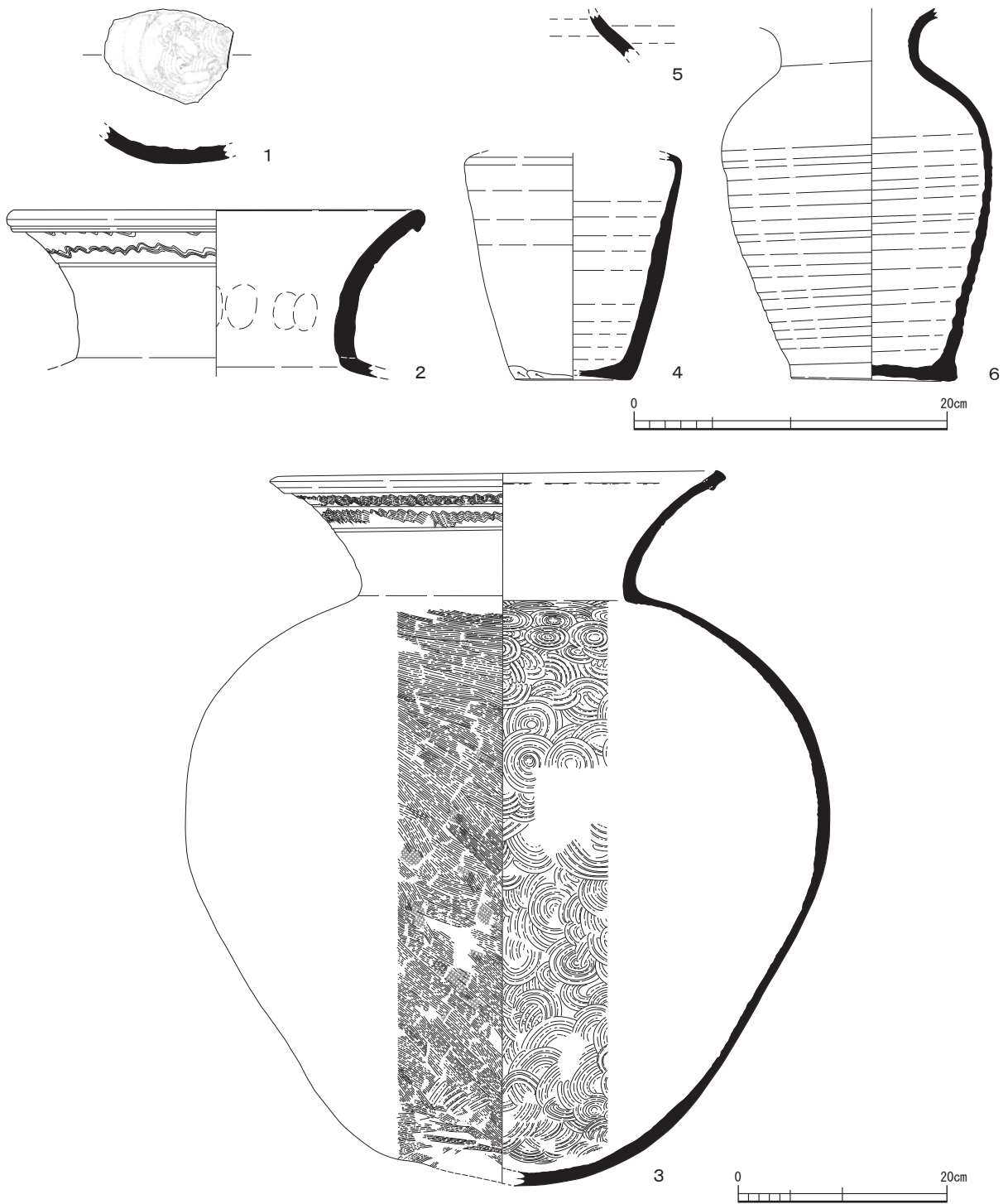
图3 土器实测图 (1 : 4 · 1 : 6)
