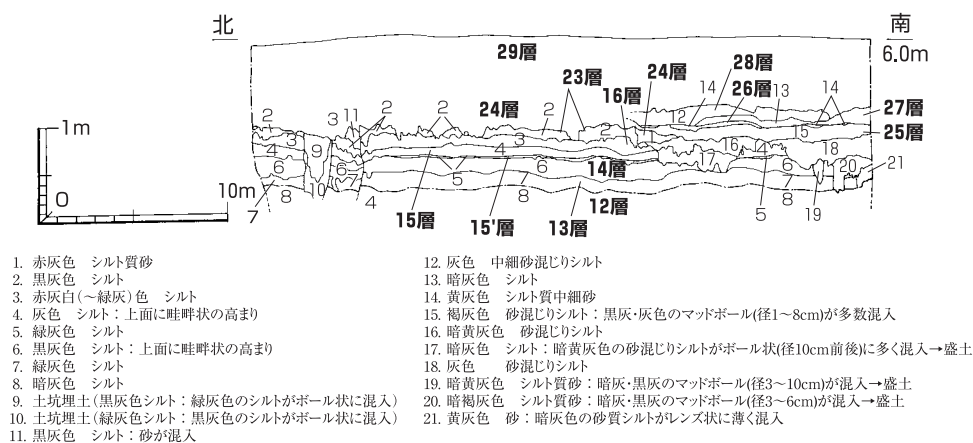
第51図 D地区東壁断面図
