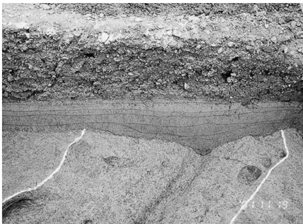
2. 2J-48-1 トレンチ 溝検出状況 (西壁)
