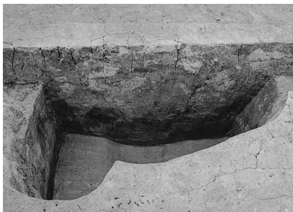
SK1013 断面 (南から)
