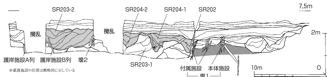
第53図 SR203土層断面と灌漑施設の位置
